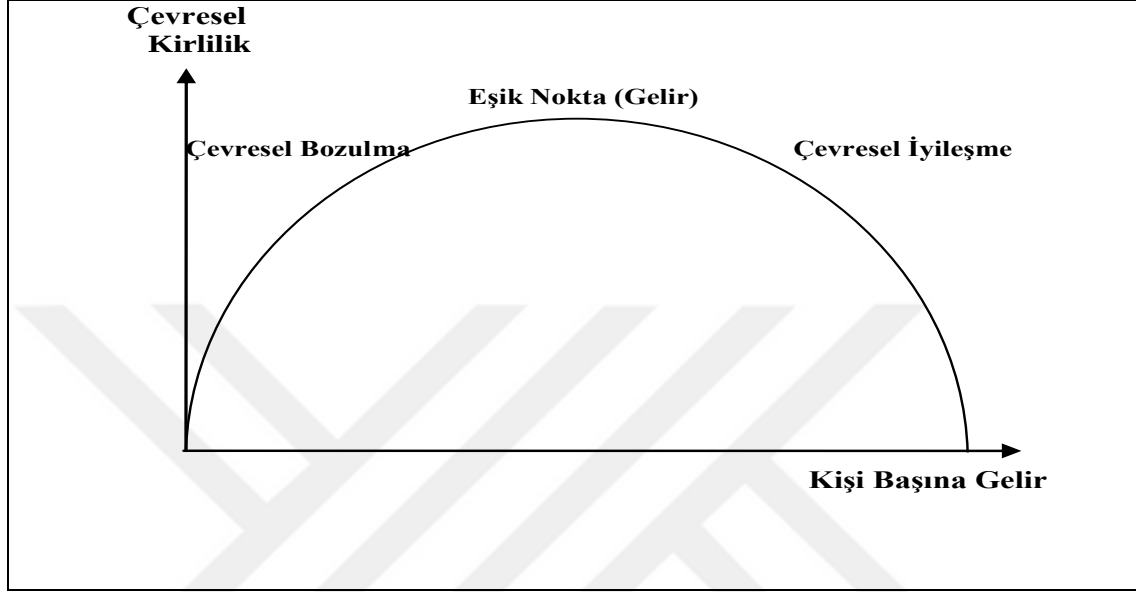
Şekil 13: Çevresel Kuznets Eğrisi Hipotezi
