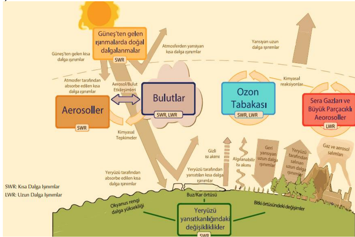
Şekil 5: Sera Etkisi
