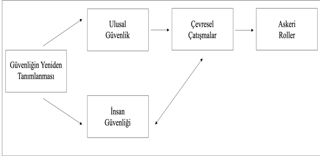
Şekil 19: Güvenlik ve İklim Değışikliğı Etkileşimi
