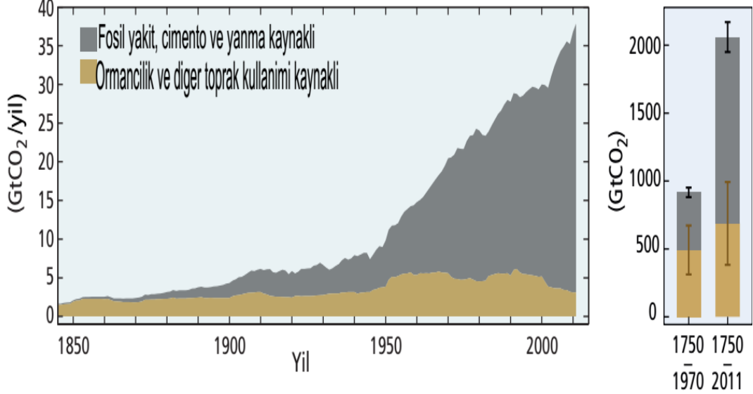
Şekil 4: İnsan Kaynaklı Küresel CO 2 Emisyonları
