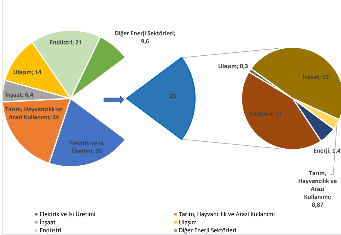
Şekil 11: Sera Gazı Emisyonlarının Sektörlere Göre Dağılımı (2014)
