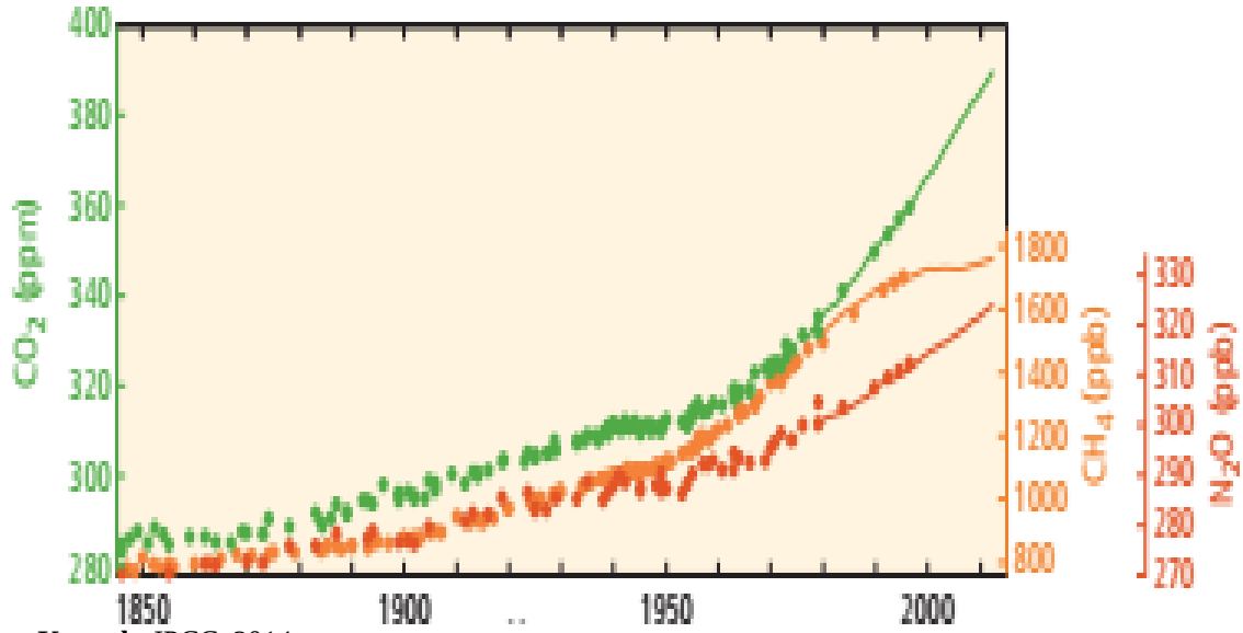
Şekil 3 Küresel Sera Gazları Yoğunluğundaki Değişmeler (1850-2000)
