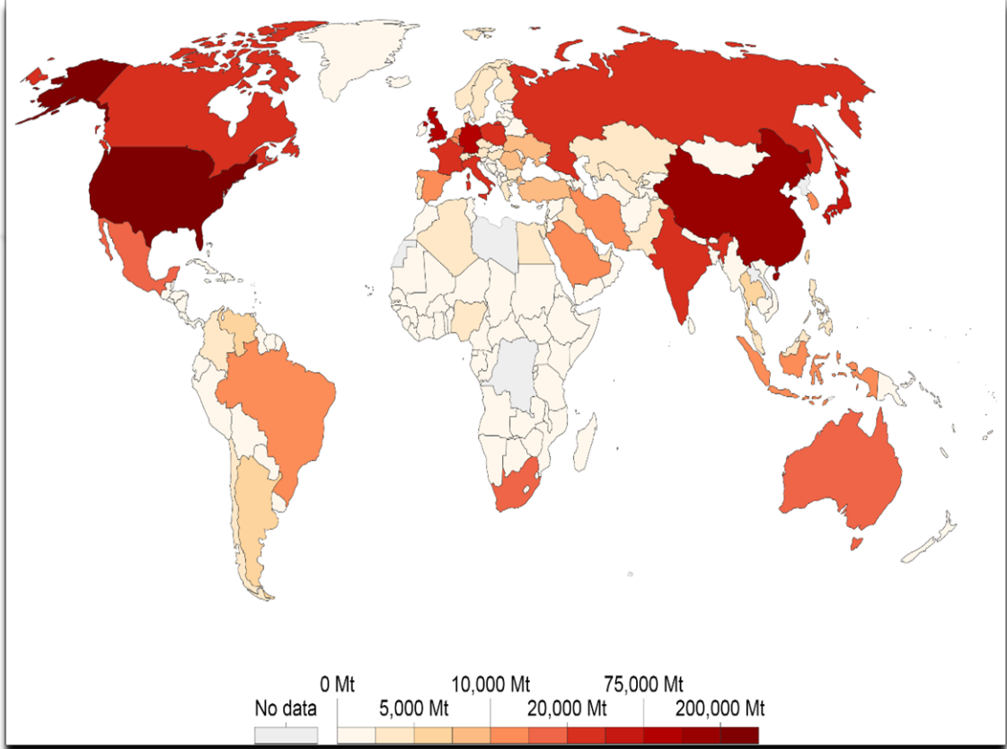
Şekil 16: Ülkelerin Kümülatif CO 2 Emisyonu Miktarları (1750-2014, milyon ton)
