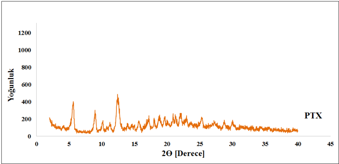
Şekil 5.17. (Devam) Kollidon® SR ile hazırlanan nanopartiküllerin ve kullanılan saf maddelerin x-ışını kırınım analiz difraktogramları
