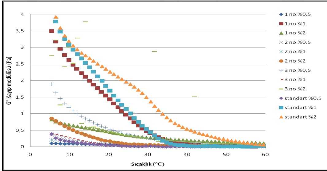
Şekil 4.8 Xanthomonas izolatları ve standart X. campestris DSM 19000 suşundan elde edilen ksantan gamların 5-60 °C aralığındaki birikim ve kayıp modülü eğrileri (1 no- X. hortorum pv. pelargonii , 2 no- X. axonopodis pv. begoniae , 3 no- X. axonopodis pv. vesicatoria izolatı Standart ise X. campestris DSM 19000 suşundan elde edilen gama aittir )
