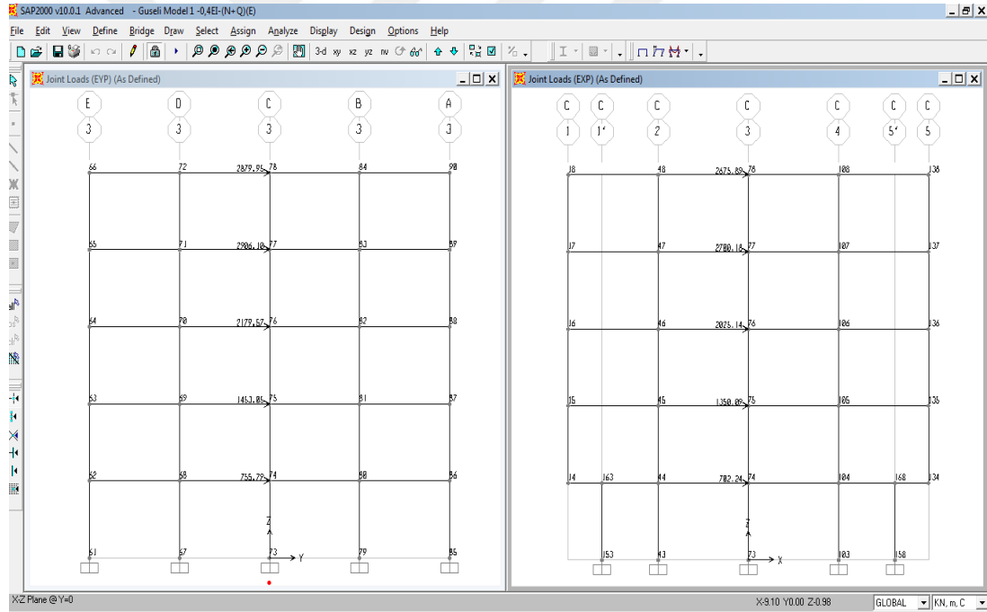
Şekil 4.45 : B2 binası, SAP2000 katlara etkiyen eşdeğer deprem yükleri.
