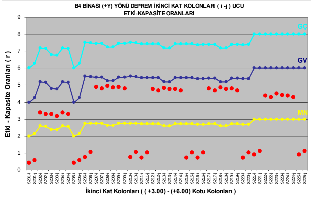
Şekil 4.83 : B4 binası (+Y) yönü deprem durumu, ikinci kat kolonları, (i – j ucu) kolon hasar durum grafiği.
