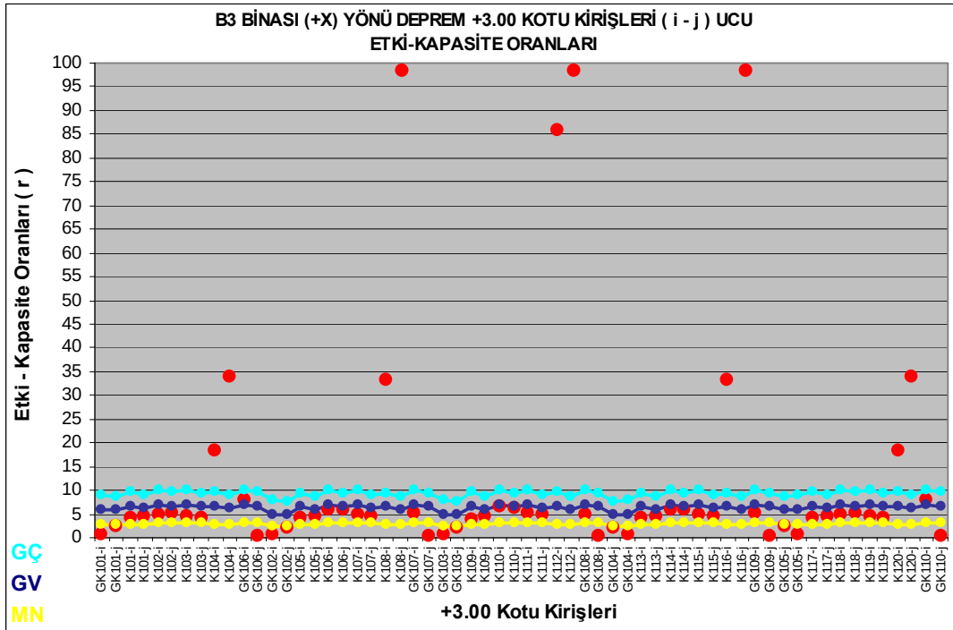
Şekil 4.62 : B3 binası (+X) yönü deprem durumu, +3.00 kotu kirişleri, (i – j ucu) kiriş hasar durum grafiği.
