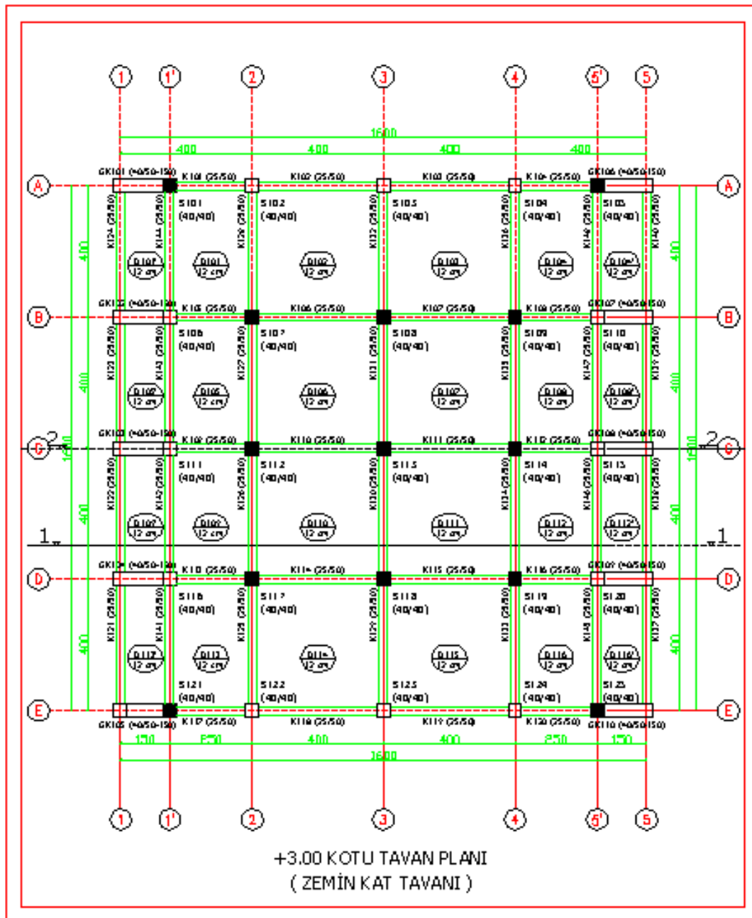
Şekil 4.54 : B3 binası +3.00 kotu kalıp planı.
