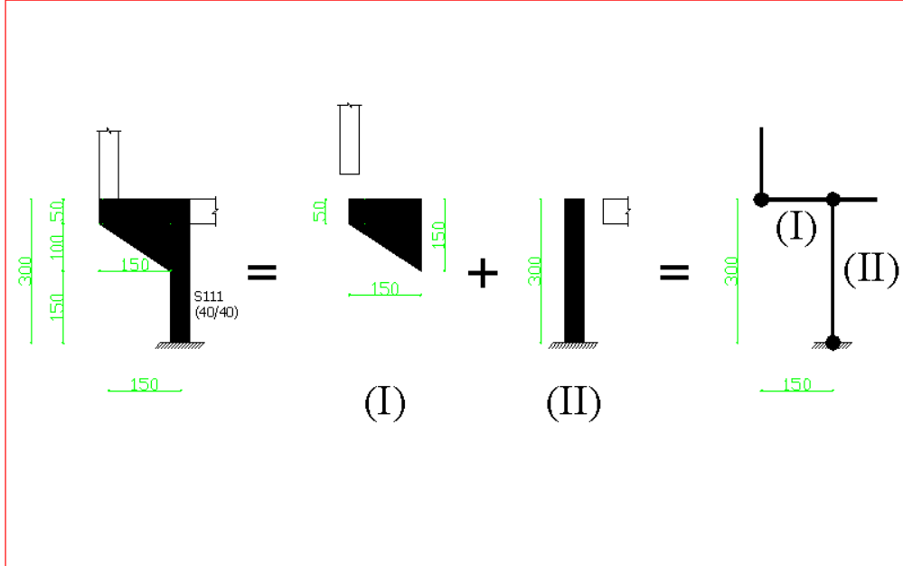
Şekil 4.57 : Guseli kolon modellemesi.
