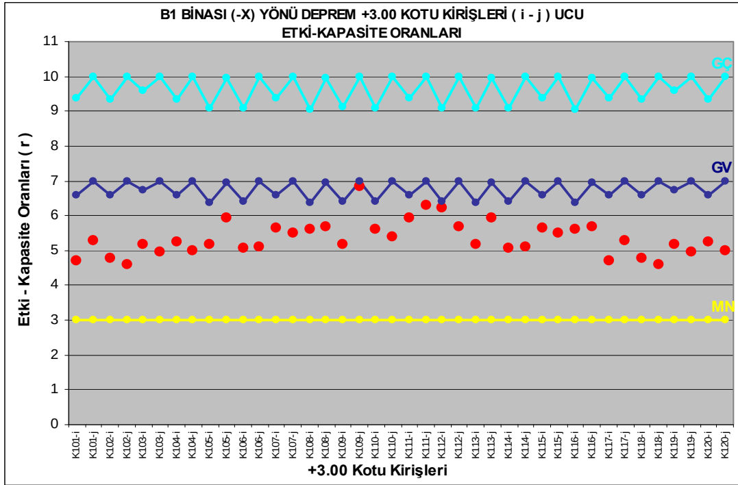
Şekil 4.22 : B1 binası (-X) yönü deprem durumu, +3.00 kotu kirişleri, (i - j ucu) kiriş hasar durum grafiği.
