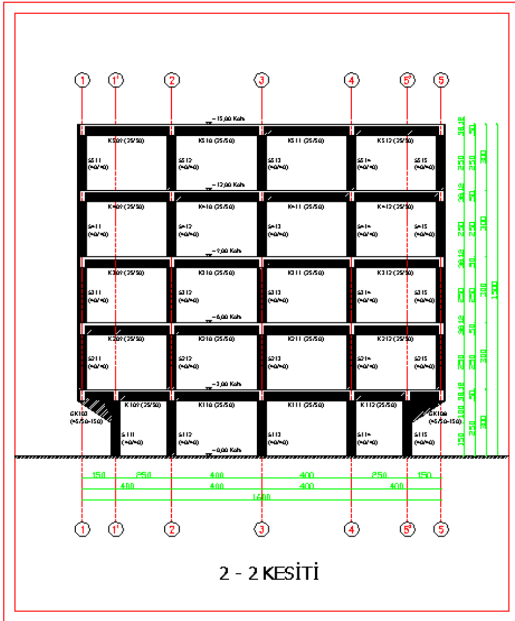
Şekil 4.56 : B3 binası 2-2 boyuna kesiti.
