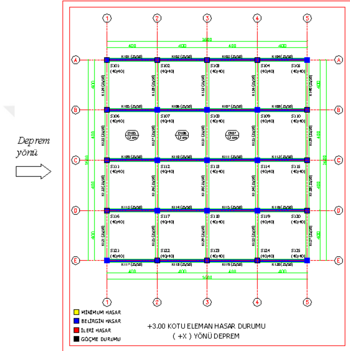
Şekil 4.38 : B1 binası (+X) yönü deprem eleman hasar durumu.
