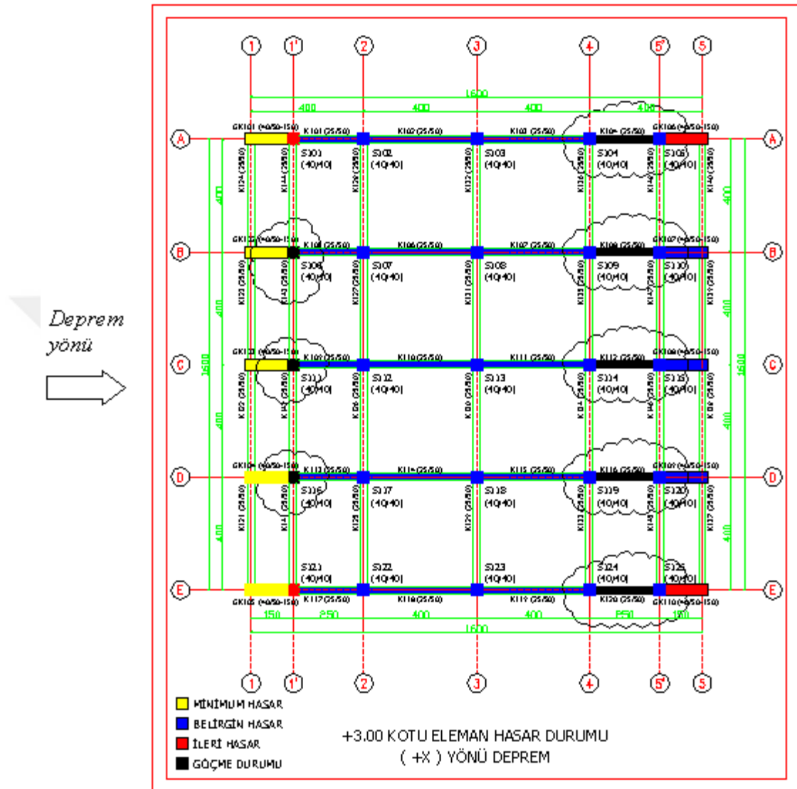
Şekil 4.68 : B3 binası (+X) yönü deprem eleman hasar durumu.
