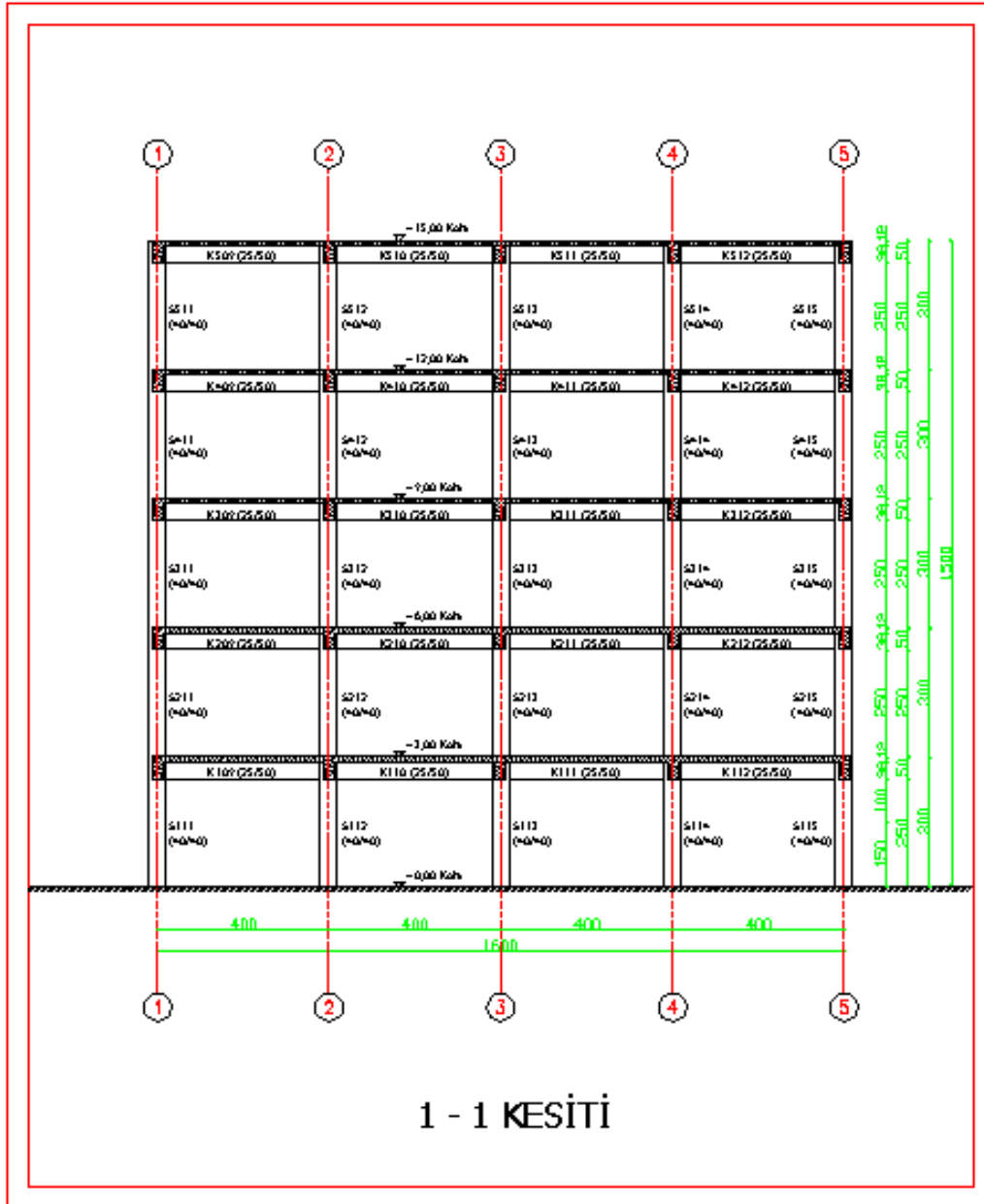
Şekil 4.3 : B1 binası 1-1 boyuna kesiti.
