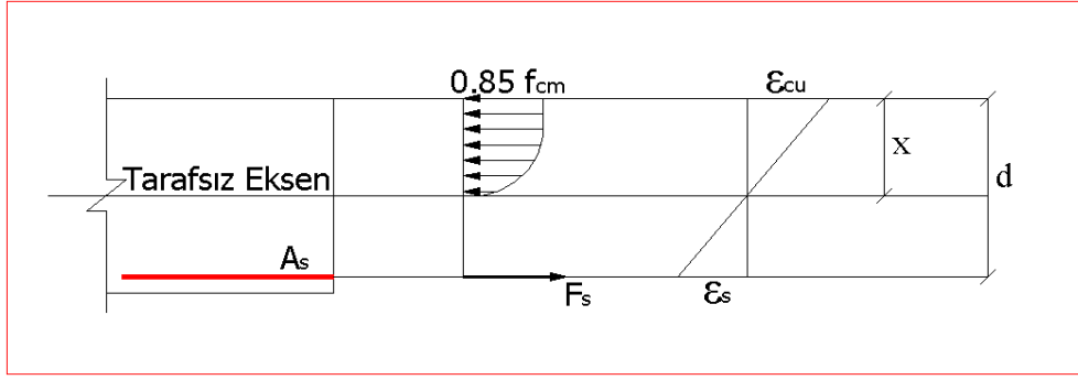
Şekil 4.19 : Kiriş kesiti dengeli durumu.
