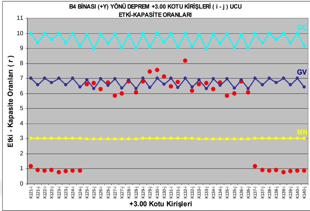
Şekil 4.79 : B4 binası (+Y) yönü deprem durumu, +3.00 kotu kirişleri, (i – j ucu) kiriş hasar durum grafiği.
