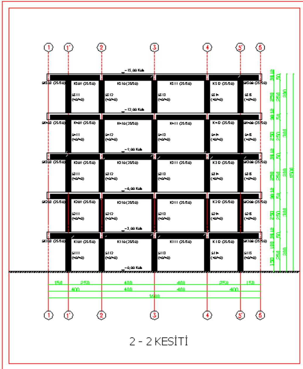
Şekil 4.72 : B4 binası 2-2 boyuna kesiti.
