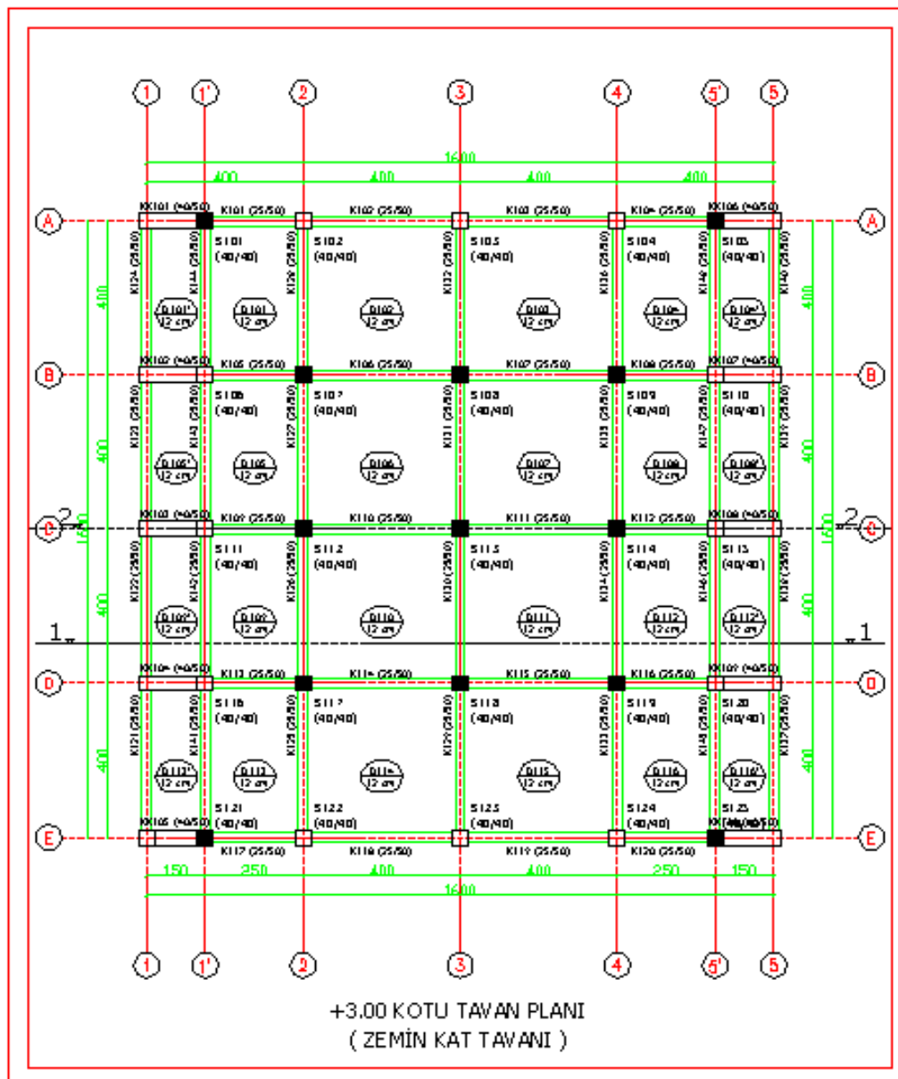
Şekil 4.39 : B2 binası +3.00 kotu kalıp planı.
