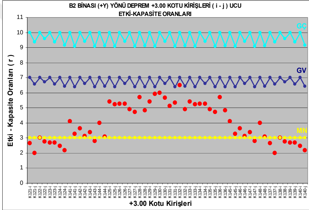
Şekil 4.47 : B2 binası (+Y) yönü deprem durumu, +3.00 kotu kirişleri, (i – j ucu) kiriş hasar durum grafiği.
