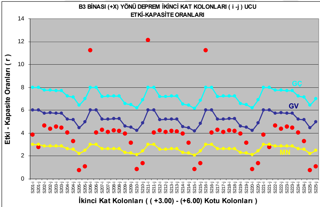
Şekil 4.65 : B3 binası (+X) yönü deprem durumu, ikinci kat kolonları, (i – j ucu) kolon hasar durum grafiği.
