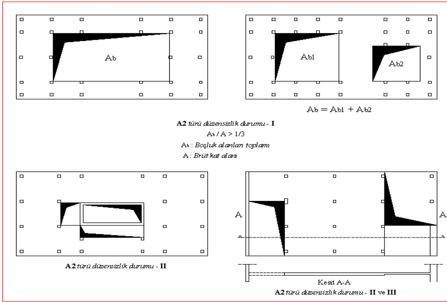
Şekil 3.2 : A2 – döşeme süreksizliği - ( TDY-07, Şekil 2.2).
