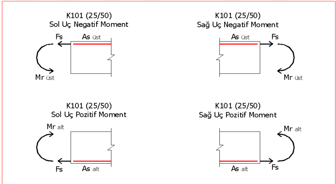
Şekil 4.16 : Kiriş kapasite momenti.
