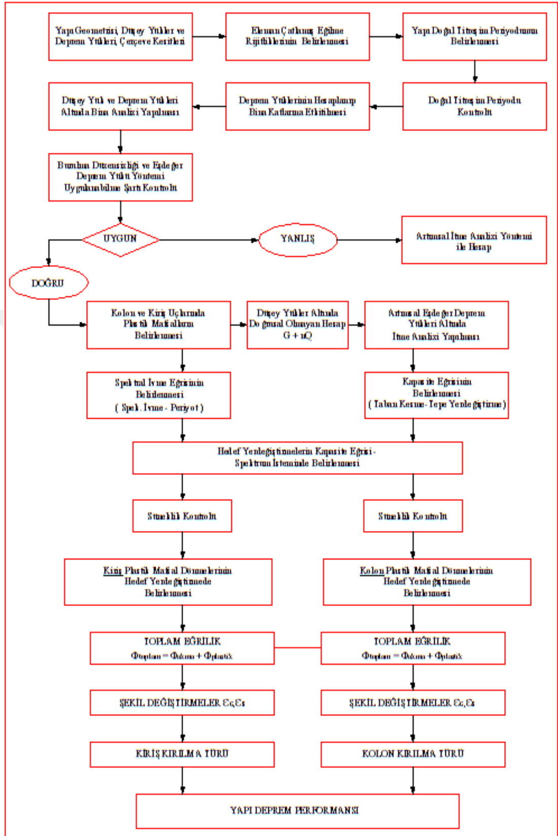
Şekil 2.2 : Doğrusal olmayan hesap yöntemi akış diyagramı.
