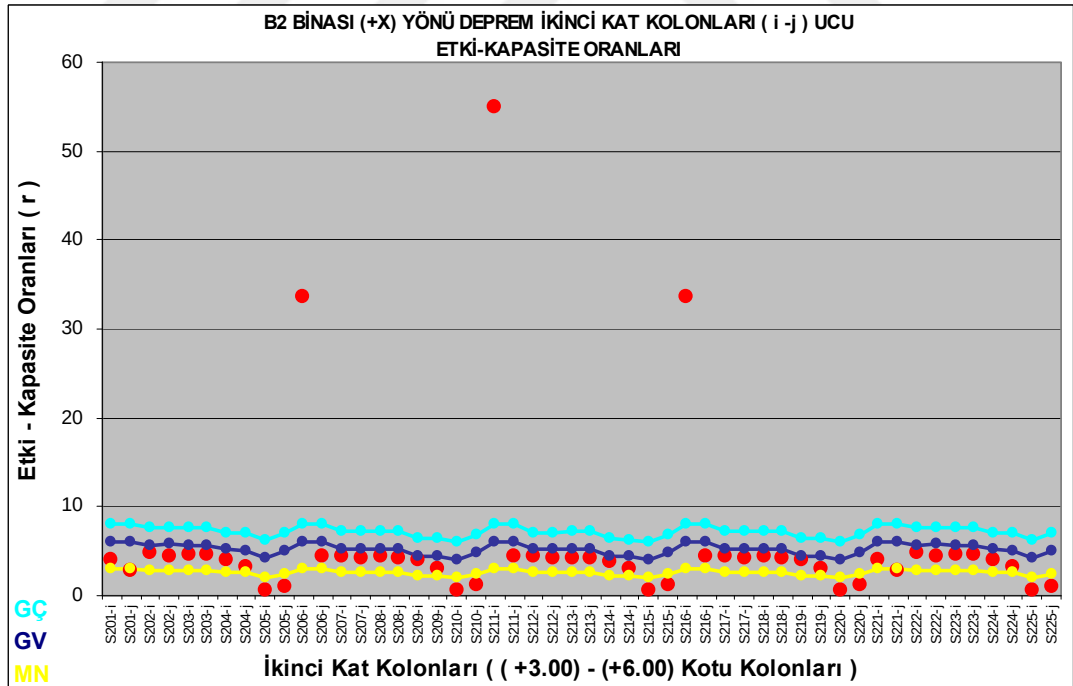
Şekil 4.49 : B2 binası (+X) yönü deprem durumu, ikinci kat kolonları, (i – j ucu) kolon hasar durum grafiği.
