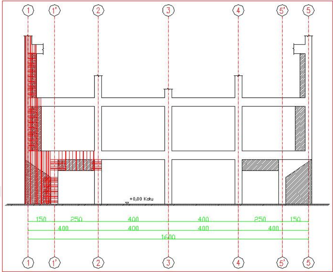
Şekil 6.1: Düşey doğrultuda süreksizlik taşıyan ve çıkmaların bulunduğu yapılar için şematik güçlendirme önerisi.
