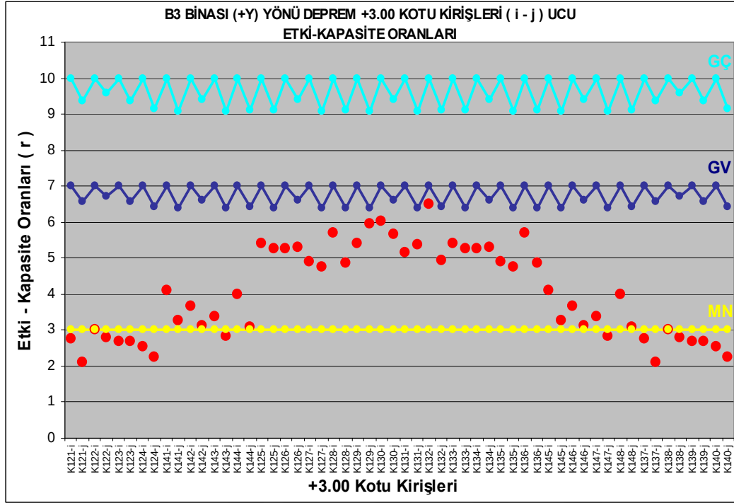
Şekil 4.63 : B3 binası (+Y) yönü deprem durumu, +3.00 kotu kirişleri, (i – j ucu) kiriş hasar durum grafiği.
