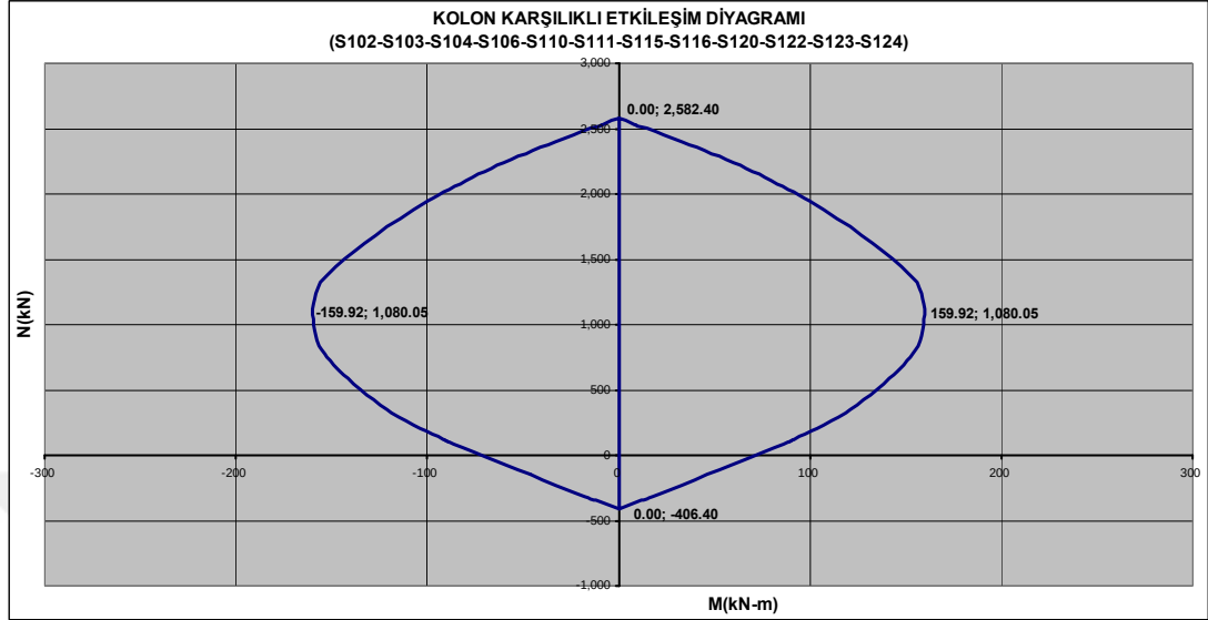
Şekil 4.28 : S102 ve benzer kolonların karşılıklı etkileşim diyagramı.
