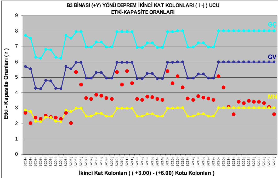
Şekil 4.67 : B3 binası (+Y) yönü deprem durumu, ikinci kat kolonları, ( i – j ucu) kolon hasar durum grafiği.
