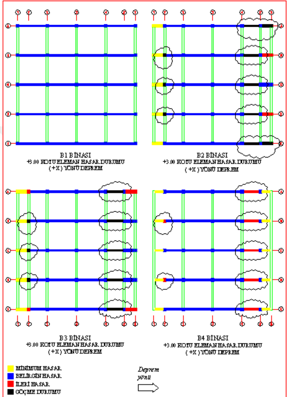
Şekil 5.1 : B1, B2, B3 ve B4 binaları, (+X) yönü deprem, birinci kat planları, eleman hasar durum karşılaştırması.
