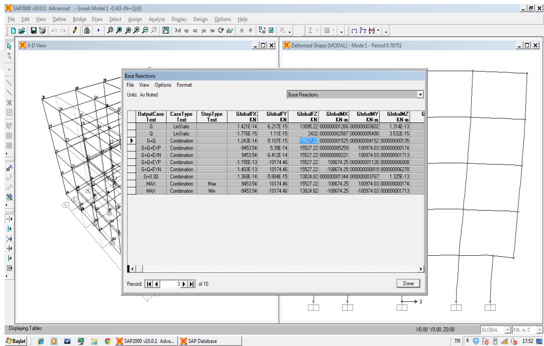
Şekil 4.43 : B2 binası SAP2000 mesnet reaksiyonları.
