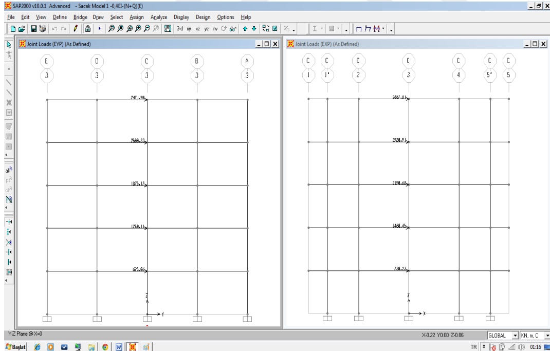
Şekil 4.77 : B4 binası, SAP2000 katlara etkiyen eşdeğer deprem yükleri.
