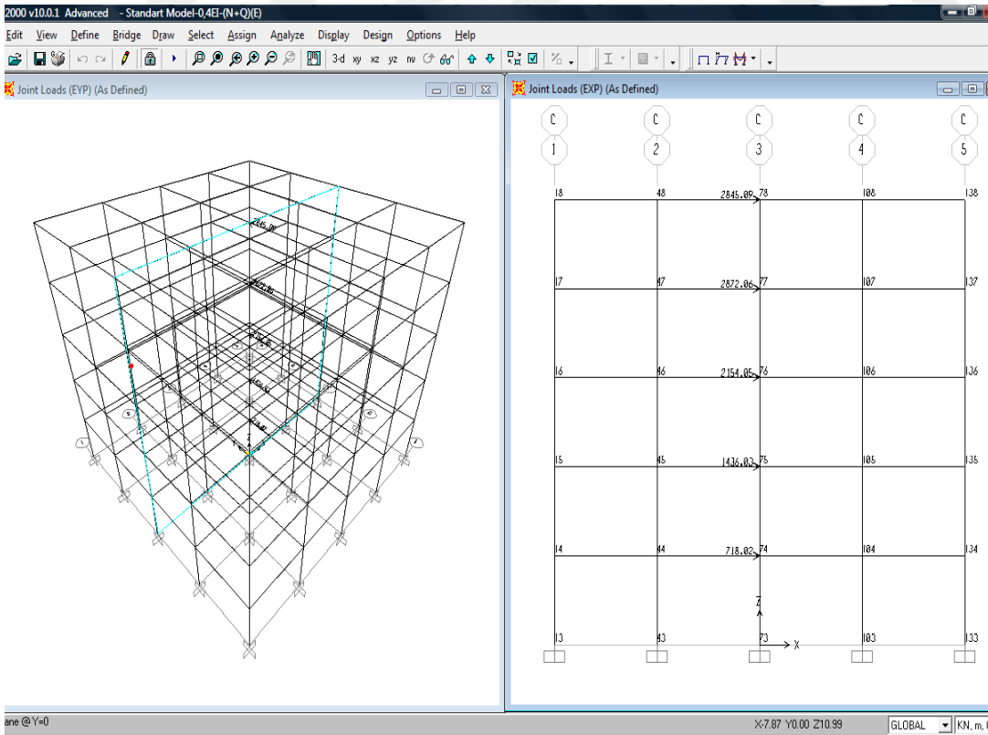
Şekil 4.13 : B1 binası, SAP2000 katlara etkiyen eşdeğer deprem yükleri.
