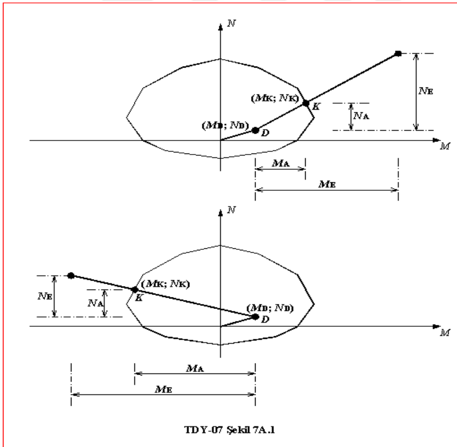
Şekil 4.29 : Moment – eksenel kuvvet etkileşim diyagramı ile moment ve normal kuvvet kapasitelerinin belirlenmesi ( TDY-07, Bilgilendirme Eki 7.A).
