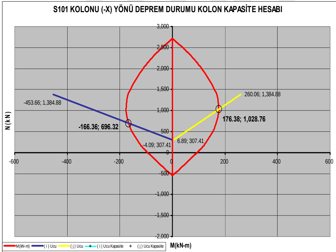
Şekil 4.31 : S101 kolonu (-X) yönü deprem durumu kolon kapasite hesabı.
