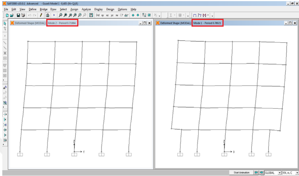
Şekil 4.60 : B3 binası SAP2000 (X) ve (Y) yönü bina doğal titreşim periyotları.
