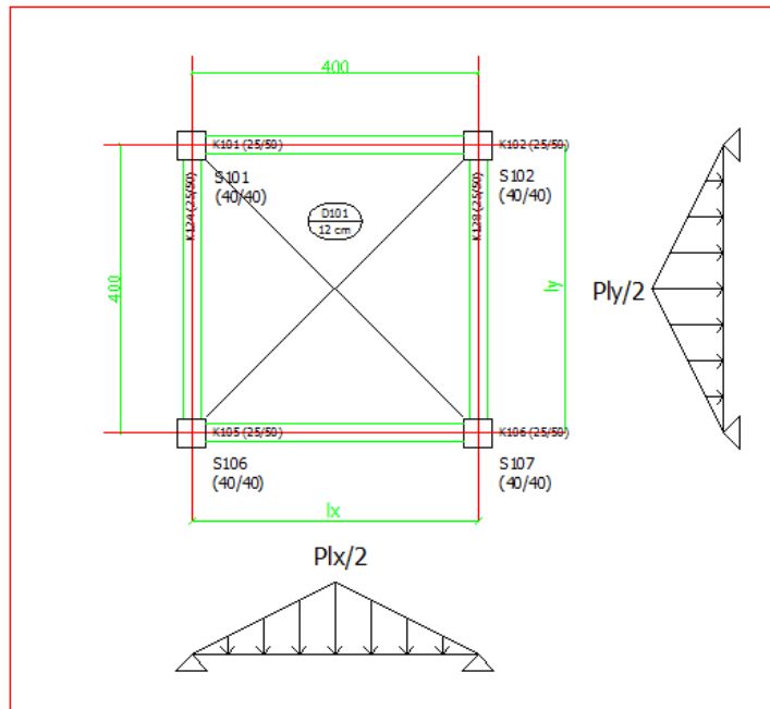
Şekil 4.6 : B1 binası döşeme yük dağılımı.
