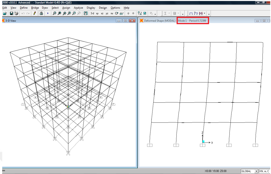
Şekil 4.12 : B1 binası SAP2000 bina birinci doğal titreşim periyodu.
