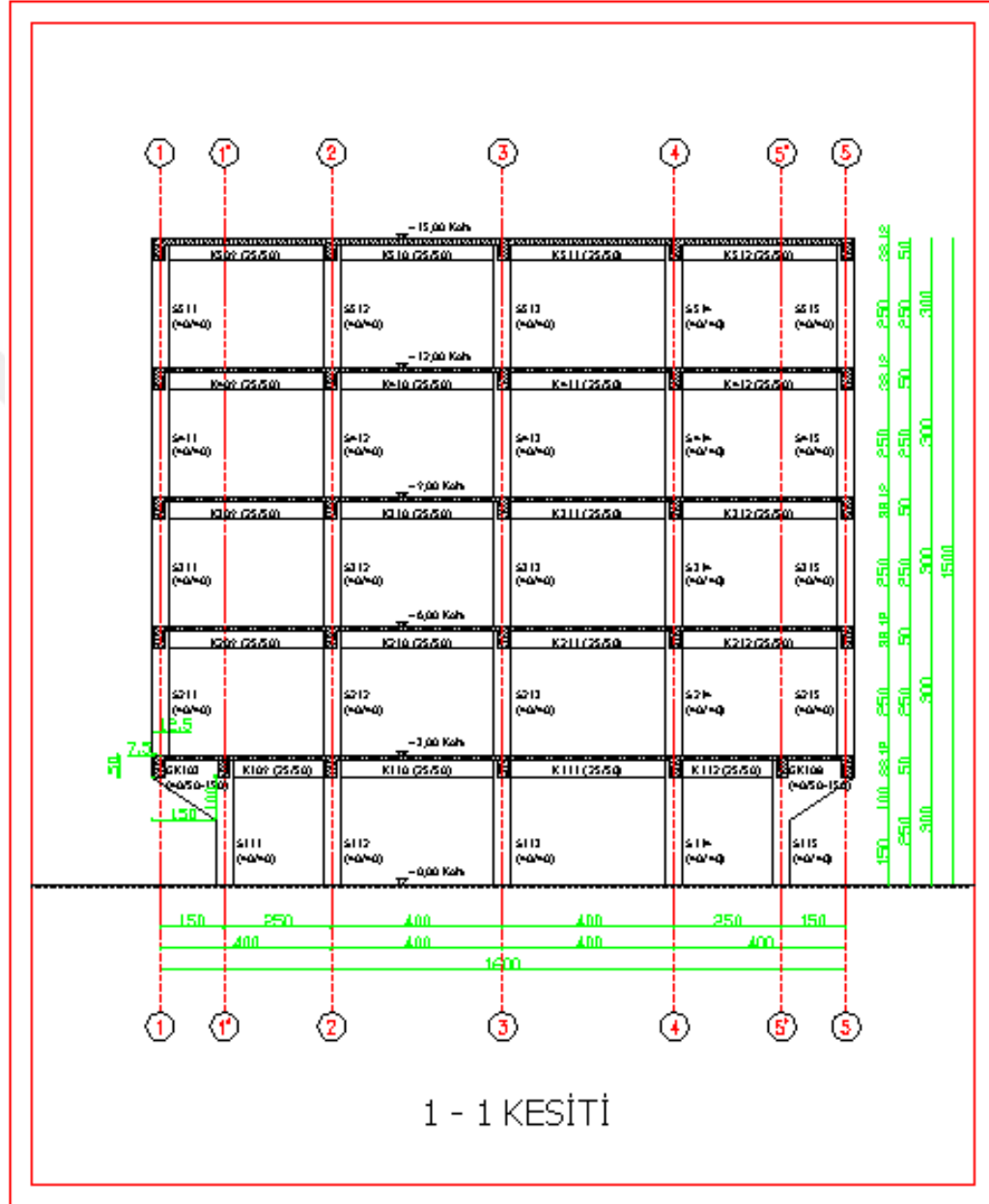
Şekil 4.55 : B3 binası 1-1 boyuna kesiti.
