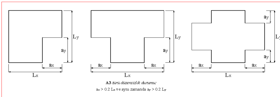
Şekil 3.3 : A3 – planda çıkıntılar bulunması - ( TDY-07, Şekil 2.3).
