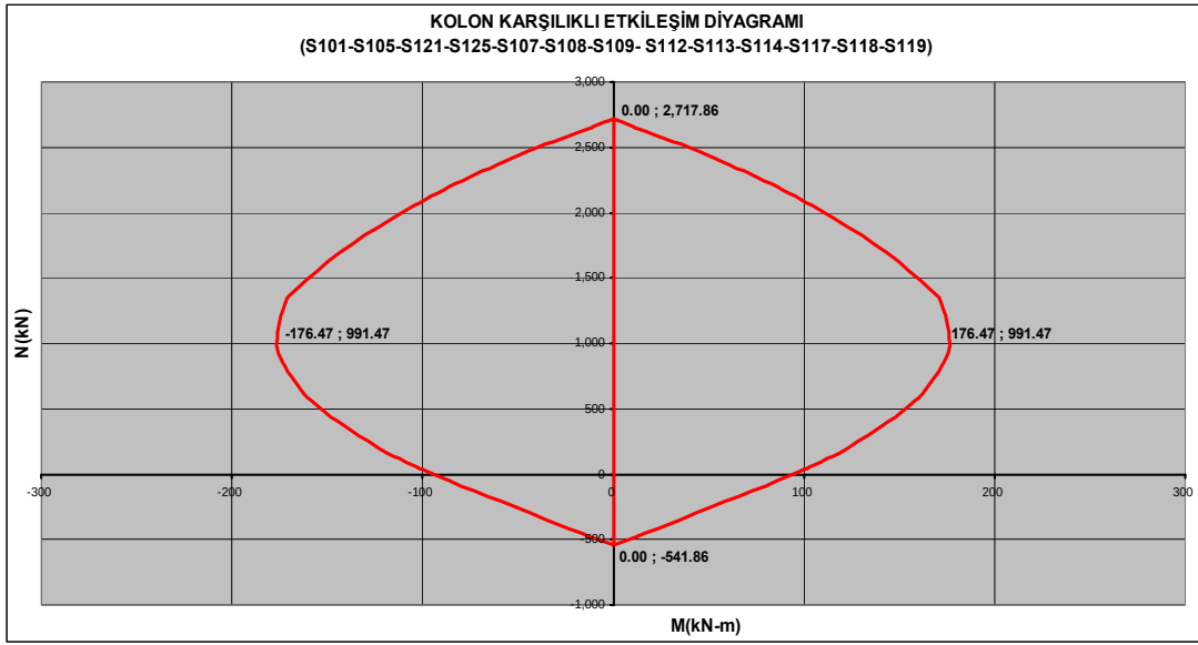
Şekil 4.27 : S101 ve benzer kolonların karşılıklı etkileşim diyagramı.
