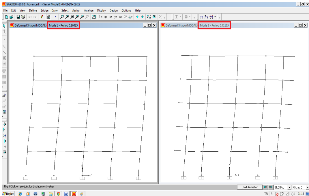
Şekil 4.76 : B4 binası SAP2000 (X) ve (Y) yönü bina doğal titreşim periyotları.
