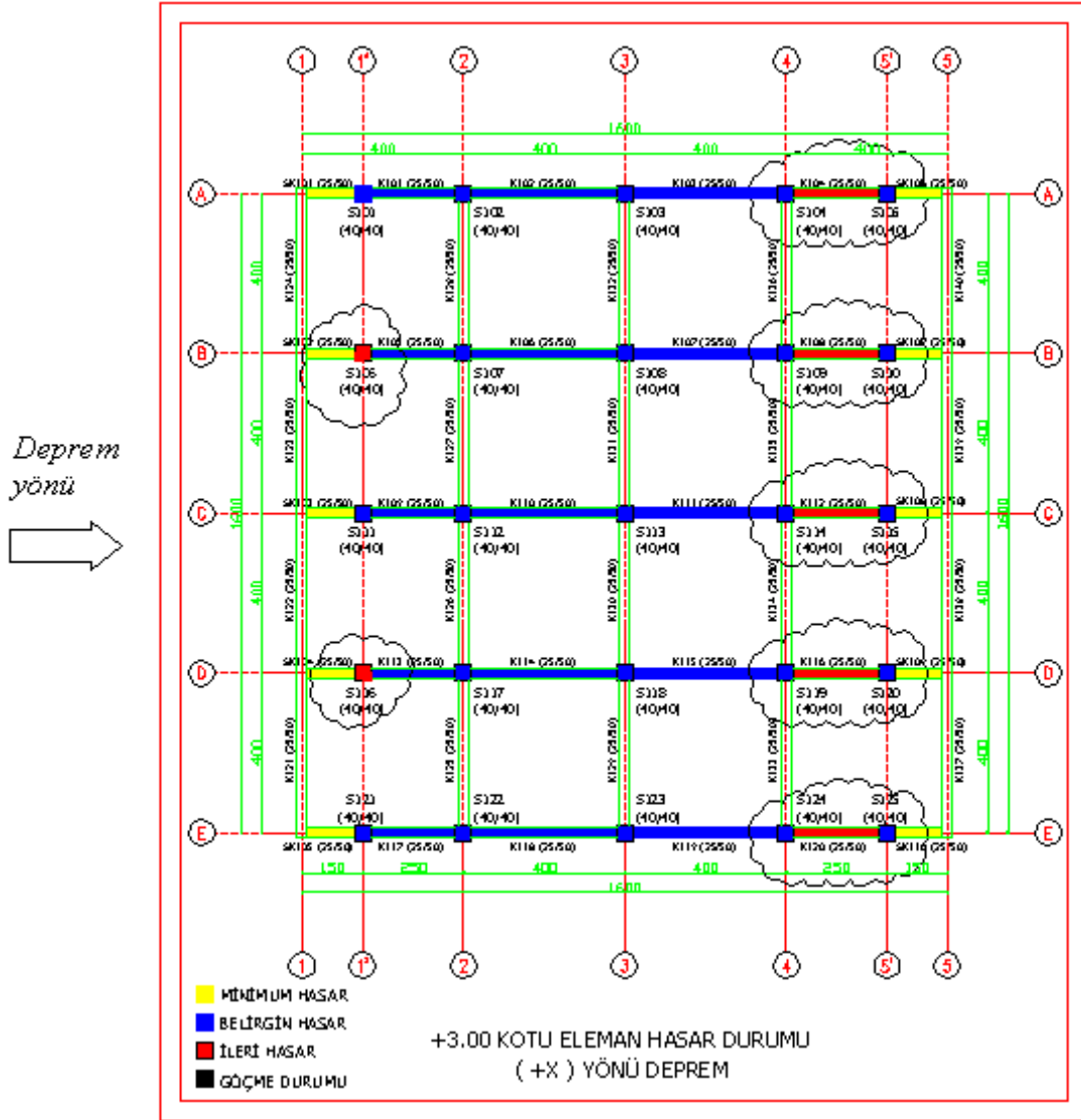
Şekil 4.84 : B4 binası (+X) yönü deprem eleman hasar durumu.
