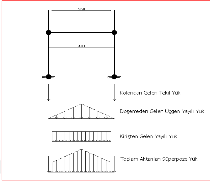
Şekil 4.8 : B1 binası süperpoze yük şematik gösterimi.
