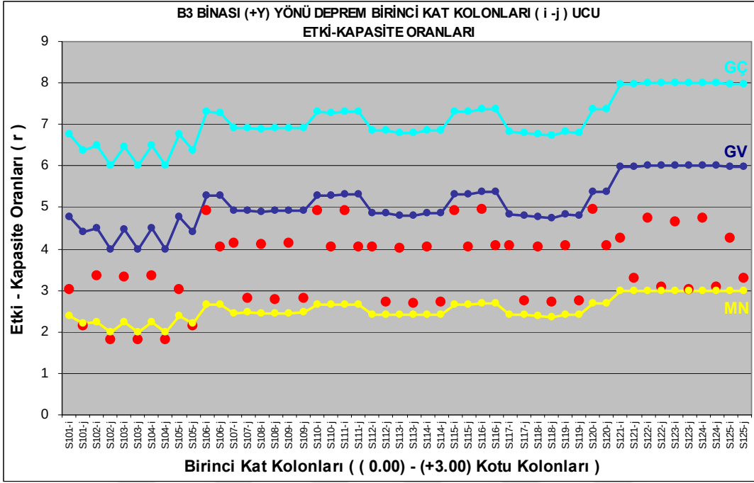
Şekil 4.66 : B3 binası (+Y) yönü deprem durumu, birinci kat kolonları, ( i – j ucu) kolon hasar durum grafiği.
