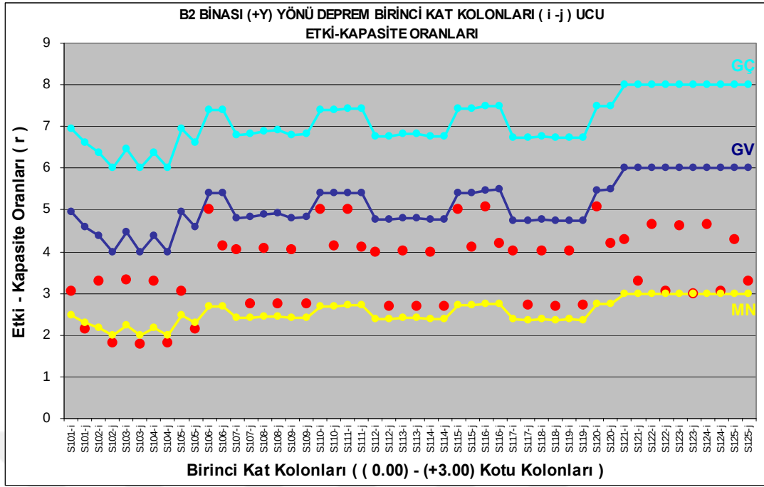
Şekil 4.50 : B2 binası (+Y) yönü deprem durumu, birinci kat kolonları, ( i – j ucu ) kolon hasar durum grafiği.
