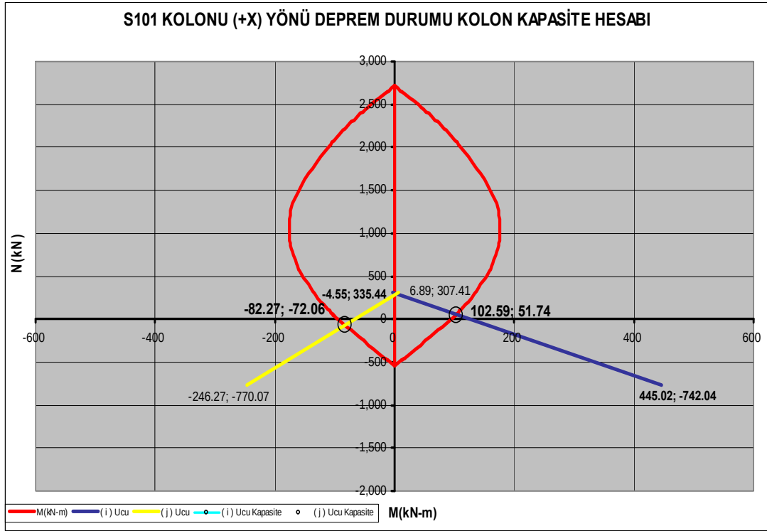
Şekil 4.30 : S101 kolonu (+X) yönü deprem durumu kolon kapasite hesabı.
