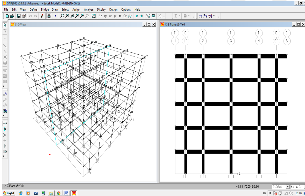
Şekil 4.73 : B4 binası SAP2000 modeli.
