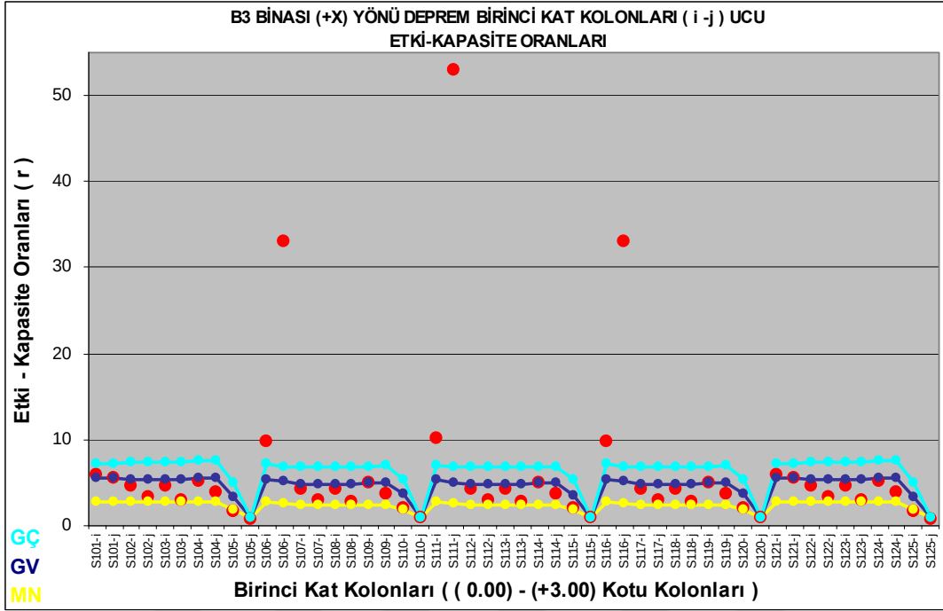
Şekil 4.64 : B3 binası (+X) yönü deprem durumu, birinci kat kolonları, (i – j ucu) kolon hasar durum grafiği.
