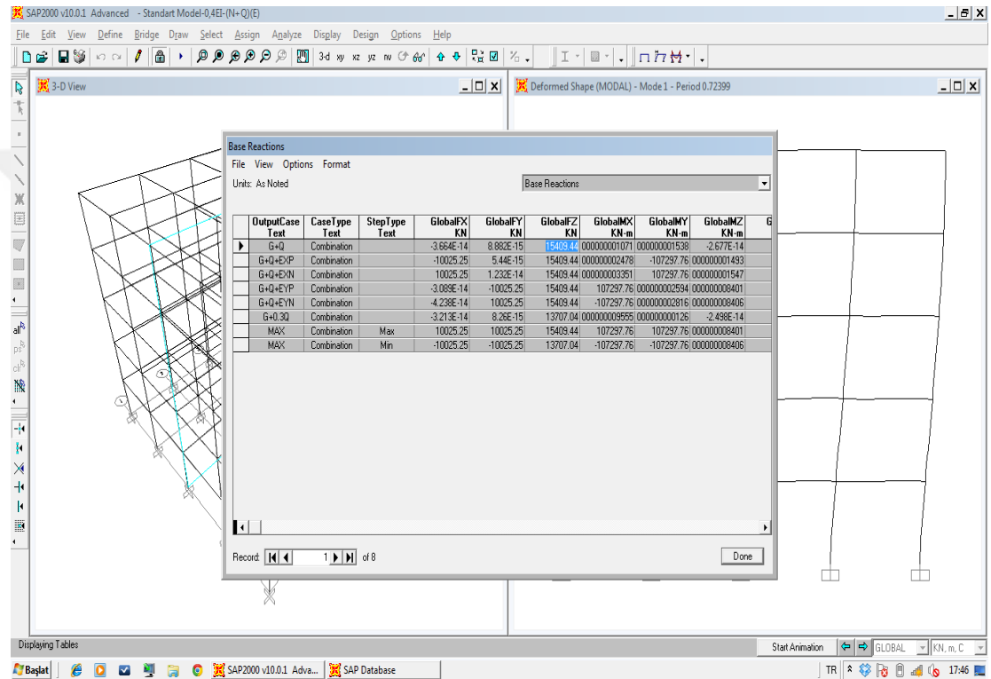
Şekil 4.10 : B1 binası SAP2000 mesnet reaksiyonları.
