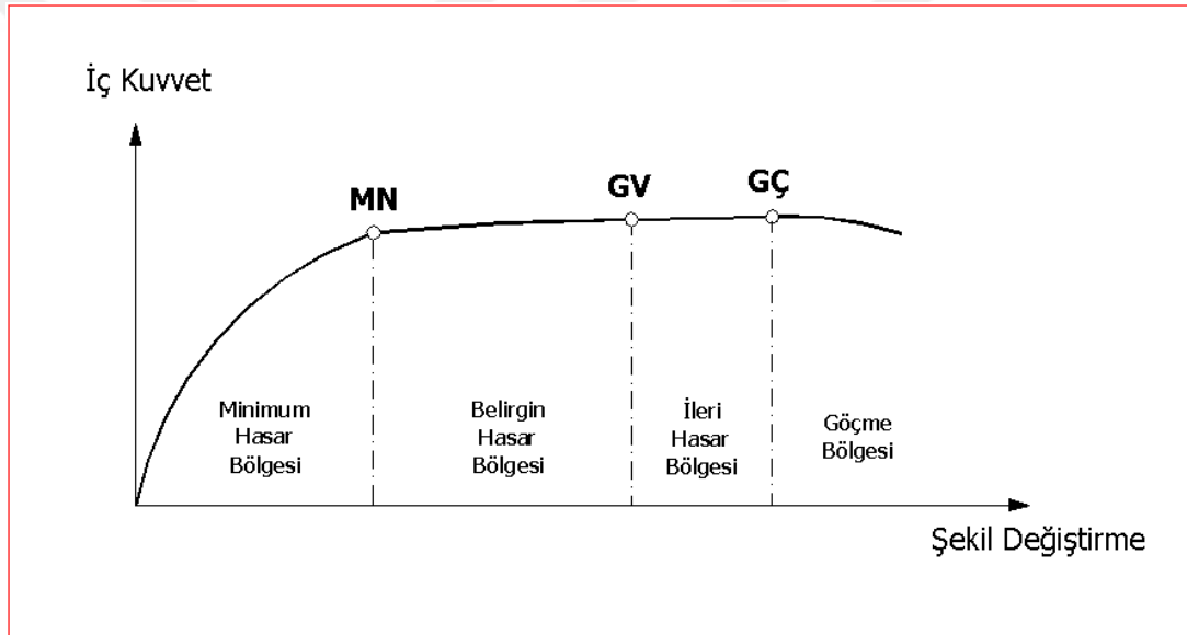
Şekil 4.20 : Kesit hasar bölgeleri.
