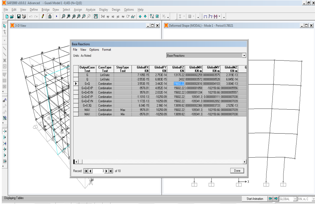
Şekil 4.59 : B3 binası SAP2000 mesnet reaksiyonları.
