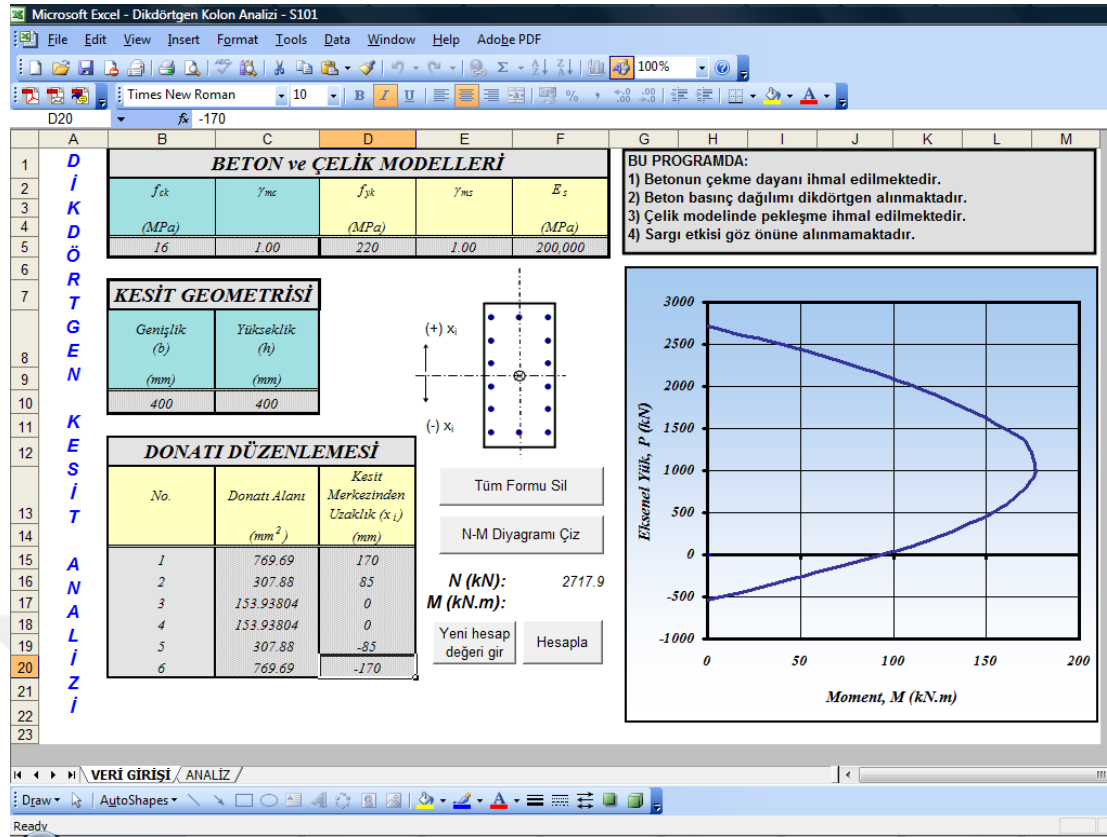
Şekil 4.26 : Dikdörtgen kolon analizi ile ‘kolon karşılıklı etkileşim diyagramı’ çizimi.
