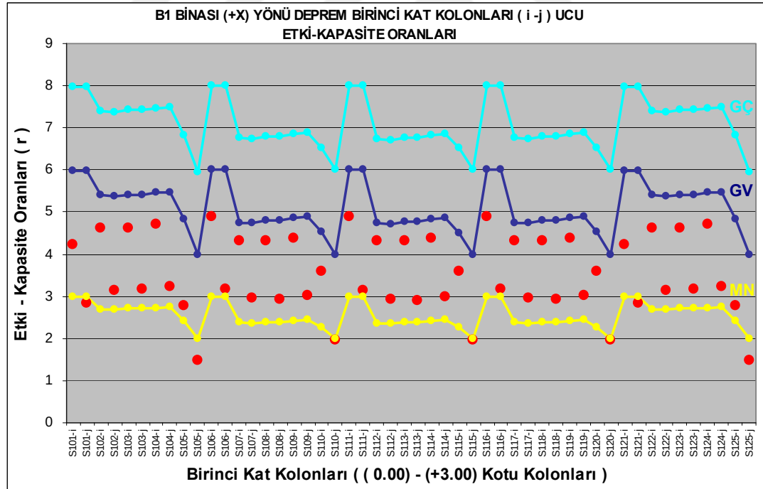
Şekil 4.32 : B1 binası (+X) yönü deprem durumu, birinci kat kolonları, (i – j ucu) kolon hasar durum grafiği.
