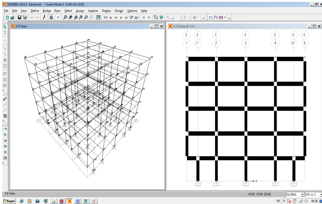
Şekil 4.42 : B2 binası SAP2000 modeli.
