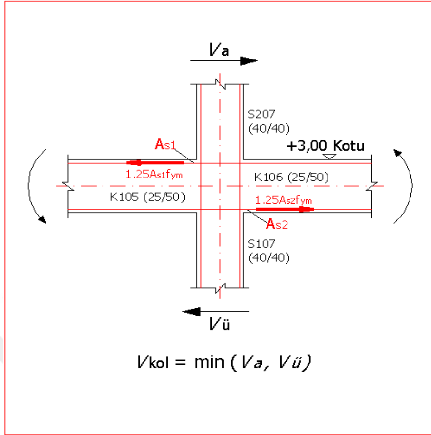
Şekil 4.36 : B1 binası, S107 kolonu (+3.00) kotu birleşim bölgesi.
