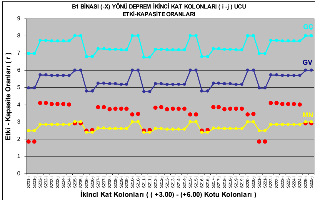
Şekil 4.35 : B1 binası (-X) yönü deprem durumu, ikinci kat kolonları, (i – j ucu) kolon hasar durum grafiği.
