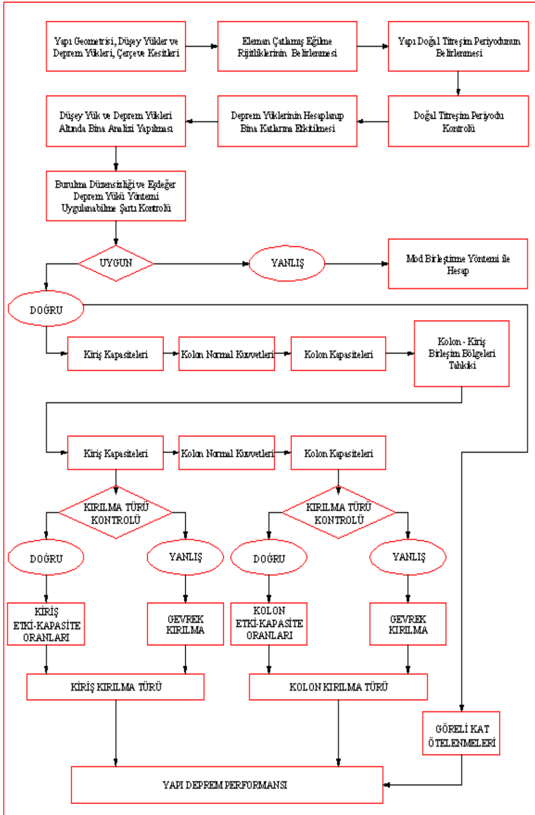
Şekil 2.1 : Doğrusal elastik hesap yöntemi akış diyagramı.
