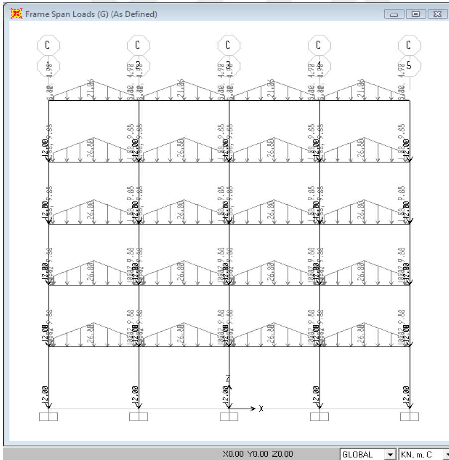
Şekil 4.9 : B1 binası SAP 2000 C aksı (G) yüklemesi yük dağılımı.
