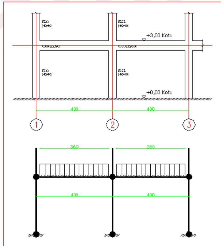
Şekil 4.7 : B1 binası kiriş yayılı yük şematik gösterimi.
