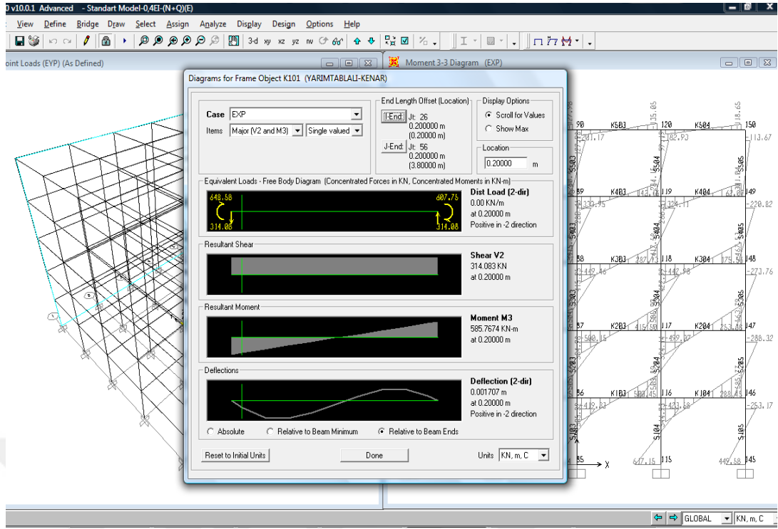
Şekil 4.17 : B1 binası K101 kirişi mesnet reaksiyonları.
