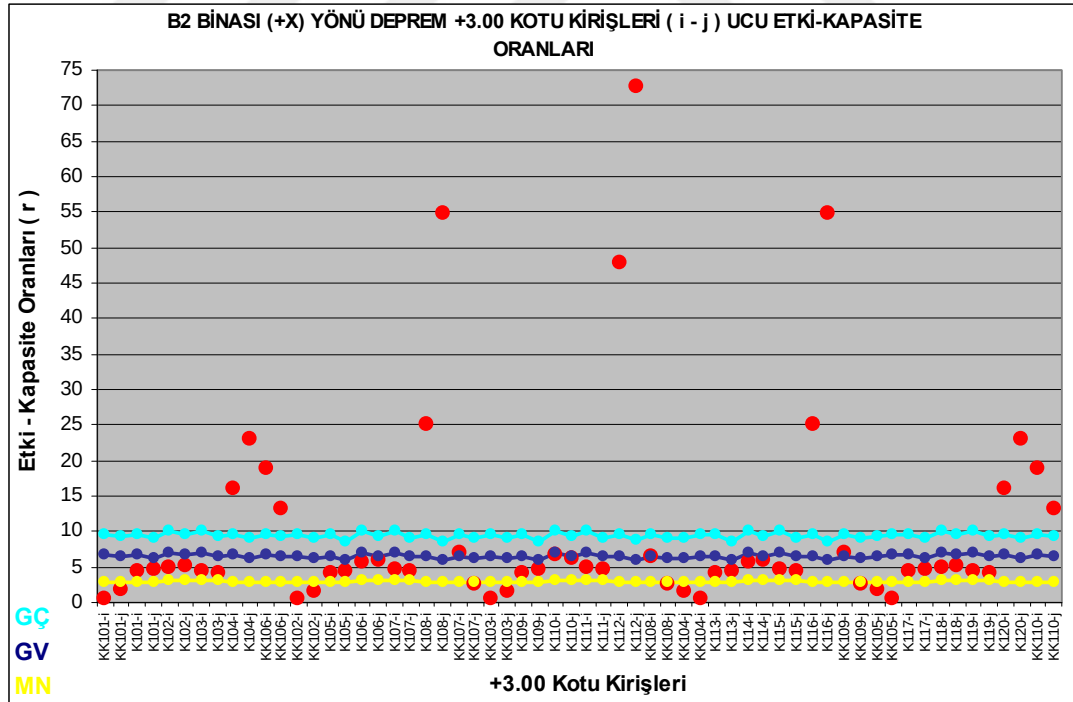
Şekil 4.46 : B2 binası (+X) yönü deprem durumu, +3.00 kotu kirişleri, (i – j ucu) kiriş hasar durum grafiği.
