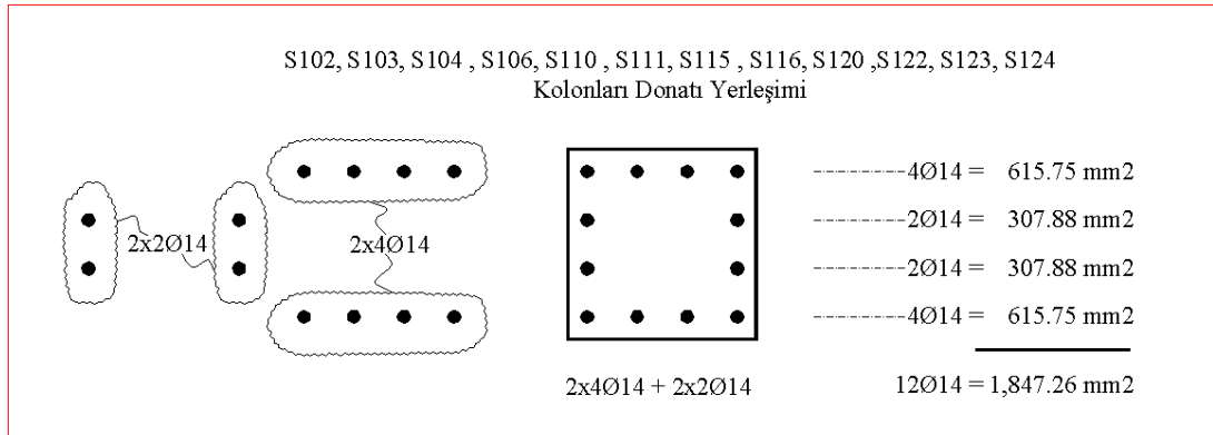
Şekil 4.25 : S102, S103, S104, S106, S110, S111, S115, S116, S120, S122, S123, S124 kolonları donatı yerleşimi.
