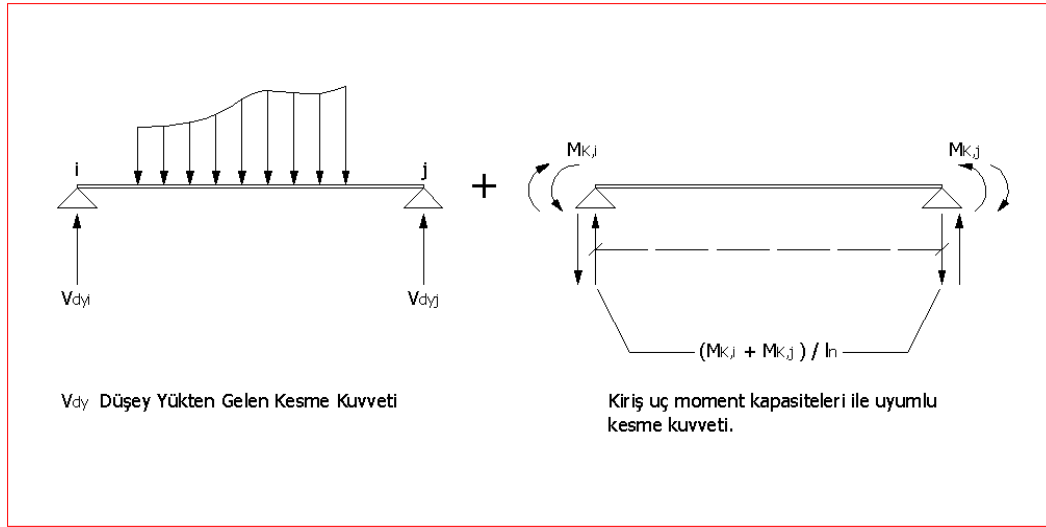
Şekil 4.14 : Kiriş kesme güvenliği tahkiki.
