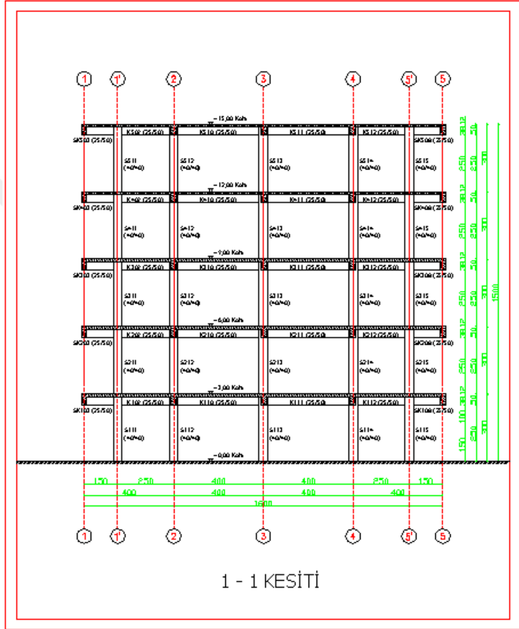
Şekil 4.71 : B4 binası 1-1 boyuna kesiti.
