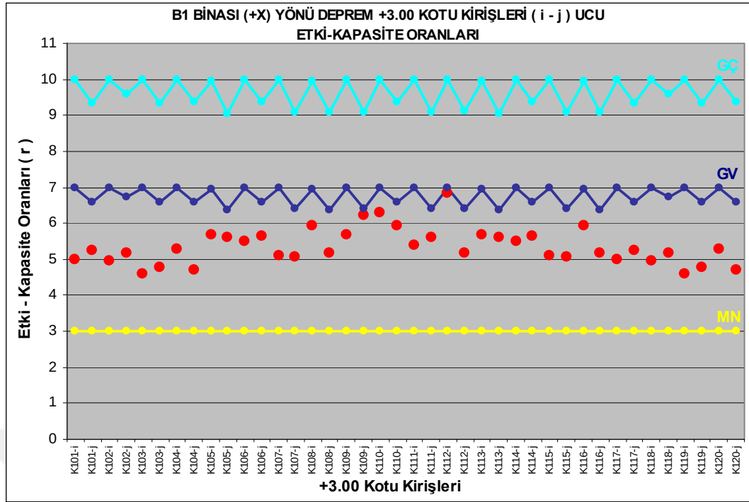
Şekil 4.21 : B1 binası (+X) yönü deprem durumu, +3.00 kotu kirişleri, (i - j ucu) kiriş hasar durum grafiği.
