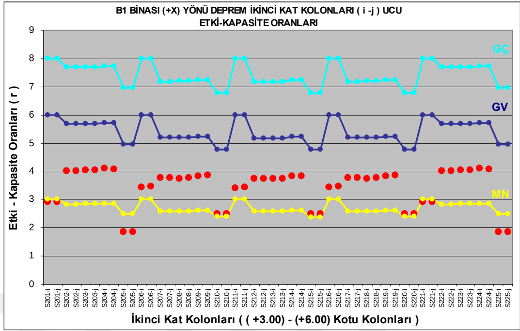
Şekil 4.34 : B1 binası (+X) yönü deprem durumu, ikinci kat kolonları, (i – j ucu) kolon kassar durum grafiği.
