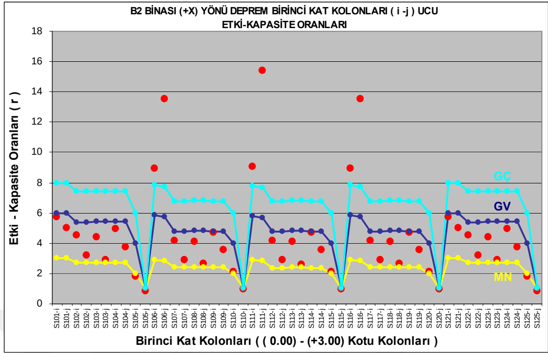
Şekil 4.48 : B2 binası (+X) yönü deprem durumu, birinci kat kolonları, (i – j ucu) kolon hasar durum grafiği.
