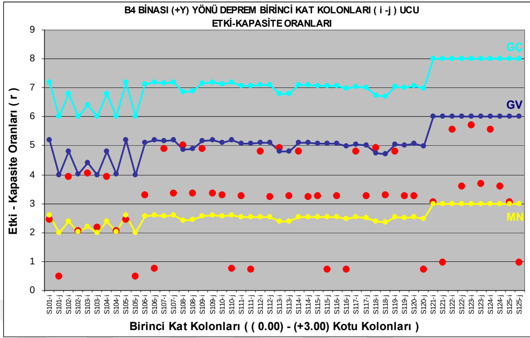
Şekil 4.82 : B4 binası (+Y) yönü deprem durumu, birinci kat kolonları, (i – j ucu) kolon hasar durum grafiği.
