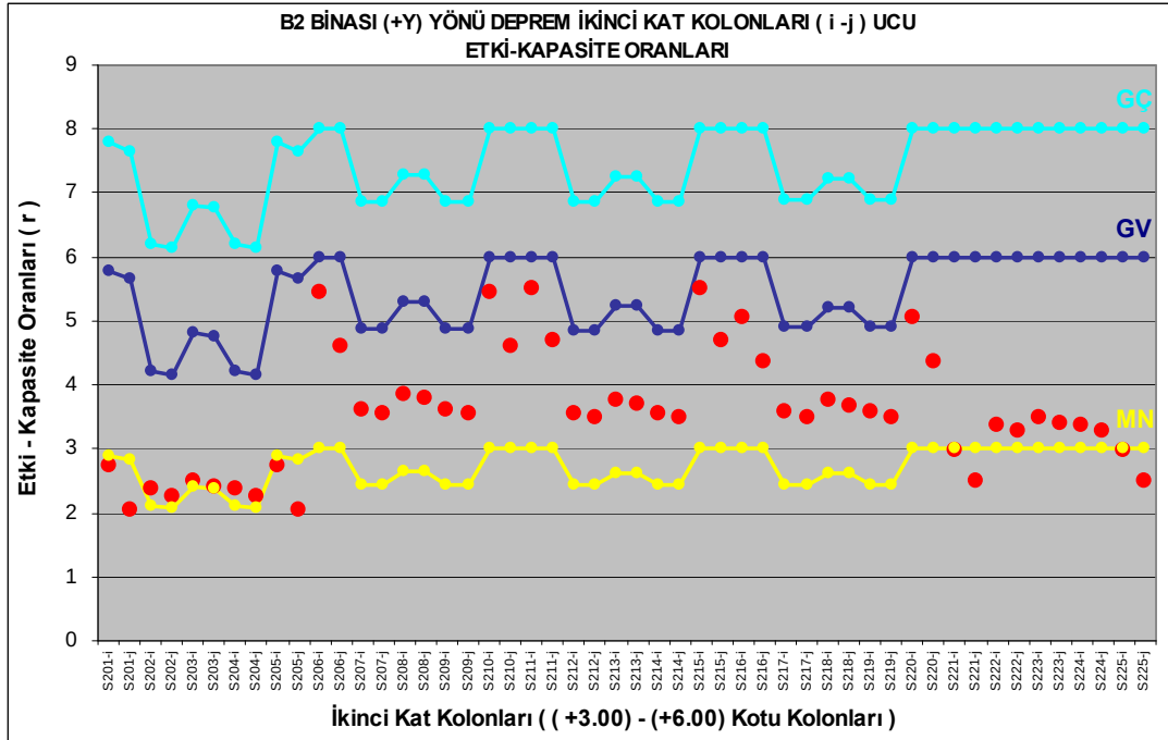
Şekil 4.51 : B2 binası (+Y) yönü deprem durumu, ikinci kat kolonları, ( i – j ucu ) kolon hasar durum grafiği.
