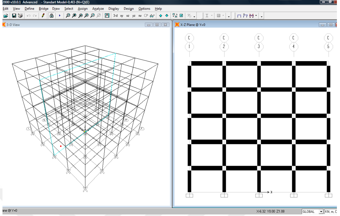
Şekil 4.5 : B1 binası SAP2000 modeli.
