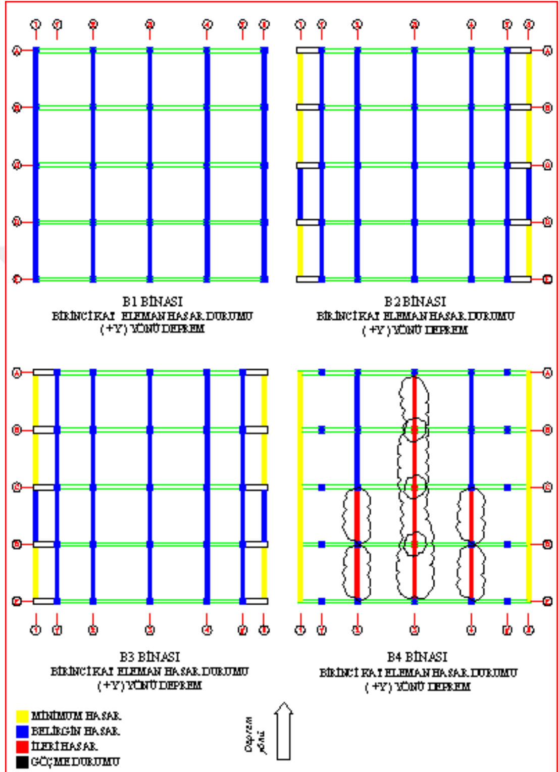
Şekil 5.2 : B1, B2, B3 ve B4 binaları, (+Y) yönü deprem, birinci kat planları, eleman hasar durum karşılaştırması.
