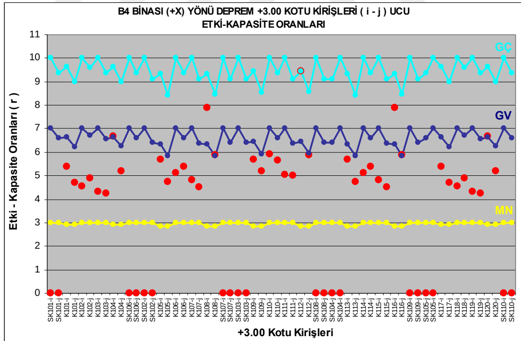
Şekil 4.78 : B4 binası (+X) yönü deprem durumu, +3.00 kotu kirişleri, (i – j ucu) kiriş hasar durum grafiği.
