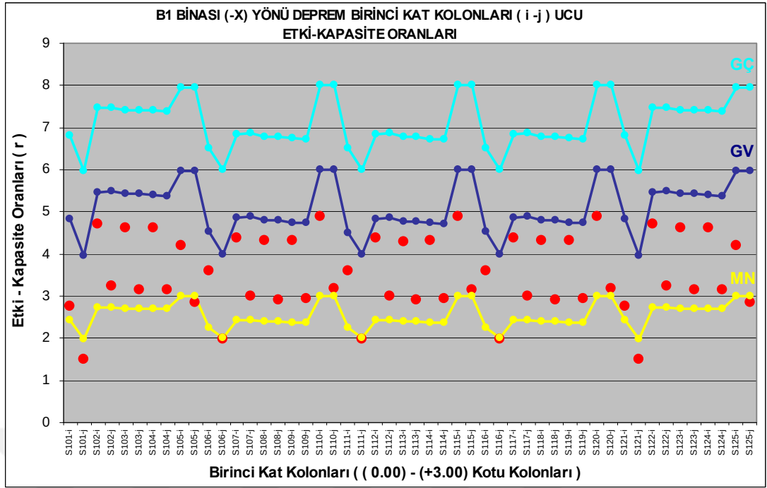
Şekil 4.33 : B1 binası (-X) yönü deprem durumu, birinci kat kolonları, (i – j ucu) kolon hasar durum grafiği.
