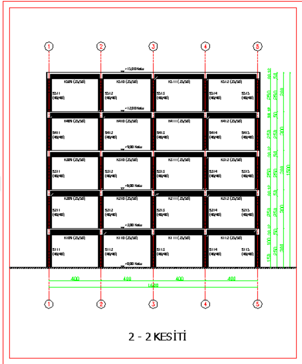
Şekil 4.4 : B1 binası 2-2 boyuna kesiti.
