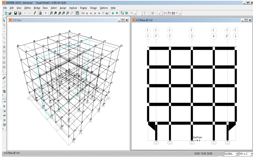
Şekil 4.58 : B3 binası SAP2000 modeli.
