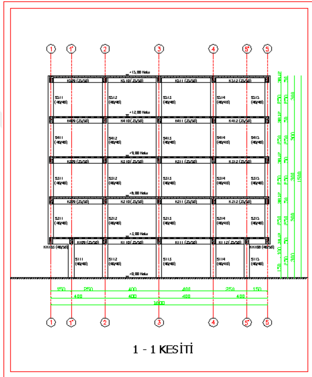
Şekil 4.40 : B2 binası 1-1 boyuna kesiti.
