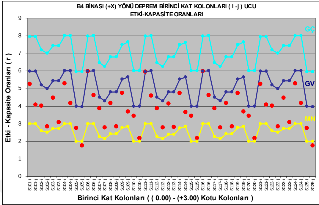
Şekil 4.80 : B4 binası (+X) yönü deprem durumu, birinci kat kolonları, (i – j ucu) kolon hasar durum grafiği.
