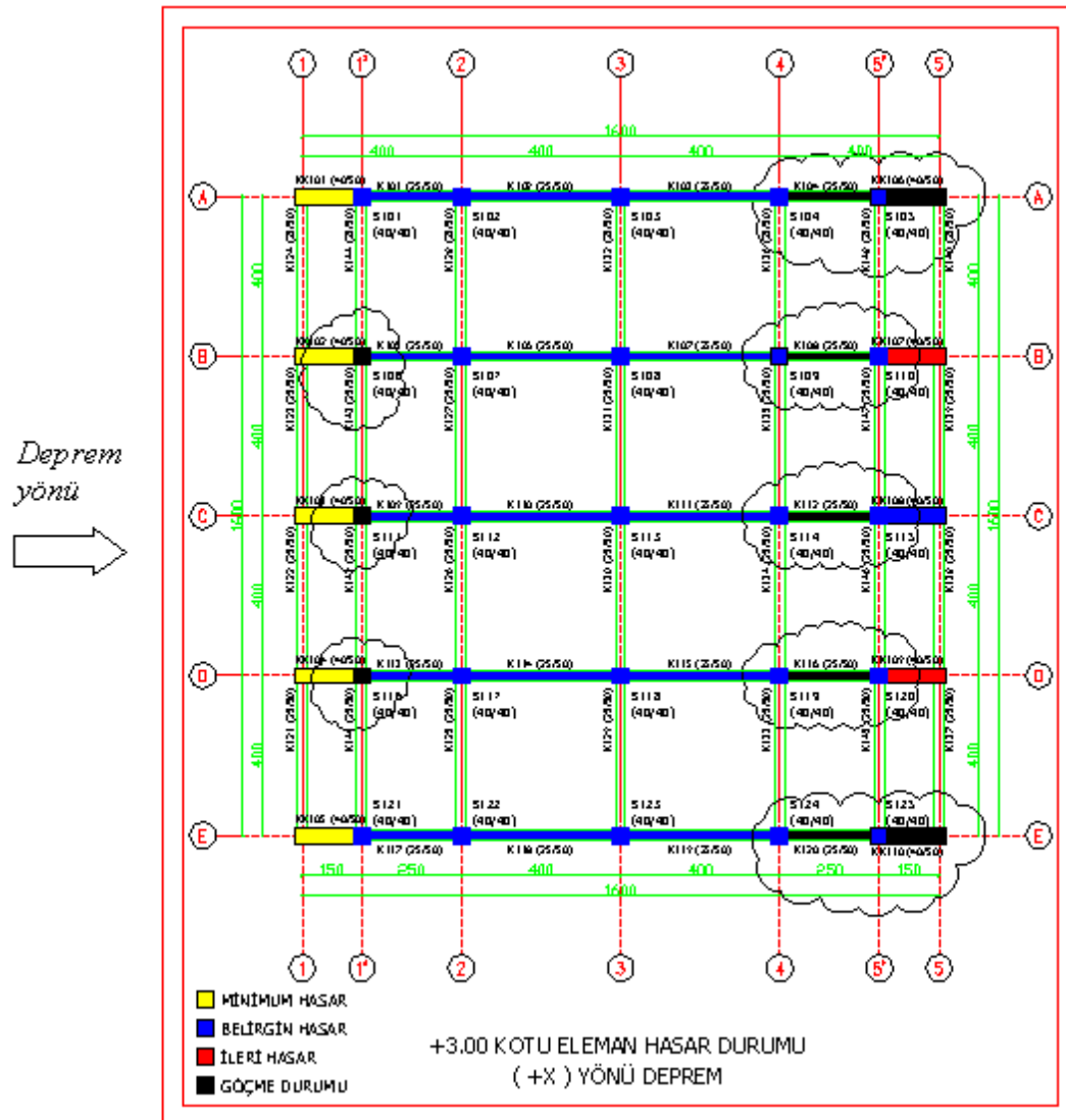
Şekil 4.52 : B2 binası (+X) yönü deprem eleman hasar durumu.
