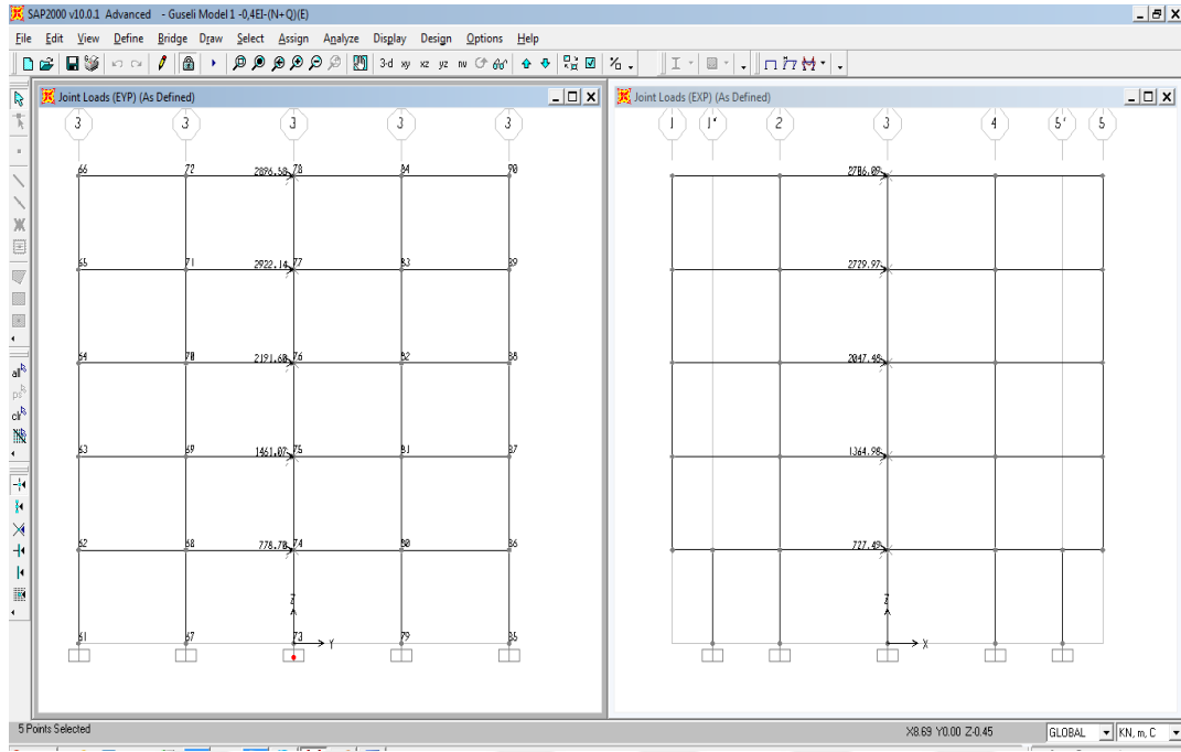
Şekil 4.61 : B3 binası, SAP2000 katlara etkiyen eşdeğer deprem yükleri.
