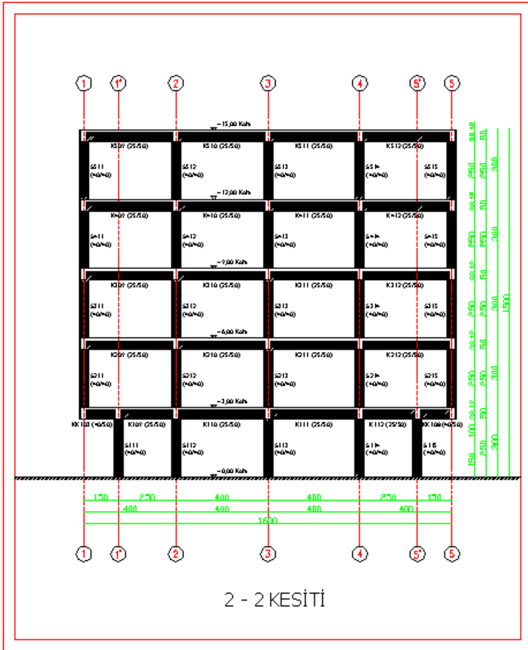
Şekil 4.41 : B2 binası 2-2 boyuna kesiti.
