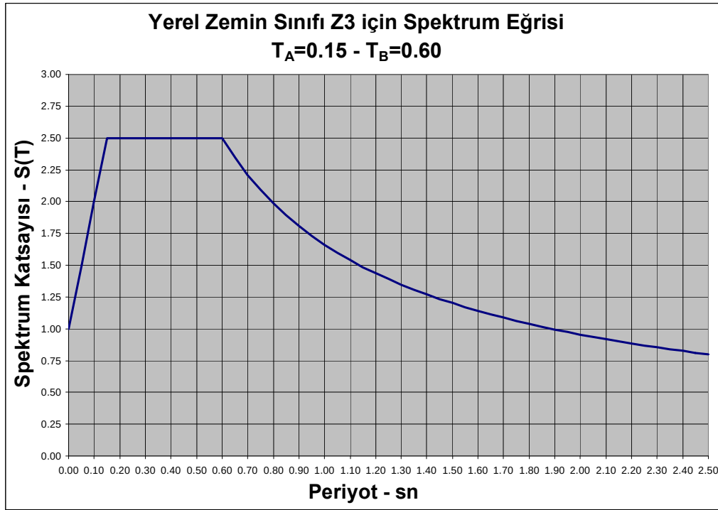
Şekil 4.11 : Yerel zemin sınıfı Z3 için spektrum eğrisi.
