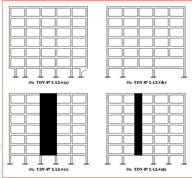
Şekil 3.4 : B3 - taşıyıcı sistemin düşey elemanlarının süreksizliği - (TDY-07, Şekil 2.3).
