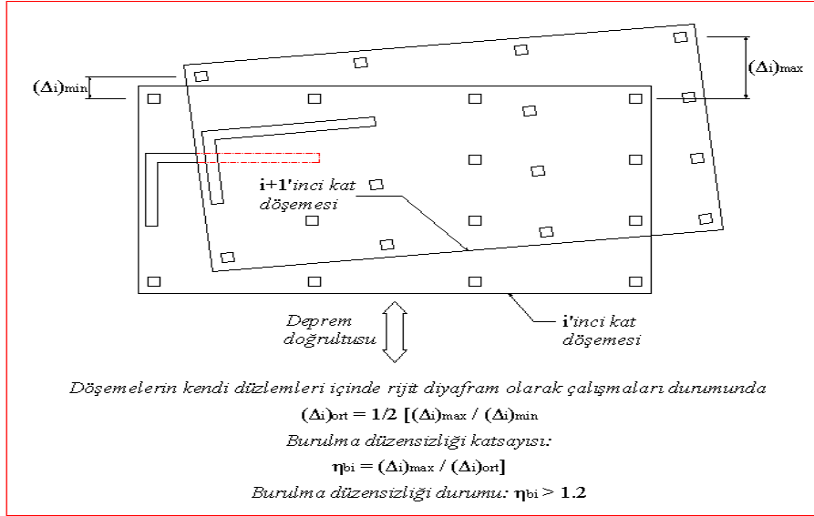
Şekil 3.1 : A1 – burulma düzensizliği - ( TDY-07, Şekil 2.1).
