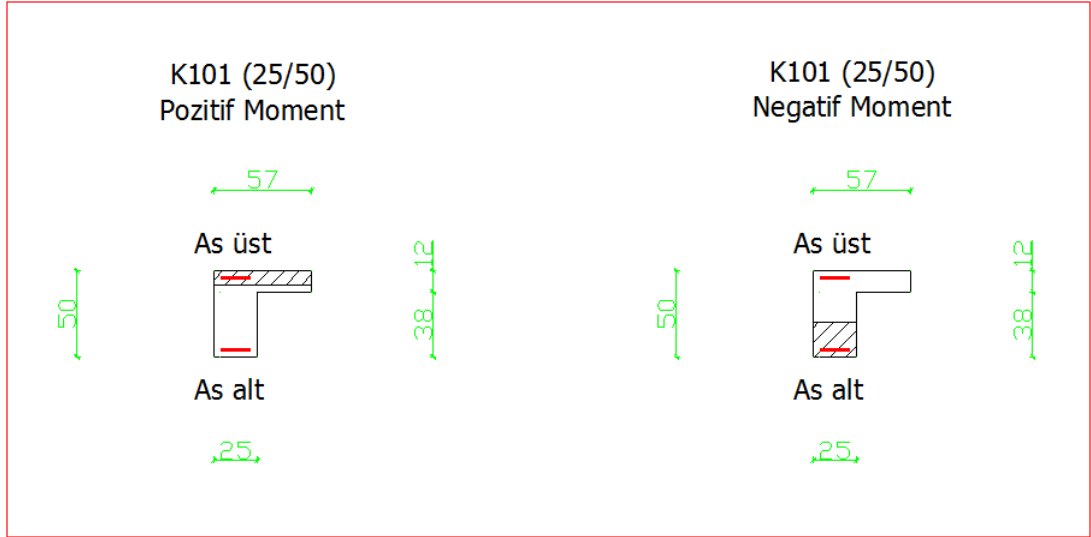
Şekil 4.15 : Kiriş çekme ve basınç bölgeleri.
