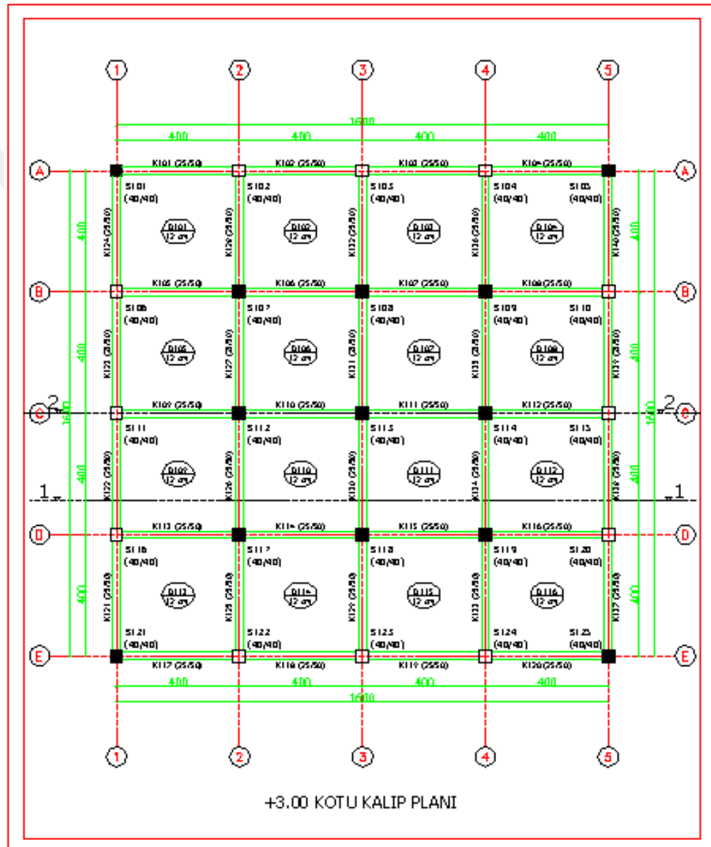
Şekil 4.2 : B1 binası +3.00 kotu kalıp planı.
