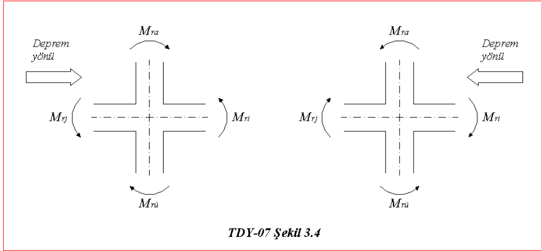
Şekil 4.23 : ( \pm X ) deprem durumu birleşim bölgesi çalışma şekli ( TDY-07, 3.3.5).
