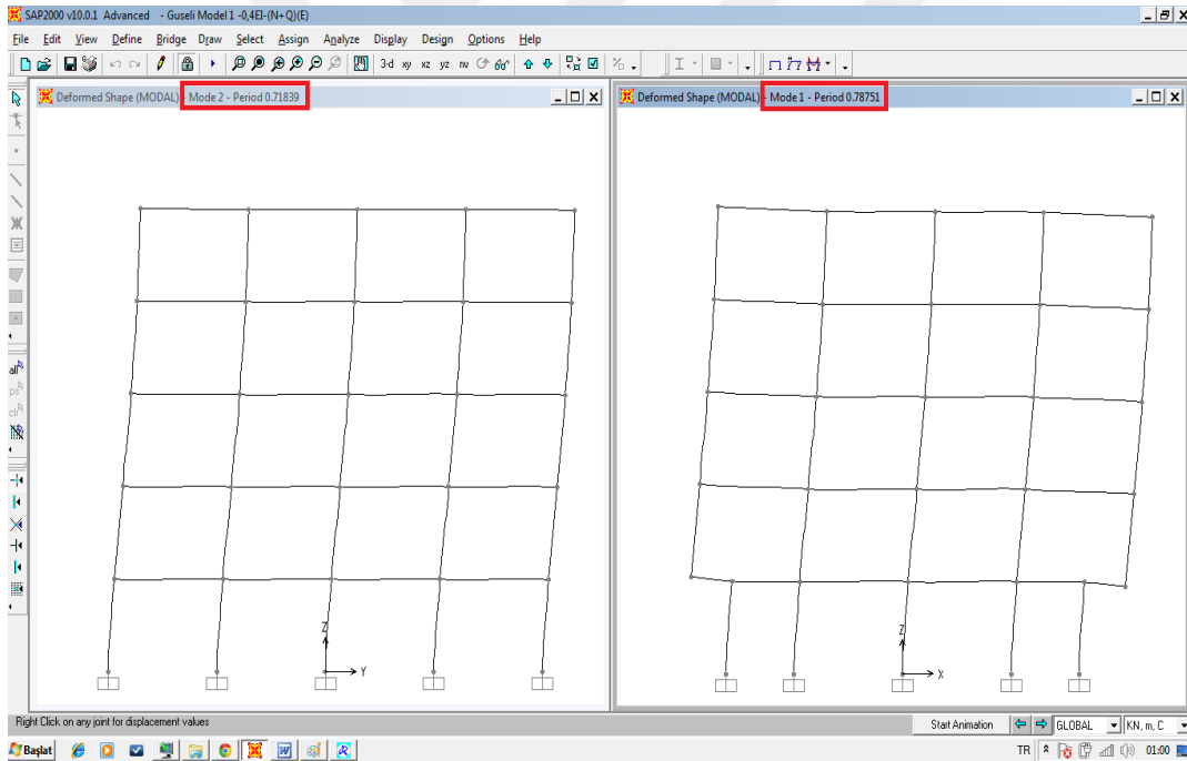
Şekil 4.44 : B2 binası SAP2000 (X) ve (Y) yönü bina doğal titreşim periyotları.
