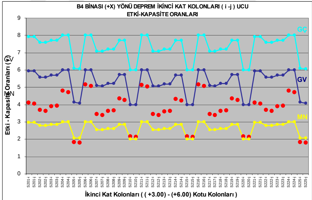
Şekil 4.81 : B4 binası (+X) yönü deprem durumu, ikinci kat kolonları, (i – j ucu) kolon hasar durum grafiği.
