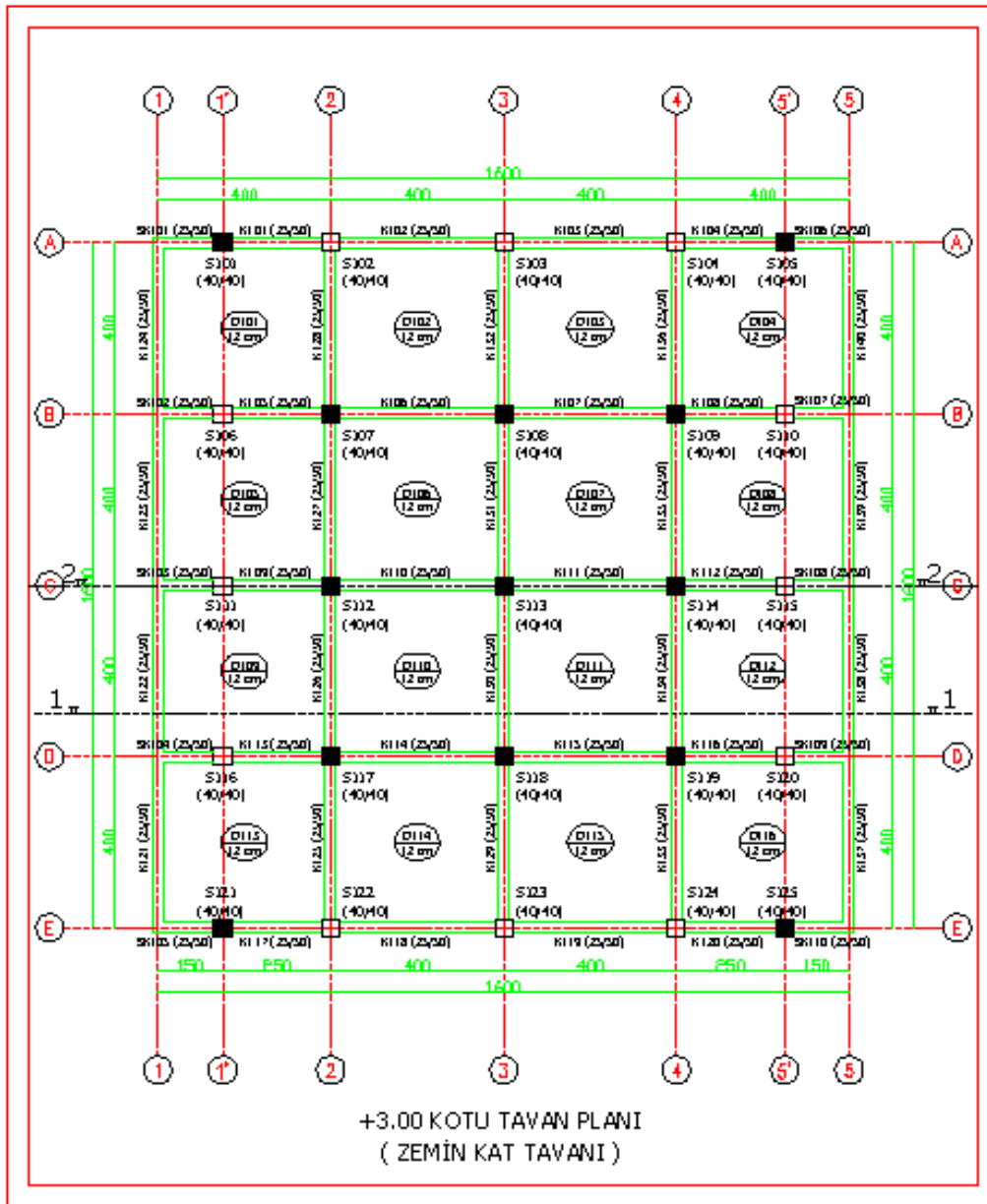
Şekil 4.70 : B4 binası +3.00 kotu kalıp planı.
