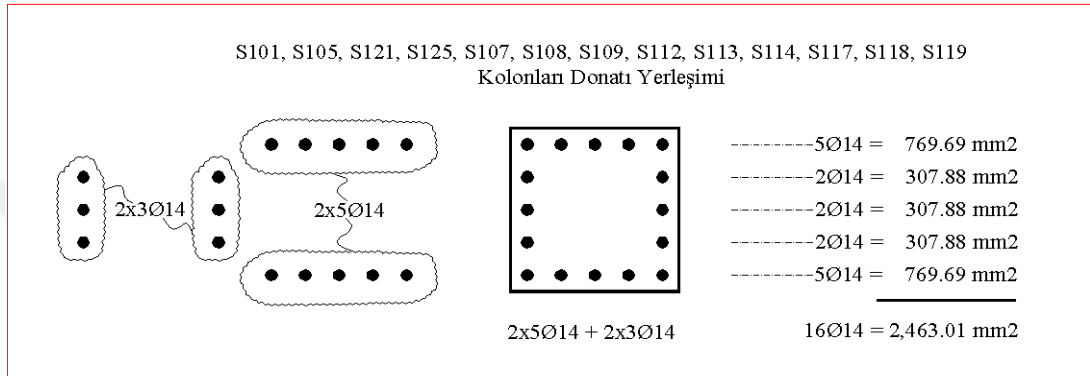
Şekil 4.24 : S101, S105, S121, S125, S107, S108, S109, S112, S113, S114, S117, S118, S119 kolonları donatı yerleşimi.
