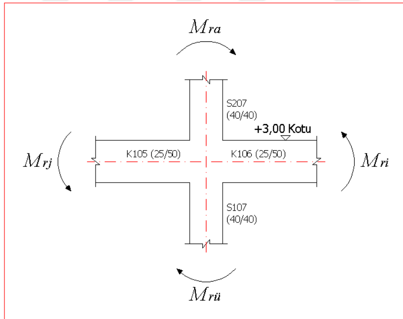
Şekil 4.37 : B1 binası, S107 kolonu (+3.00) kotu kolon-kiriş birleşim bölgesi.
