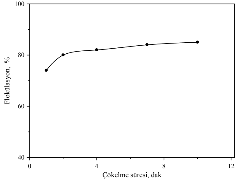
Şekil 4.10. n-Heptan ile talkın flokülasyonu üzerine çökelme süresinin etkisi.
