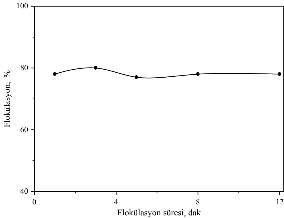
Şekil 4.9.. n-Heptan ile talkın flokülasyonu üzerine flokülasyon süresinin etkisi.
