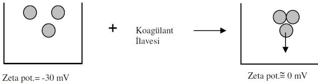
Şekil 2.3. Bir süspansiyondaki disperse partiküllerin koagülasyonu (Çelik ve Ersoy, 2004; Alptekin, 2006)
