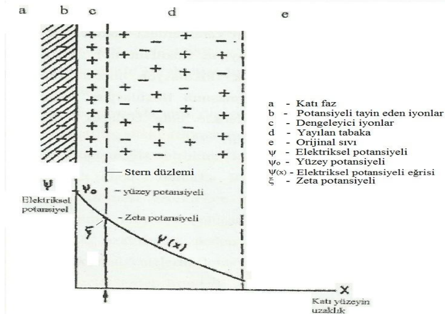
Şekil 2.4. Elektriksel çift tabaka ve zeta potansiyeli (Atak, 1982; İpekoğlu, 1997)
