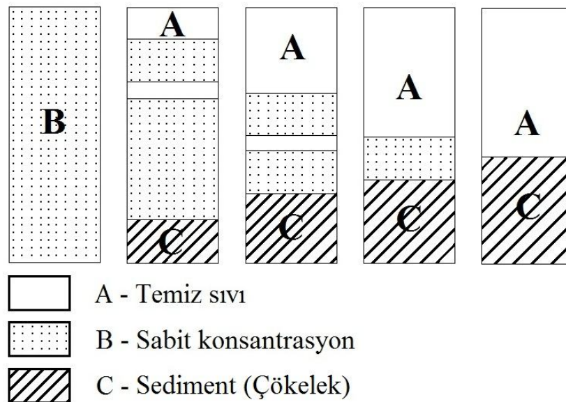
Şekil 2.2. Sedimentasyon olayının şematik gösterimi (Oğul, 2005; Beyazyüz, 2010)
