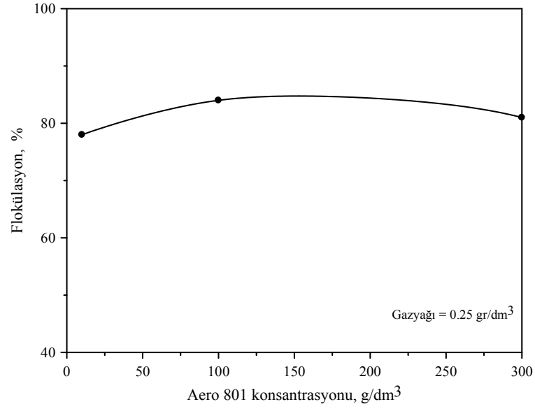
Şekil 4.17. 0.25 g/dm 3 gazyağı miktarında Aero 801 konsantrasyonunun talkın flokülasyonuna etkisi.
