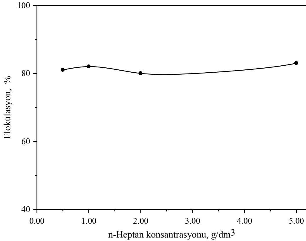
Şekil 4.6. n-Heptan konsantrasyonunun talkın flokülasyonuna etkisi.
