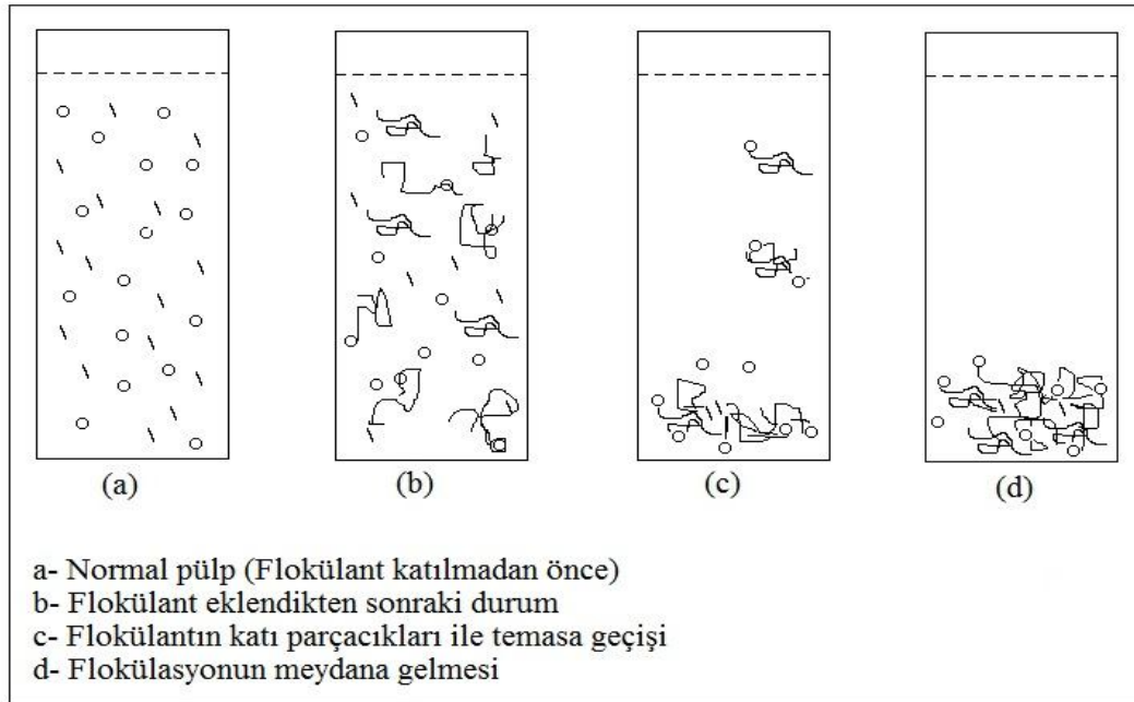
Şekil 2.6. Flokülasyon oluşum şekli (Oğul, 2005; Beyazyüz, 2010)
