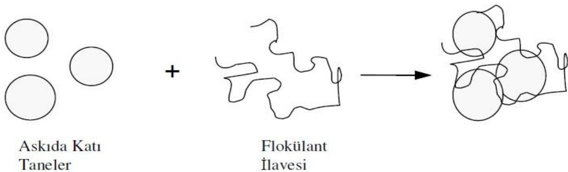
Şekil 2.7. Polimer köprü teşekkülü ile askıda katı tanelerin flokülasyonu (Alptekin, 2006; İpekoğlu, 2007)
