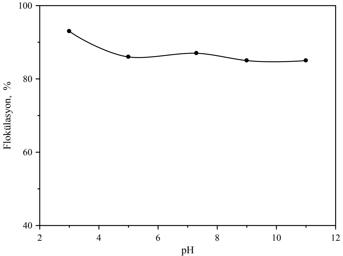
Şekil 4.2. Gazyağı ile talkın flokülasyonu üzerine pH'ın etkisi.
