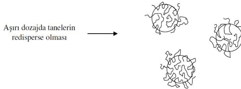
Şekil 2.14. Aşırı flokülant dozajında tanelerin yeniden disperse hale gelmesi (flokülantların sterik engel oluşturması) (Ersoy, 2003; Alptekin, 2006; Öner, 2011)
