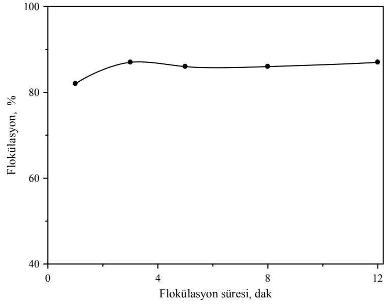
Şekil 4.4. Gazyağı ile talkın flokülasyonu üzerine flokülasyon süresinin etkisi.
