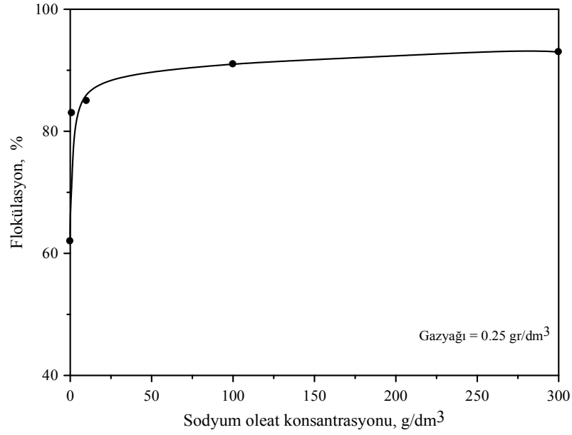
Şekil 4.19. 0.25 g/dm 3 gazyağı miktarında sodyum oleat konsantrasyonunun talkın flokülasyonuna etkisi.
