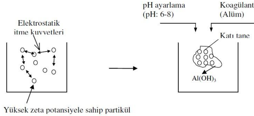
Şekil 2.5. Süpürme koagülasyon (Sweep coagulation) (Gregory, 1989; Alptekin, 2006)
