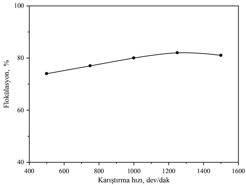
Şekil 4.8. n-Heptan ile talkın flokülasyonu üzerine karıştırma hızının etkisi.
