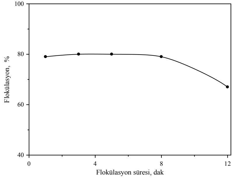
Şekil 4.14. n-Hekzan ile talkın flokülasyonu üzerine flokülasyon süresinin etkisi.
