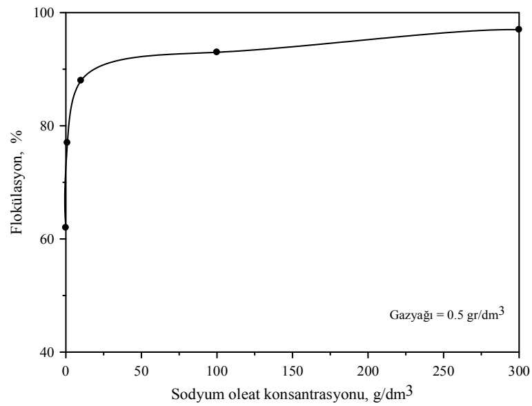
Şekil 4.18. 0.5 g/dm 3 gazyağı miktarında sodyum oleat konsantrasyonunun talkın flokülasyonuna etkisi.
