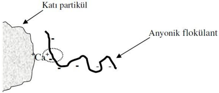
Şekil 2.11. Süspansiyondaki katı partikül (mineral) yüzeyindeki \text{Ca}^{+2} iyonu ile anyonik flokülant arasındaki kovalent bağ (katyonik köprü) oluşumu (Yarar, 2001; Alptekin, 2006)
