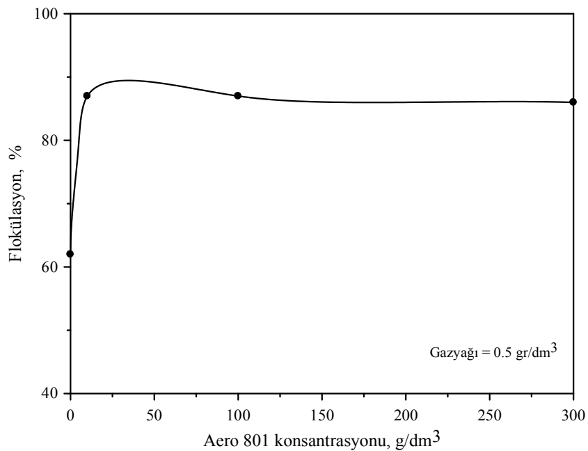
Şekil 4.16. 0.5 \text{ g/dm}^3 gazyağı miktarında Aero 801 konsantrasyonunun talkın flokülasyonuna etkisi.
