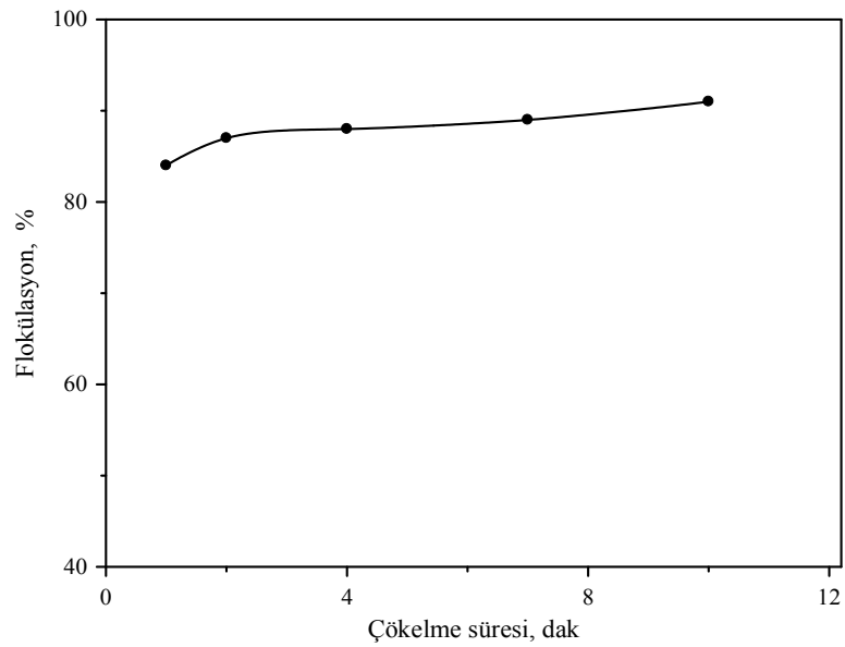
Şekil 4.5. Gazyağı ile talkın flokülasyonu üzerine çökelme süresinin etkisi.
