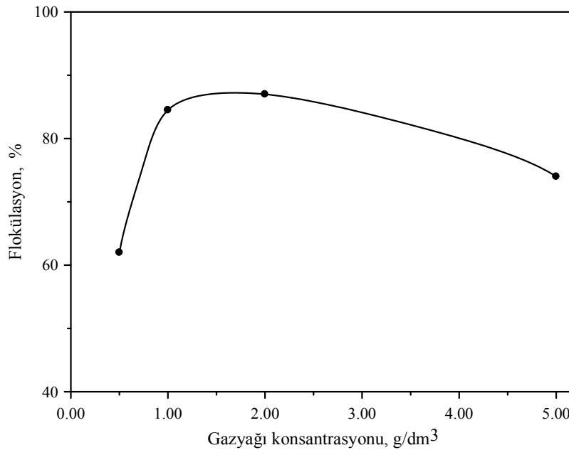
Şekil 4.1. Gazyağı konsantrasyonunun talkın flokülasyonuna etkisi.
