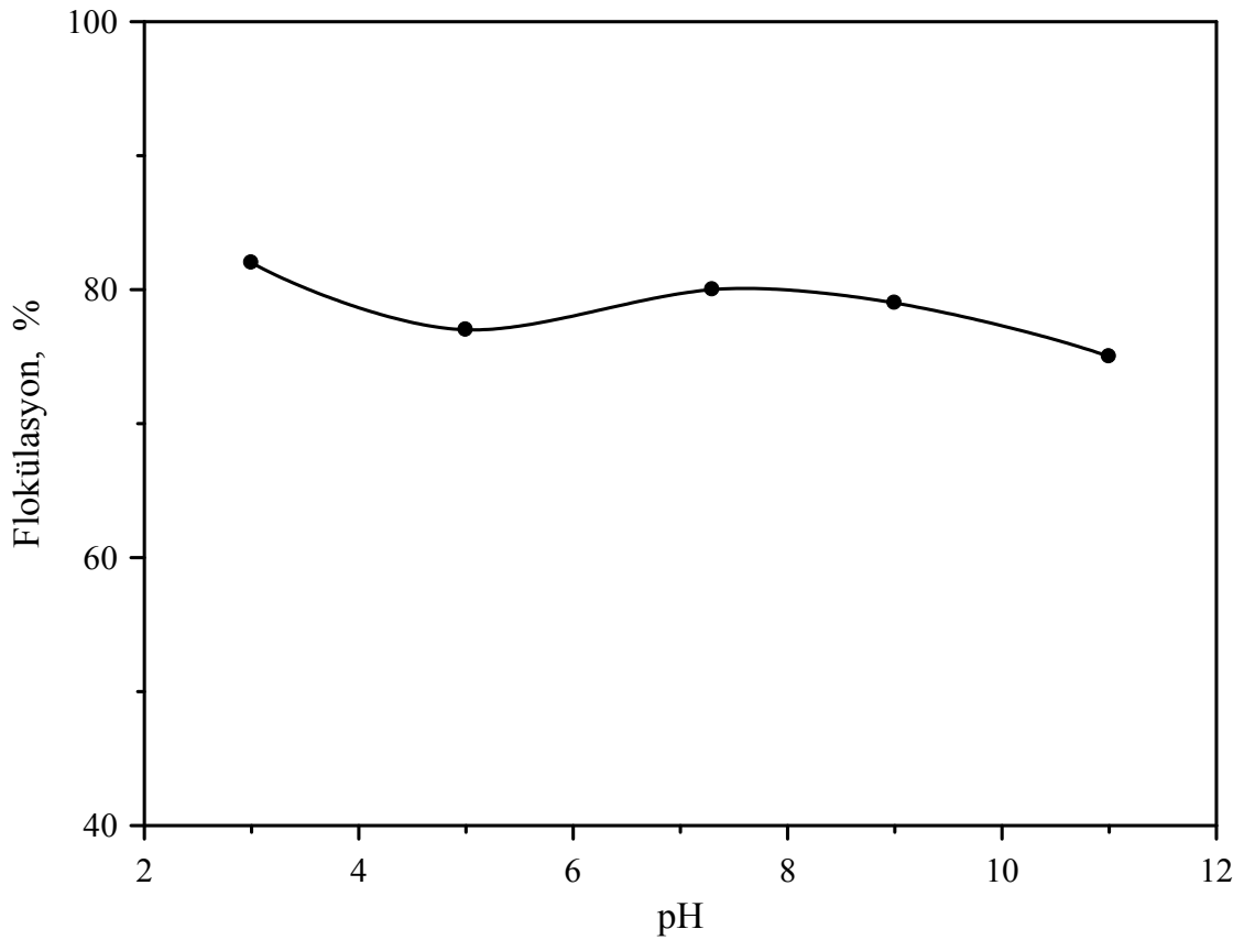
Şekil 4.12. n-Hekzan ile talkın flokülasyonu üzerine pH'ın etkisi.
