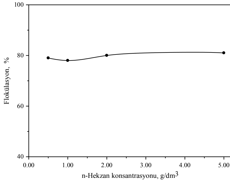
Şekil 4.11. n-Hekzan konsantrasyonunun talkın flokülasyonuna etkisi.
