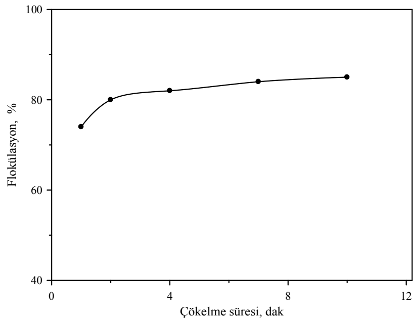
Şekil 4.15. n-Hekzan ile talkın flokülasyonu üzerine çökelme süresinin etkisi.
