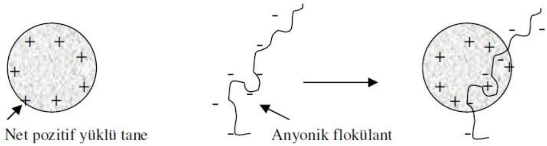
Şekil 2.9. Anyonik flokülantın pozitif yüklü katı yüzeyine elektrostatik çekim kuvvetleri yardımıyla adsorplanması (Ersoy, 2003; Alptekin, 2006)
