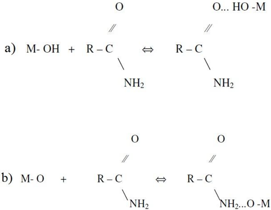
Şekil 2.10. Polimer molekülü ile mineral arasında H-bağı oluşumu (Ateşok, 1988; Öner, 2011)
