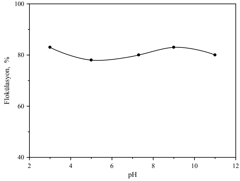
Şekil 4.7. n-Heptan ile talkın flokülasyonu üzerine pH'ın etkisi
