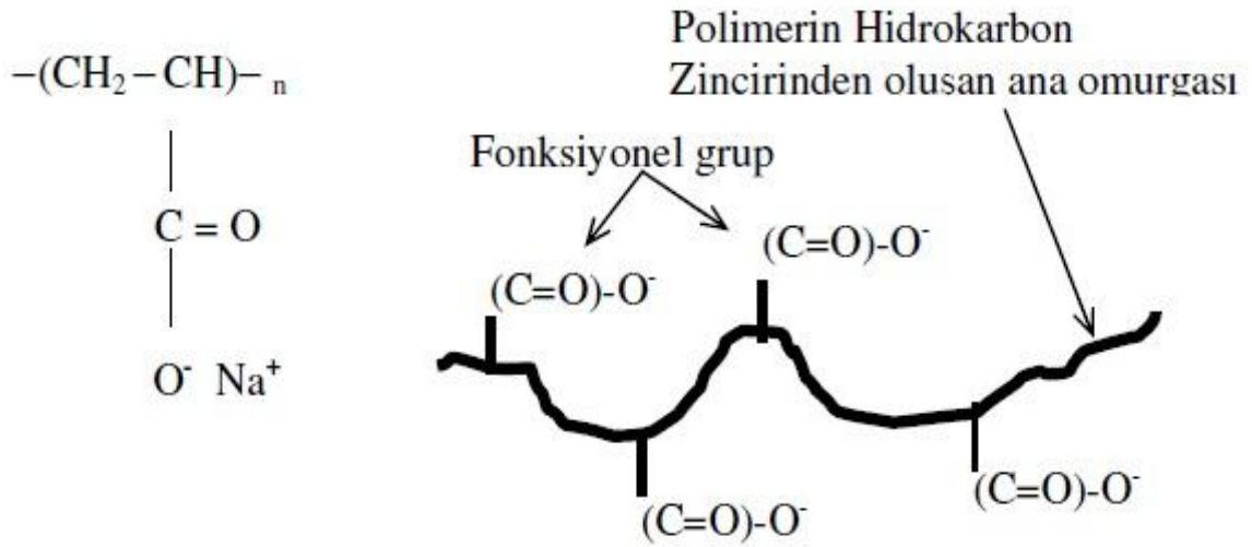
Şekil 2.12. PAA esaslı anyonik flokülanın (Na-Poliakrilat) yapısı (Gregory, 1989; Alptekin, 2006)
