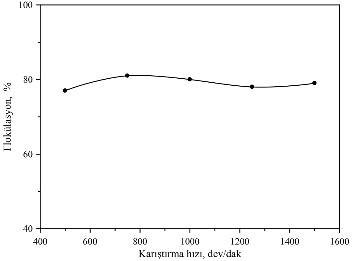
Şekil 4.13. n-Hekzan ile talkın flokülasyonu üzerine karıştırma hızının etkisi.
