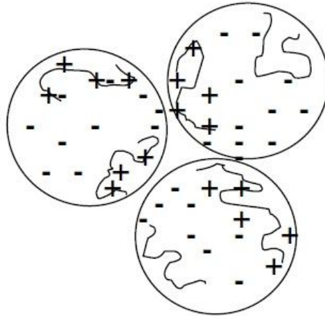
Şekil 2.8. Elektrostatik yük yamaması yöntemiyle flokülasyon (Ersoy, 2003; Alptekin, 2006)
