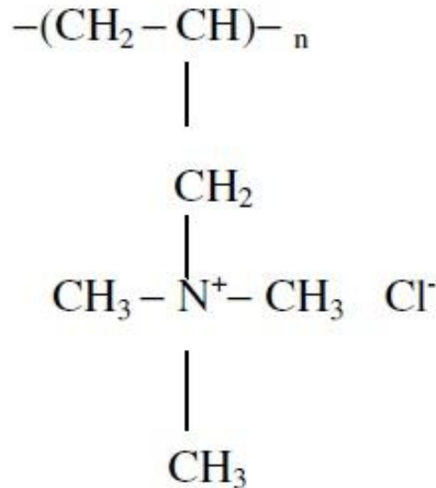
Şekil 2.13. PAA esaslı katyonik bir flokülant olan kuaterneraminli poliakrilamid'in yapısı (Gregory, 1989; Alptekin, 2006)
