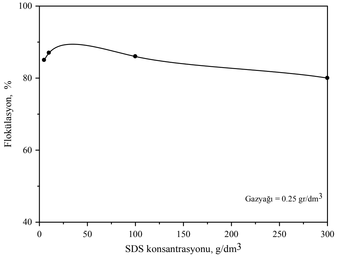
Şekil 4.21. 0.25 g/dm³ gazyağı miktarında SDS konsantrasyonunun talkın flokülasyonuna etkisi.
