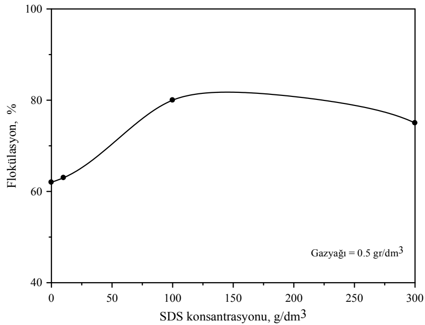
Şekil 4.20. 0.5 g/dm 3 gazyağı miktarında SDS konsantrasyonunun talkın flokülasyonuna etkisi.
