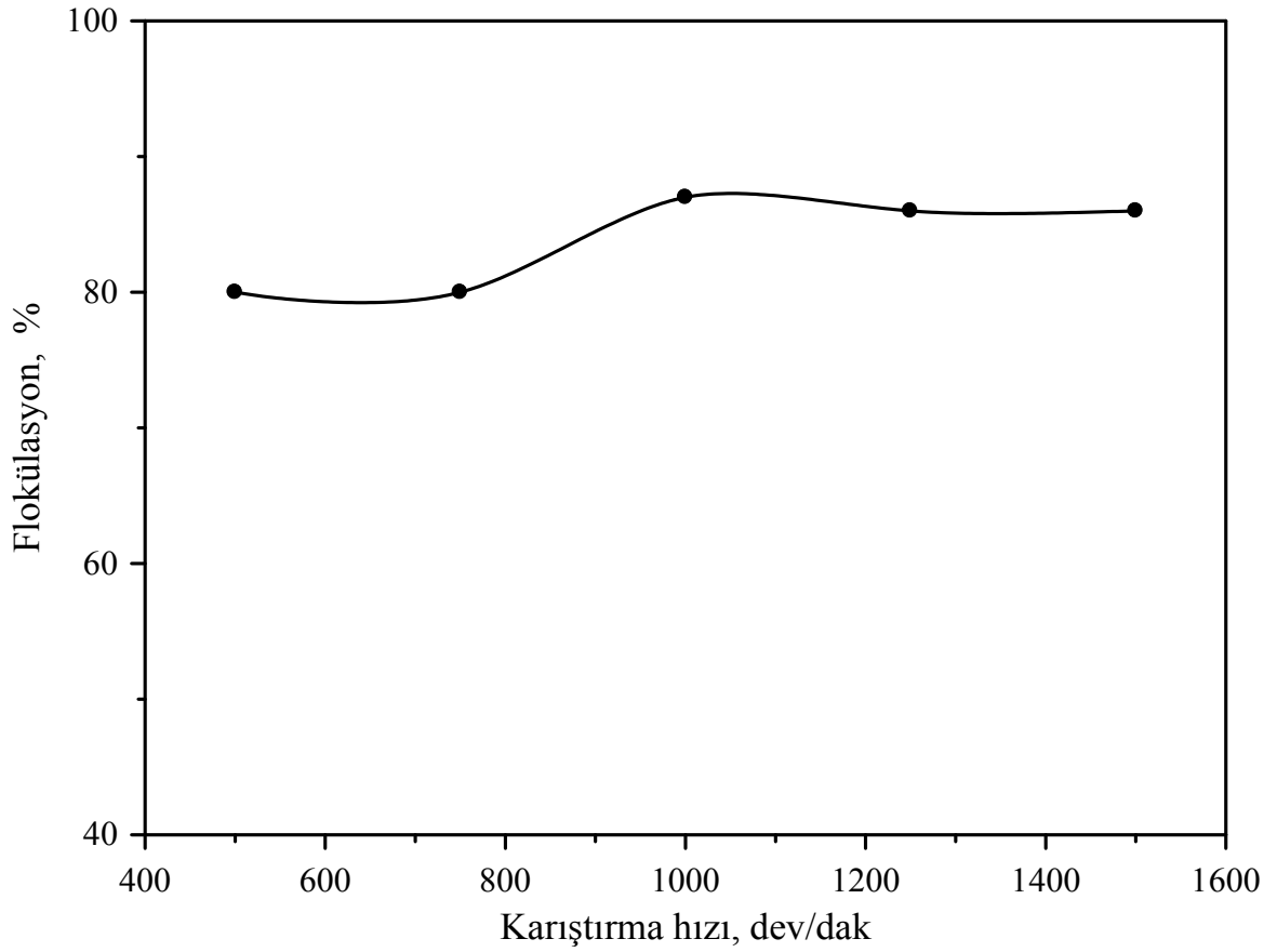
Şekil 4.3. Gazyağı ile talkın flokülasyonu üzerine karıştırma hızının etkisi.
