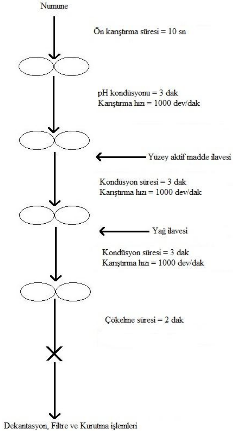
Şekil 3.5. Yüzey aktif madde ve yağ kullanılan flokülasyon deneylerinde izlenen akım şeması
