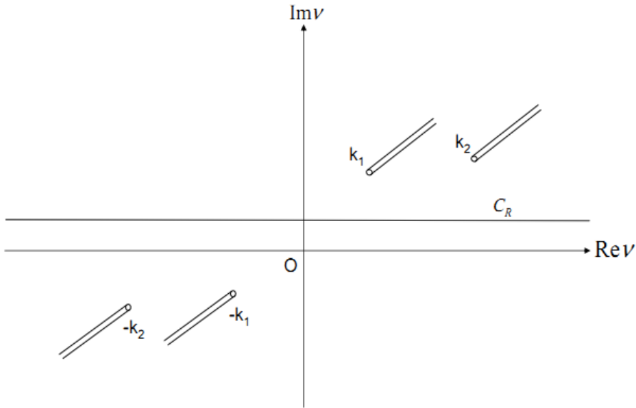
Şekil 2.3 : Karmaşık v düzlemi ve \hat{G}_0 dönüşümü için süreksizlik çizgisi [18].
