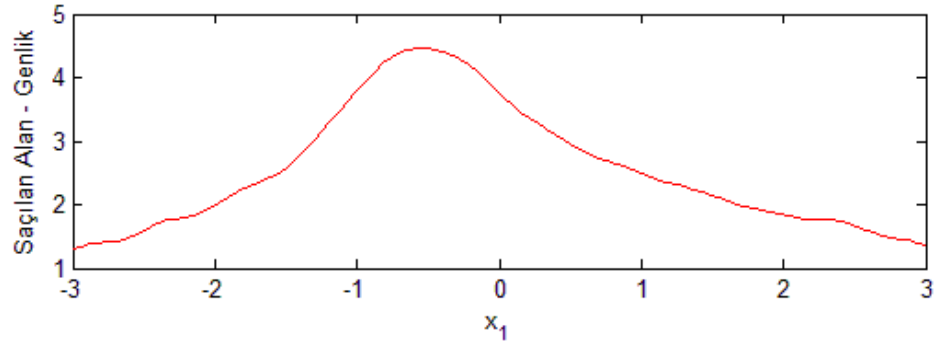
Şekil 5.10 : Örnek 4 için saçılan alan.
