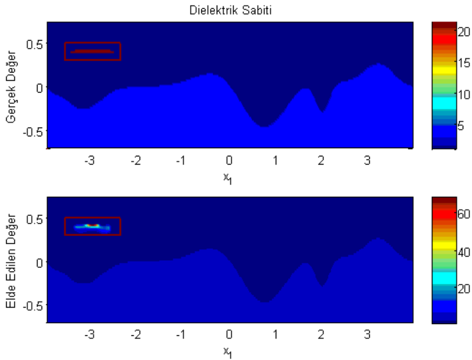
Şekil 5.17 : Örnek 7 için dielektrik sabitinin karşılaştırılması.
