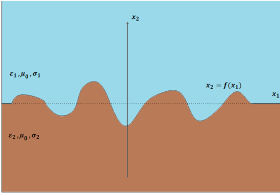
Şekil 2.1 : Düzgün olmayan yüzey ile ayrılmış iki parçalı uzay.
