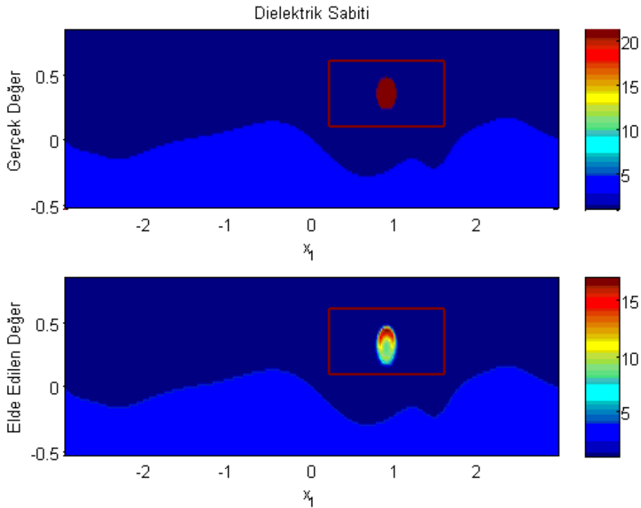
Şekil 5.9 : Örnek 3 için dielektrik sabitinin karşılaştırılması.
