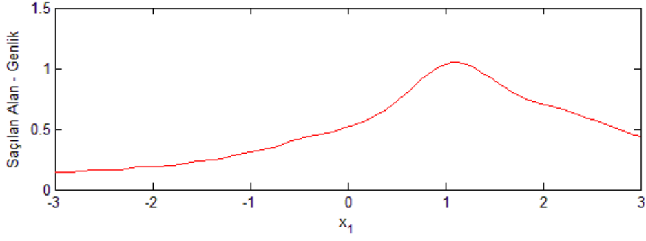
Şekil 5.1 : Örnek 1 için saçılan alan.
