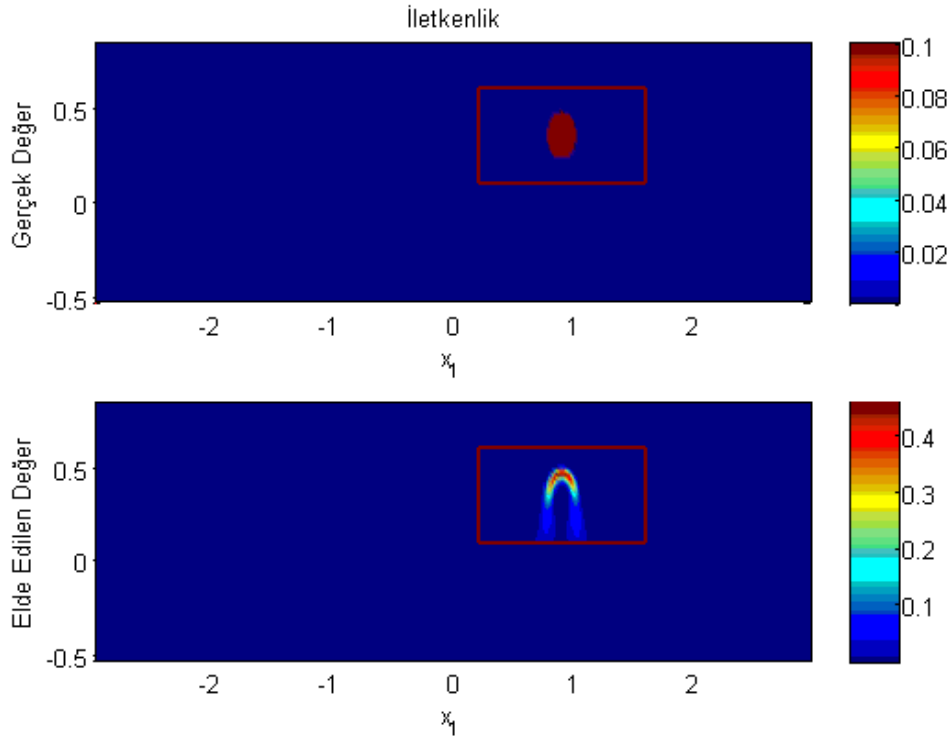
Şekil 5.5 : Örnek 1 için iletkenlik değerinin karşılaştırılması.
