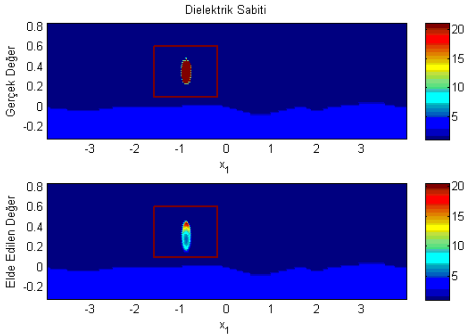
Şekil 5.15 : Örnek 6 için dielektrik sabitinin karşılaştırılması.
