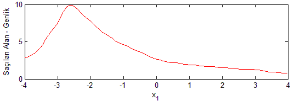
Şekil 5.16 : Örnek 7 için saçılan alan.
