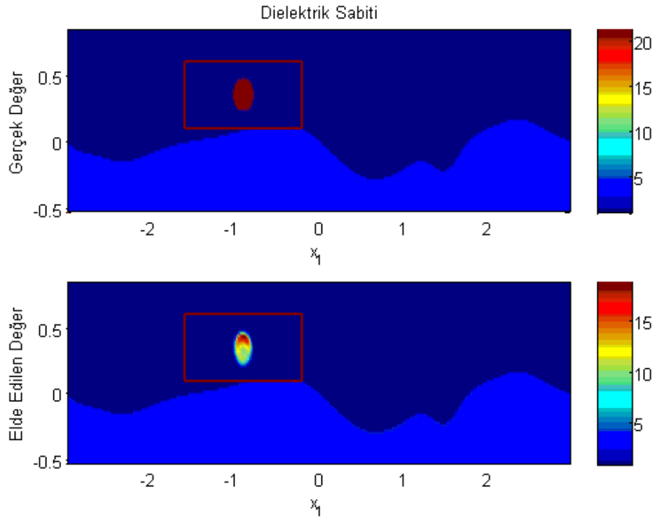
Şekil 5.11 : Örnek 4 için dielektrik sabitinin karşılaştırılması.
