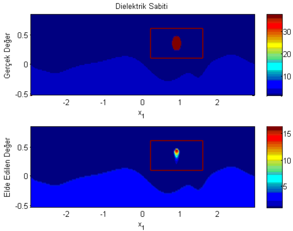
Şekil 5.7 : Örnek 2 için dielektrik sabitinin karşılaştırılması.
