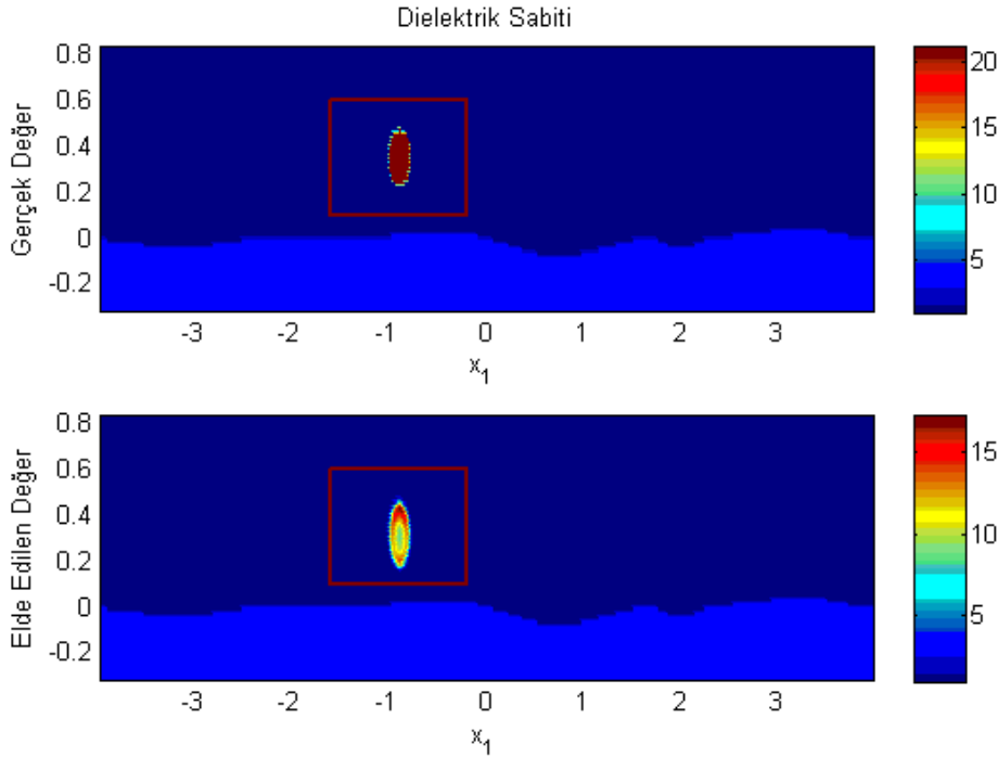
Şekil 5.13 : Örnek 5 için dielektrik sabitinin karşılaştırılması.
