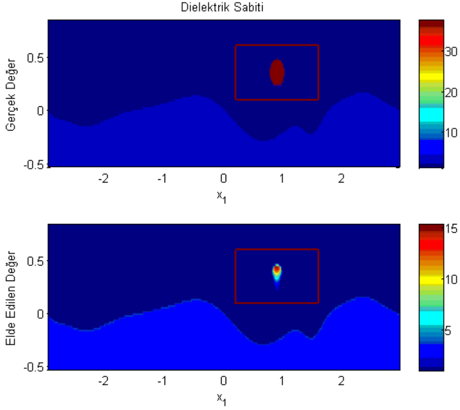
Şekil 5.4 : Örnek 1 için dielektrik sabitinin karşılaştırılması.
