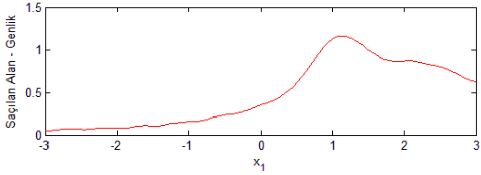
Şekil 5.8 : Örnek 3 için saçılan alan.
