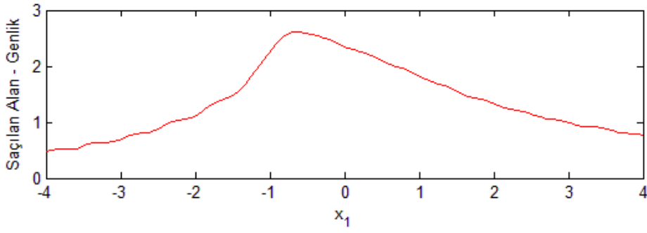
Şekil 5.12 : Örnek 5 için saçılan alan
