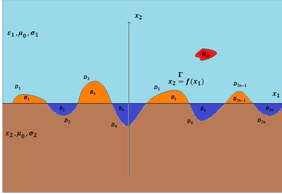
Şekil 2.4 : Düzgün olmayan yüzey üzerindeki cismi içeren geometri.
