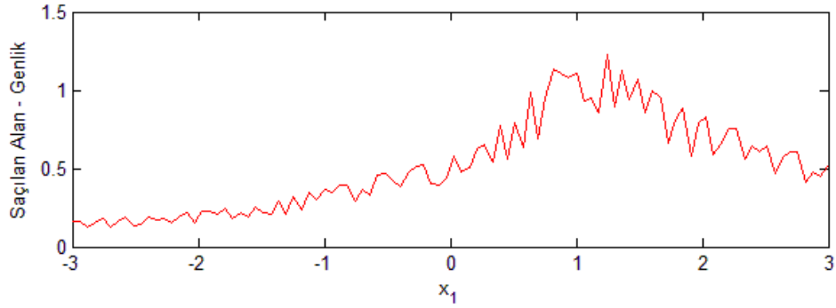
Şekil 5.6 : Örnek 2 için saçılan alan.
