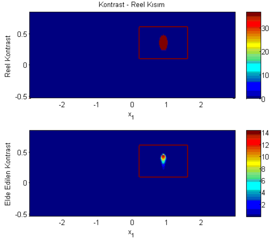
Şekil 5.2 : Örnek 1 için kontrast fonksiyonunun reel kısımlarının karşılaştırılması.
