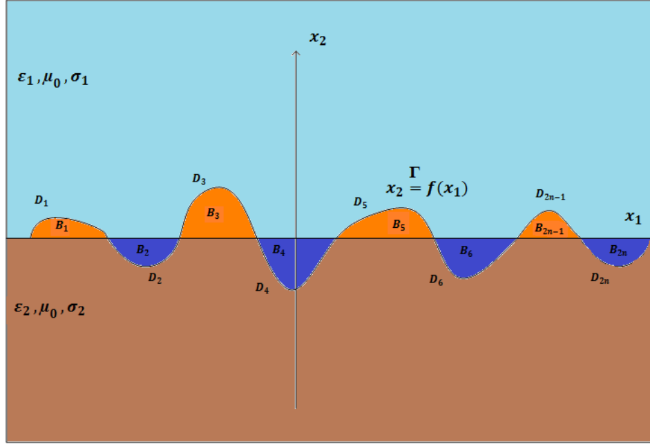
Şekil 2.2 : Düzgün ara kesitli iki parçalı uzay ve gömülü cisimler.
