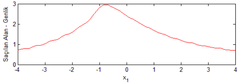
Şekil 5.14 : Örnek 6 için saçılan alan.
