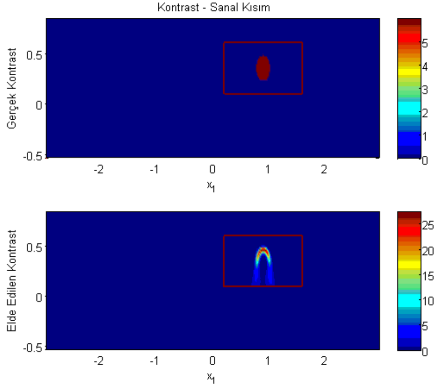
Şekil 5.3 : Örnek 1 için kontrast fonksiyonunun sanal kısımlarının karşılaştırılması.
