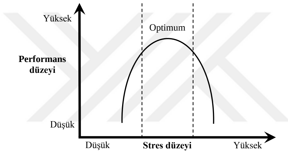
Şekil 2: Stres ve Performans Arasındaki Ters U İlişkisi
