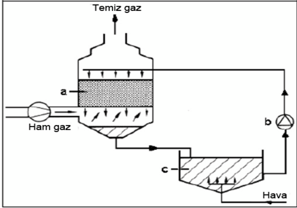
Şekil 2.6 : Biyo yıkayıcı.
