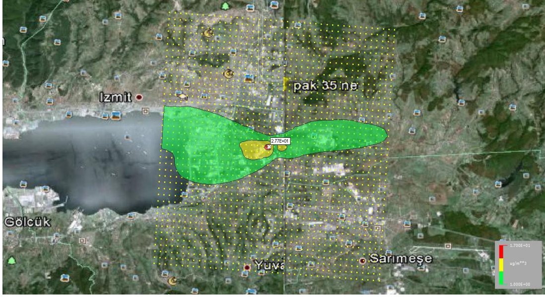
Şekil 7.7 : Yıllık konsantrasyon.
