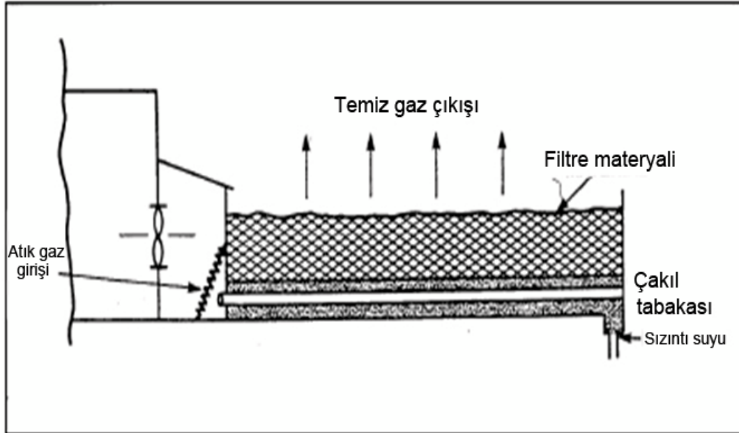
Şekil 2.5 : Biyofiltrasyon.
