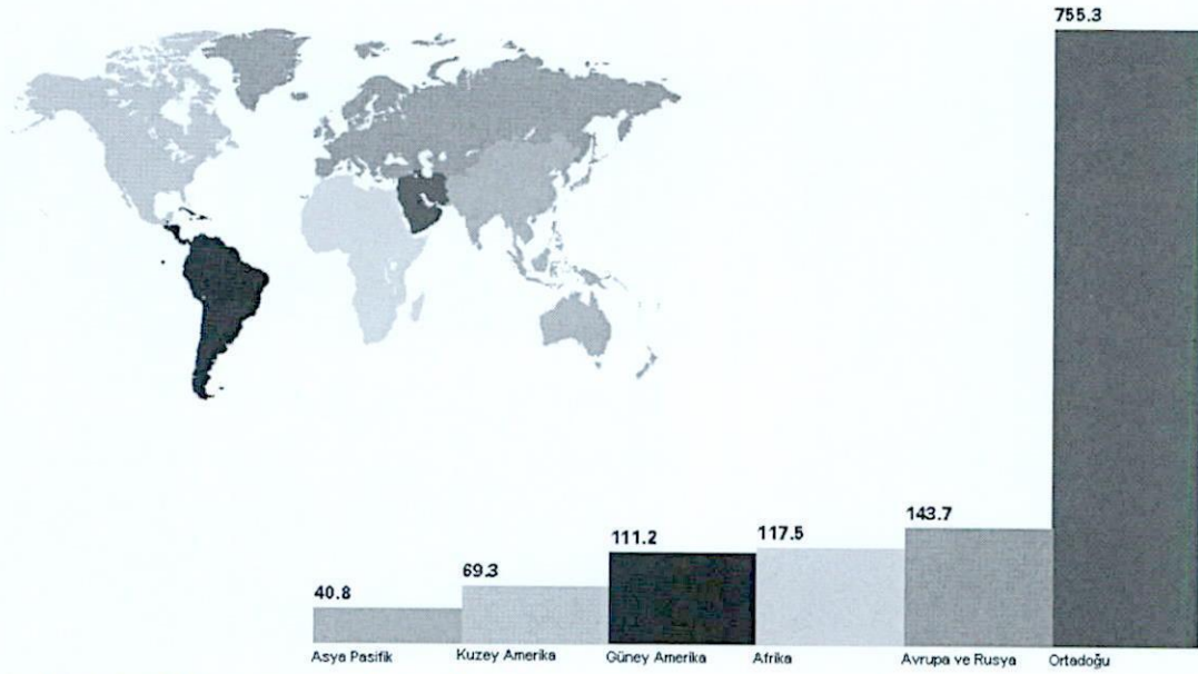
Şekil-5: 2007 Yılı İtibariyle Dünya İspatlanmış Petrol Rezervleri (Milyar Varil) (BP Statistical Review of World Energy [web], 2008)
