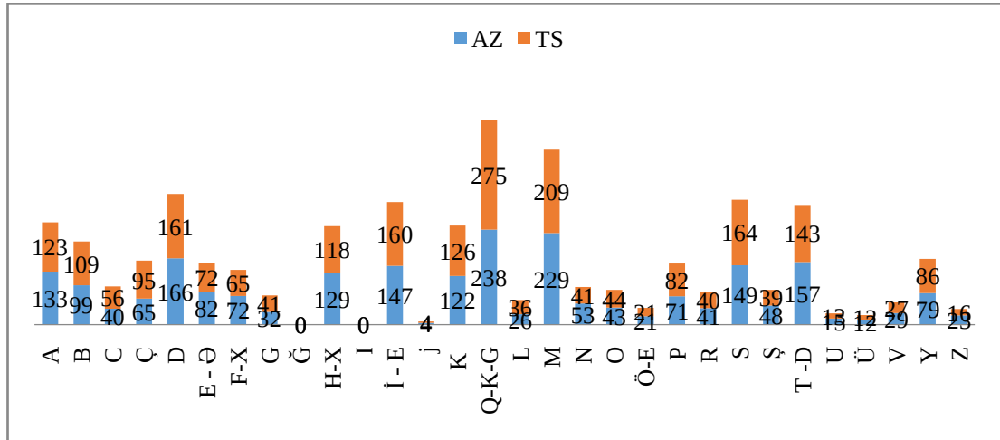
Şekil 1.2.3. Kısmi yalancı eş değer çok anlamlı adlar
