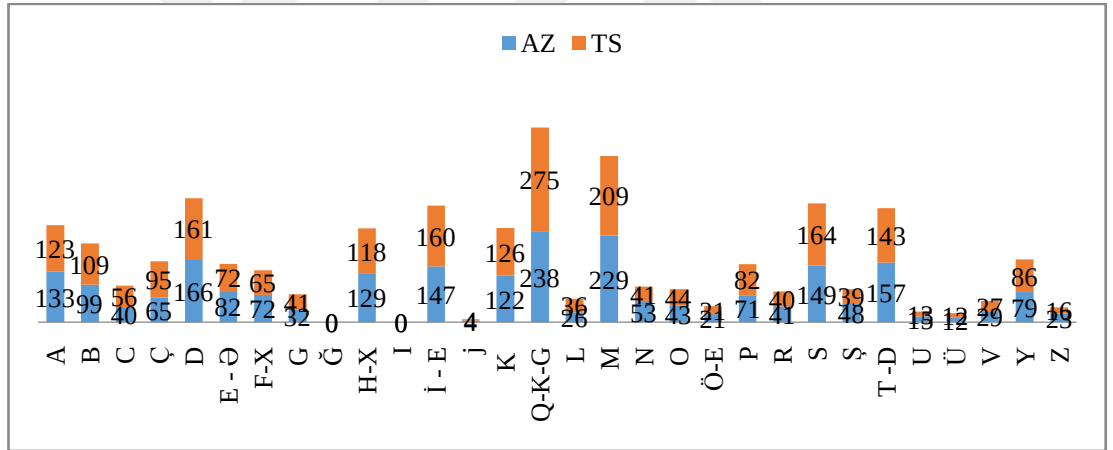
Şekil 1.2.2. Tam yalancı eş değer çok anlamlı adlar
