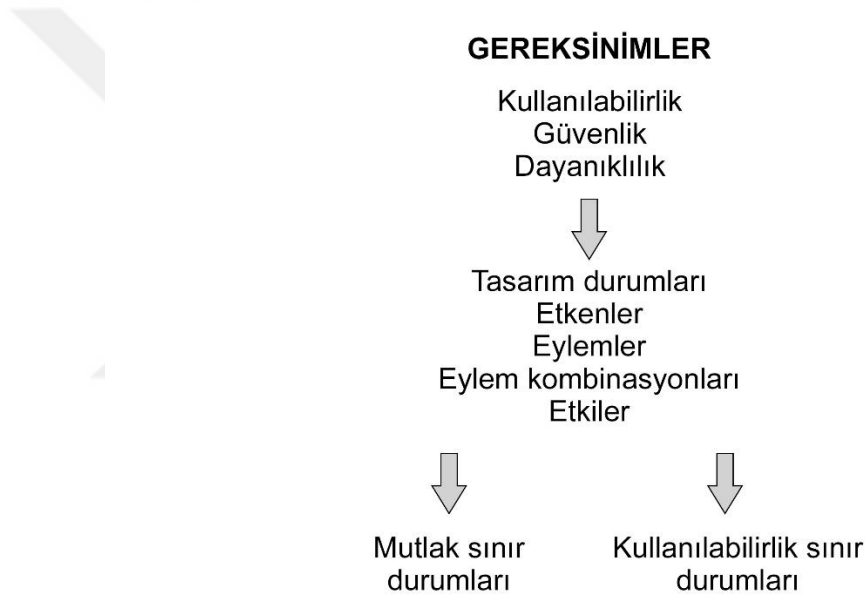
Şekil 2.18: Tasarım prosedüründe kullanılan gereksinimler ve terminoloji [39].
