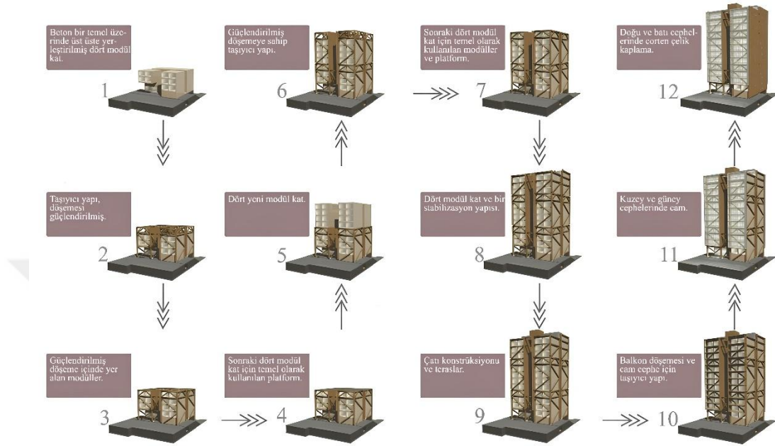
Şekil 3.19: Yapının taşıyıcı sistem diyagramı ([55]'den uyarlanarak görselleştirilmiştir).
