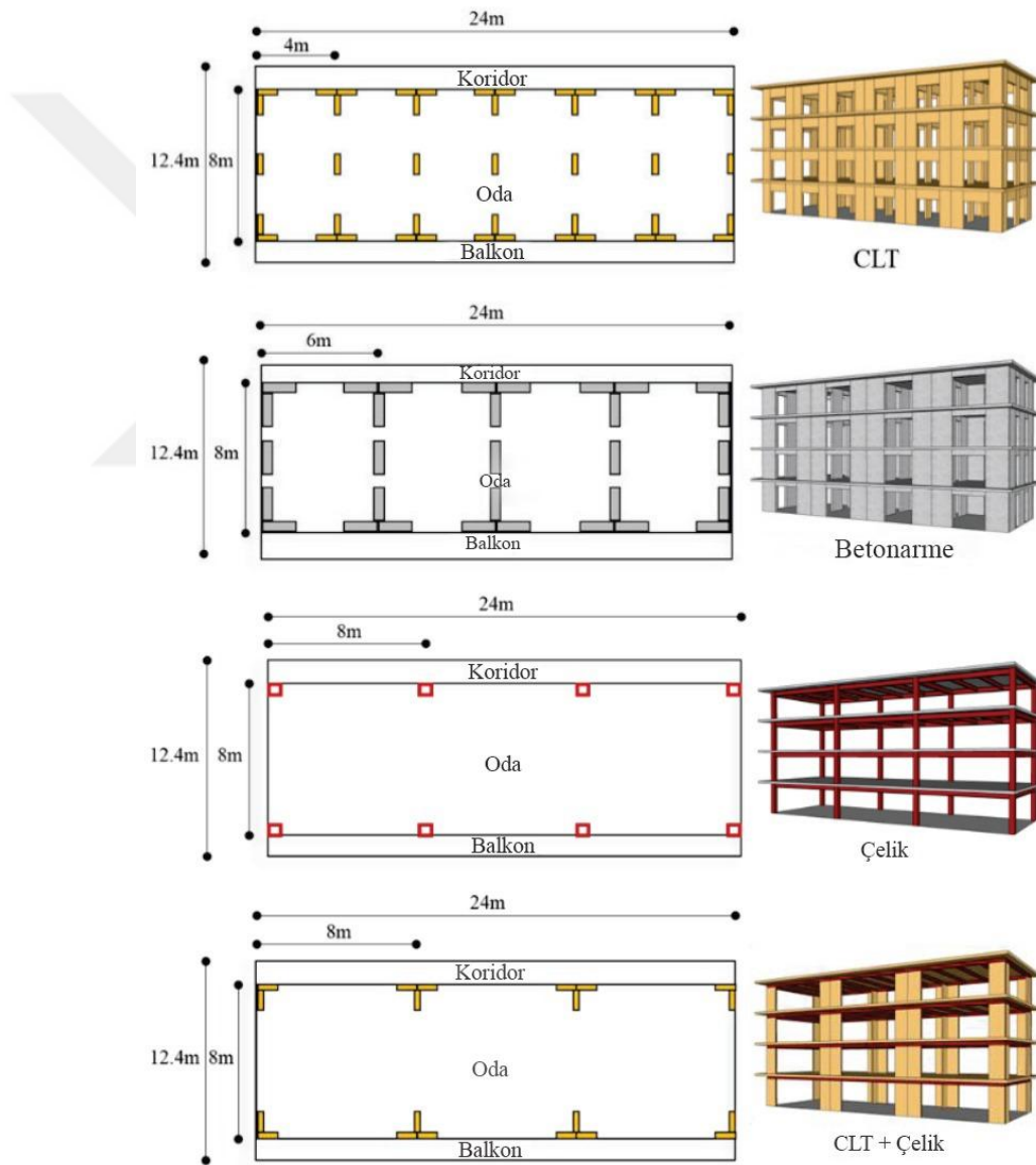
Şekil 3.16: Önerilen CLT-çelik hibrit sistem ve diğer CLT, betonarme, çelik sistem yapılar ve plan çizimleri [53].
