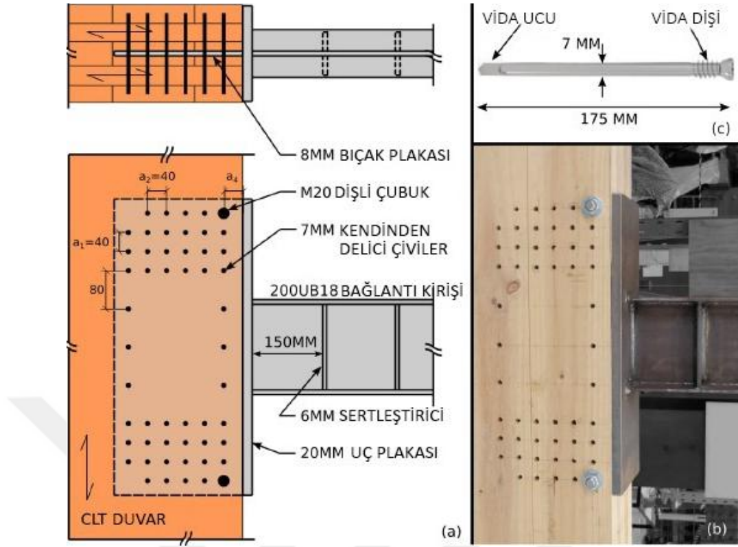
Şekil 3.5: CLT duvar ile çelik bağlantı kirişi arasındaki bağlantı detayı ve kendinden delici vida [48].
