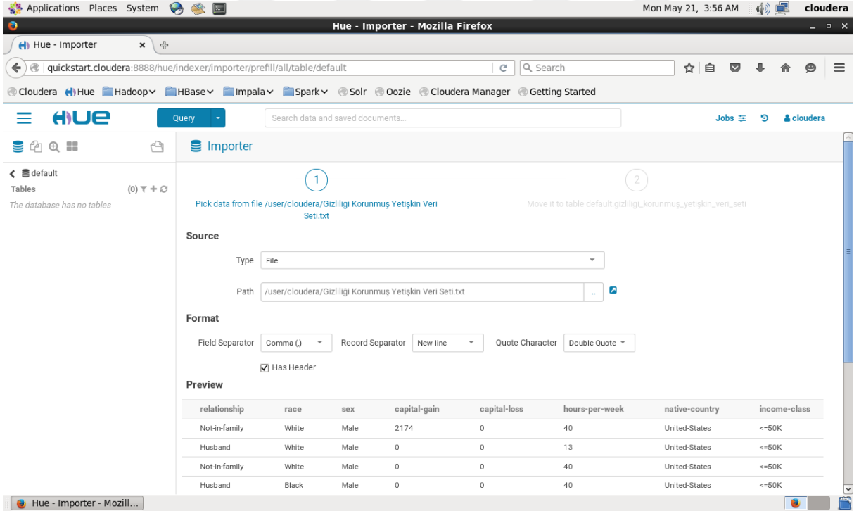
Şekil 3.24: Oluşturulacak tablo için alan ayırıcı ve kayıt ayırıcının ayarlanması (2).
