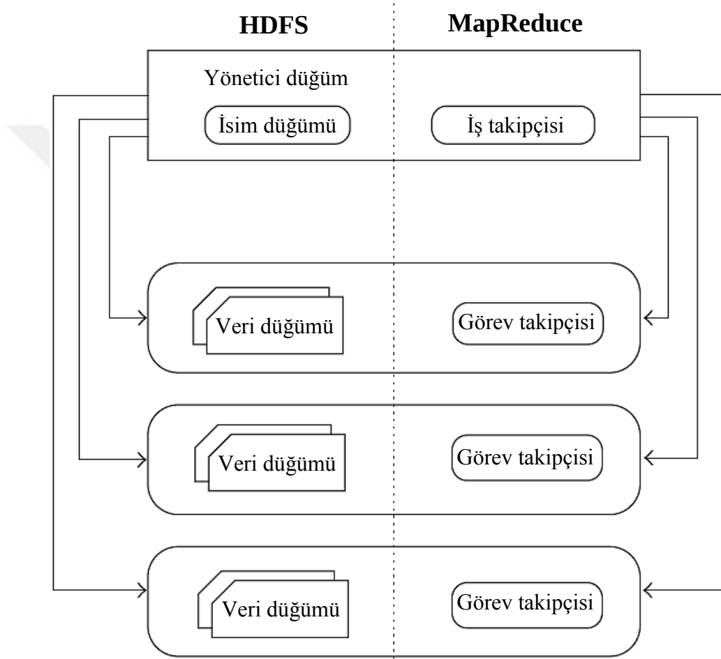
Şekil 2.11: HDFS ve MapReduce'un sistem mimarileri.
