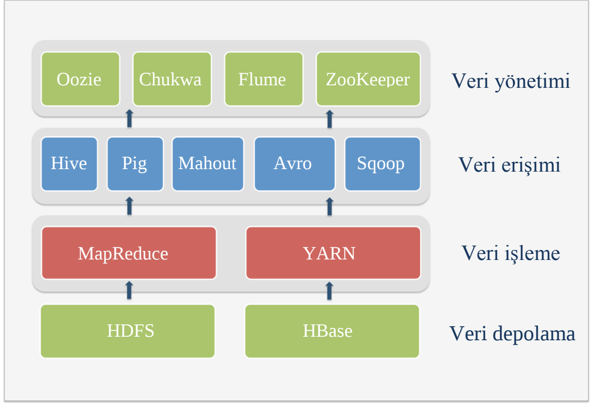
Şekil 2.10: Hadoop ekosistemi ve bileşenlerin ilişkisi.
