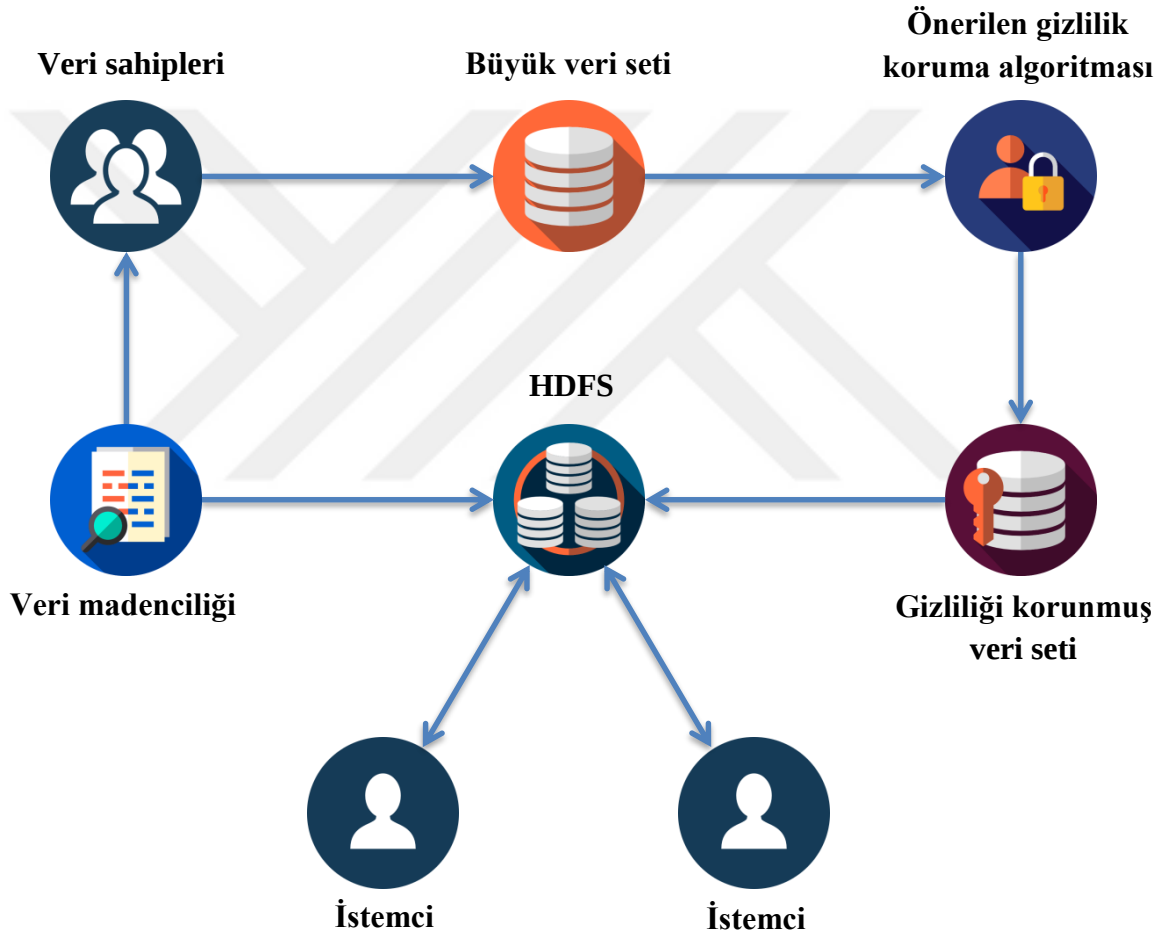
Şekil 3.7: Hadoop üzerinde gizlilik korumalı veri dağıtıklaştırma mimarisi.
