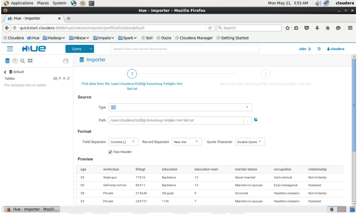
Şekil 3.23: Oluşturulacak tablo için alan ayırıcı ve kayıt ayırıcının ayarlanması (1).
