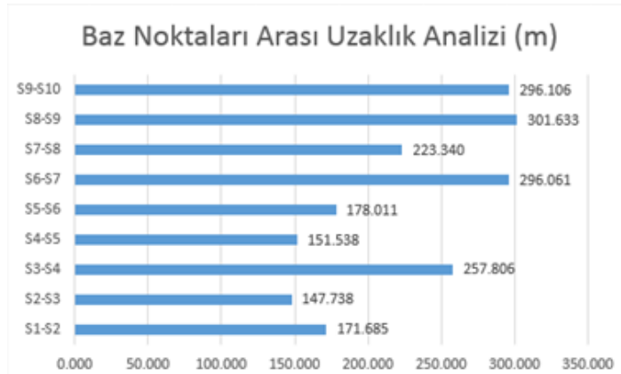
Şekil 3.22. Yer kontrol noktaları arası yatay uzunluk grafiği
