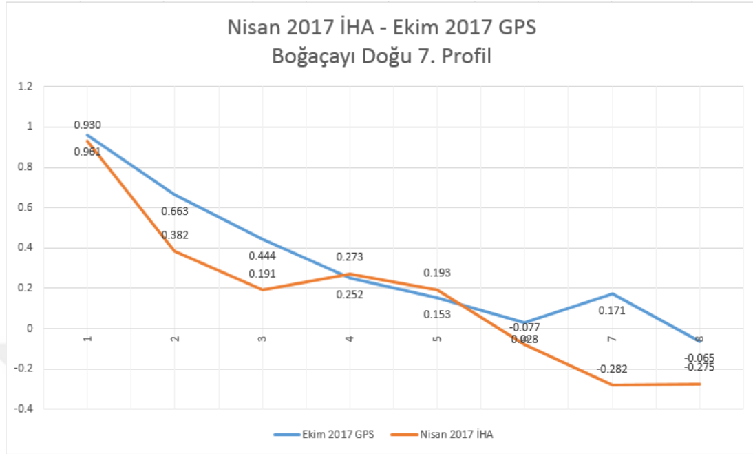
8.7. EK 7 Nisan 2017 İHA – Ekim 2017 GPS Boğaçayı Doğu 7. Profil
