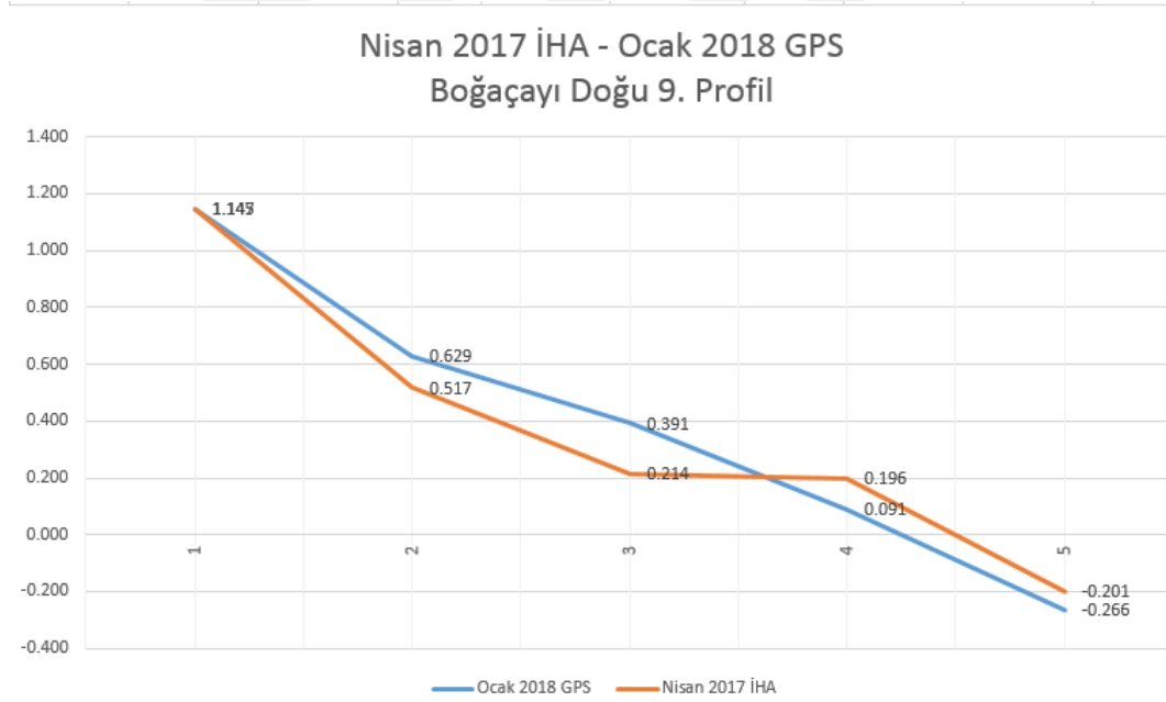
8.26. EK 26 Nisan 2017 İHA – Ocak 2018 GPS Boğaçayı Doğu 9. Profil
