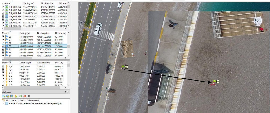
Şekil 3.31. Konyaaltı Boğaçayı taşınabilir YKN ITRF 96 koordinatı - resim koordinatı ilişkisinin kurulması
