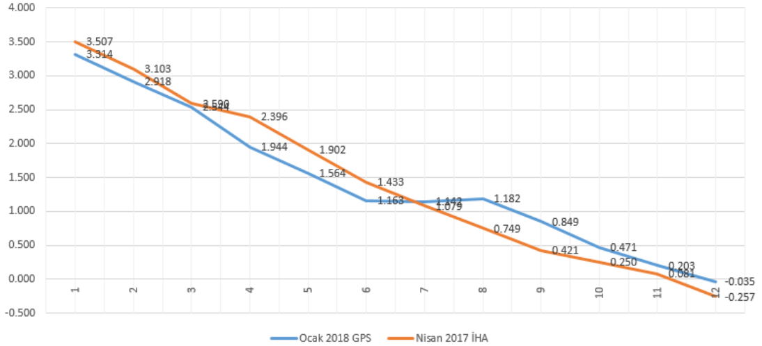
8.32. EK 32 Nisan 2017 İHA – Ocak 2018 GPS Boğaçayı Batı 5. Profil
