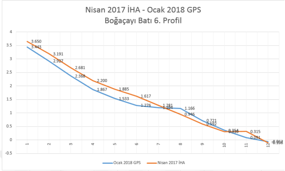
8.33. EK 33 Nisan 2017 İHA – Ocak 2018 GPS Boğaçayı Batı 6. Profil
