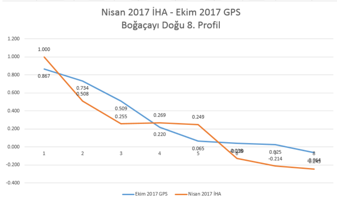
8.8. EK 8 Nisan 2017 İHA – Ekim 2017 GPS Boğaçayı Doğu 8. Profil
