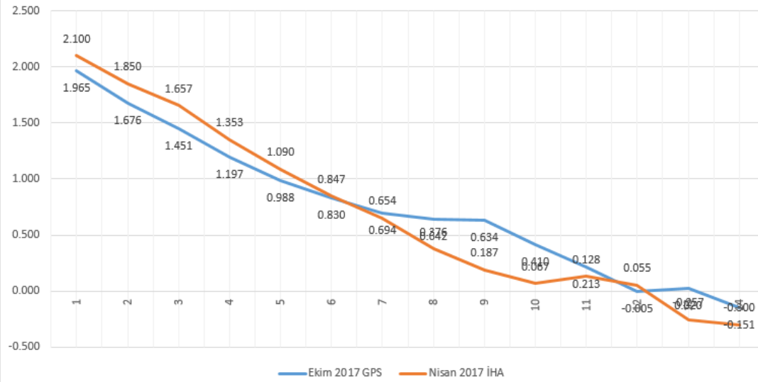
Nisan 2017 İHA - Ekim 2017 GPS Boğaçayı Doğu 10. Profil
