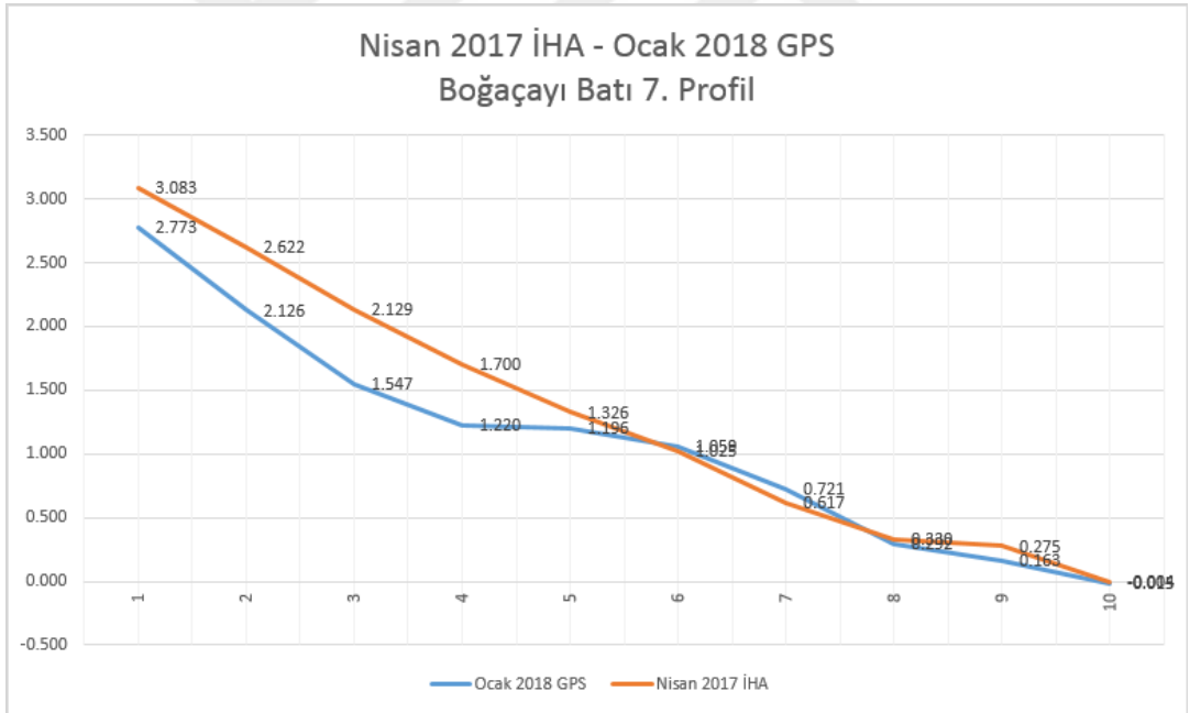
8.34. EK 34 Nisan 2017 İHA – Ocak 2018 GPS Boğaçayı Batı 7. Profil
