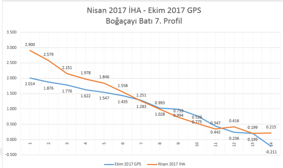
8.17. EK 17 Nisan 2017 İHA – Ekim 2017 GPS Boğaçayı Batı 7. Profil
