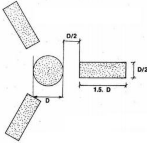
Şekil 3.24. BÖHY'ye göre olması gereken hava işaretçisi
