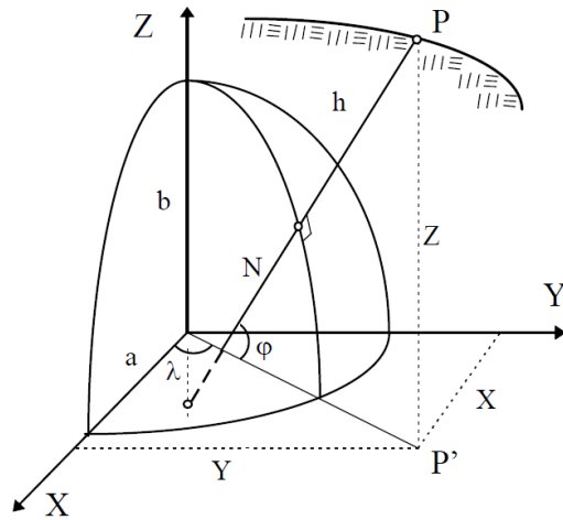
Şekil 3.33. Elipsoital dik ve eğri koordinatlar (Üstün, 1996)
