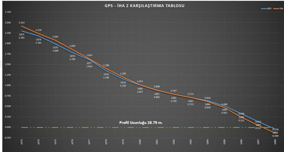
Şekil 6.1. Boğaçayı doğusu 3. Profil 15 Ekim 2016 İHA – 23 Ekim 2016 GPS profil karşılaştırması
