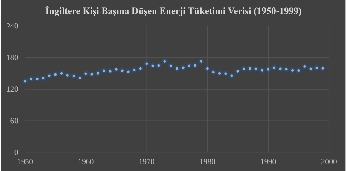
Şekil 4-107. İngiltere Kişi Başına Düşen Enerji Tüketimi Verisi (1950-1999)
