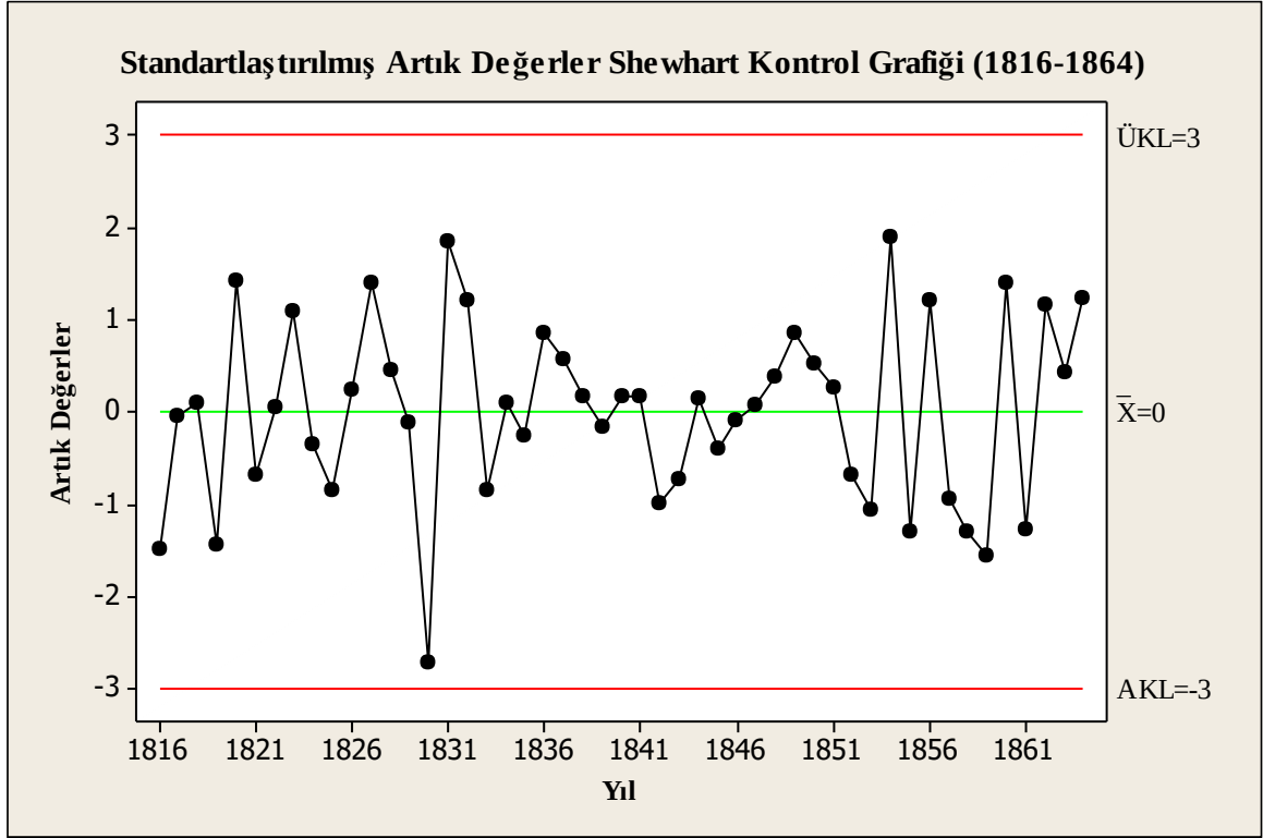
Şekil 4-46. Standardlaştırılmış Artık Değerler Shewhart Kontrol Grafiği (1816-1864)
