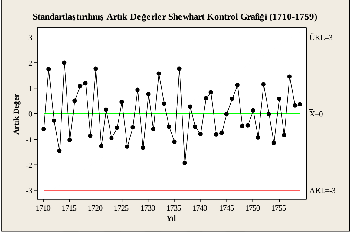
Şekil 4-5. Standardlaştırılmış Artık Değerler Shewhart Kontrol Grafiği (1710-1759)
