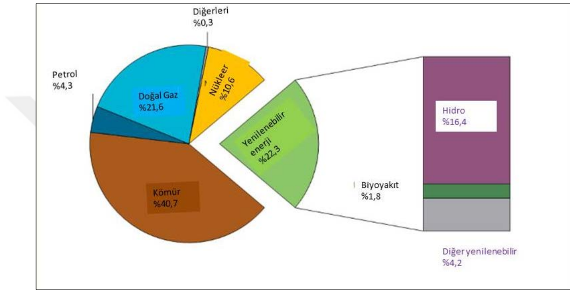
Şekil 2.3. 2014 yılına ait Dünya toplam birincil enerji arzı (IEA 2016)
