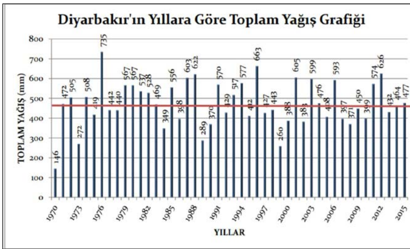
Şekil 4.4. : Diyarbakır İli İçin 1970-2015 Yılları Arası Yıllık Ortalama Yağış Miktarları (Kg/m 2 ) (Kaynak: Türkiye Meteorolojik Veri Arşivi)
