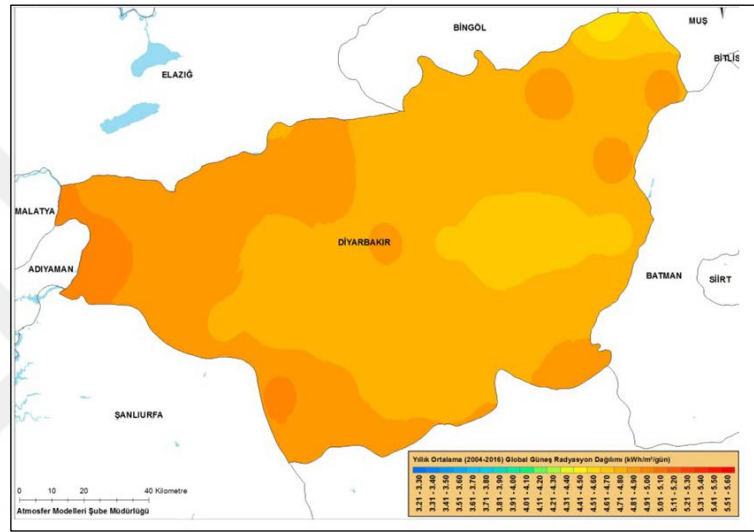
Şekil 4.5. Diyarbakır ili Güneş Enerji Potansiyel Haritası
