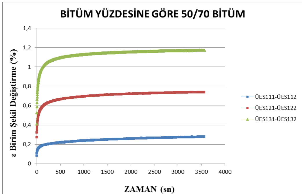
Şekil 4.13. Üç eksenli statik 50/70 bitümde 3 farklı bitüm yüzdesinde zamana göre yüzdesel şekil değişimi
