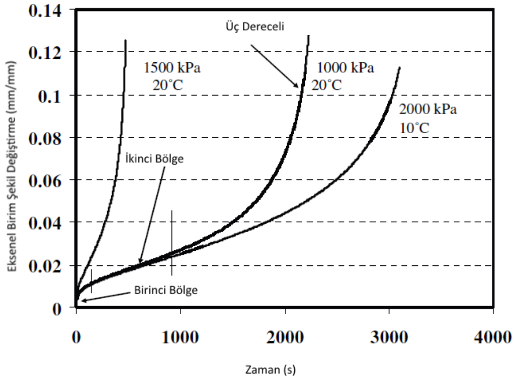
Şekil 2.7. Tek eksenli deney sonuçları (Taherkhania, 2011)
