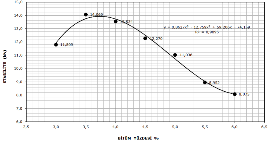
Şekil 4.2. Stabilite - Bitüm yüzdesi grafiği
