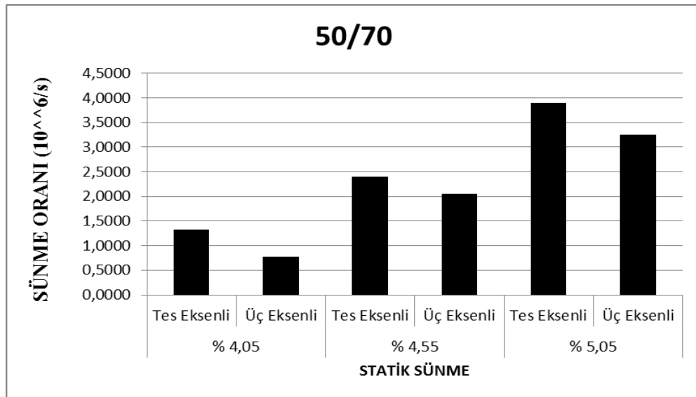
Şekil 4.17. 50/70 bitüm statik sünme deneyi sünme oranları karşılaştırılmalı sonuçları
