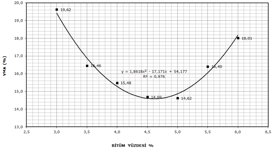
Şekil 4.4. VMA – Bitüm yüzdesi grafiği
