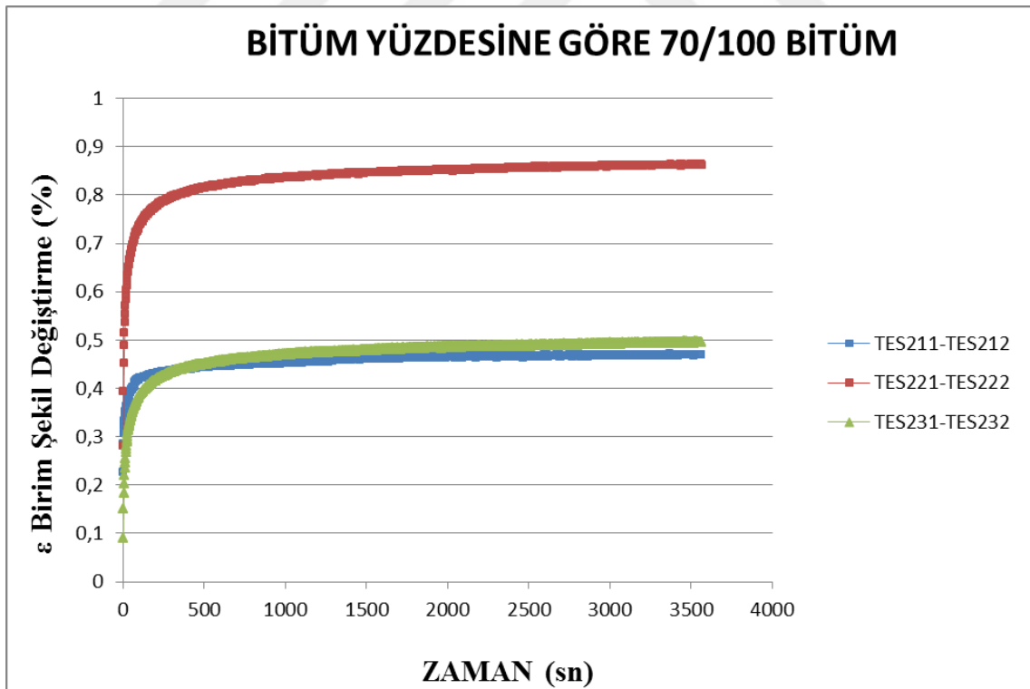
Şekil 4.9. Tek eksenli statik 70/100 bitümde 3 farklı bitüm yüzdesinde zamana göre yüzdesel şekil değişirme
