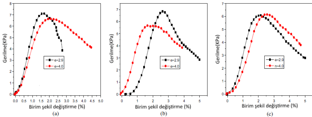
Şekil 2.6. (a) 90 mm, (b) 100 mm ve (c) 105 mm yükseklikleri için farklı boşluk oranlarında gerilme-birim şekil değiştirme eğrileri (Zhang ve ark., 2015)
