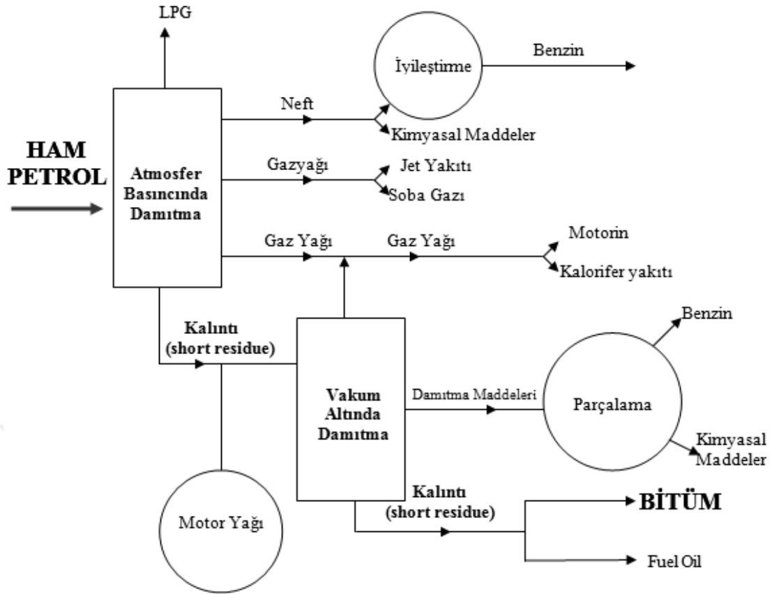
Şekil 3.1. Bitümün elde edilme aşamaları (Lav ve Lav, 2004)
