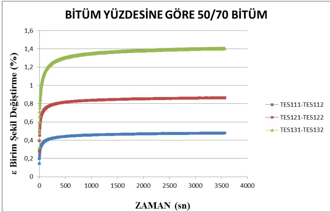
Şekil 4.8. Tek eksenli statik 50/70 bitümde 3 farklı bitüm yüzdesinde zamana göre yüzdesel şekil değişirme
