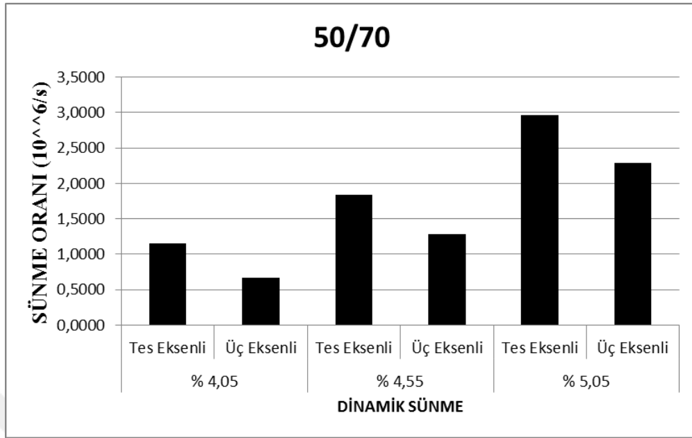
Şekil 4.18. 50/70 bitüm dinamik sünme deneyi sünme oranları karşılaştırılmalı sonuçları
