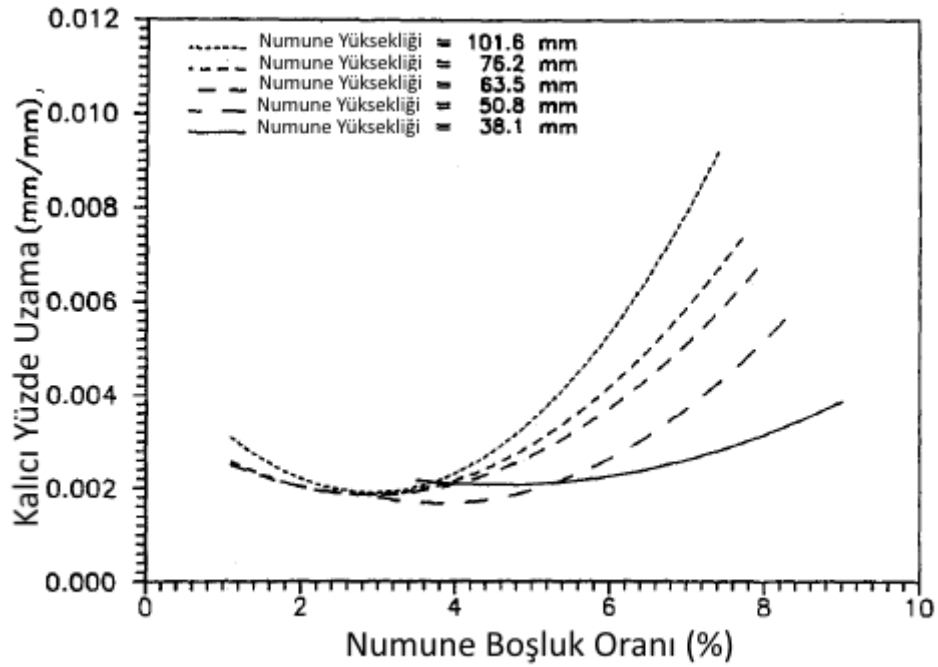
Şekil 2.13. Tek eksenli deneyi farklı yüksekliklerdeki test sonuçları (Brown ve Foo, 1994)
