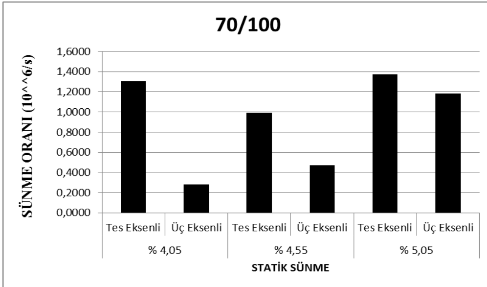
Şekil 4.19. 70/100 bitüm statik sünme deneyi sünme oranları karşılaştırılmalı sonuçları
