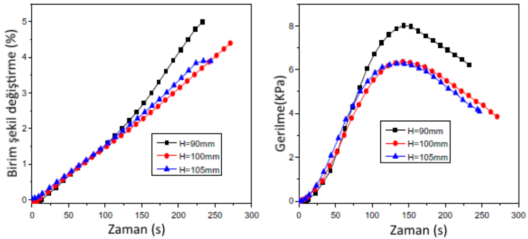
Şekil 2.5. Hava boşluğu içeriği % 5,7 olan farklı yüksekliklerdeki numuneler için birim şekil değiştirme-zaman ve gerilme-zaman eğrileri (Zhang ve ark., 2015)
