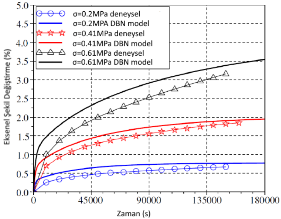
Şekil 2.9. 10 °C’de üç farklı gerilme seviyesinde deneysel değerlerin ve DBN modeli gösterimi (Sohm ve ark., 2010)
