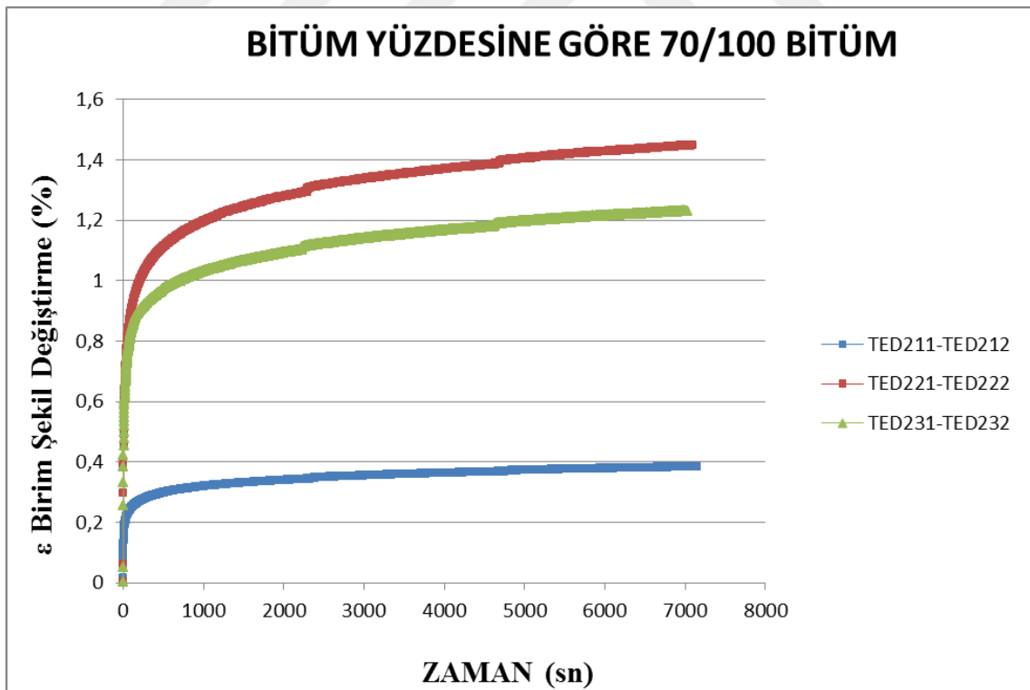
Şekil 4.11. Tek eksenli dinamik 70/100 bitümde 3 farklı bitüm yüzdesinde zamana göre yüzdesel şekil değişirme
