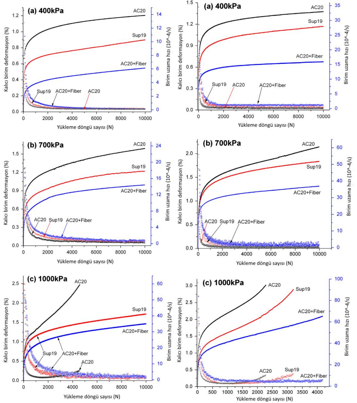
Şekil 2.12. Sol: Üç eksenli deney sonuçları – Sağ: Kısmi üç eksenli deney sonuçları (Xu ve ark., 2014)
