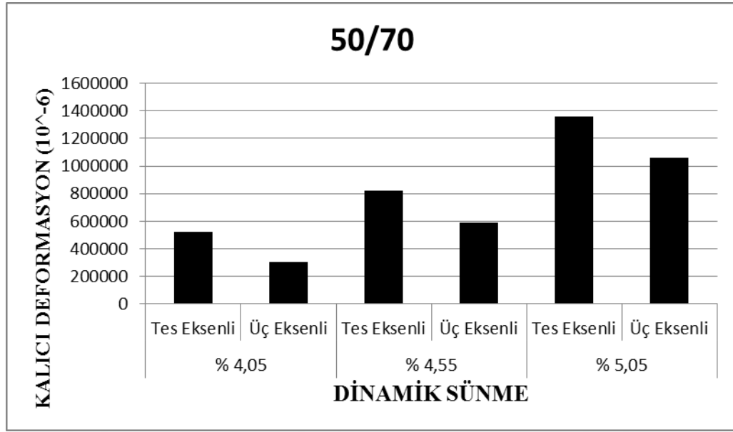
Şekil 4.22. 50/70 bitüm dinamik sünme deneyi kalıcı deformasyonları karşılaştırılmalı sonuçları
