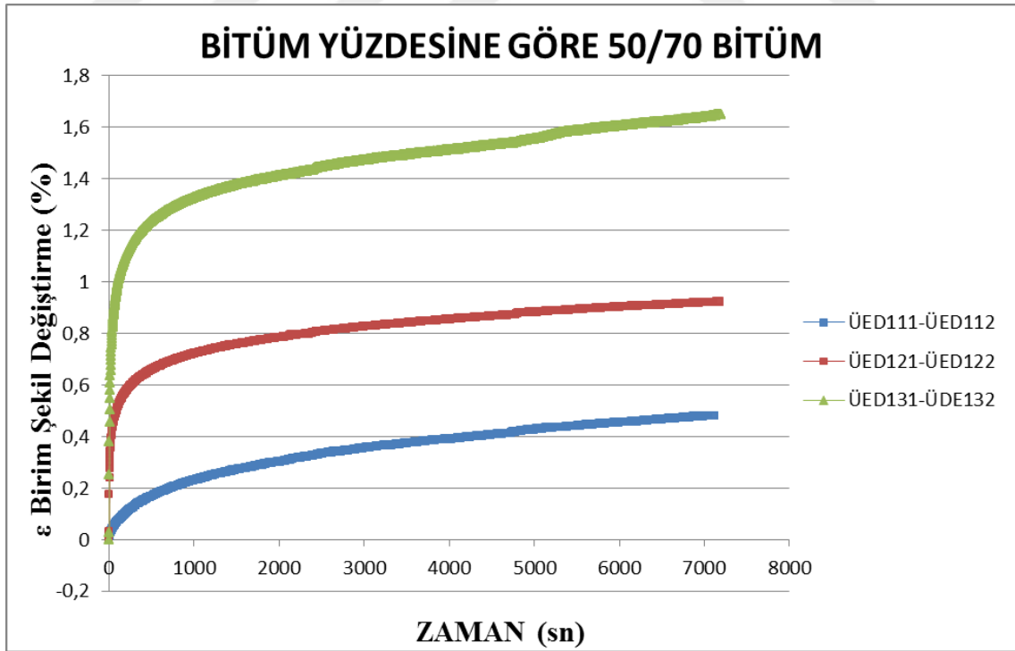
Şekil 4.15. Üç eksenli dinamik 50/70 bitümde 3 farklı bitüm yüzdesinde zamana göre yüzdesel şekil değiştirme
