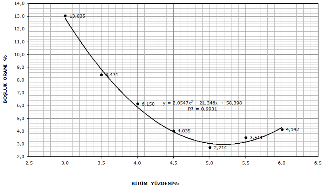
Şekil 4.3. Boşluk oranı – Bitüm yüzdesi grafiği
