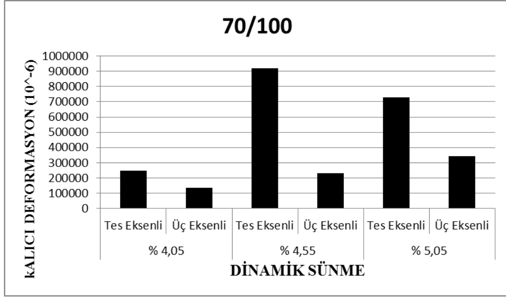
Şekil 4.24. 70/100 bitüm dinamik sünme deneyi kalıcı deformasyonları karşılaştırılmalı sonuçları
