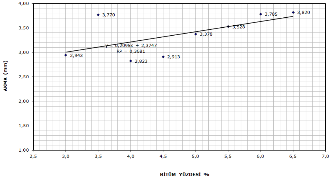
Şekil 4.5. Akma – Bitüm yüzdesi grafiği
