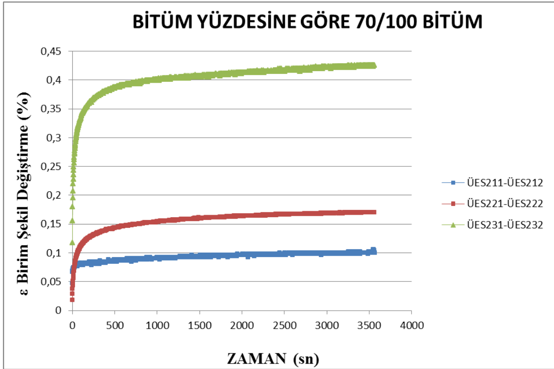
Şekil 4.14. Üç eksenli statik 70/100 bitümde 3 farklı bitüm yüzdesinde zamana göre yüzdesel şekil değiştirme
