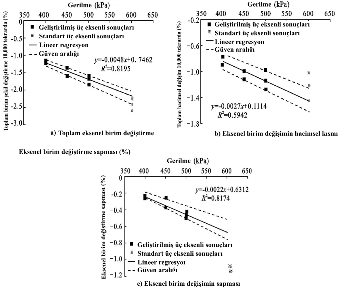
Şekil 2.2. Standart ve geliştirilmiş üç eksenli deneyleri arasındaki sonuç farkları (Hofko, 2015)
