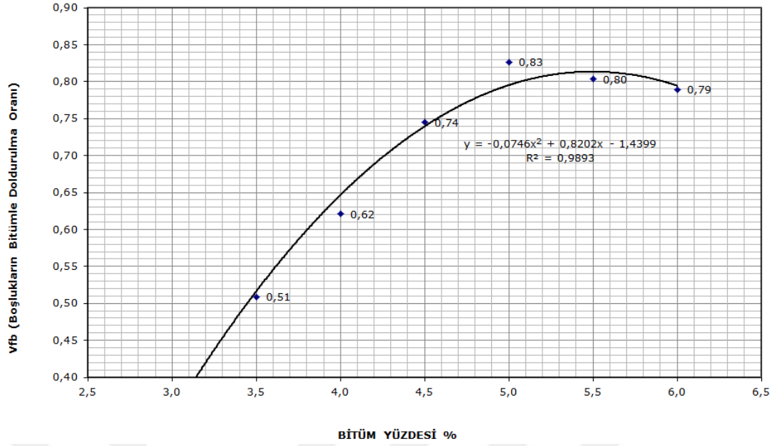
Şekil 4.6. Vfb - Bitüm yüzdesi grafiği
