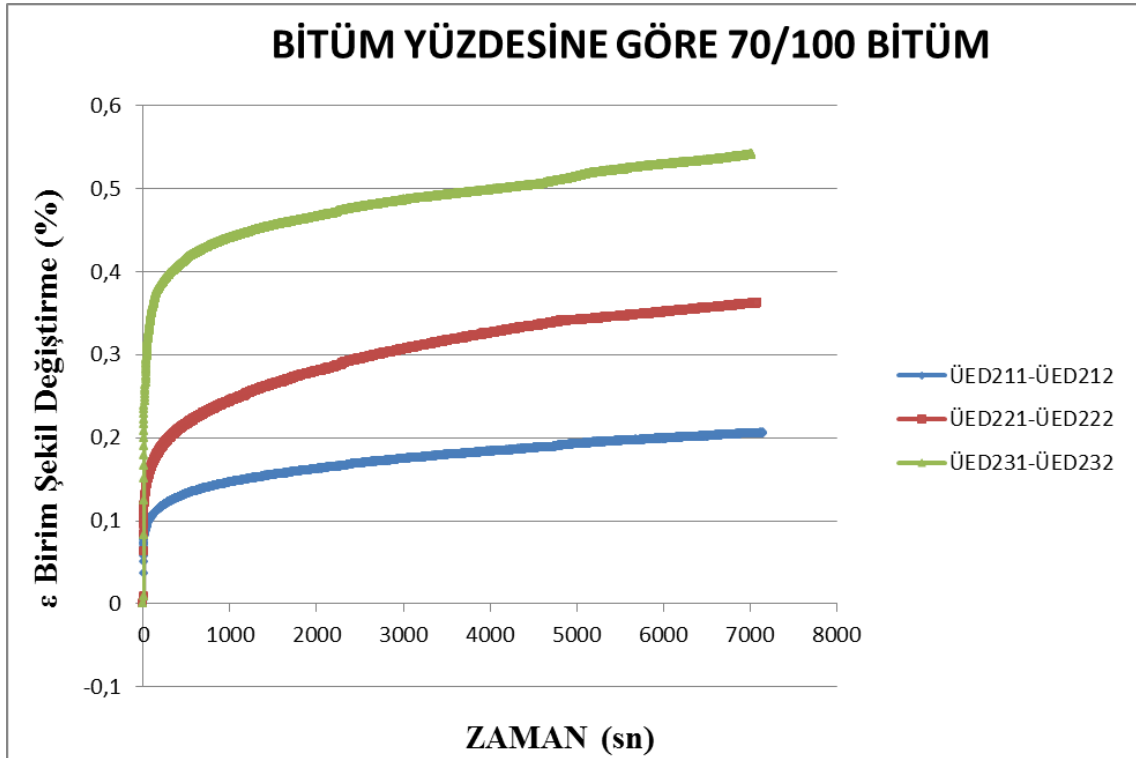
Şekil 4.16. Üç eksenli dinamik 70/100 bitümde 3 farklı bitüm yüzdesinde zamana göre yüzdesel şekil değişirme
