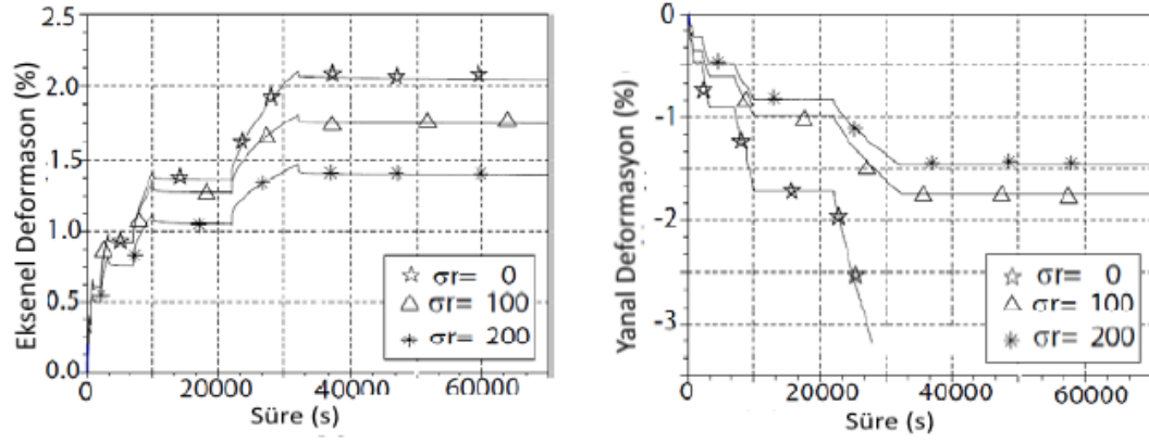
Şekil 2.10. Farklı yanal basınçlarda Eksenel deformasyon - Süre ve Yanal deformasyon - Süre grafikleri (Blanc ve ark., 2015)
