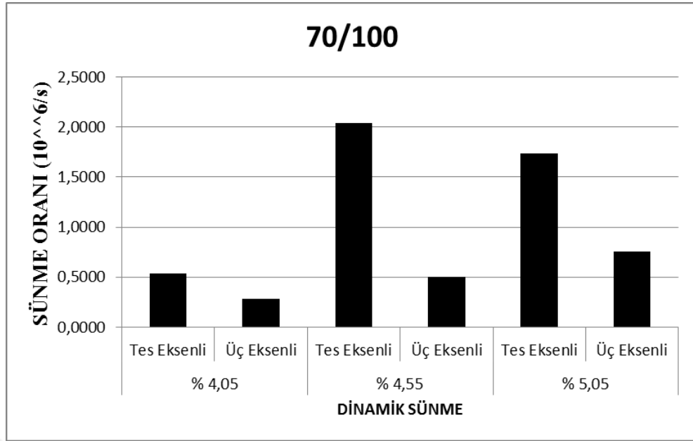
Şekil 4.20. 70/100 bitüm dinamik sünme deneyi sünme oranları karşılaştırılmalı sonuçları
