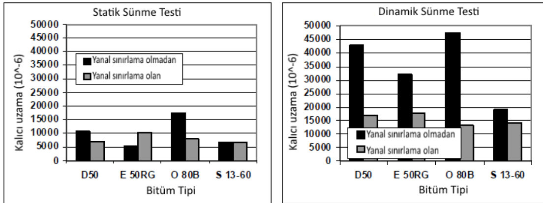
Şekil 2.4. Statik ve dinamik testleri kalıcı çekme sonuçları (Dołzycki ve Judycki, 2008)
