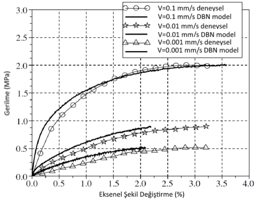
Şekil 2.8. 20 °C'de üç farklı uzama oranında DBN modeli ve deneysel değerlerin gösterimi (Sohm ve ark., 2010)
