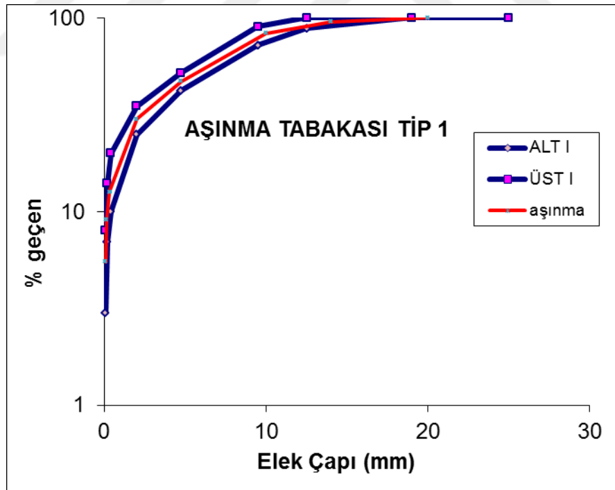
Şekil 3.4. Agrega gradasyon eğrisi
