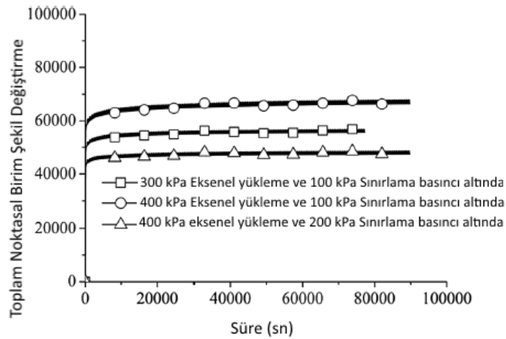
Şekil 2.15. 60 °C’de üç farklı koşulda gerçekleştirilen testlerin sürünme eğrileri (Gayathri ve ark., 2016)
