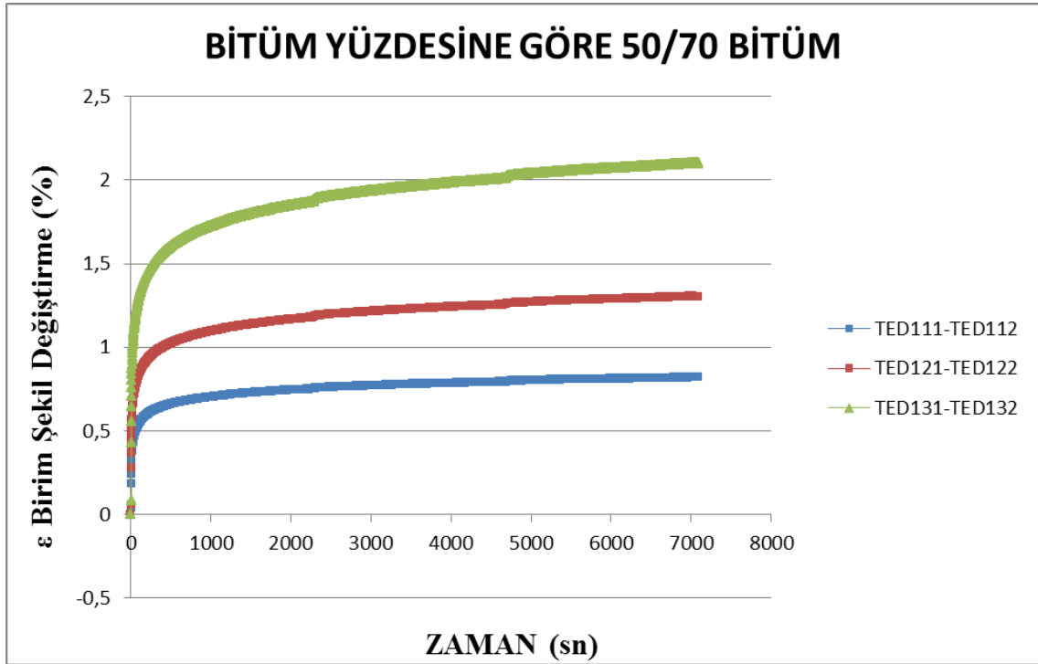
Şekil 4.10. Tek eksenli dinamik 50/70 bitümde 3 farklı bitüm yüzdesinde zamana göre yüzdesel şekil değişirme
