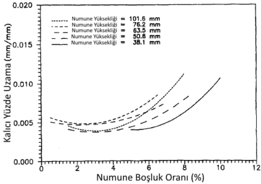
Şekil 2.14. Üç eksenli deneyi farklı yüksekliklerdeki test sonuçları (Brown ve Foo, 1994)
