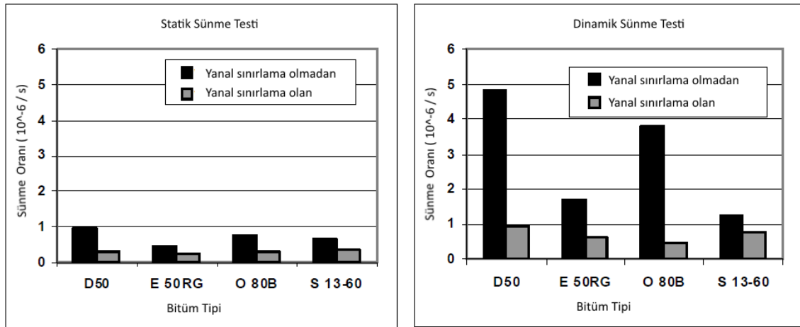
Şekil 2.3. Statik ve dinamik testleri sünme oranları (Dołzycki ve Judycki, 2008)
