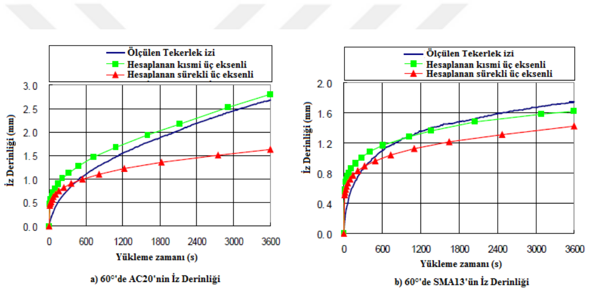
Şekil 2.1. 60 °C’de ölçülen tekerlek izi ile hesaplanmış arasındaki karşılaştırmalar (Huang ve Zhang, 2010)
