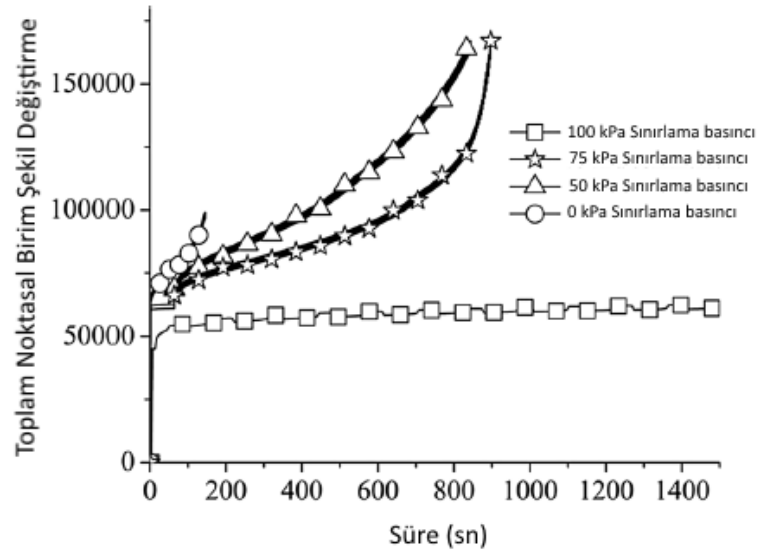
Şekil 2.16. 60 °C'de 600 kPa yükleme altında farklı sınırlama basınçları ile elde edilen sürünme eğrileri (Gayathri ve ark., 2016)
