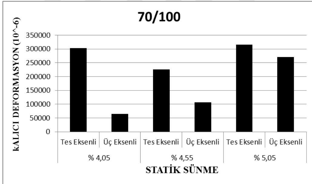
Şekil 4.23. 70/100 bitüm statik sünme deneyi kalıcı deformasyonları karşılaştırılmalı sonuçları
