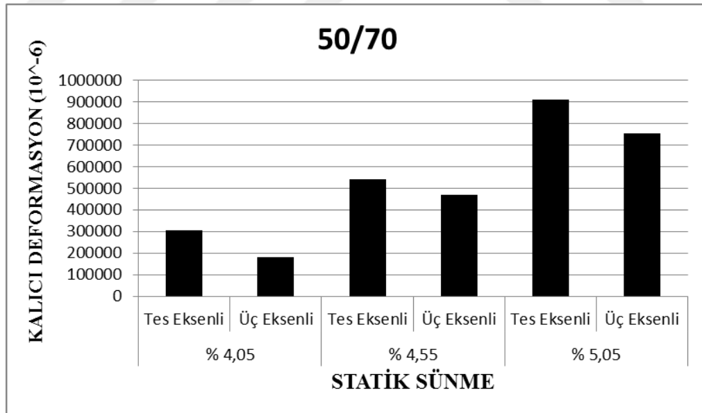
Şekil 4.21. 50/70 bitüm statik sünme deneyi kalıcı deformasyonları karşılaştırılmalı sonuçları
