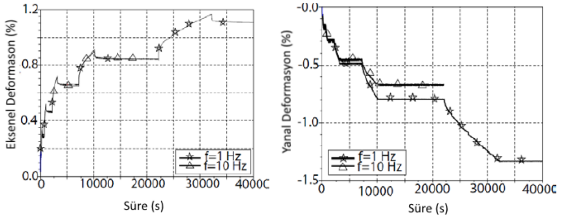
Şekil 2.11. Farklı yükleme frekanslarında Eksenel deformasyon – Süre ve Yanal deformasyon – Süre grafikleri (Blanc ve ark., 2015)
