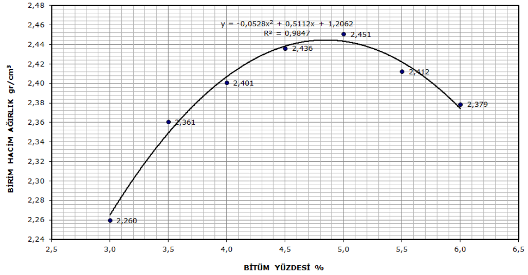
Şekil 4.1. Bitüm yüzdesi – Birim hacim ağırlık grafiği
