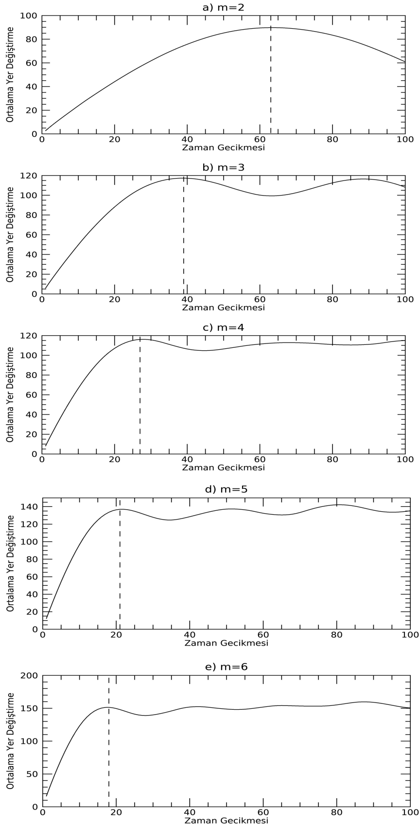
Şekil 4.5. a) 2 boyut; b) 3 boyut; c) 4 boyut; d) 5 boyut; e) 6 boyut için ortalama yer değişime fonksiyonu.
