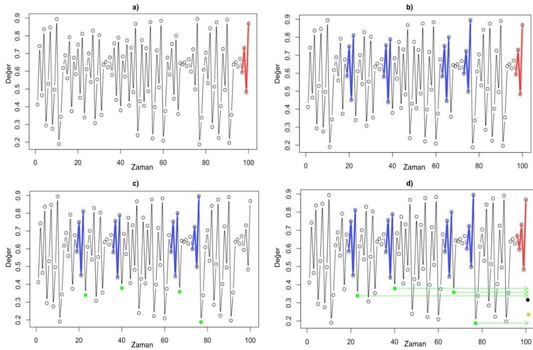
Şekil 3.4. Simplex Projection algoritması ile tahmin oluşturulma süreçleri.
