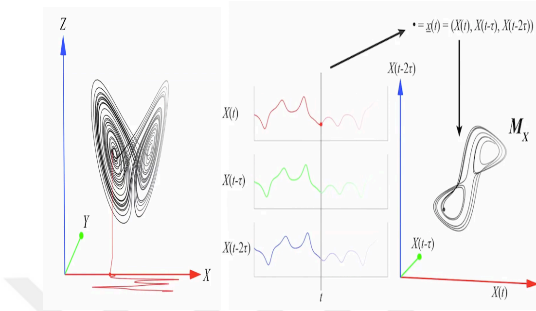
Şekil 3.3. Takens teoremi ile gölge-çekici oluşturulma sürecinin şekilsel gösterimi.
