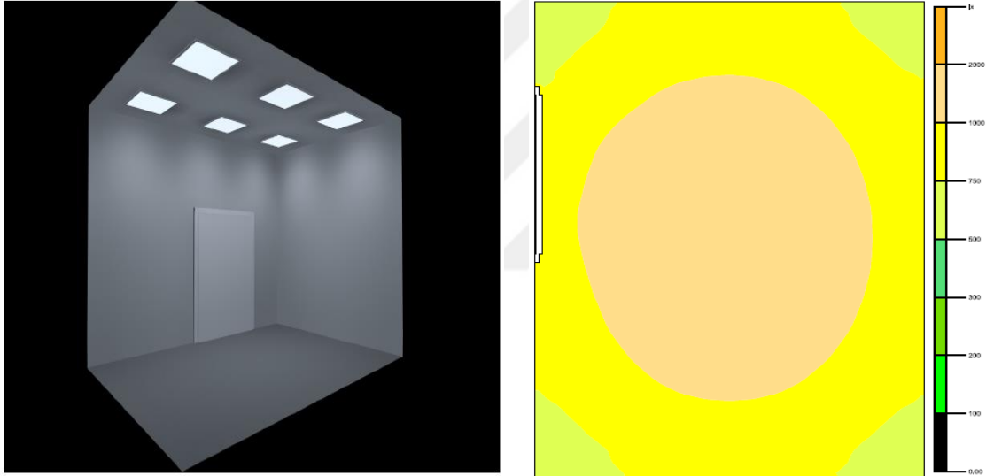
Şekil 3.26. İzolasyon odası 3 boyut aydınlatma araçlarının yerleşimi, aydınlık seviyeleri
