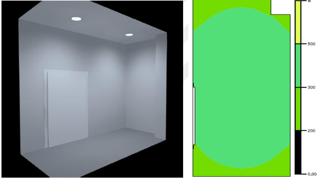
Şekil 3.37. Giriş engelli wc 3 boyut aydınlatma araçlarının yerleşimi, aydınlık seviyeleri
