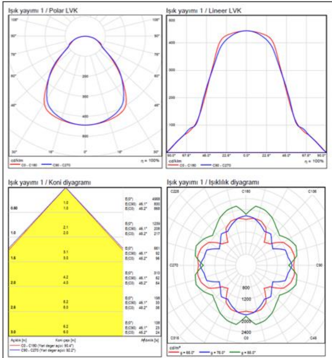
GWS2906S ASTRID 60X60 FULLPANEL e ait ışık yayım diyagramları
