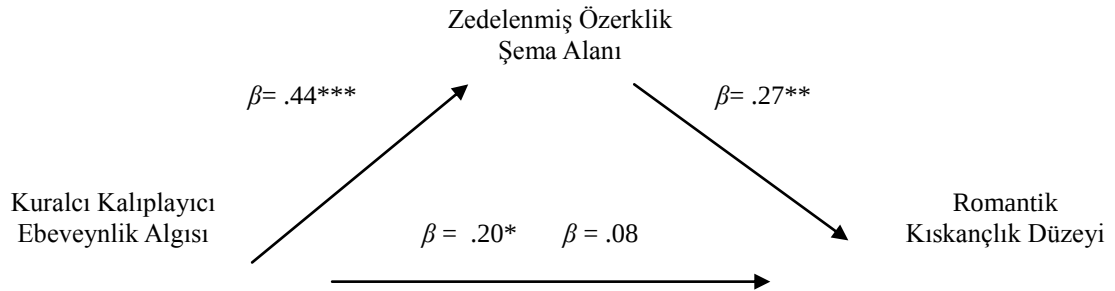
Şekil 3.1. Algılanan Kuralcı/Kalıplayıcı Ebeveynlik Biçiminin Romantik Kıskançlık Düzeyini Yordamasında Zedelenmiş Özerklik Şema Alanının Aracı Rolüne İlişkin Beta Katsayıları
