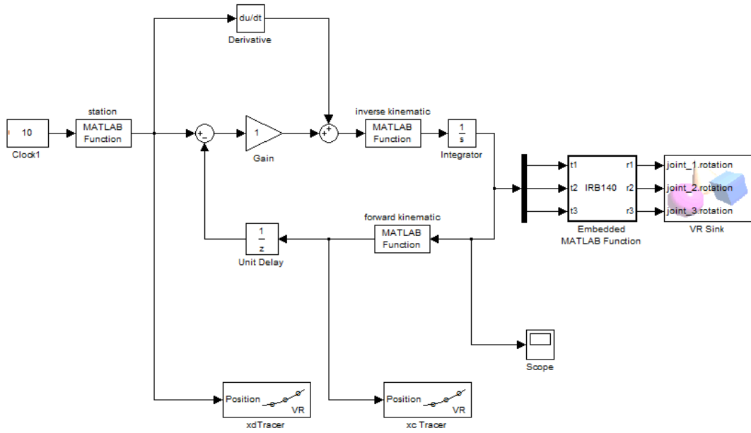
Şekil 2.11 : IRB 140 yörünge modeli.
