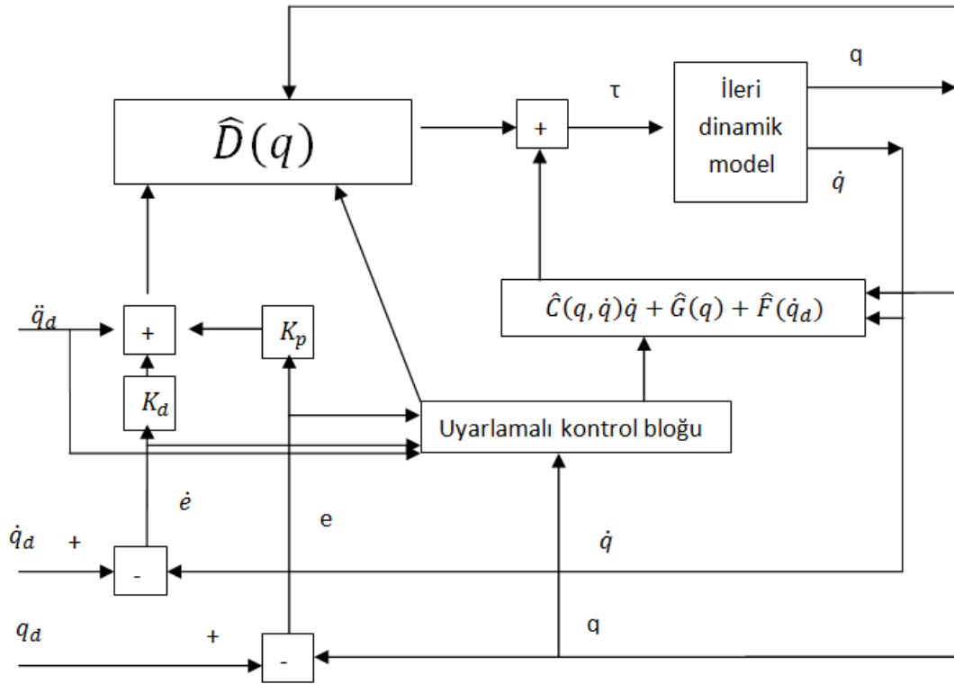
Şekil 6.1 : Uyarlamalı tork kontrol şeması.
