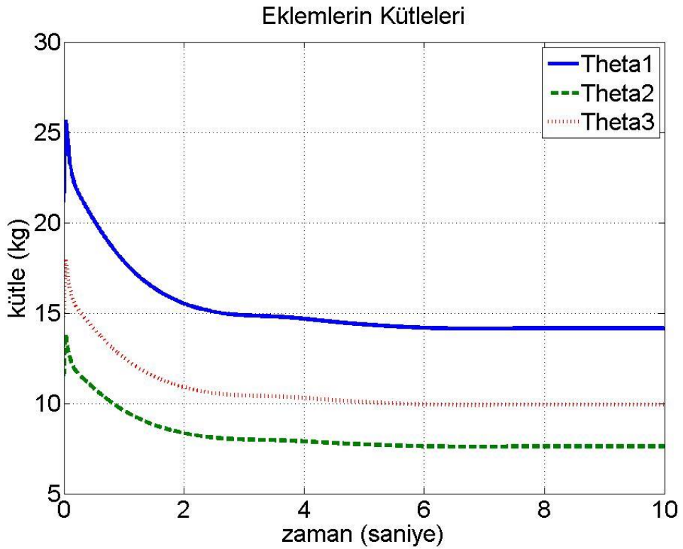
Şekil 6.16 : Eklemler kütleleri 1.5 ile çarpıldığında eklemlerin kütleleri.
