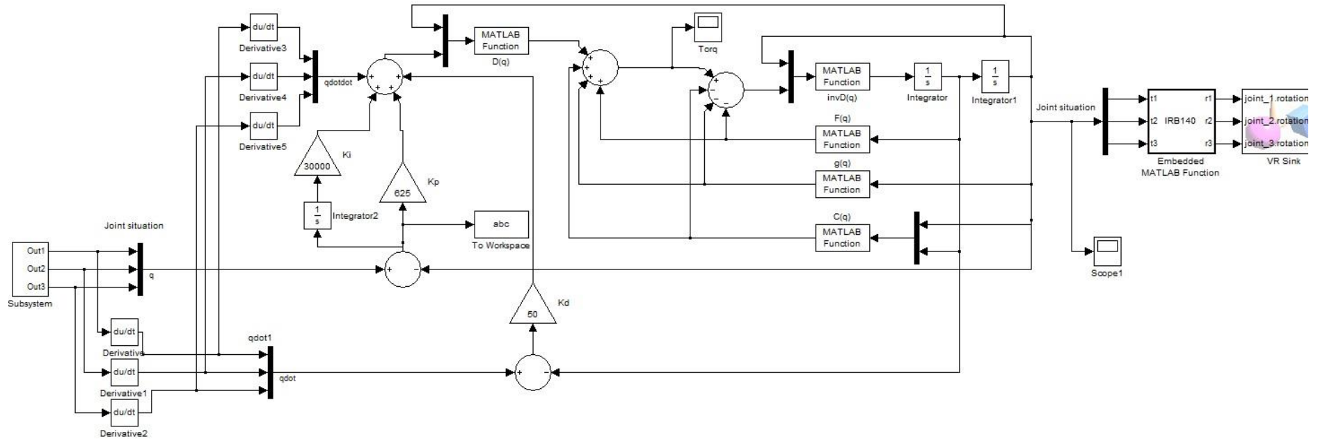
Şekil 5.15 : PID tork kontrol modeli.
