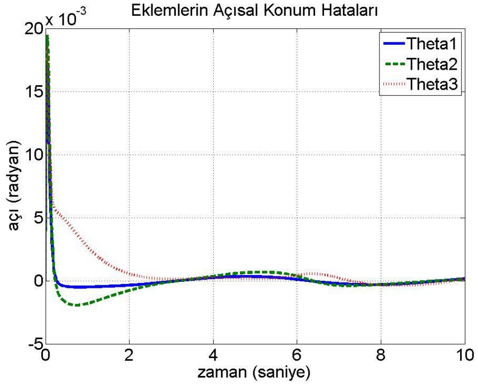
Şekil 6.15 : Eklemler kütleleri 0.5 ile çarpıldığında eklemlerin açısal konum hataları.
