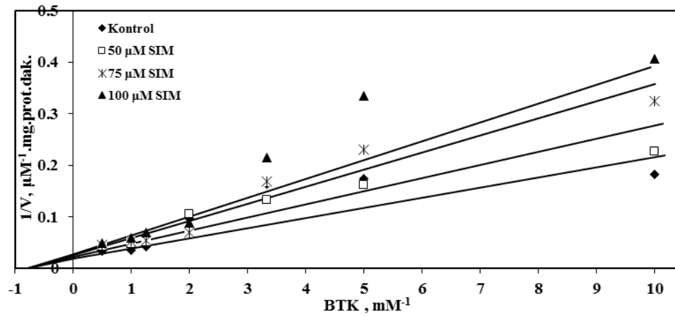
Şekil 4.22. Simvastatin-BKE, Lineweaver-Burk grafiğı.
