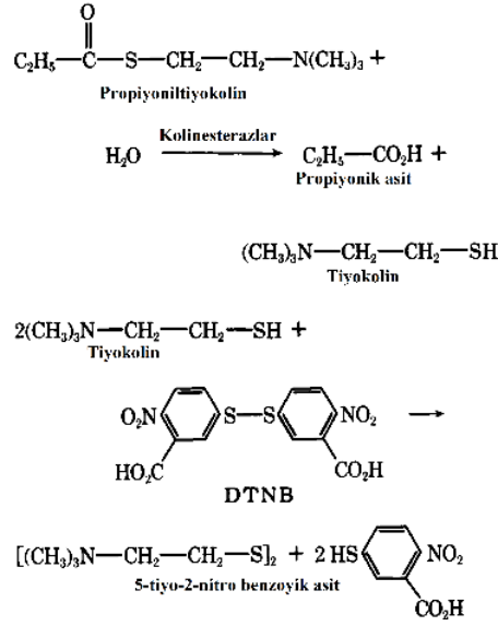
Şekil 3.1. Ellman reaksiyonu (94).
