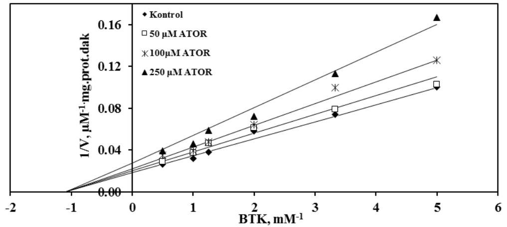
Şekil 4.16. Atorvastatin-BKE, Lineweaver-Burk grafiğı.
