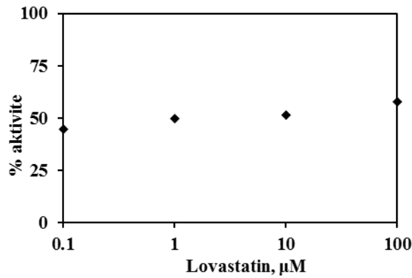
Şekil 4.23. Lovastatin-AKE % aktivite grafiği.
