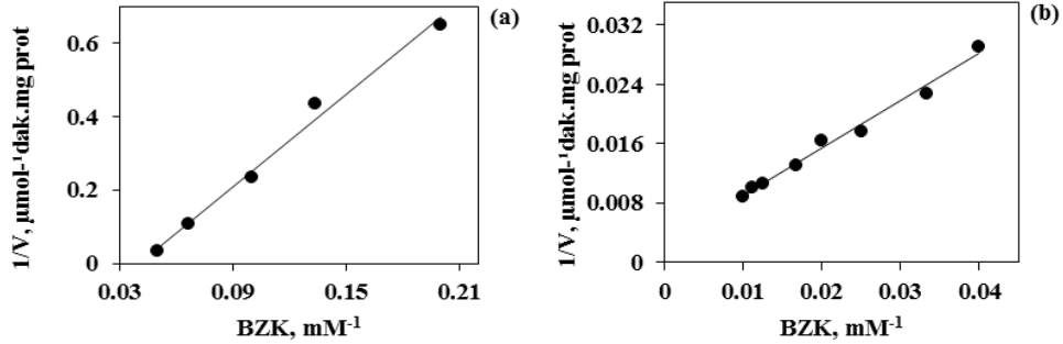
Şekil 4.12. BZK için Lineweaver-Burk grafiği. (a) 5-20 µM arası BZK derişimlerini, (b) 40-100 µM arası BZK derişimlerini içermektedir.
