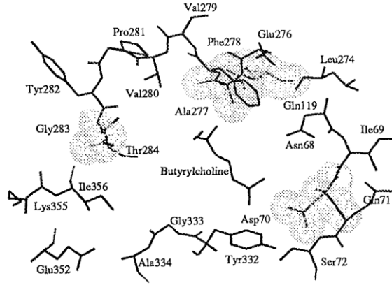
Şekil 2.7. BKE aktif merkez girintisinin amino asit diziliminin gösterimi (41).
