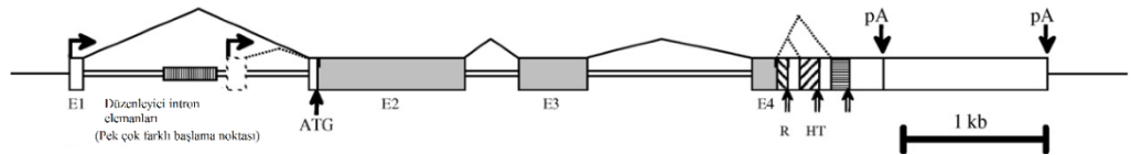
Şekil 2.1. AKE geni şeması (10).
