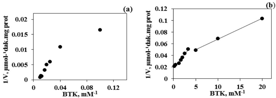
Şekil 4.6. BTK için Lineweaver-Burk grafiğı, (a) 4-100 mM arası derişimleri, (b) Lineer bölgenin BTK derişimlerini kapsamaktadır.
