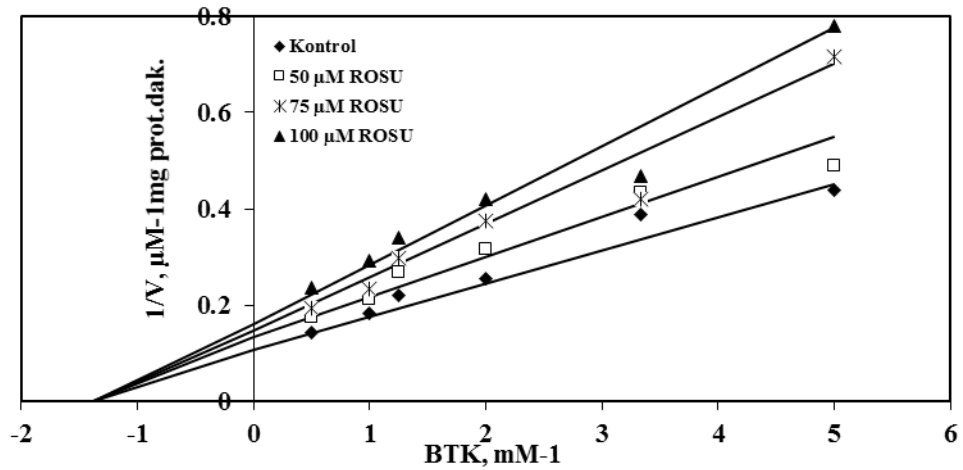
Şekil 4.18. Rosuvastatin-BKE, Lineweaver-Burk grafiğı.
