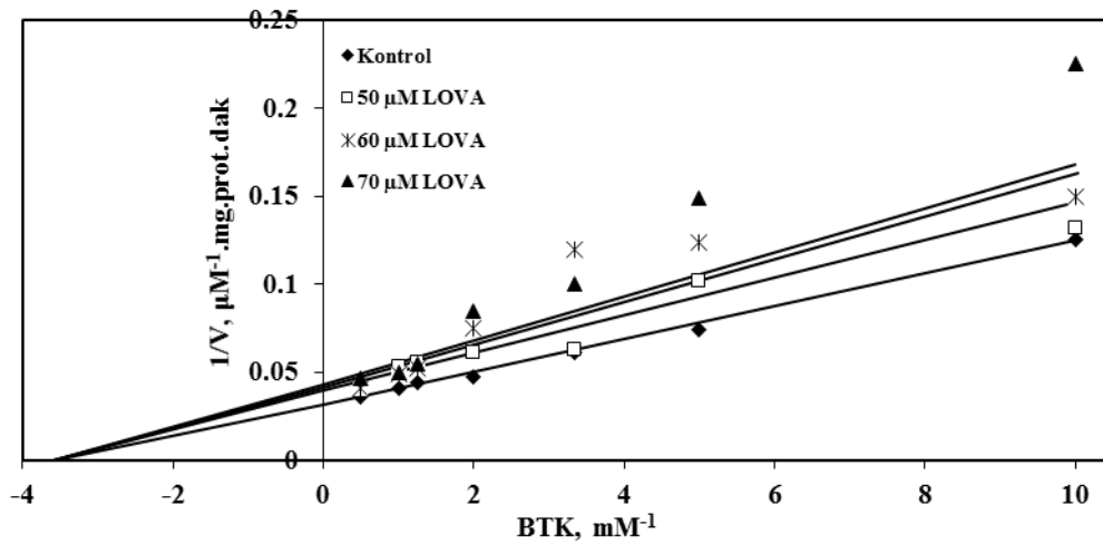
Şekil 4.20. Lovastatin-BKE, Lineweaver-Burk grafiğı.
