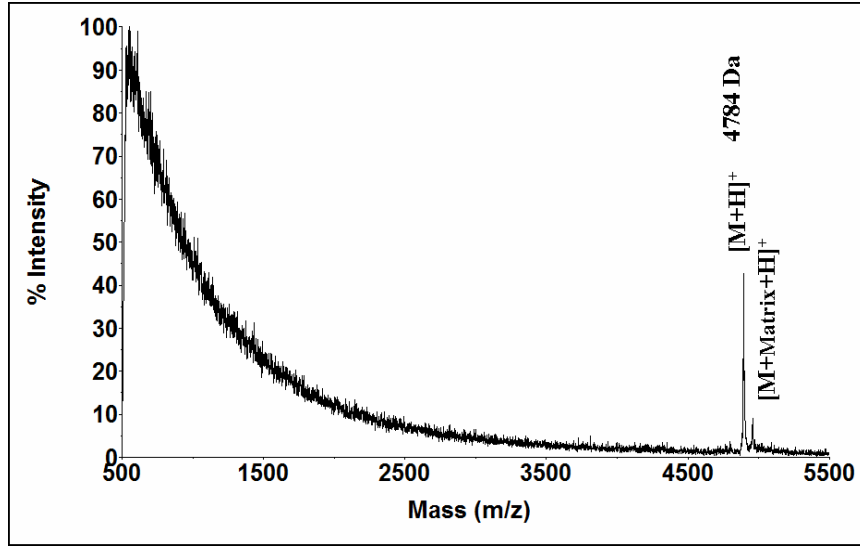
Şekil 3.7. C_{284}H_{156}CuK_4N_{32}O_{24}Ti_2Zn ( 12a ) bileşiğinin 2,5-dihidroksibenzoik asit MALDI matrisi içerisinde kaydedilen pozitif iyon lineer mod MALDI-TOF-MS Spektrumu (Nitrojen Lazeri /337nm/100 Lazer vuruşu)
