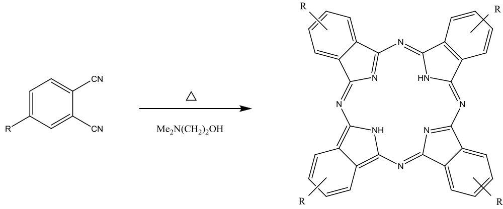
Şekil 1.3. Ftalonitril türevinden metallsız Pc eldesi
