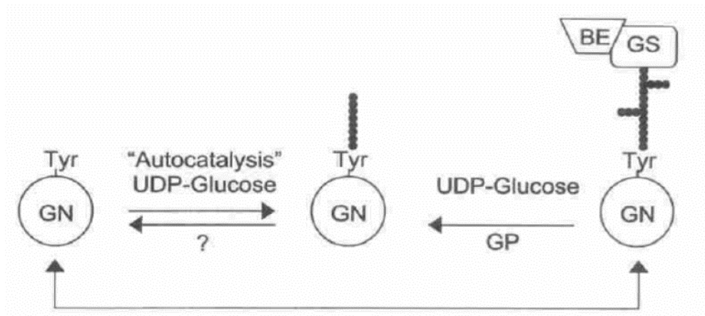
Şekil 2.6. Glikojen sentezi.
