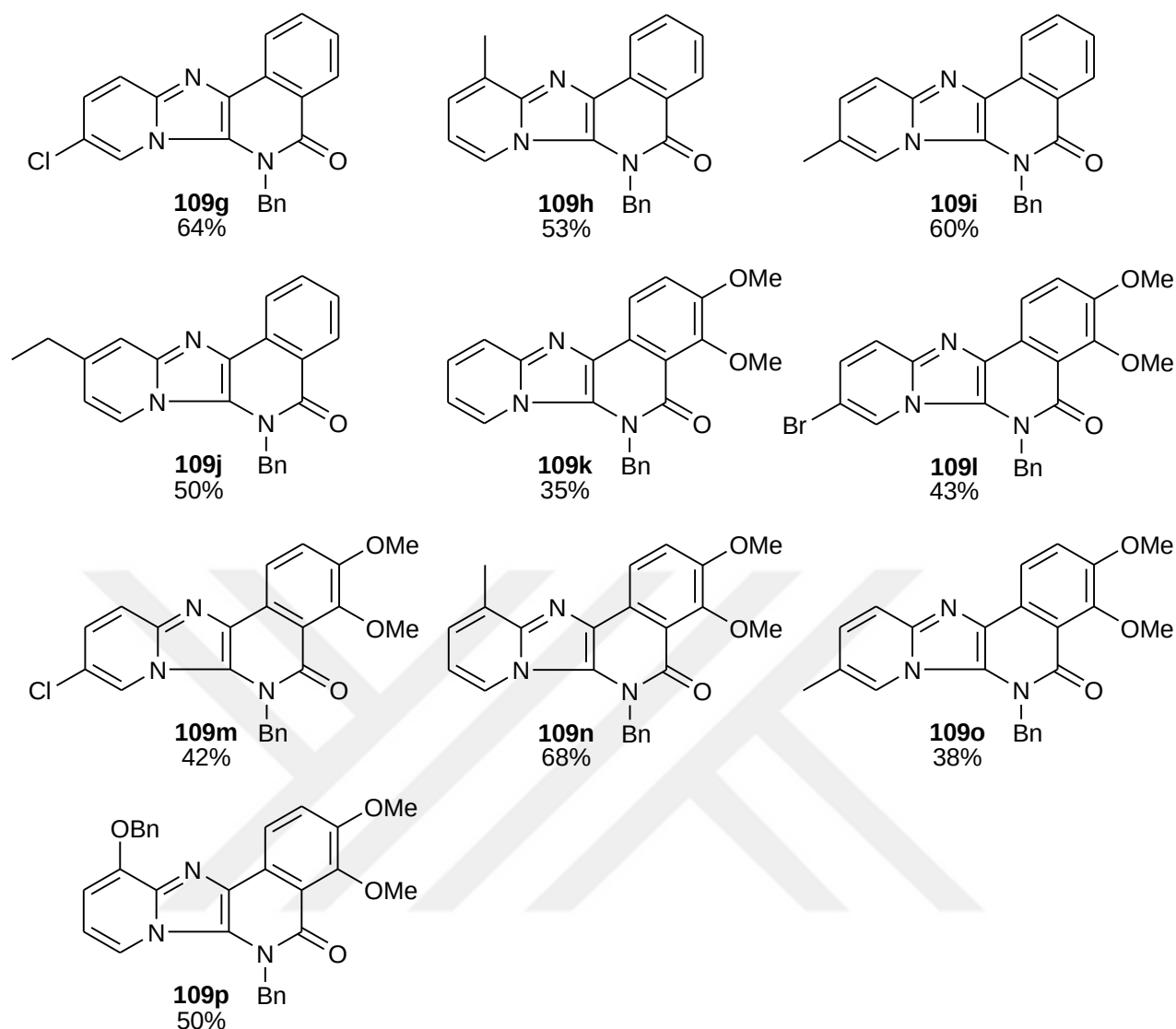
Abbildung 14. Strukturen und Ausbeuten der Pyrido[2',1':2,3]imidazo[4,5-c]isoquinolin-5(6 H )-one 109a-p
