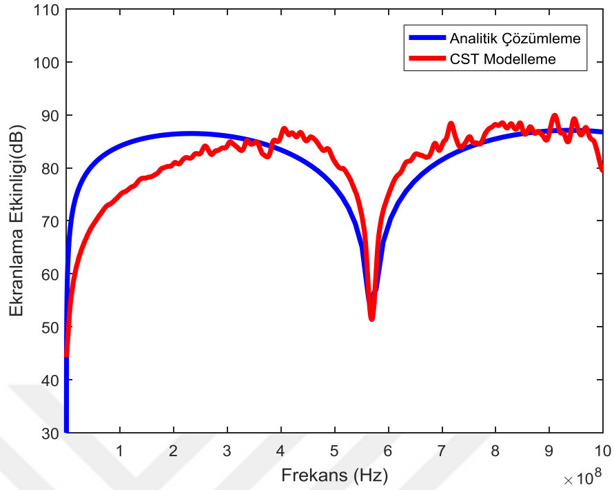
Şekil 4.11. d = 1.5 mm için silindirik kabuğun eksenindeki ekranlama etkinliği ( R = 20 cm, \sigma = 40000 S/m)
