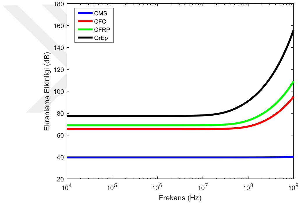
Şekil 5.7. Kompozit malzemelerin ekranlama etkinliği performanslarının karşılaştırması
