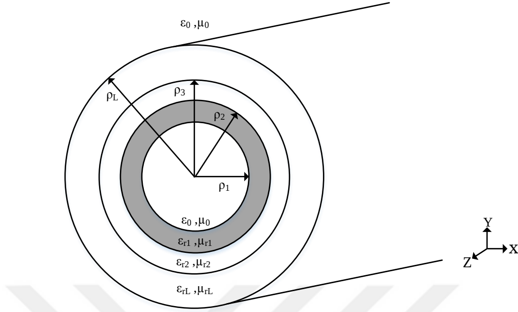
Şekil 3.3. Silindirik kabuk modeli
