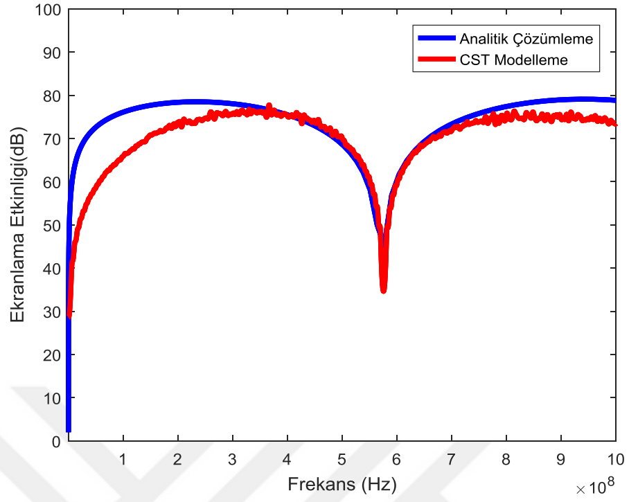
Şekil 4.7. d = 0.6 mm için silindirik kabuğun eksenindeki ekranlama etkinliği ( R = 20 cm, \sigma = 40000 S/m)
