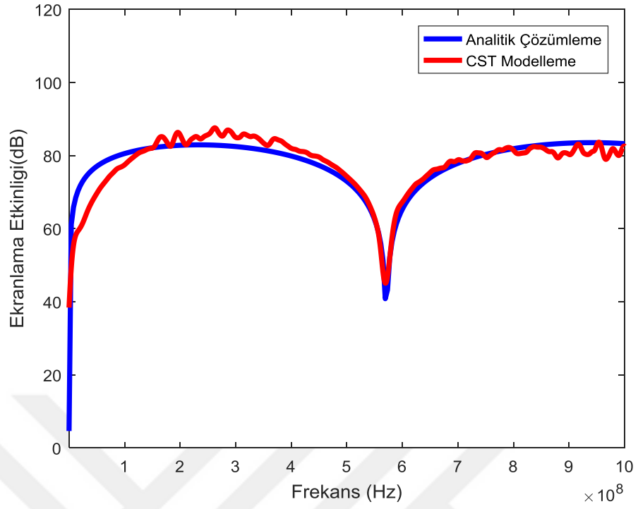
Şekil 4.9. d = 1 mm için silindirik kabuğun eksenindeki ekranlama etkinliği ( R = 20 cm, \sigma=40000 S/m)
