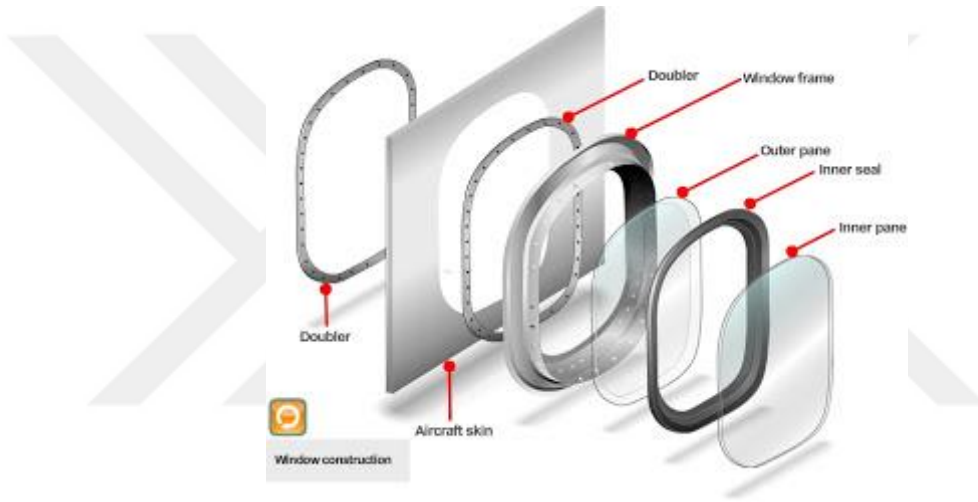
Şekil 5.12. Uçak camının yapısı
