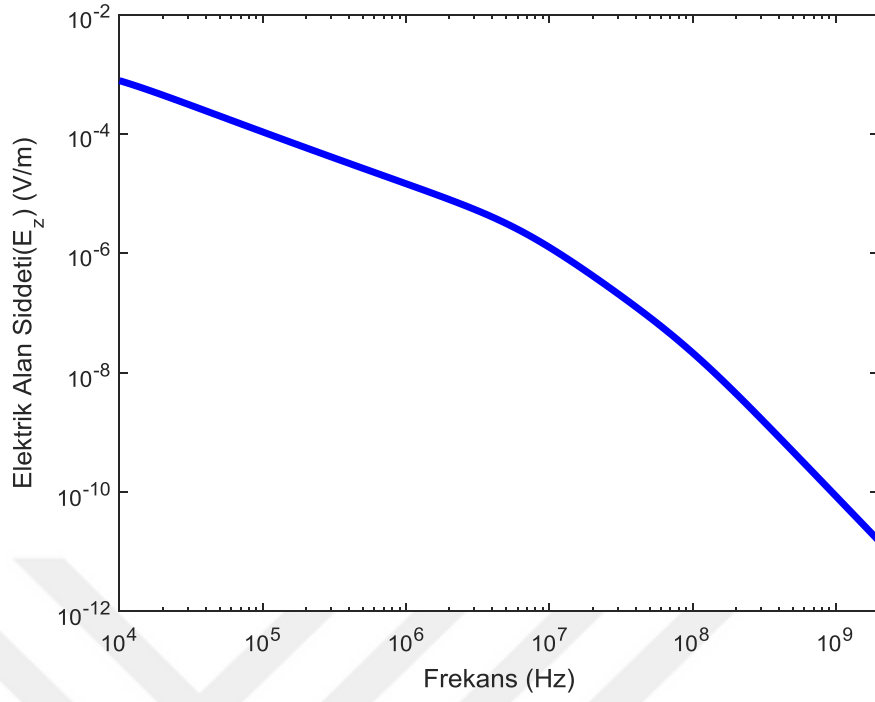
Şekil 5.14. Silindirik kabuğun ekseninde oluşan elektrik alan şiddeti
