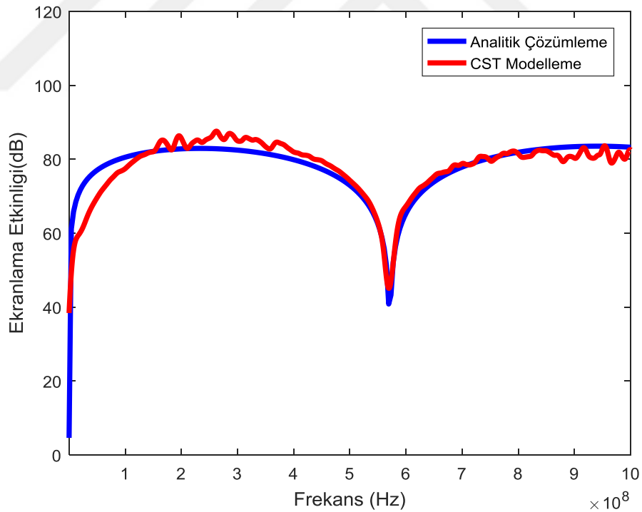
Şekil 4.3. Silindirik kabuğun ekseninde ekranlama etkinliği ( R = 20 cm, d = 1 mm)
