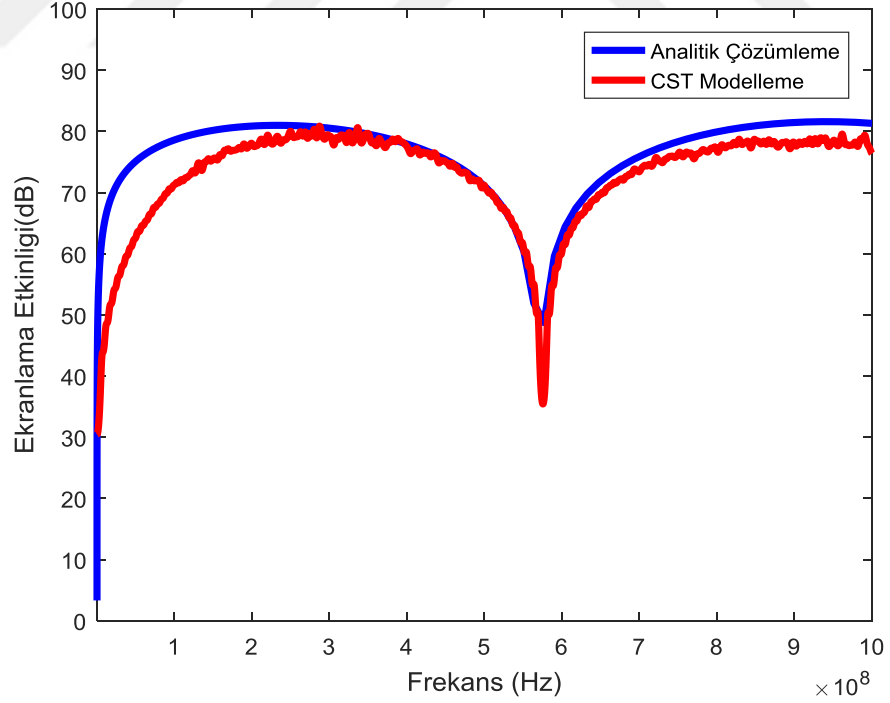
Şekil 4.8. d = 0.8 mm için silindirik kabuğun eksenindeki ekranlama etkinliği ( R = 20 cm, \sigma = 40000 S/m)
