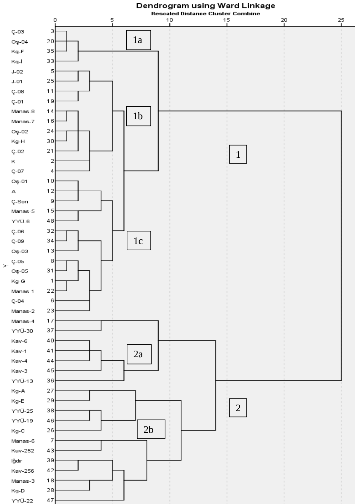
Şekil 4. 26. Kavun genotiplerinde morfolojik ölçüm ve gözlemler kullanılarak Ward metoduna göre yapılan analiz sonucunda ortaya çıkan dendrogram
