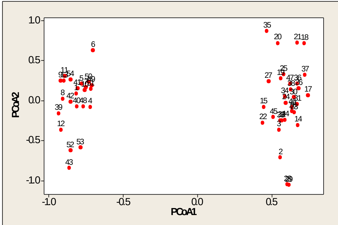
Şekil 4.28. GeneAIEx programı kullanılarak yapılan Principle Coordinate Analizi
