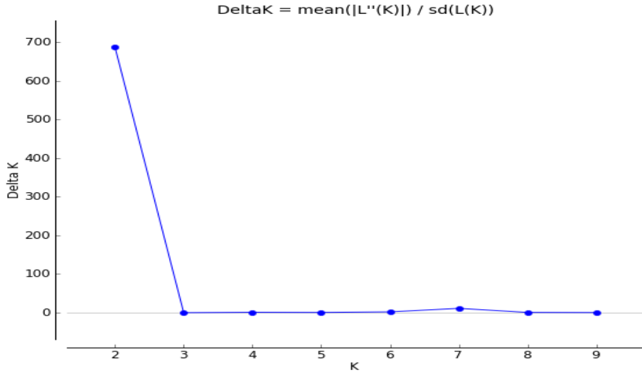
Şekil 4.30. Structure analiz sonucu
