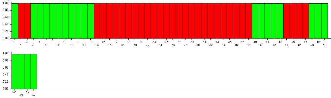
Çizelge 4.5. Structure programı sonucunda iki alt popülasyona ayrılan genotiplerin üyelik katsayıları
