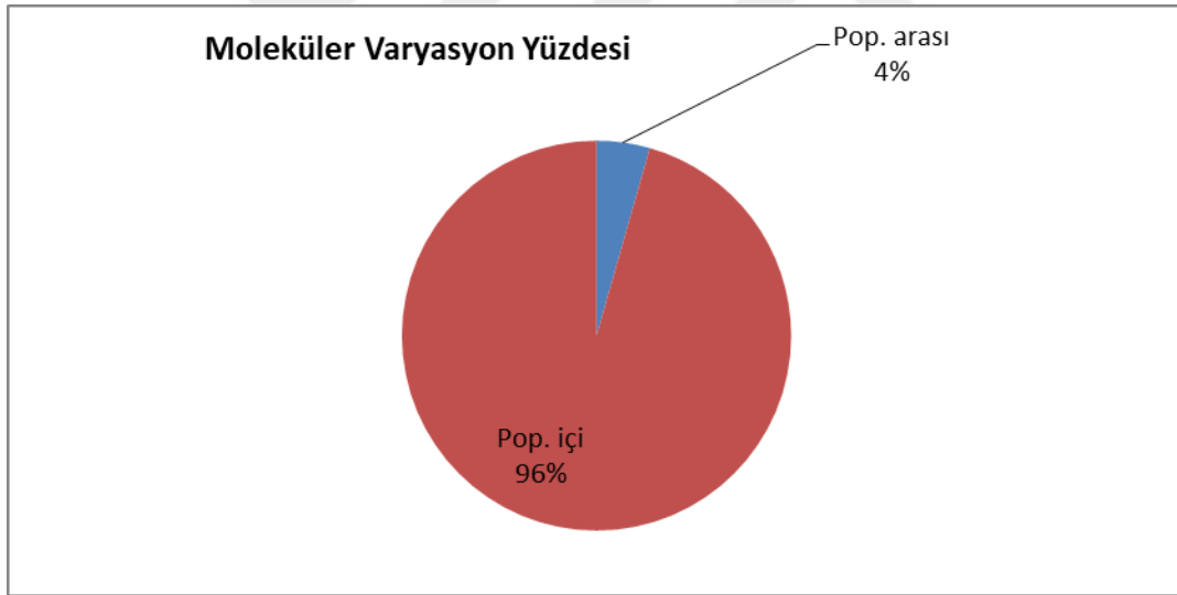
Şekil 4.31. SSR makörleri verilerinden üretilen Moleküler Varyans Analizi grafiği
