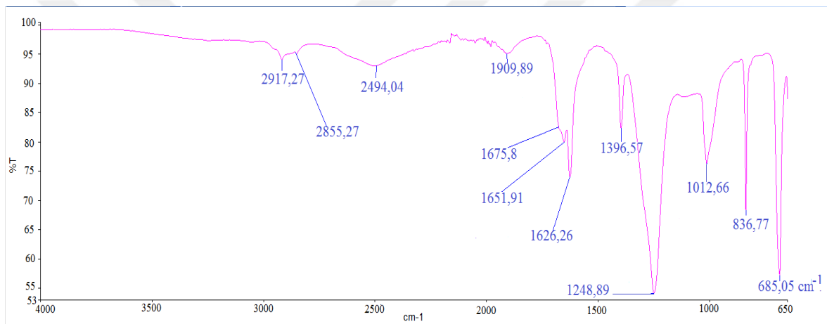
Şekil 4.29. Chlorella -AuNP FTIR analizi
