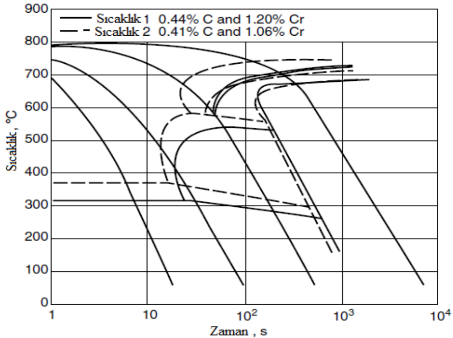
Şekil 2.12 DIN 41Cr4 çeliğin iki sıcaklık arasındaki bileşim farkının, ilgili SSD diyagramındaki dönüşüm eğrilerinin konumu üzerindeki etkisi (Hougardy 1978).
