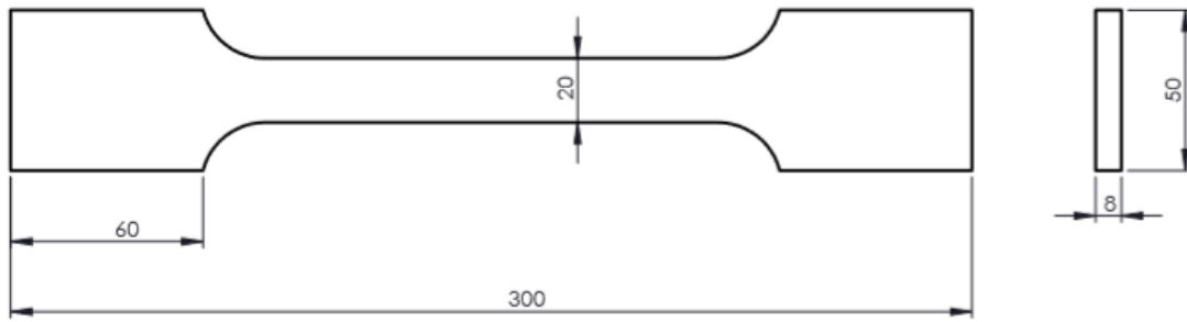
Şekil 3.4 Isıl işlem yapılacak numunelerin teknik resmi (İnt.Kyn.12).
