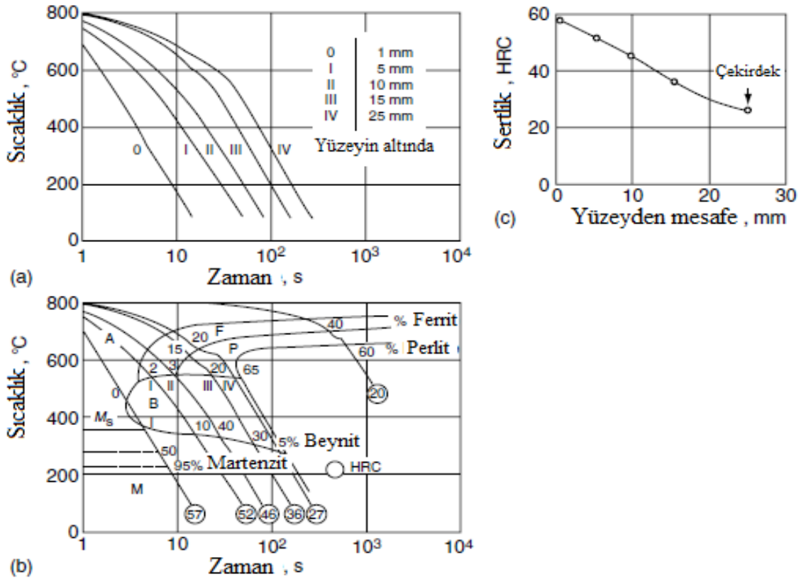
Şekil 2.15 Yuvarlak çubuk kesitinde sertlik dağılımının tahmini. (a) Soğutma eğrileri, belirtildiği gibi yüzeyin altında farklı noktalarda ölçülür. (b) (a)'dan üst üste bindirilmiş soğutma eğrileri ile ilgili çeliğin SSD şeması. (c) Soğutma üzerine çubuk kesitindeki sertlik dağılımı, (b)'den sertlik değerleri okunarak elde edilir (Thelning 1984).
