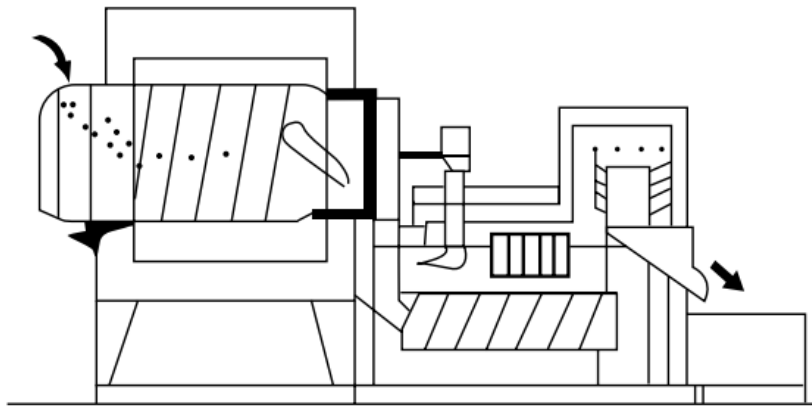
Şekil 2.57 Vidalı konveyör ısıtma fırını şematik gösterimi (Thelning 1984).
