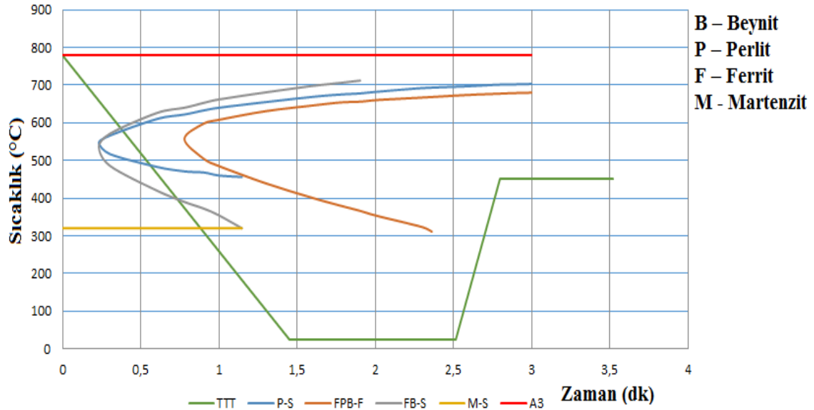
Şekil 4.3 (Devam) 1045 malzeme için ısıtma işlemi bilgileri kullanılarak matematiksel fonksiyonlar sonucu oluşturulan ZSD diyagramı ve farklı soğutma ortamlarında kesilen faz bölgeleri. (a) Suda soğutma esnasında kesilen faz bölgeleri. (b) Tuzlu suda soğutma esnasında kesilen faz bölgeleri. (c) Yağda soğutma esnasında kesilen faz bölgeleri.
