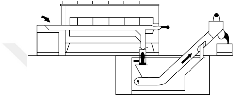
Şekil 2.56 Sallar tabanlı ısıtma fırını şematik gösterimi (Thelning 1984).
