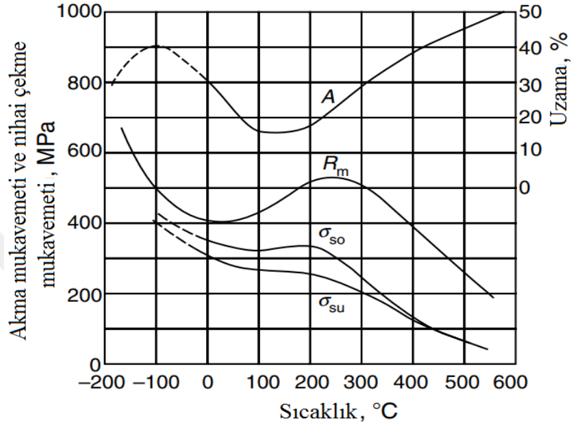
Şekil 2.19 Düşük karbonlu alaşımsız çeliğin artan sıcaklıktaki bazı mekanik özelliklerindeki değişiklik. A, uzama; R m , nihai çekme mukavemeti; σ so , üst akma dayanımı; σ su , daha düşük akma mukavemeti (Eckstein 1987).
