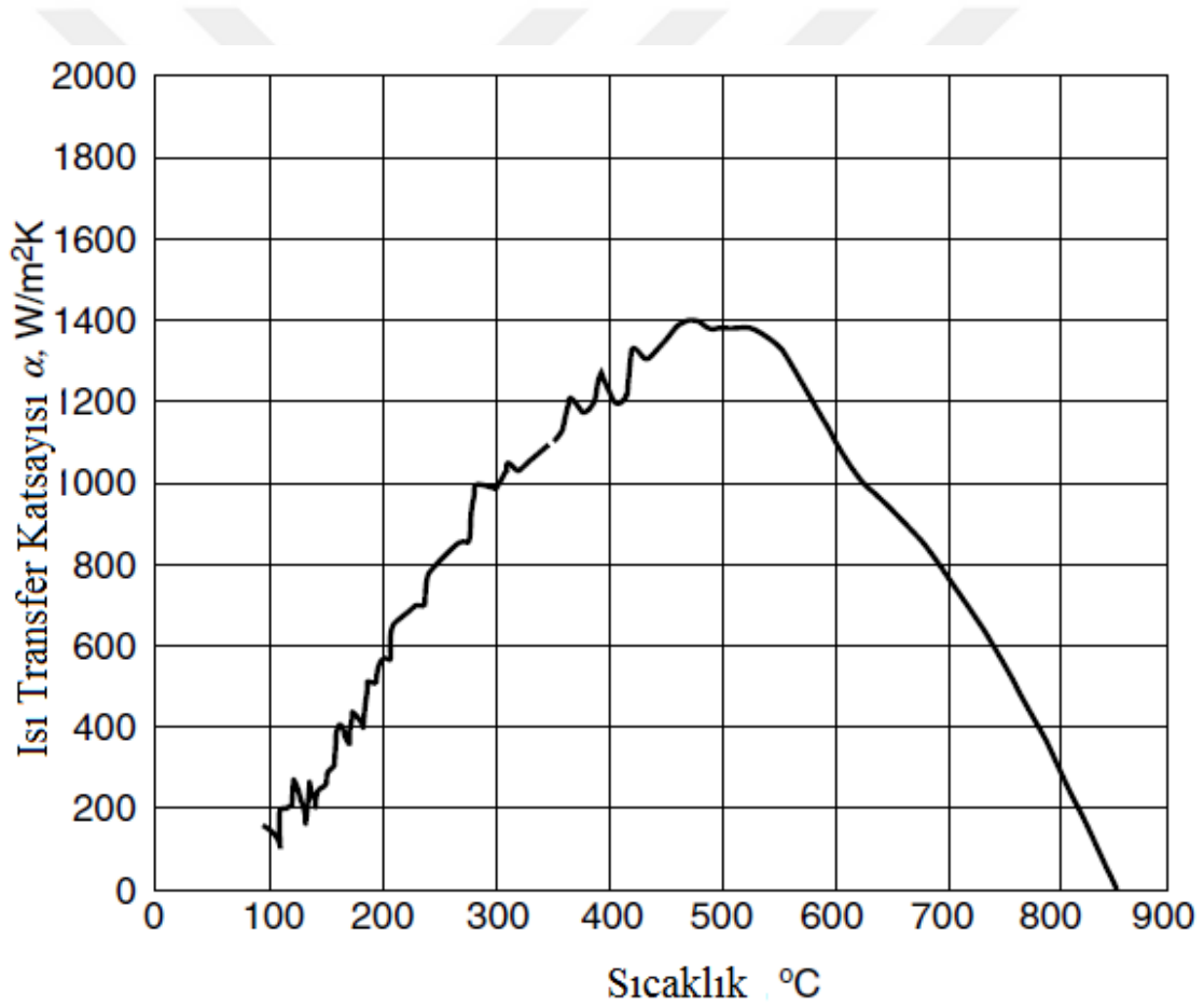
Şekil 2.3 Ölçülen yüzey sıcaklığı - zaman geçişinden hesaplanan 50 mm çapında 200 mm'lik bir paslanmaz çelik silindiri 20 °C'lik yağda söndürürken ısı transfer katsayısı ve yüzey sıcaklığı grafiği (Filetin vd. 1992).
