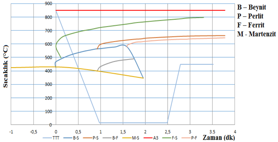
Şekil 4.5 St 52 malzeme için ısı işlemlerinin ZSD diyagramı ve farklı soğutma ortamlarında kesilen faz bölgeleri. (a) Suda soğutma esnasında kesilen faz bölgeleri. (b) Tuzlu suda soğutma esnasında kesilen faz bölgeleri. (c) Yağda soğutma esnasında kesilen faz bölgeleri.
