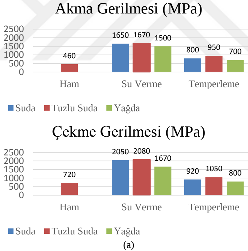
Şekil 4.8 Deneyde kullanılan malzemelerin ham ve ısıt işlemler sonrası akma ve çekme gerilmesi değerleri. (a) 1040 malzeme. (b) 1045 malzeme. (c) 1050 malzeme. (d) St 52 malzeme. (e) St 60 malzeme.
