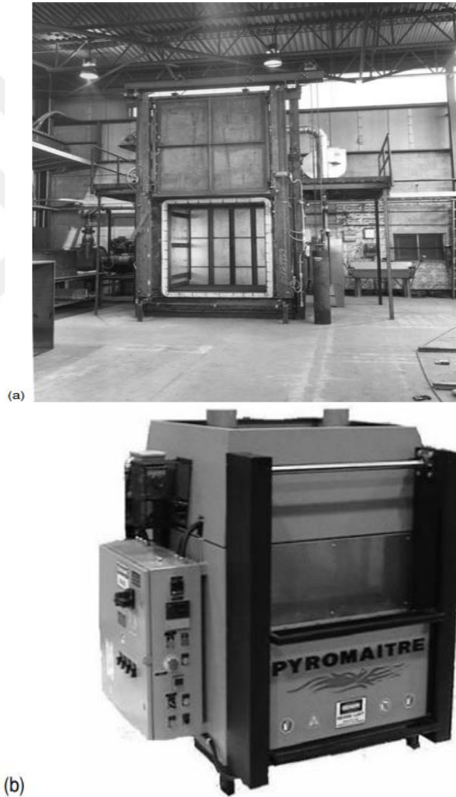
Resim 2.1 (a) Elektrikle ısıtılan kutu fırını. (b) Küçük parçaları ısıtmak için kullanılan küçük 'yüksek hızlı' laboratuvar fırını ve aynı zamanda üretim ölçekli sürekli gerilim giderici fırınlar için gerilim giderici ve temperleme süreçleri geliştirmek için ısıtma ve soğutma döngülerini modellemek için kontrol edilebilir (İnt.Kyn.1).
