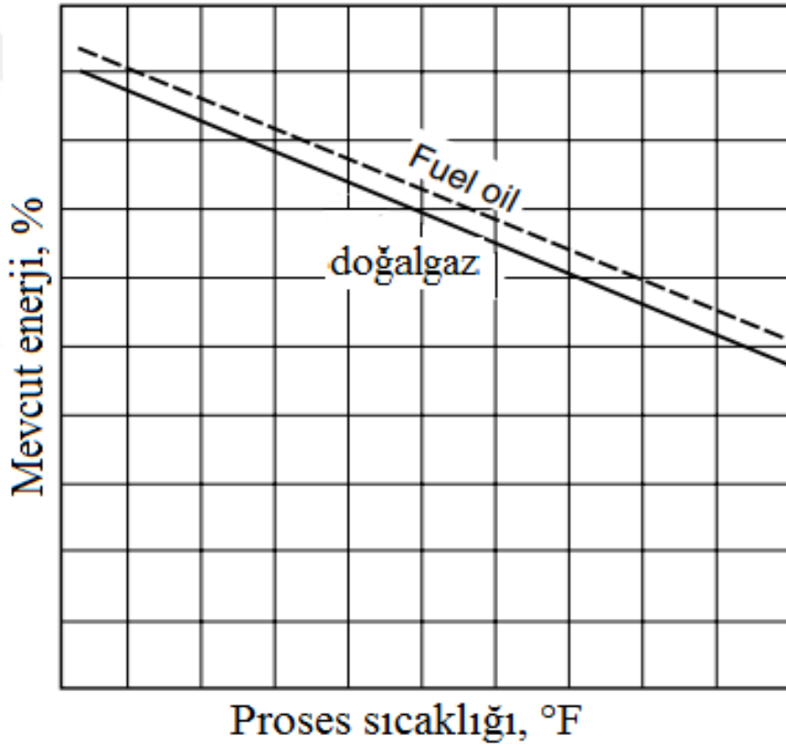
Şekil 2.59 Mevcut ısı enerjisinin yakıt yağı ve doğal gaz için egzoz sıcaklığına bağımlılığı (Piotrak 1981, 1982).
