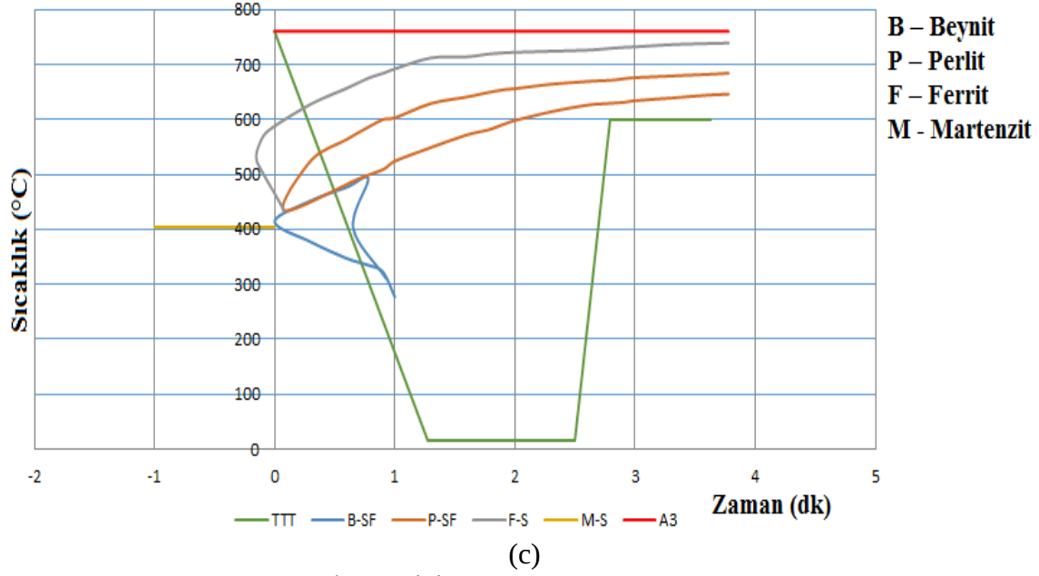
Şekil 4.2 (Devam) 1040 malzeme için ısıtma işlemi prosesi kullanılarak matematiksel fonksiyonlar sonucu oluşturulan ZSD diyagramı ve farklı soğutma ortamlarında kesilen faz bölgeleri. (a) Suda soğutma esnasında kesilen faz bölgeleri. (b) Tuzlu suda soğutma esnasında kesilen faz bölgeleri. (c) Yağda soğutma esnasında kesilen faz bölgeleri.
