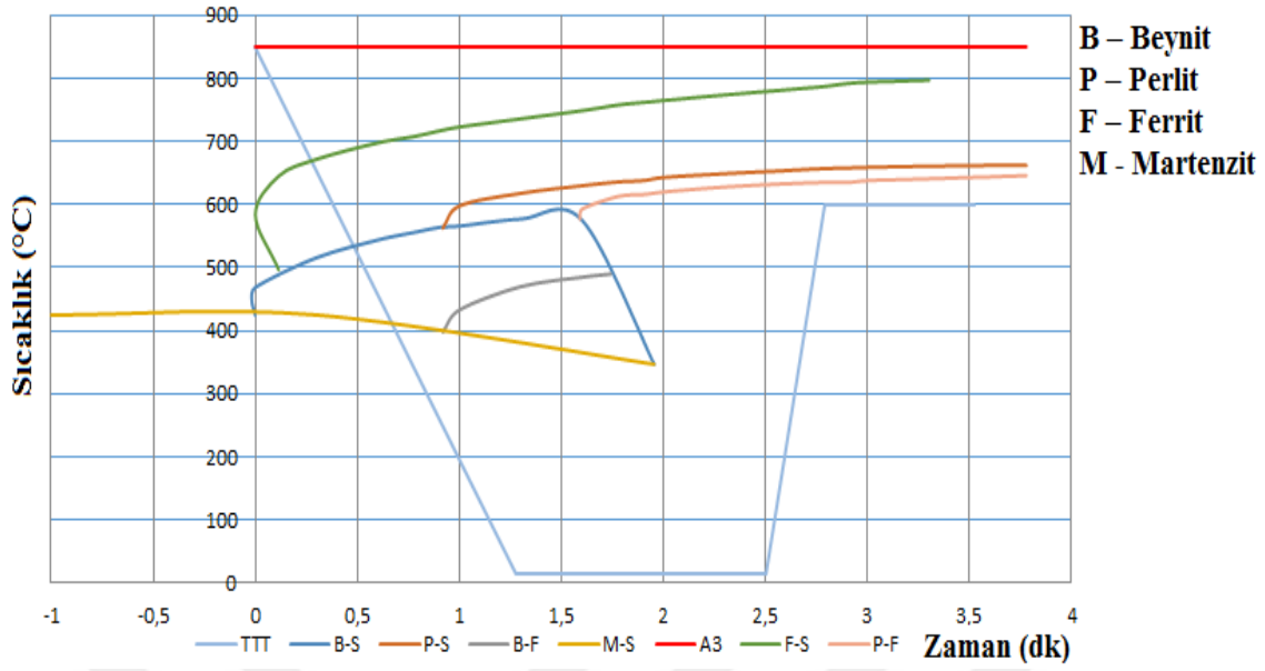
Şekil 4.6 (Devam) St 60 malzeme için ısıtma işlemi sonrası farklı soğutma ortamlarında kesilen faz bölgeleri. (a) Suda soğutma esnasında kesilen faz bölgeleri. (b) Tuzlu suda soğutma esnasında kesilen faz bölgeleri. (c) Yağda soğutma esnasında kesilen faz bölgeleri.
