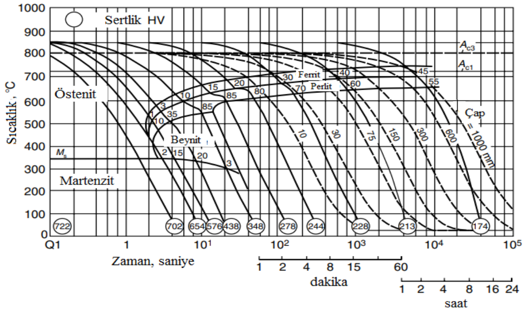
Şekil 2.32 Havada soğutulmuş farklı çaplarda ki yuvarlak çubukların çekirdeğinde ölçülen üst üste bindirilmiş soğutma eğrileri ile alaşımsız çelik DIN Ck45 (östenit sıcaklığı 850 °C) SSD diyagramı (Spur ve Stöferle 1987).
