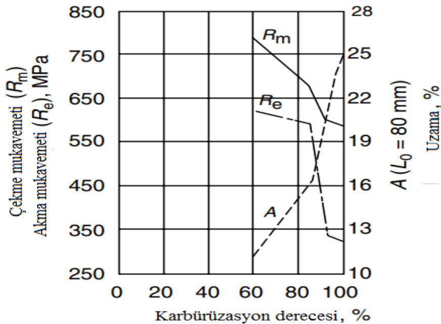
řekil 2.46 Nihai ekme mukavemeti, akma mukavemeti ve alařımsız DIN C75 ötektoid eliėin artan karbürizasyonu ile uzama deėiřimi (Eckstein 1987).
