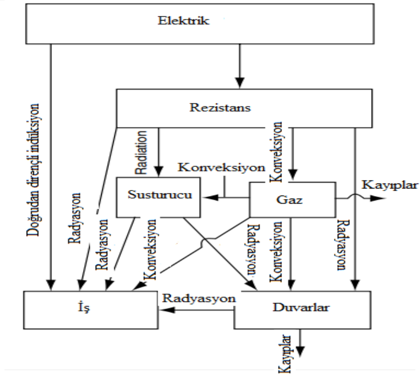
Şekil 2.75 Çeşitli fırın bileşenleri için ısı transfer süreçlerinin özeti (Nicholson vd. 1966). Isıtılmış parça içindeki ısı transferi diferansiyel denklemden modellenenir.
