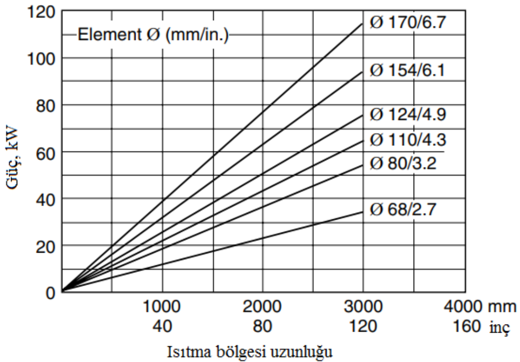
Şekil 2.60 900 °C fırın sıcaklığında olası yükleme (Thelning 1984).
