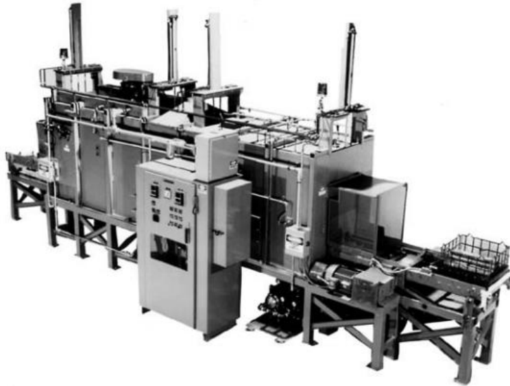
Resim 2.5 Srekli fırın rnekleri (İnt.Kyn.3 ve 4).
