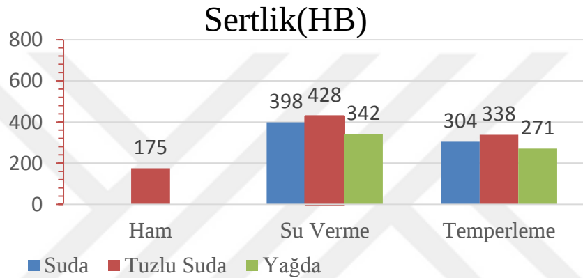
Şekil 4.7 (Devam) Deneyde kullanılan malzemelerin ham ve ısıl işlemler sonrası sertlik değerleri. (a) 1040 malzeme. (b) 1045 malzeme. (c) 1050 malzeme. (d) St 52 malzeme. (e) St 60 malzeme.
