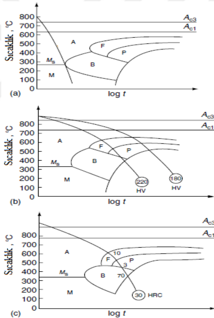
Şekil 2.14 Sadece SSD diyagramlarının kullanılabileceği sürekli soğutma ısıl işlem süreçleri. (a) Tam martenzitik yapı elde etmek için doğrudan söndürme; (b) gerekli sertlikte bir ferrit– perlit yapısı elde etmek için yavaş soğutma; (c) karışık bir yapının elde edildiği sürekli soğutma rejimi (Thelning 1984).
