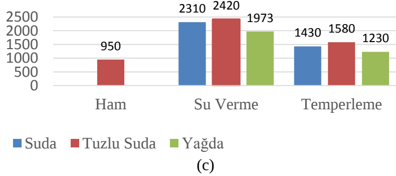
Şekil 4.8 (Devam) Deneyde kullanılan malzemelerin ham ve ısıt işlemler sonrası akma ve çekme gerilmesi değerleri. (a) 1040 malzeme. (b) 1045 malzeme. (c) 1050 malzeme. (d) St 52 malzeme. (e) St 60 malzeme.
