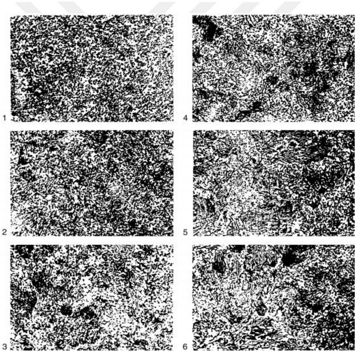
Şekil 2.41 Alman şirketi Edelstahlwerke Buderus A.G.-Wetzlar'ın DIN 100Cr6 çeliğinin yumuşak tavlama sonrasında küreselleşme derecesinin değerlendirilmesi için iç standardı. Büyütme 500x (Spur ve Stöferle 1987).
