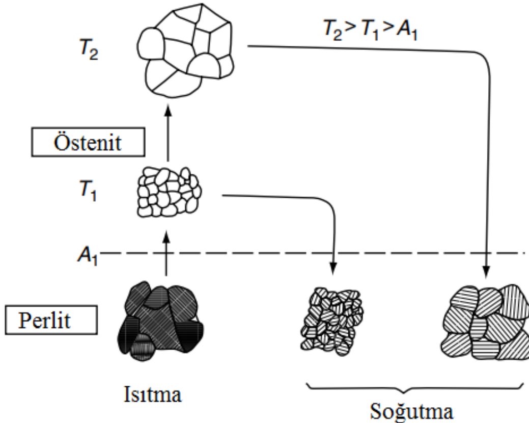
Şekil 2.29 Ötektoid bir çelik yapısının normalleştirme işleminden sonra tane büyüklüğü üzerinde östenitleştirici sıcaklığın etkisinin şematik sunumu (Eckstein 1987).
