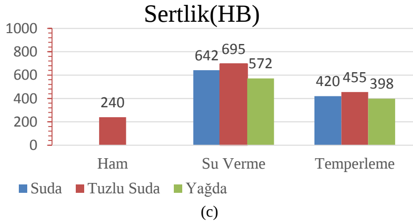
Şekil 4.7 Deneyde kullanılan malzemelerin ham ve ısıt işlemler sonrası sertlik değerleri. (a) 1040 malzeme. (b) 1045 malzeme. (c) 1050 malzeme. (d) St 52 malzeme. (e) St 60 malzeme.
