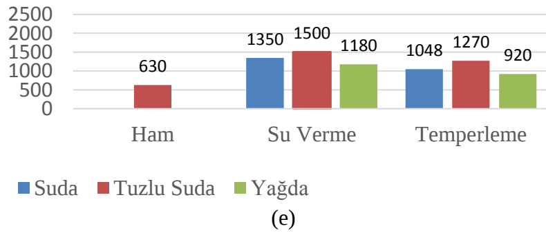
Şekil 4.8 (Devam) Deneyde kullanılan malzemelerin ham ve ısıt işlemler sonrası akma ve çekme gerilmesi değerleri. (a) 1040 malzeme. (b) 1045 malzeme. (c) 1050 malzeme. (d) St 52 malzeme. (e) St 60 malzeme.
