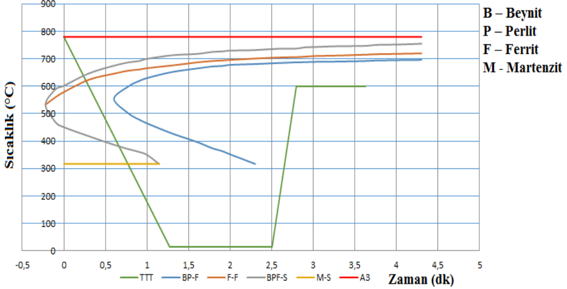
Şekil 4.4 (Devam) 1050 malzeme için ısıtma işlemi bilgileri kullanılarak matematiksel fonksiyonlar sonucu oluşturulan ZSD diyagramı ve farklı soğutma ortamlarında kesilen faz bölgeleri. (a) Suda soğutma esnasında kesilen faz bölgeleri. (b) Tuzlu suda soğutma esnasında kesilen faz bölgeleri. (c) Yağda soğutma esnasında kesilen faz bölgeleri.
