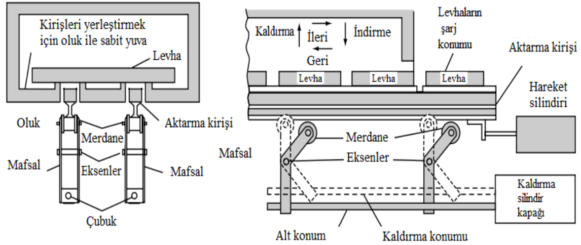
Şekil 2.54 Yürüyen tabanlı fırın mekanizması (Thelning 1984).
