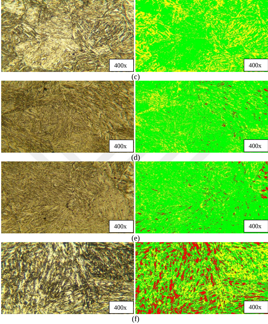
Resim 4.5 (Devam) St 60 çelik mikroyapı ve faz analizi fotoğrafları. (a) Ham hali. (b) Suda soğutma sonrası. (c) Suda soğutma ve temperleme sonrası. (d) Tuzlu suda soğutma sonrası. (e) Tuzlu suda soğutma ve temperleme sonrası. (f) Yağda soğutma sonrası. (g) Yağda soğutma ve temperleme sonrası. Büyütme 400x.
