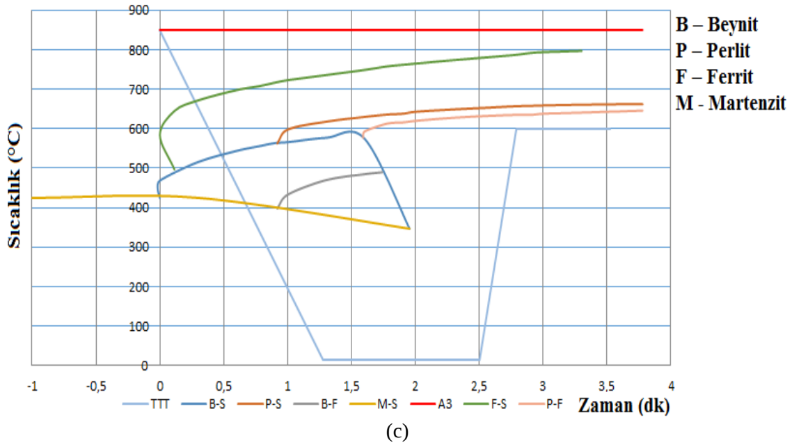
Şekil 4.5 (Devam) St 52 malzeme için ısııl işlem proses bilgileri kullanılarak matematiksel fonksiyonlar sonucu oluşturulan ZSD diyagramı ve farklı soğutma ortamlarında kesilen faz bölgeleri. (a) Suda soğutma esnasında kesilen faz bölgeleri. (b) Tuzlu suda soğutma esnasında kesilen faz bölgeleri. (c) Yağda soğutma esnasında kesilen faz bölgeleri.
