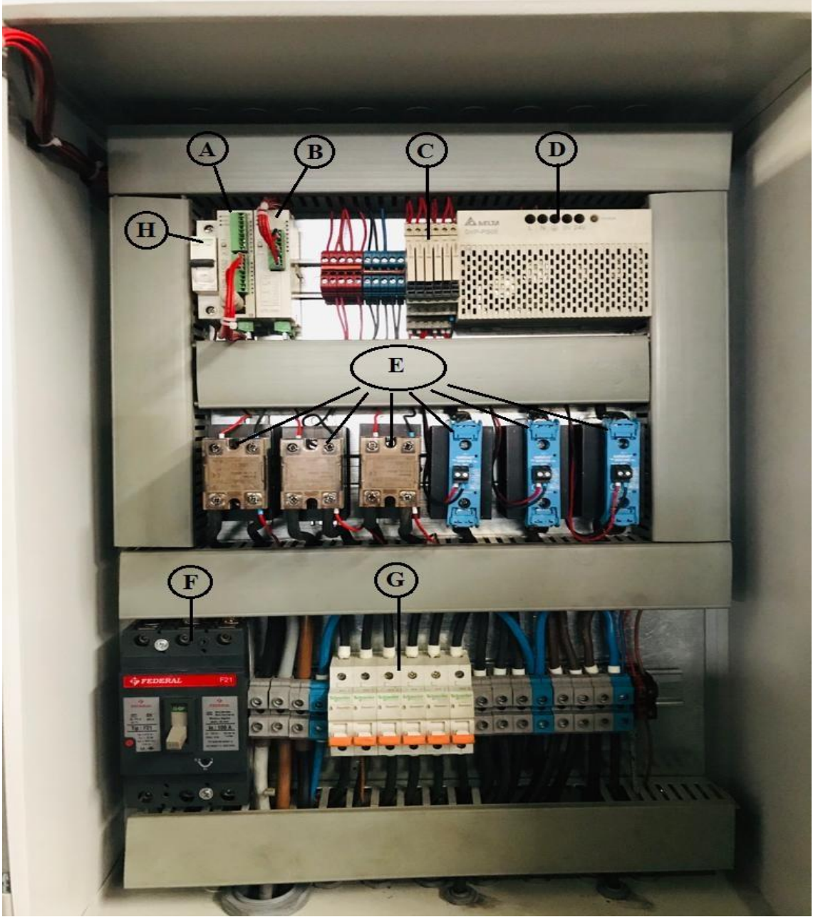
Resim 4.8 Isıl işlem fırını güç paneli iç donanım resmi.
