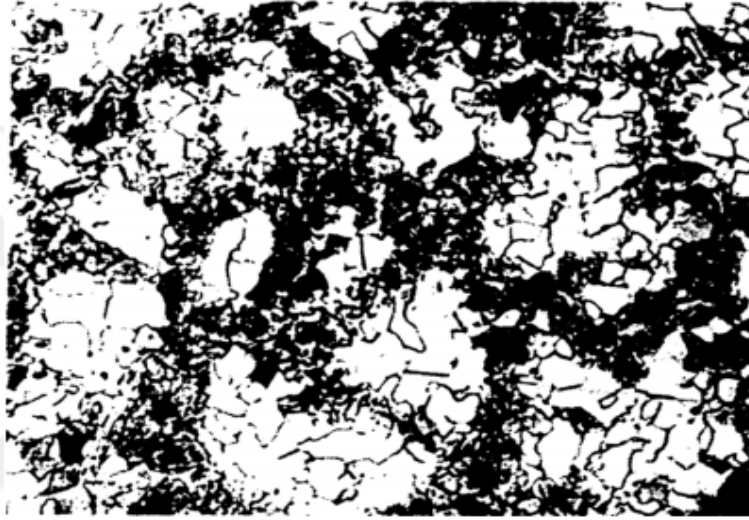
Şekil 2.30 Alaşımsız DIN C35 çeliğinin normalleştirilmesi sırasında hatalı sıcaklık kontrolünün bir sonucu olarak ferrit ve perlitin homojen olmayan dağılımı. Büyütme 100x (Spur ve Stöferle 1987).
