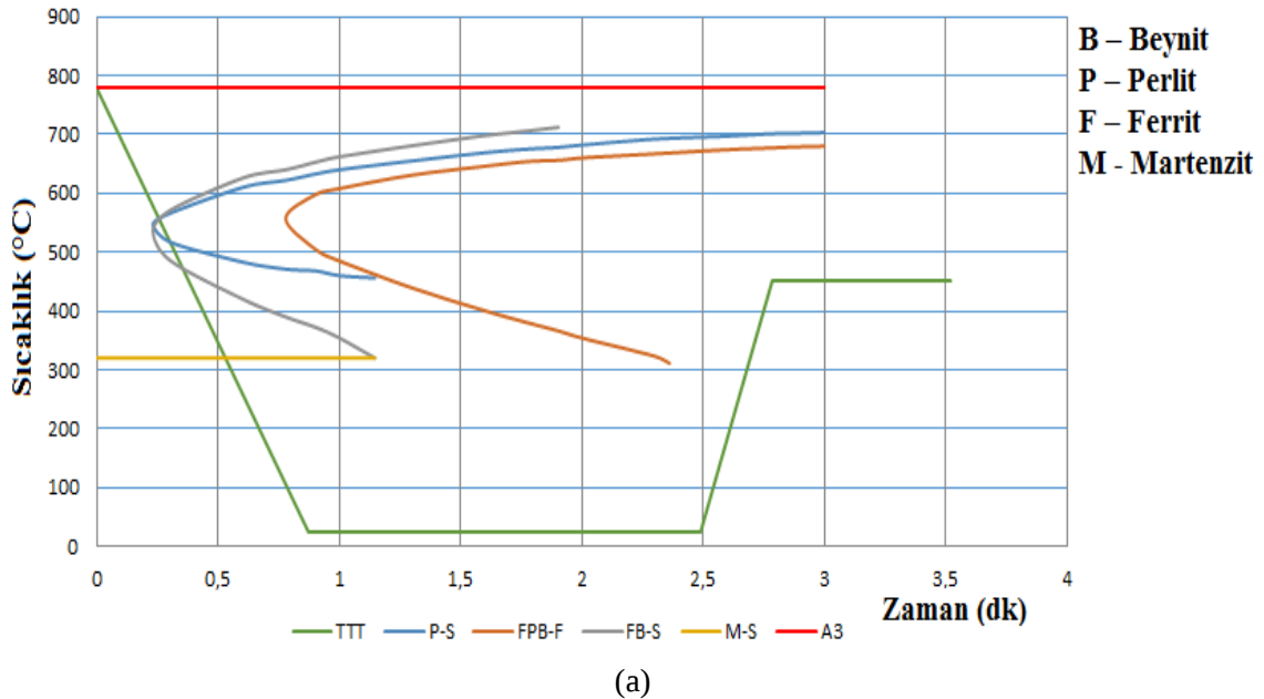
Şekil 4.3 1045 malzeme için ısı işlemleri bilgileri kullanılarak matematiksel fonksiyonlar sonucu oluşturulan ZSD diyagramı ve farklı soğutma ortamlarında kesilen faz bölgeleri. (a) Suda soğutma esnasında kesilen faz bölgeleri. (b) Tuzlu suda soğutma esnasında kesilen faz bölgeleri. (c) Yağda soğutma esnasında kesilen faz bölgeleri.
