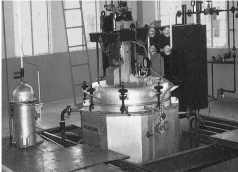
Resim 2.3 Çukur tipi ısıtma işlem fırını (Thelning 1984).
