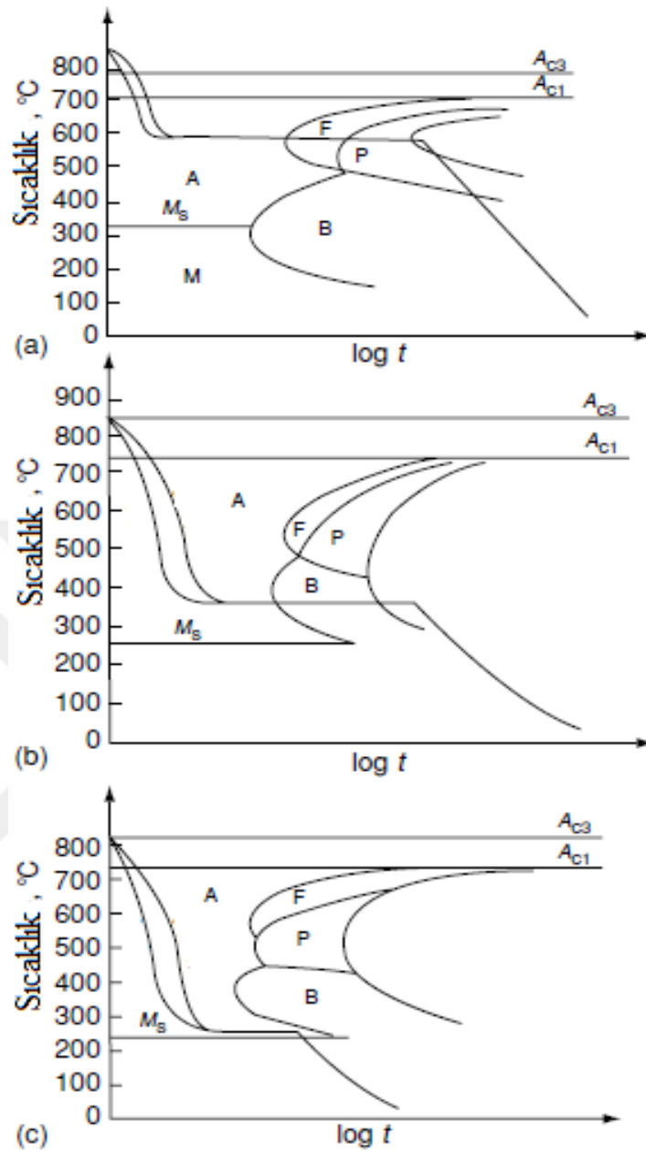
Şekil 2.13 Sadece IT diyagramlarının kullanılabildiği izotermal ısıtım süreçleri. (a) İzotermal tavlama; (b) östempereleme; (c) martemperleme (Thelning 1984).
