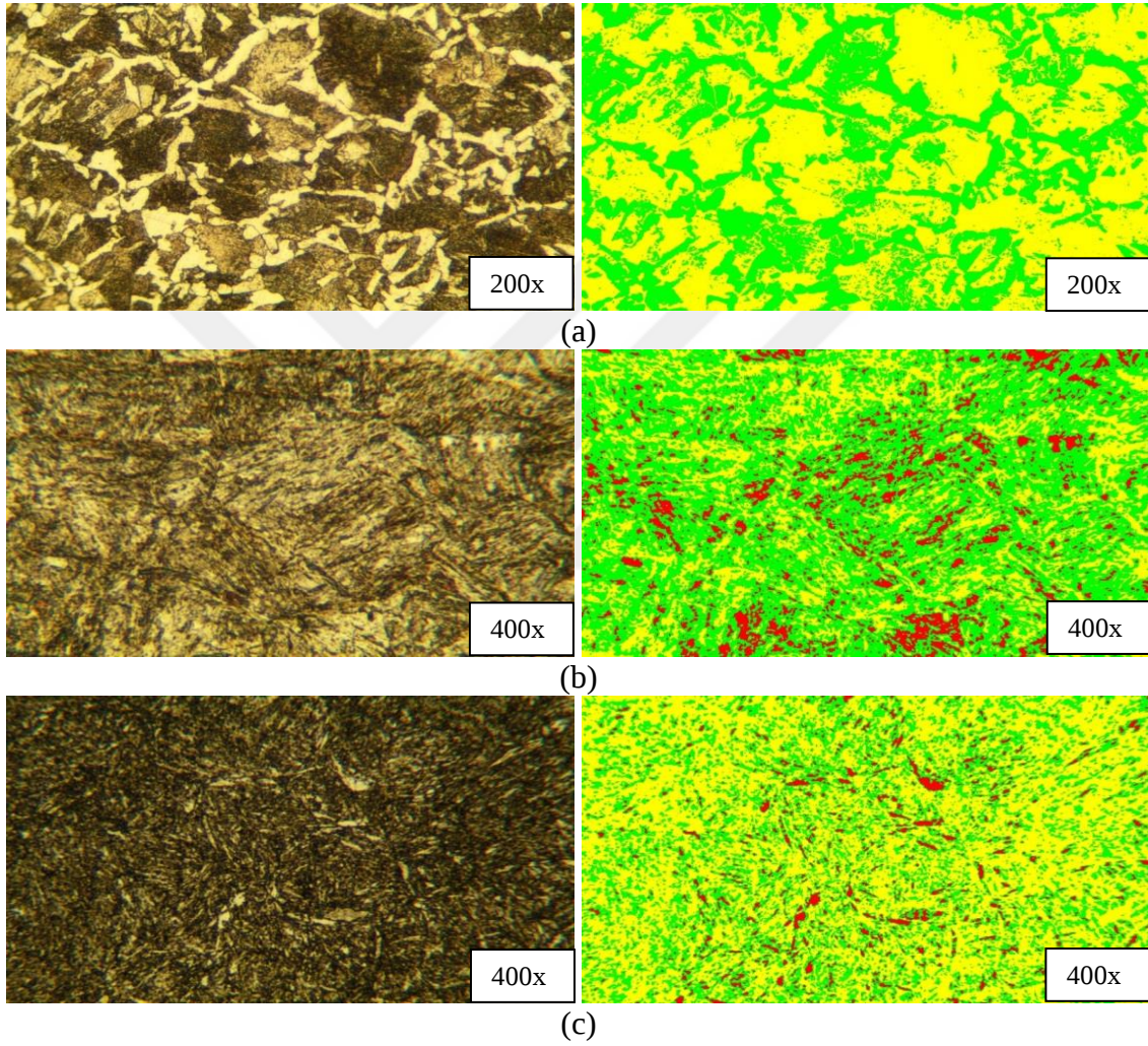
Resim 4.3 1050 elik mikroyapı ve faz analizi fotoğrafları. (a) Ham hali. (b) Suda soğutma sonrası. (c) Suda soğutma ve temperleme sonrası. (d) Tuzlu suda soğutma sonrası. (e) Tuzlu suda soğutma ve temperleme sonrası. (f) Yağda soğutma sonrası. (g) Yağda soğutma ve temperleme sonrası. Büyütme 200x ve 400x.
