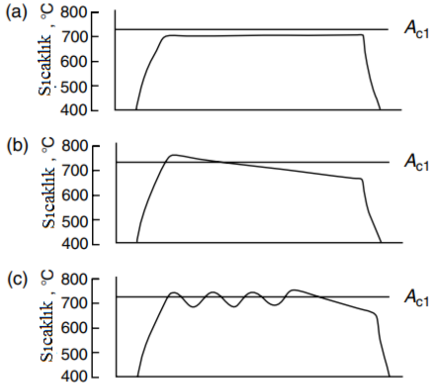
Şekil 2.44 Yumuşak tavlama sıcaklık-zaman rejimleri. (a) Alaşımsız çelikler ve bey nitik veya martenitik başlangıç yapısına sahip alaşımlı çelikler için A_{C1} 'in altında 20 °C'de tavlama; (b) A_{C1} 'in üstünde 10 °C'de tavlama (başlangıç) ve alaşımlı çelikler için A_{C1} 'in altında 30 °C'ye düşürme; (c) hiper ötektoid çelikler için A_{C1} yaklaşık \pm 5 °C tavlama (Spur ve Stöferle 1987).
