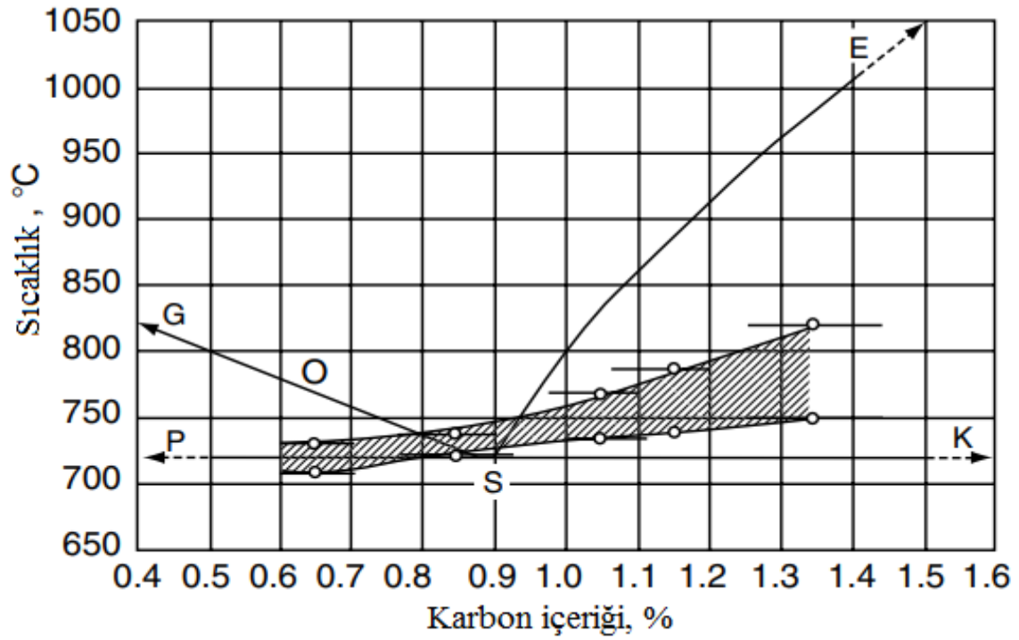
Şekil 2.43 Karbon içeriği %0,6–1,35 C olan alaşımsız çeliklerin yumuşak tavlama için 4 sıcaklık aralığı (Spur ve Stöferle 1987).
