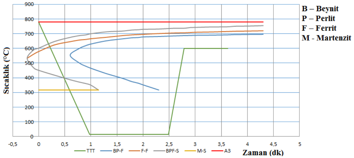
Şekil 4.4 1050 malzeme için ısı işlem prosesi bilgileri kullanılarak matematiksel fonksiyonlar sonucu oluşturulan ZSD diyagramı ve farklı soğutma ortamlarında kesilen faz bölgeleri. (a) Suda soğutma esnasında kesilen faz bölgeleri. (b) Tuzlu suda soğutma esnasında kesilen faz bölgeleri. (c) Yağda soğutma esnasında kesilen faz bölgeleri.
