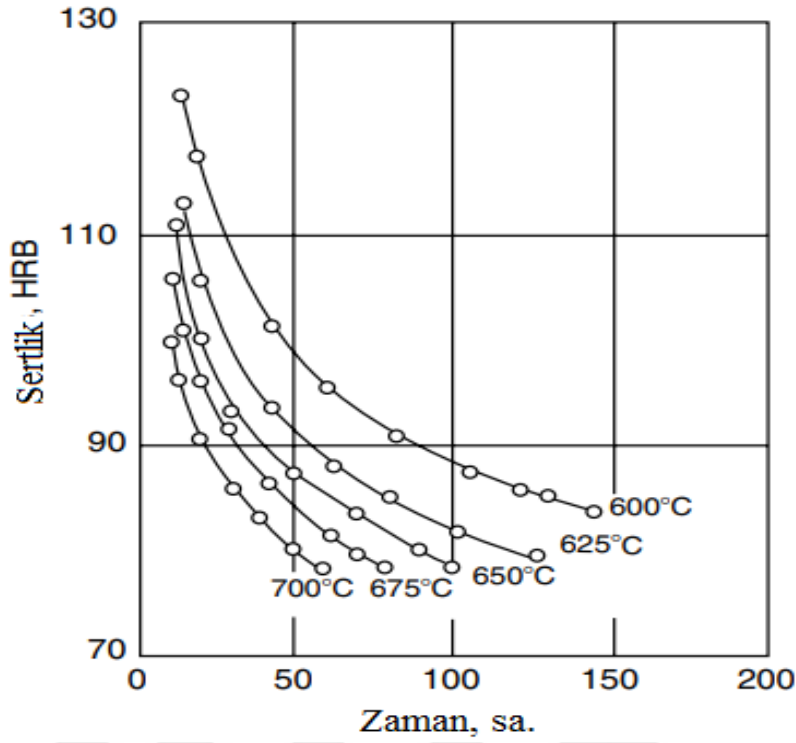
Şekil 2.47 Karbürüzasyon süresine ve sıcaklığına bağlı olarak yumuşak tavlamadan sonra %0,89 C içeren alaşımsız bir çeliğin sertliği (Eckstein 1987).
