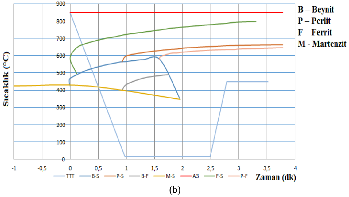
Şekil 4.6 St 60 malzeme için ısıtma işlemi prosesi bilgileri kullanılarak matematiksel fonksiyonlar sonucu oluşturulan ZSD diyagramı ve farklı soğutma ortamlarında kesilen faz bölgeleri. (a) Suda soğutma esnasında kesilen faz bölgeleri. (b) Tuzlu suda soğutma esnasında kesilen faz bölgeleri. (c) Yağda soğutma esnasında kesilen faz bölgeleri.
