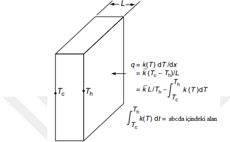
Şekil 2.72 Düz bir duvar için ısı akısının hesaplanması (Thelning 1984).
