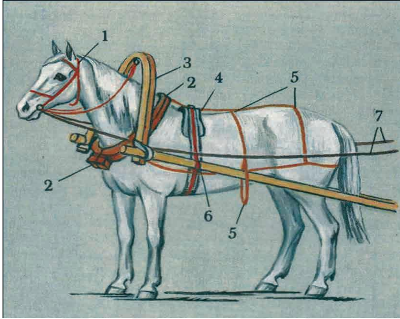
Resim 3.101. Qamıt ve araba koşum takımları: 1. jügen, 2. qamıt, 3. doğa, 4. erşik, 5. şiliya, 6. belköterme ve bawırdaq, 7. delbe (Kaynak: QEKUADJ 3, 428)
