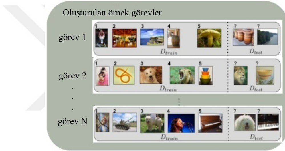
Şekil 1.3: Veri kümesinden farklı görev setlerinin oluşturulması.
