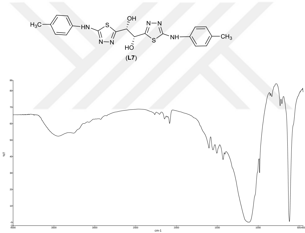
Şekil 4.19. (L7) molekülünün FT-IR spektrumu
