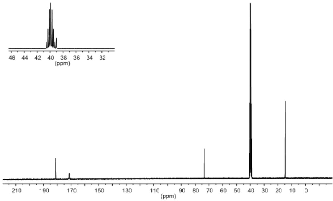
Şekil 4.15. (L5) molekülünün ^{13}\text{C} -NMR spektrumu
