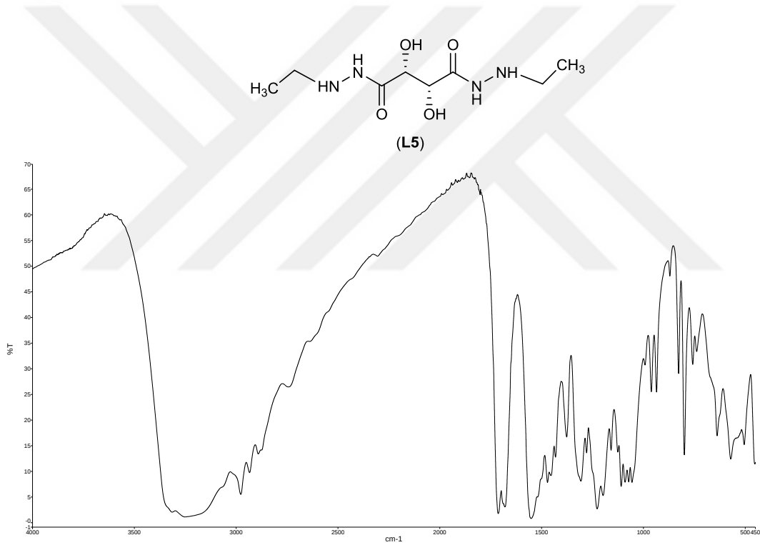
Şekil 4.13. (L5) molekülü' nün FT-IR spektrumu
