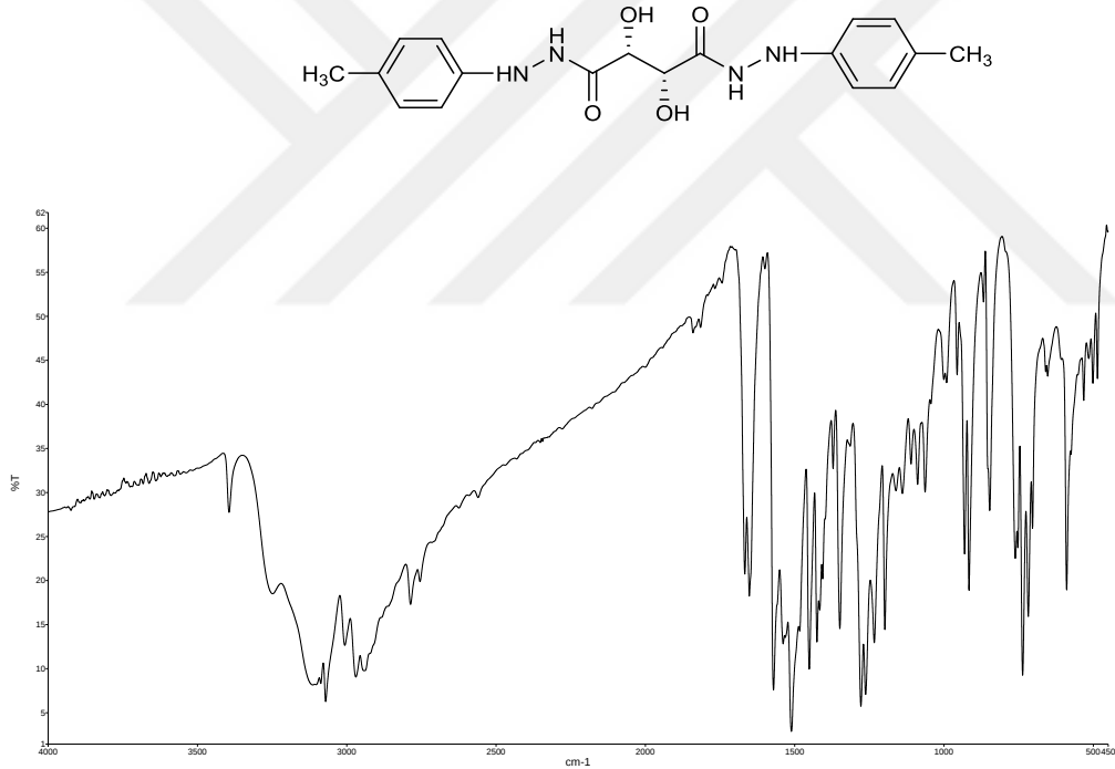
Şekil 4.4. (L2) molekülünün FT-IR spektrumu
