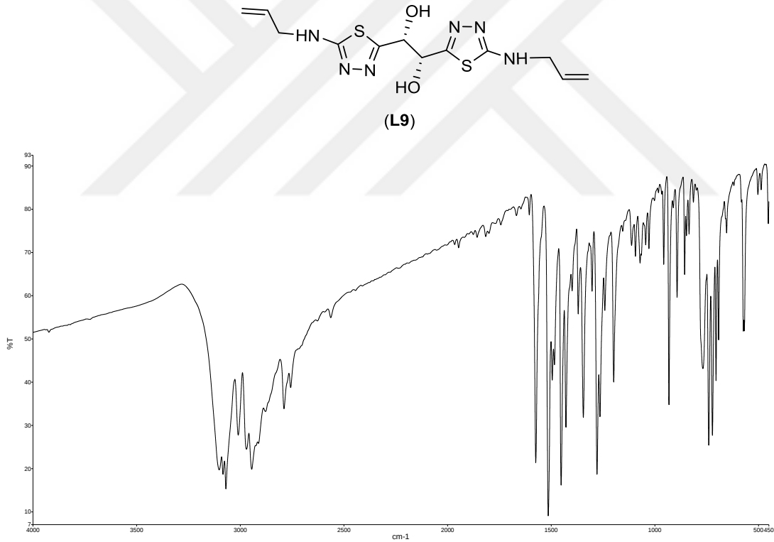
Şekil 4.25. (L9) molekülünün FT-IR spektrumu
