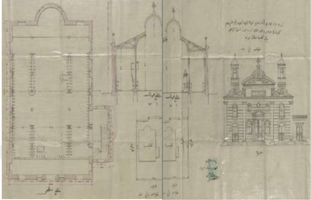
Ek 41: Edirne’de Panaiya Kilisesi’nin yeniden inşası ile ilgili hazırlanan taslaklar. (BOA, İ.AZN. , 79/32, H. 16 Cemaziyelahir 1326 / M. 16 Temmuz 1908).
