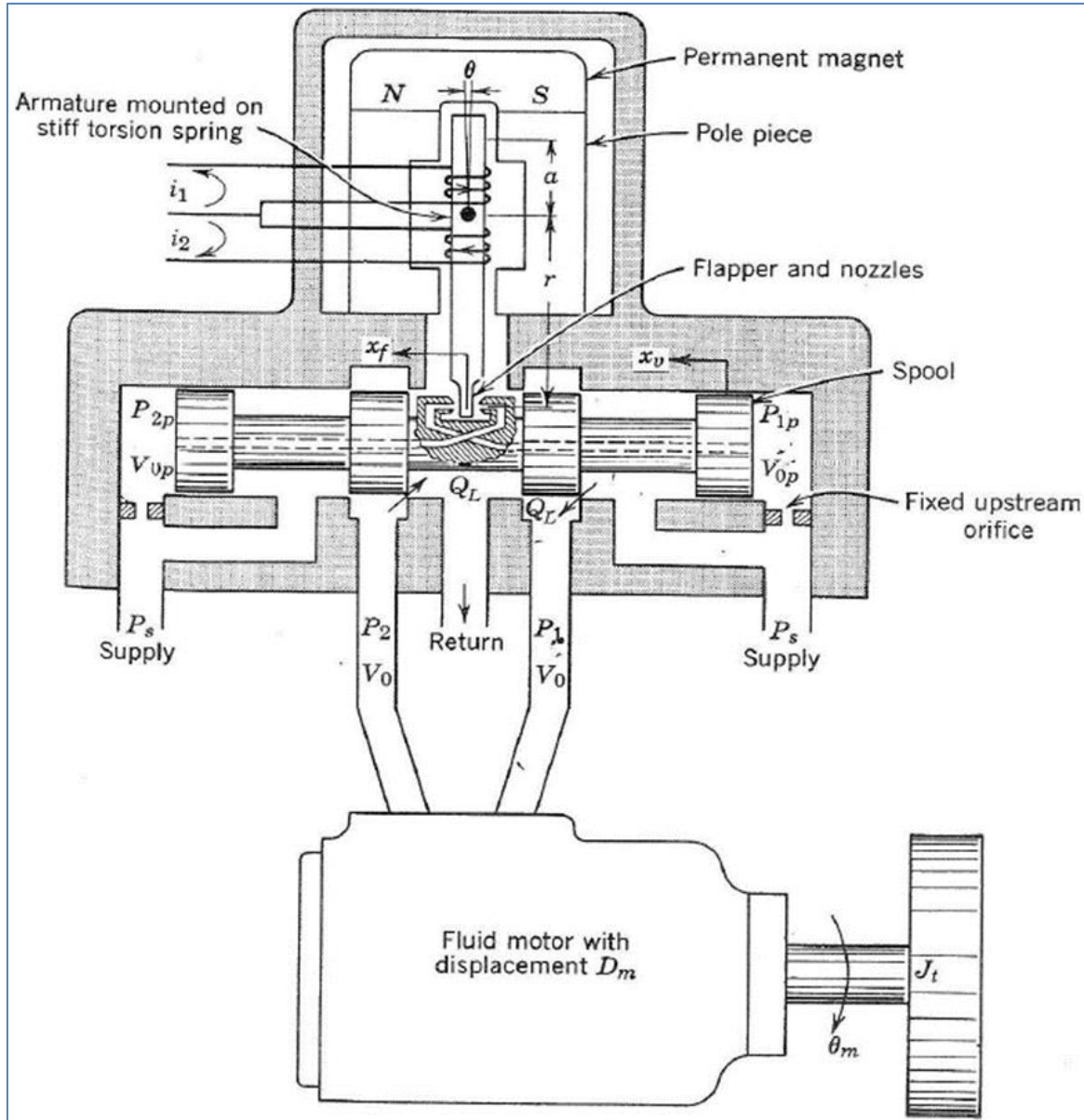
Şekil 2.6. Doğrudan geri beslemeli kanatçık nozul tip servo valf [1]
