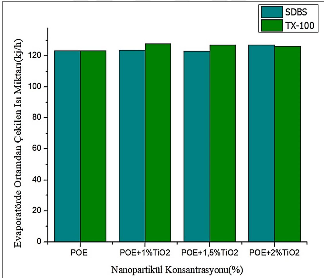
Şekil 4.29. Evaporatör tarafından ortamdan çekilen ısı miktarlarının karşılaştırılması
