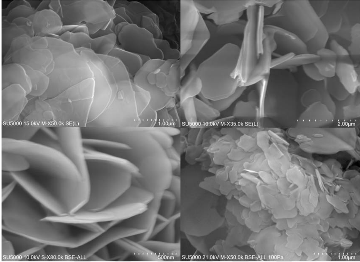
Resim 3.6. hBN nanopartikülleri için SEM analizi
