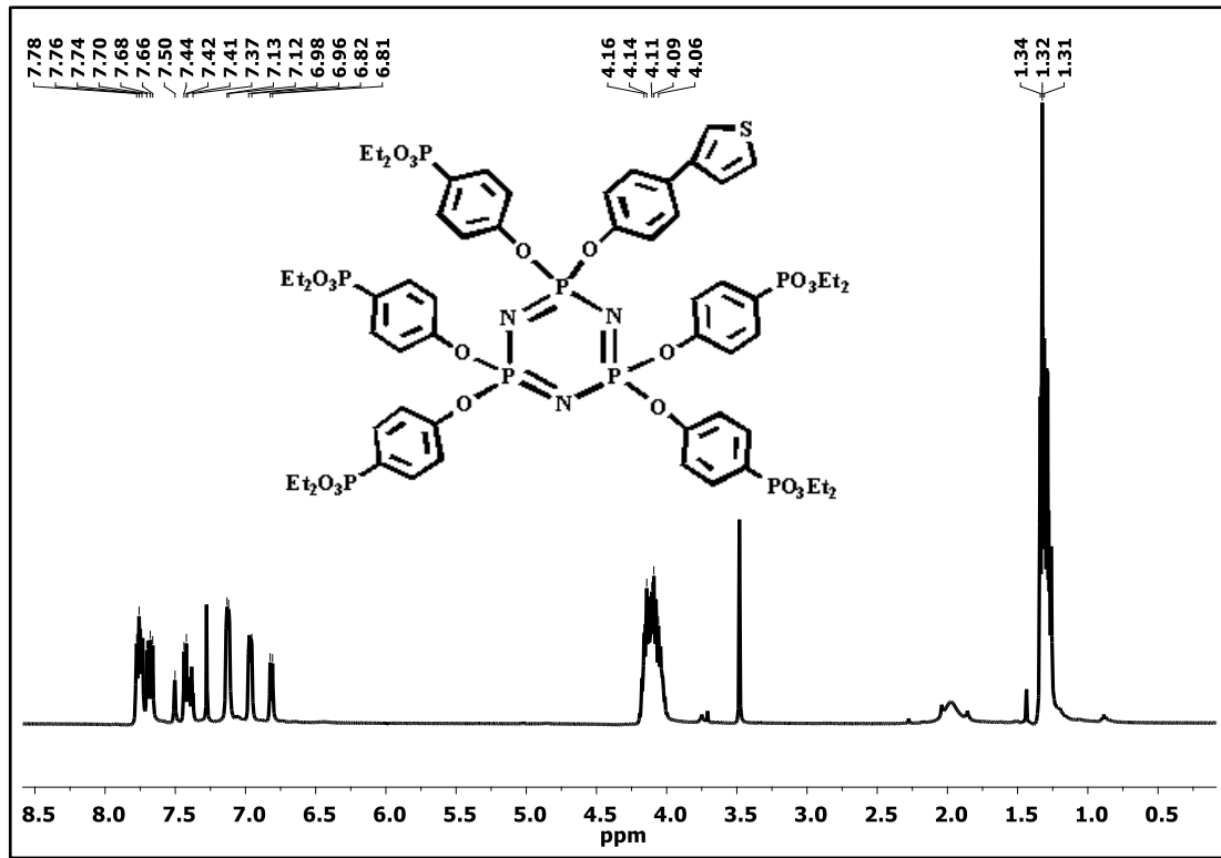
Şekil 4.21: 3 Bileşiğinin ^1\text{H} NMR Spektrumu.
