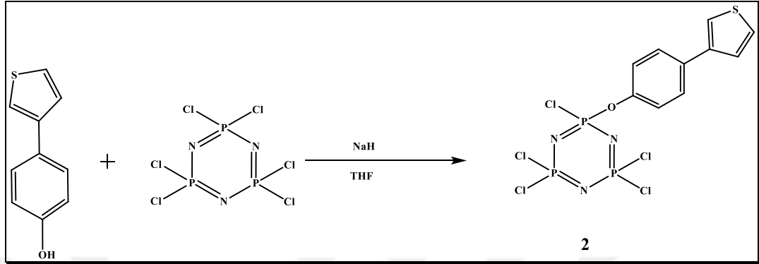
Şekil 4.2: 2 Bileşiğinin Sentezi.
