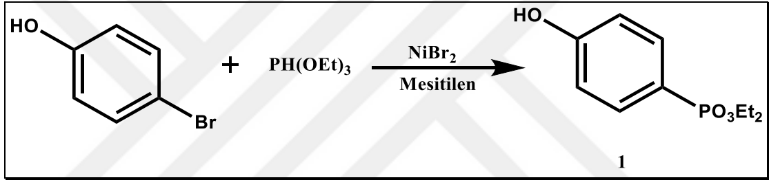
Şekil 4.1: 1 Bileşiğinin Sentezi.
