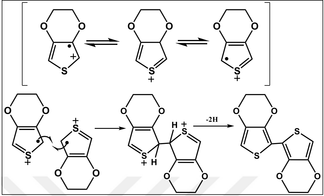
Şekil 2.13: EDOT'un Oksidatif Polimerizasyonu ile Oluşan Kenetlenme Türleri.
