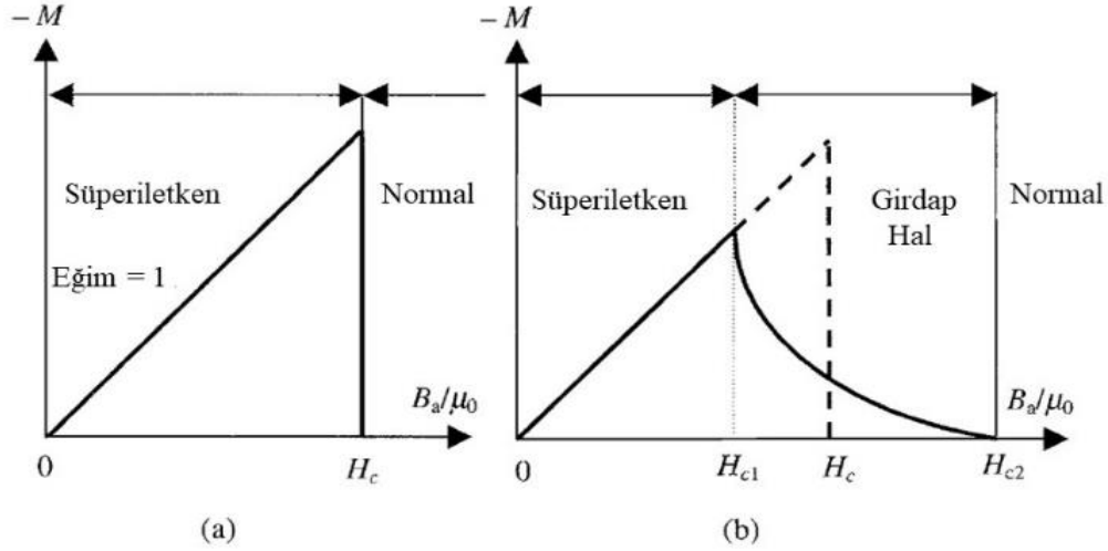
Şekil 3. 2. (a) Uzun, ince bir silindir şeklinde ideal I. tip süperiletkenin mıknatıslanma alan grafiği (b) II. tip II süperiletkenin mıknatıslanma alan grafiği. H_{c1} = B_{c1}/\mu_0 ve H_{c2} = B_{c2}/\mu_0 arasında numune karışık (girdap) durumdadır (Tari, 2003).
