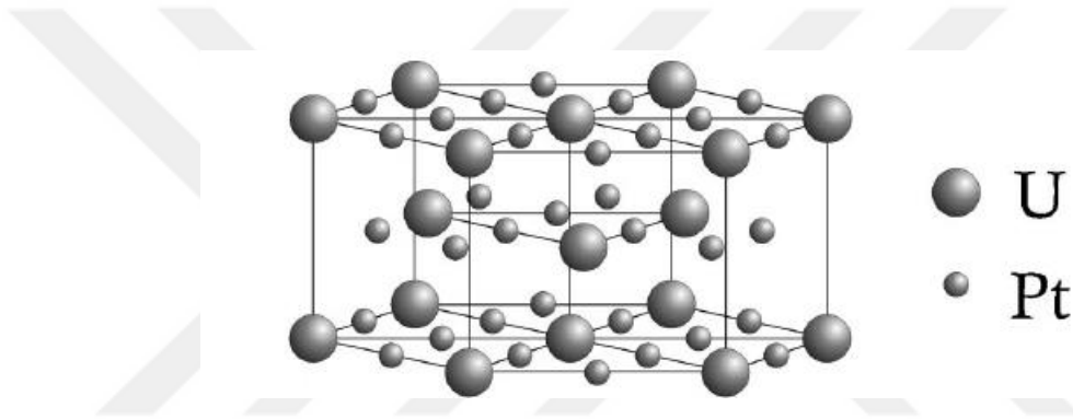
Şekil 6. 1. UPt_3 'ün kristal yapısı (Joynt ve Taillefer, 2002).
