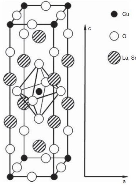
Şekil 6. 2. La_{2-x}M_xCuO_{4-y} 'in kristal yapısının gövde merkezli birim hücresi (Wesche, 2015).
