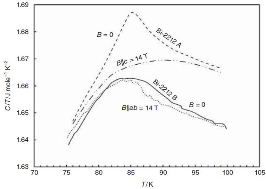
Şekil 6.18. Geçiş sıcaklığı yakınında uygulanan bir manyetik alanın varlığında ve yokluğunda iki Bi-2212 tek kristalinin öz ısıları (Wesche, 2015).
