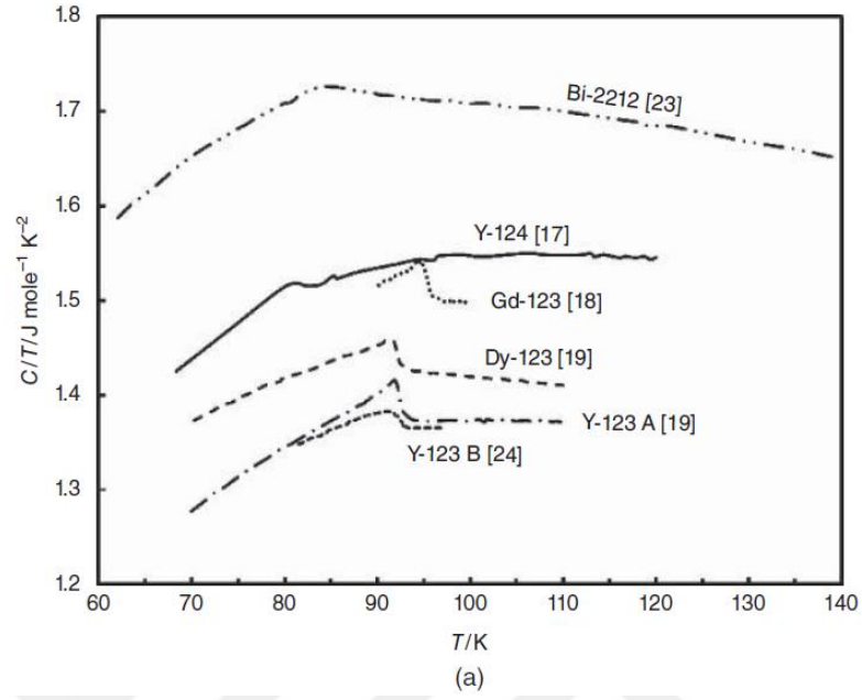
Şekil 6. 16. Geçiş sıcaklığı yakınında birkaç kuprat için yüksek T_c süperiletkenlik öz ısı (a) (Wesche, 2015).
