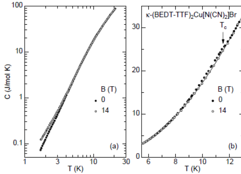
Şekil 6.29. \kappa - (BEDT - TTF)_2Cu[N(CN)_2]Br 'un öz ısıısının sıcaklığa bağımlılığı süperiletken durumda ( B = 0 T ) ve normal durumda ( B = 14 T ) (a) tam sıcaklık aralığı için ve (b) T_c = 11.5 K 'e yakın bölge için gösterilmiştir (Elsinger, vdl., 2000).
