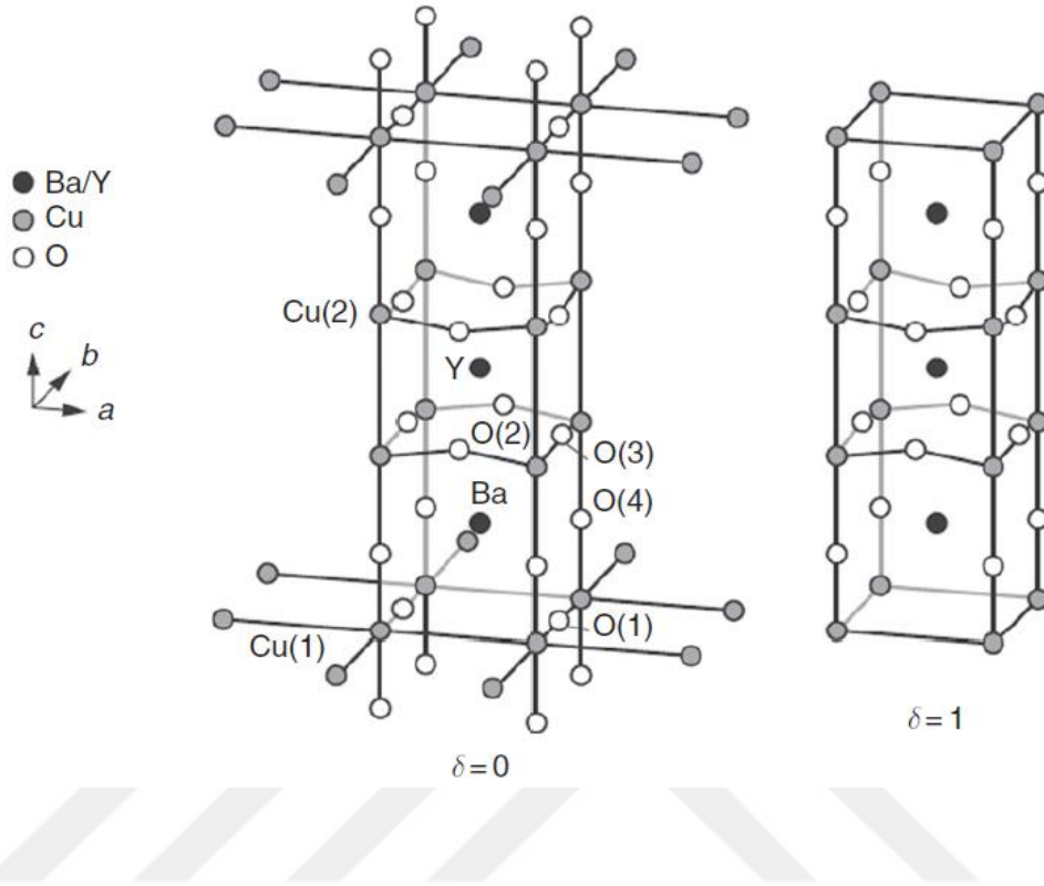
Şekil 6. 3. (a) \delta = 0 ve (b) \delta = 1 için YBa_2Cu_3O_{7-\delta} 'un kristalografik birim hücrelerinin şematik gösterimi (Fisk ve Ott, 2011).
