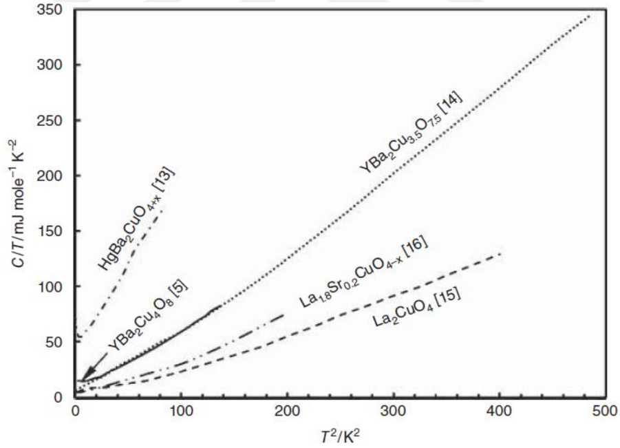
Şekil 6.15. Çeşitli kuprat, yüksek sıcaklık süperiletkenlerinin, düşük sıcaklık öz ısısı (Wesche, 2015).
