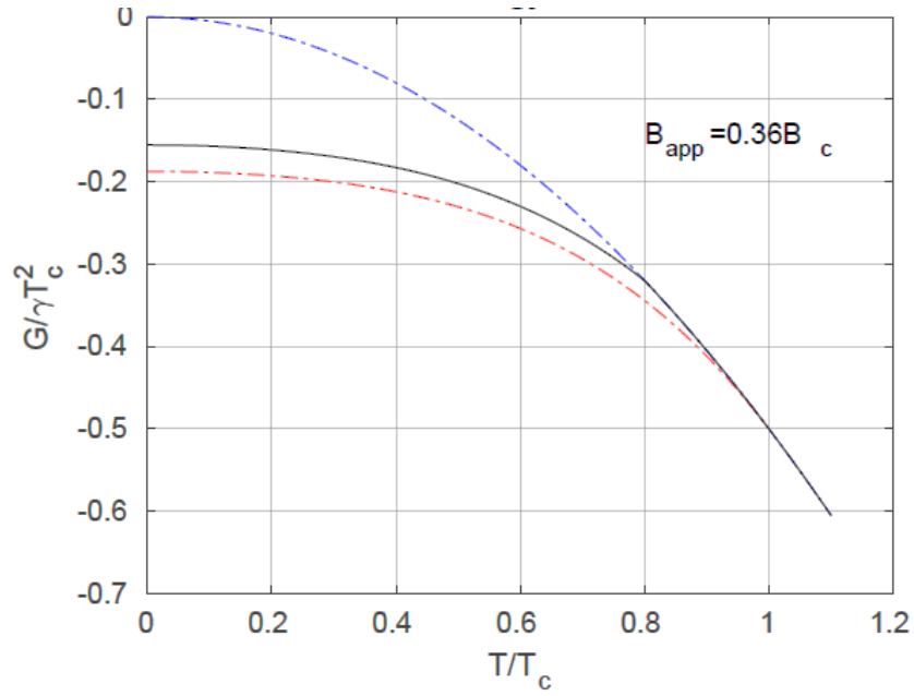
Şekil 5. 12. Normal ve süperiletken serbest enerjilerin zayıf manyetik alan varlığında sıcaklığa bağımlılığı (MATLAB kullanılarak çizilmiştir).
