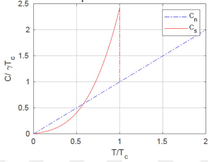
Şekil 5. 5. Normal ve süperiletken öz ısıların sıcaklığa bağımlılığı (MATLAB kullanılarak çizilmiştir).
