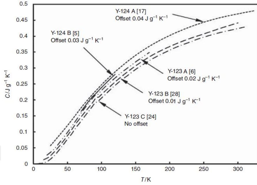
Şekil 6.20. Çeşitli yitrium bazlı kuprat süperiletkenlerin öz ısı verileri (Wesche, 2015).
