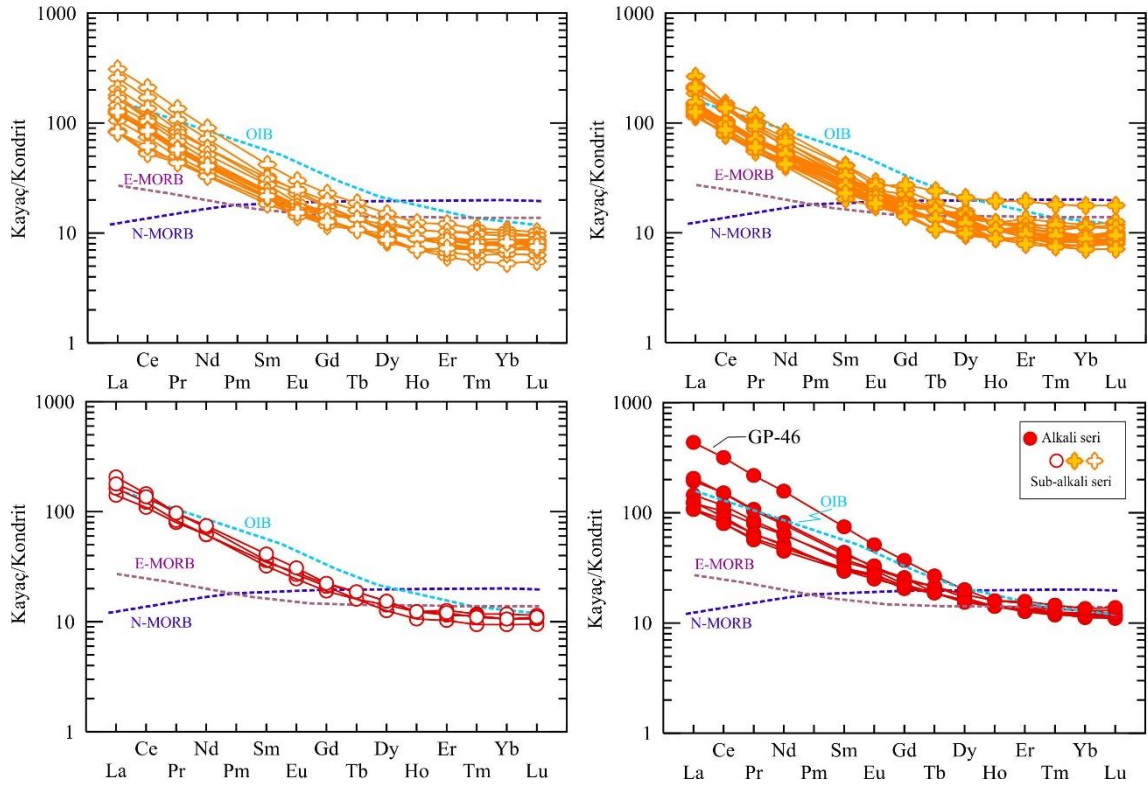
Şekil 6.10. Galatya Volkanik Provensi volkanik kayalarlarının kondrite göre normalize edilmiş nadir toprak element içerikleri diyagramı (Sun ve McDonough, 1989).
