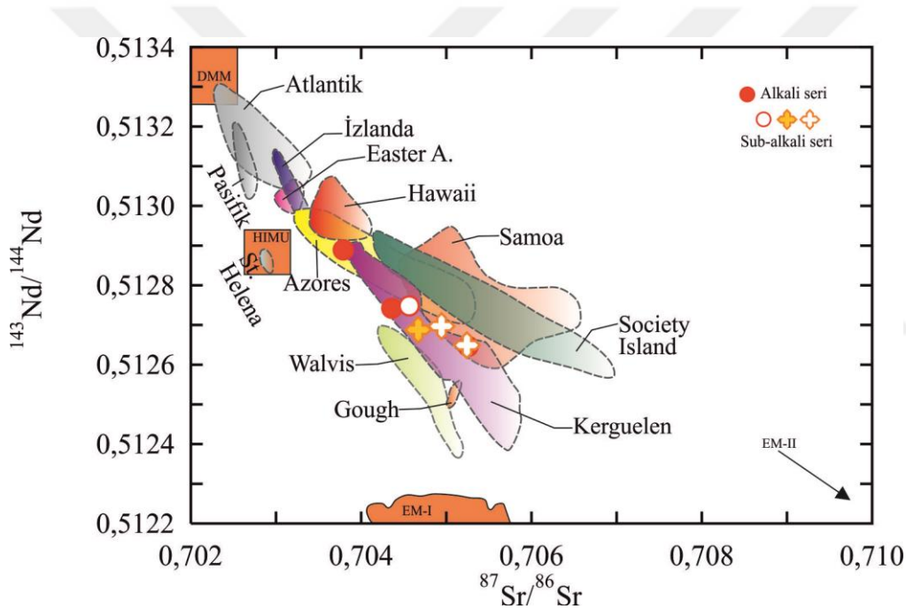
Şekil 7.13. Galatya Volkanik Provensi volkanik kayaçlarının izotopik bileşimlerinden itibaren dünyadaki diğer volkanik bölgeler ile karşılaştırılması (Volkanik bölgeler Zindler ve Hart, 1986 ve Sun ve McDonough, 1989)
