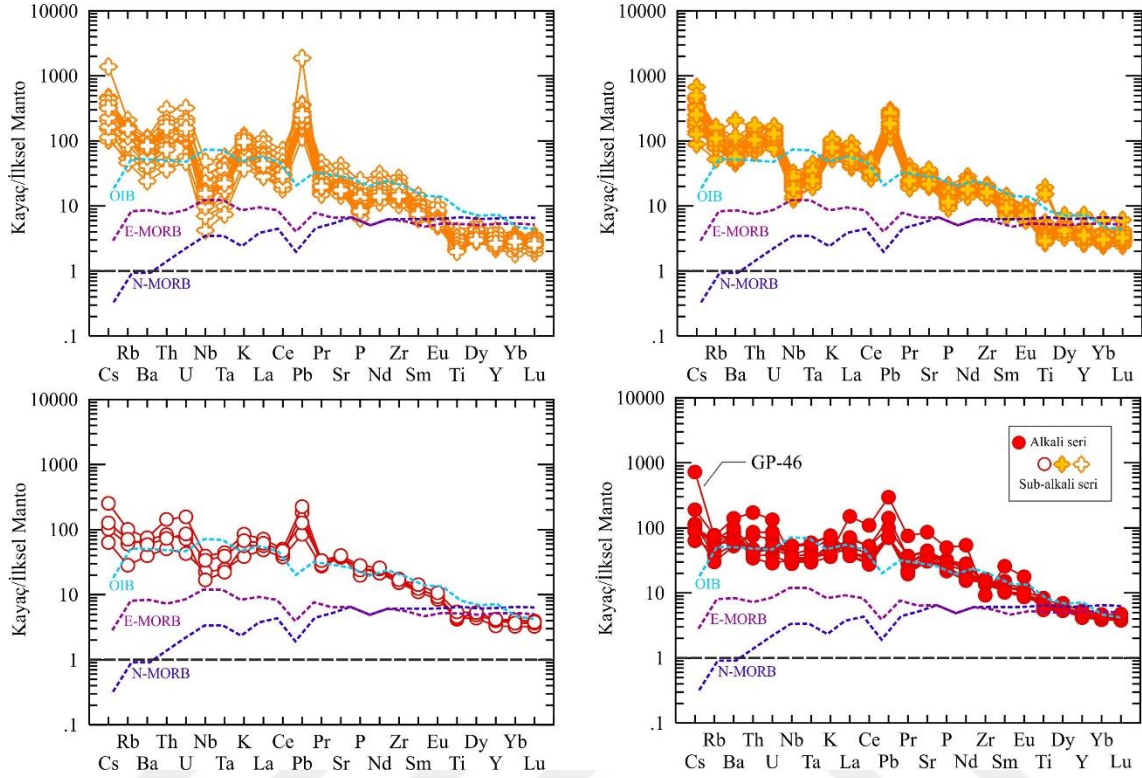
Şekil 6.8. Galatya Volkanik Provensi kayaçlarının ilksel mantoya göre normalize edilmiş çoklu element diyagramları (Sun ve McDonough, 1989).
