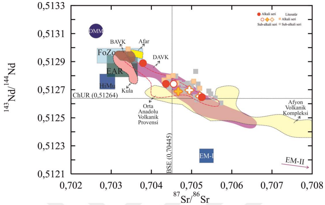
Şekil 6.12. Galatya Volkanik Provensi volkanik kayaçlarına ait izotop bileşimlerinin diğer volkanik kayaçlar ile karşılaştırılmasına ait diyagram. BAVK: Batı Anadolu Volkanik Kayaçları (Geç Miyosen; Aldanmaz vd., 2006; Kuvaterner Kula Volkanikleri (Alıcı vd., 2000), Orta Anadolu Volkanik Provensi (Orta Miyosen-Pliyosen, Di Guiseppe vd., 2018), DAVK: Doğu Anadolu Volkanik Kayaçları (Miyosen- Pleistosen, Buket ve Temel, 1998; Di Guiseppe vd., 2017); Afyon Volkanik Kompleksi (Miyosen, Prelevic vd., 2012); Afar Sorgucu (Deniel vd., 1994).
