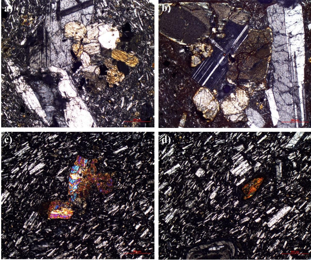
Şekil 5.6. a) Trakitik birimlerde ilk mineral birlikteliğine sahip kayalarda gözlenen a) Yarı özşekli piroksenlerin oluşturduğu glomeroporfirik doku, b) Polisentetik ikizlenmeleri ile tipik iri taneli plajiyoklaz mineralleri ve aralarını dolduran piroksenler, c) İkinci tip mineral birlikteliği gösteren kayaç içindeki orta taneli piroksenlerin oluşturduğu glomeroporfirik doku, d) Hamur içinde yönlenmiş vaziyette bulunan plajiyoklazlar.
