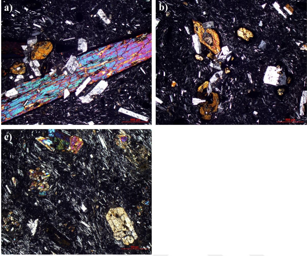
Şekil 5.5. Andezitik birimlerde gözlenen a) Mega amfibol fenokristali, b) Poikilitik doku sergileyen amfiboller ile feldispatların oluşturduğu kümelenme ve mikrolitlerdeki yönlenmeler, c) Tamamen mikrolitlerden oluşmuş hamur içerisindeki ince-orta taneli piroksen ve amfibollerin oluşturduğu glomeroporfirik doku
