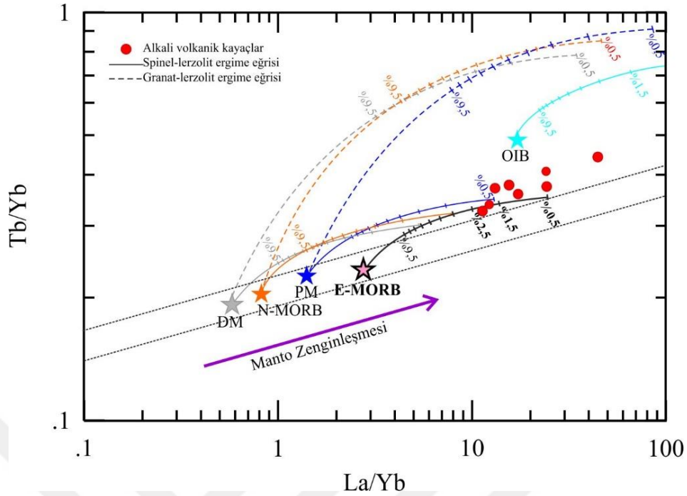
Şekil 7.5. Galatya Volkanik Provensi alkali volkanik kayaçlarına ait Tb/Yb- La/Yb diyagramı. Kısmi ergime eğrileri çiziminde kullanılan parametreler Çizelge 7.1'deki gibidir. DM: Tüketilmiş Manto (Salters ve Stracke, 2004), E-MORB: Zenginleşmiş MORB, N-MORB: Normal MORB, PM: İlk Manto ve OIB: Okyanus Adası Bazaltları (Sun ve McDonough, 1989),
