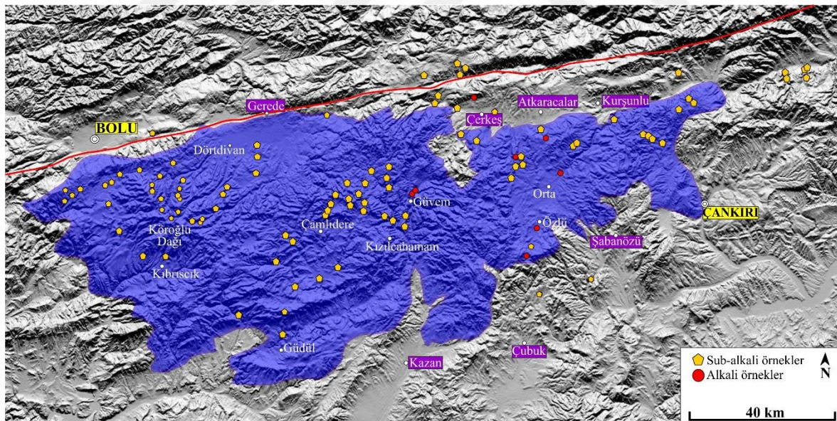
Şekil 3.1. Galatya Volkanik Provensi'nde yürütülen arazi çalışmaları esnasında alınan örneklemelerin lokasyonları
