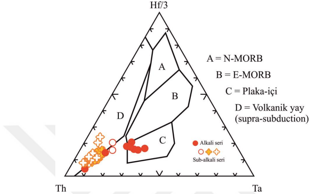
Şekil 7.11. Galatya Volkanik Provensi volkanik kayaçlarına ait tektonik ortam ayırtman diyagramı (Wood, 1980)
