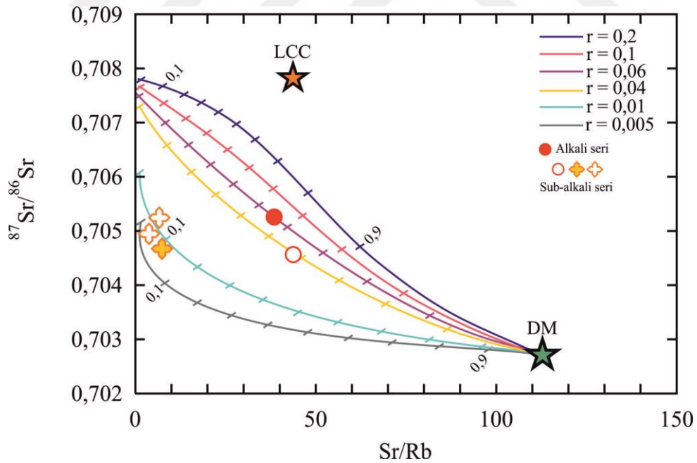
Şekil 7.3. Galatya Volkanik Provensi volkanik kayaçlarının izotop bileşimlerinden itibaren oluşturulan AFC modellemesi.
