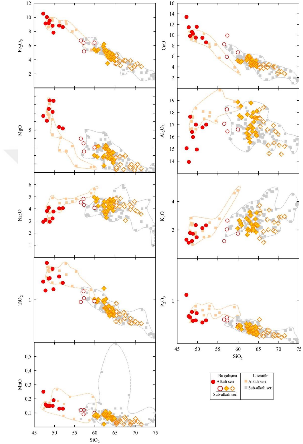
Şekil 6.4. Galatya Volkanik Provensi volkanik kayaçlarının artan \text{SiO}_2 içeriğine bağlı majör oksit değişim diyagramları
