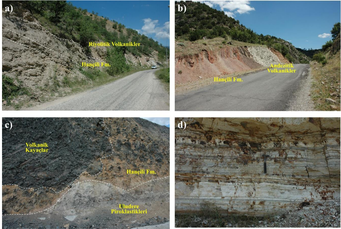
Şekil 4.2. Galatya Volkanik Provensi'nde gözlenen Hançili Formasyonu'na ait birimler: a) Kurşunlu doğusunda gözlenen riyoitik birimler tarafından üzerlenen killi kumtaşları, b) Çerkeş civarında andezitik volkanikler tarafından kesilmiş turuncu renkli marn-kumtaşı aralanması, c) Kurşunlu civarında gözlenen, volkanik kayaçlar ile arakatlı şekilde bulunan turuncumsu-sarımsı killi kumtaşları, d) Güvem, Beşkonak civarında gözlenen tabakalı, killi ve makrofosil içerikli kumtaşları.
