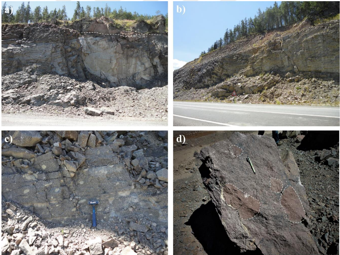
Şekil 4.18. a) Karaköy (Kıbrısık, Bolu) civarında incelenen, gri renkli lavların pembemsi lavlar içerisine sokulum yaptığı volkanik seri, b) Gri renkli lavların oluşturduğu sokulum, c) Genç lavların içinde özümselemeyen pembemsi, daha yaşlı olan lava ait parçalar, d) Boyları 40 santimetreye varan anklavlar.
