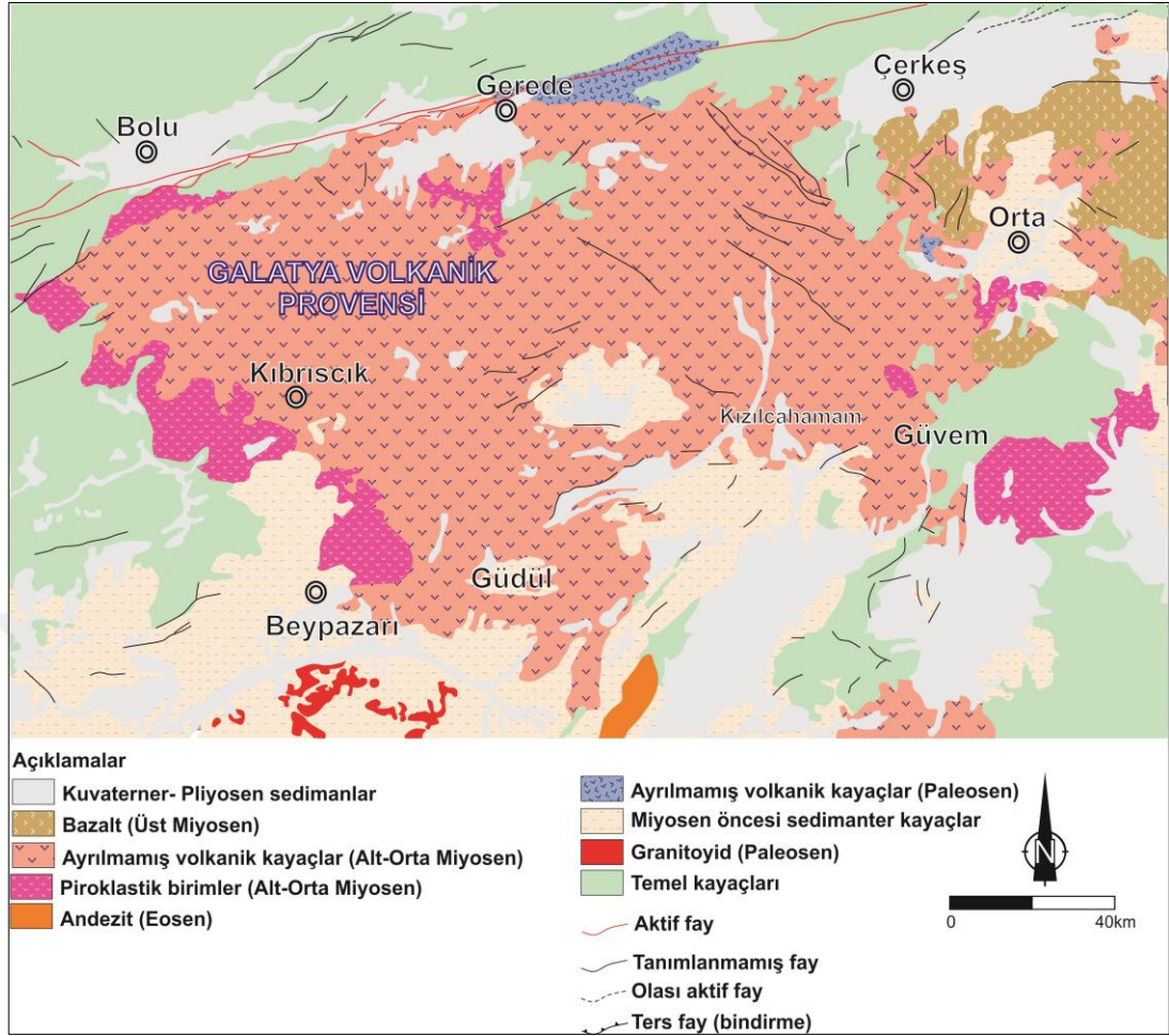
Şekil 1.2. Galatya Volkanik Provensi'nin genelleştirilmiş jeolojik haritası (MTA 1/500.000 ölçekli jeoloji haritasından değiştirilerek).
