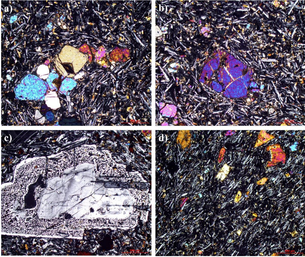
Şekil 5.8. İkinci grup mineral birlikteliğini içeren bazaltik birimlerde gözlenen a) Glomeroporfirik dokulu olivinler, b) Mikrolitler şeklinde gözlenen olivin ve oksit mineralleri ile orta taneli, parlak girişim rengi ile tipik olivin, c) Kenarları itibariyle cam kapanımları içeren feldispat, d) Orta-ince taneli özşekilsiz piroksenler
