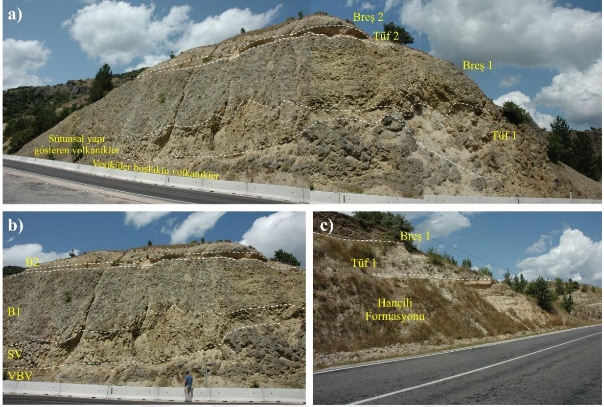
Şekil 4.7. a) Beşkonak civarında incelenen volkanik istif. Vesiküler boşluklu volkanik kayaç üzerine gelen ve sütunsal yapı gösteren volkanik kayaçlar ikinci bir fazı temsil etmektedir, b) Bu istifin KB'dan görünüşü. c) İstifin devamında tüf ve breşlerin üzerlediği Hançili Formasyonu'na ait sedimanter birimler.
