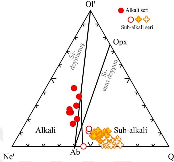
Şekil 6.3. Çalışma alanına ait örneklerin normatif mineralojilerine bağlı Ol- Ne- Q üçgen diyagramı (Ol: Olivin, Ne: Nefelin, Q: Kuvars, Al: Albit, Opx: Ortopiroksen)
