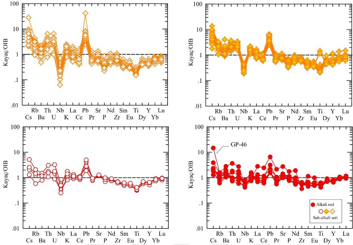
Şekil 6.9. Galatya Volkanik Provensi volkanik kayaların OIB'ye göre normalize edilmiş çoklu element diyagramları (Sun ve McDonough, 1989).
