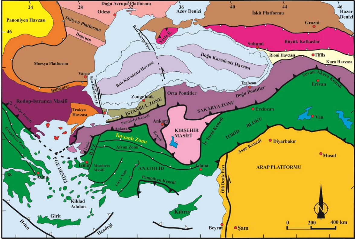
Şekil 4.1. Türkiye'nin ve çevresinin tektonik haritası (Okay ve Tüysüz'den, 1999).
