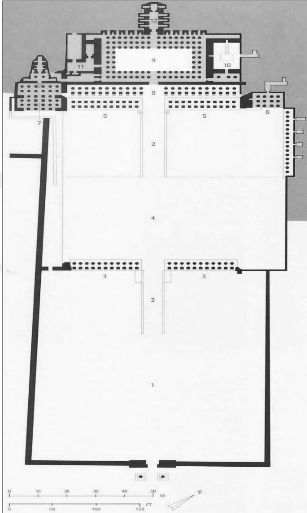
Resim 51 Hatşepsut tapınağı (Wildung 2009, s. 122)
