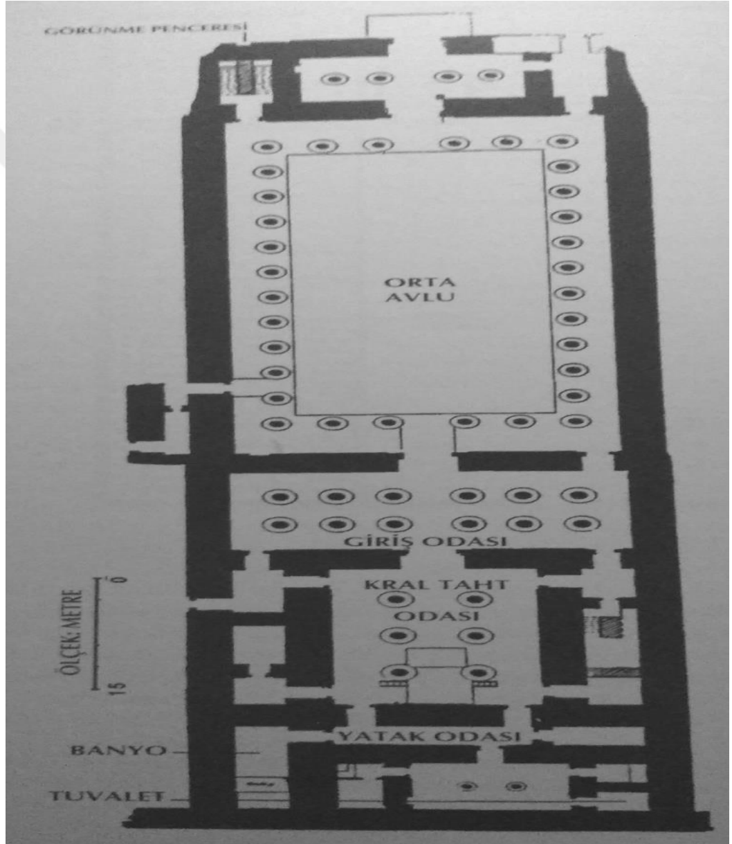
Resim 31 Merneptah sarayının planı (Brewer ve Teeter 2017, s. 170)
