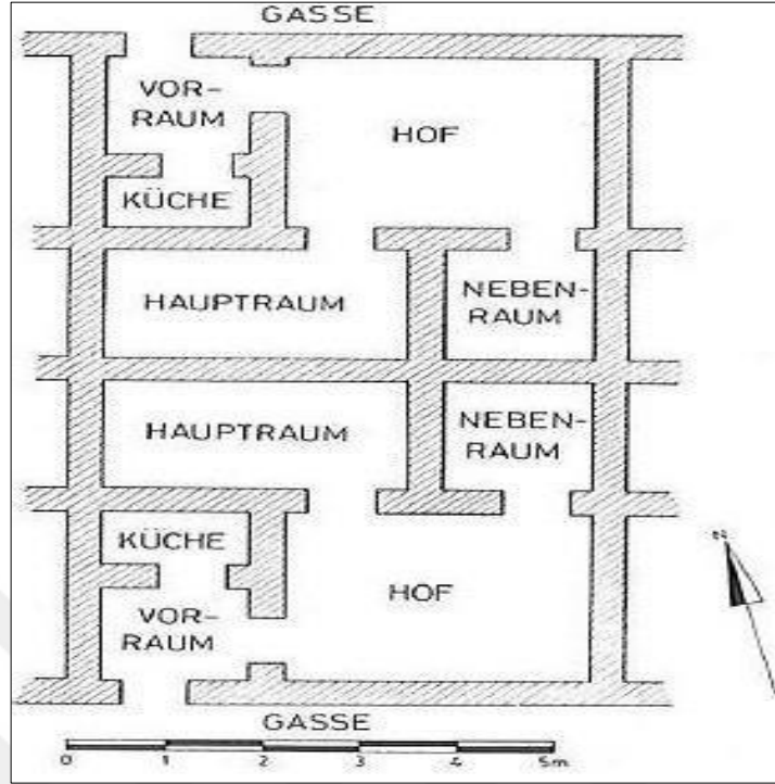
Resim 91 Dik yerleşime ait bir evin planı (Bietak 1996, s. 8)
