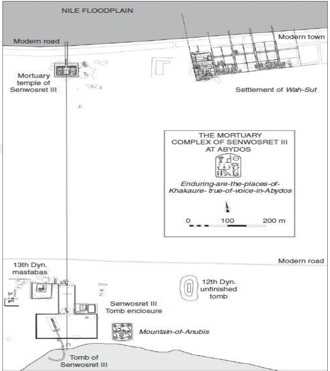
Resim 19 III. Senusret tapınağının planı (Moeller 2016, s. 291)
