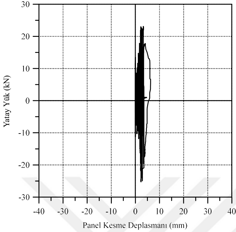
Şekil 4.13. DC50-2L yatay yük-panel kesme deplasmanı grafiği
