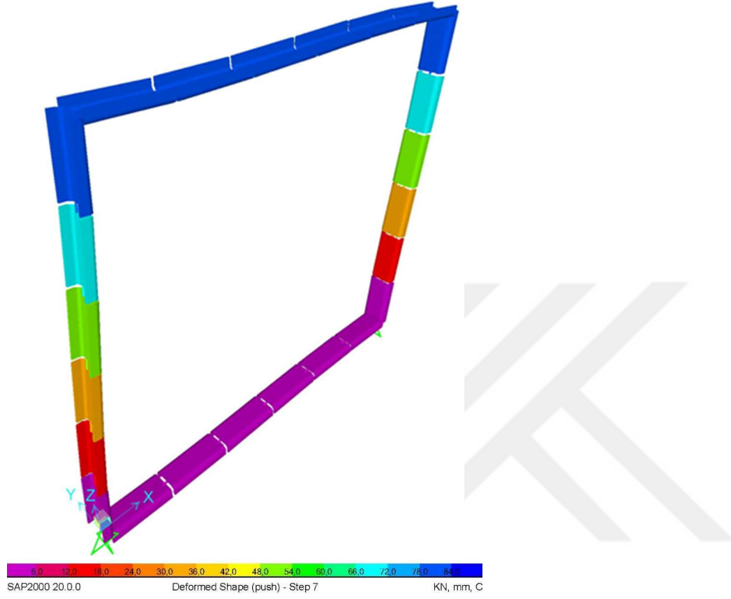
Şekil 3.3. Çerçevenin %3,00 kat ötelenme oranı adımımda deplasman analizi
