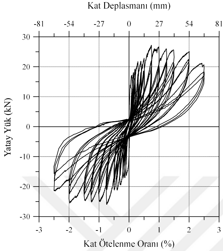
Şekil 4.14. TD bilşik çevrimsel yatay yük-kat ötelenme grafiğı
