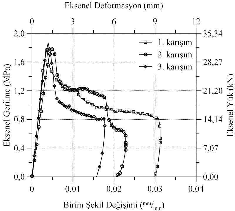
Şekil 3.8. Alçı harcı karışımların gerilme birim şekil değiştirme grafiği
