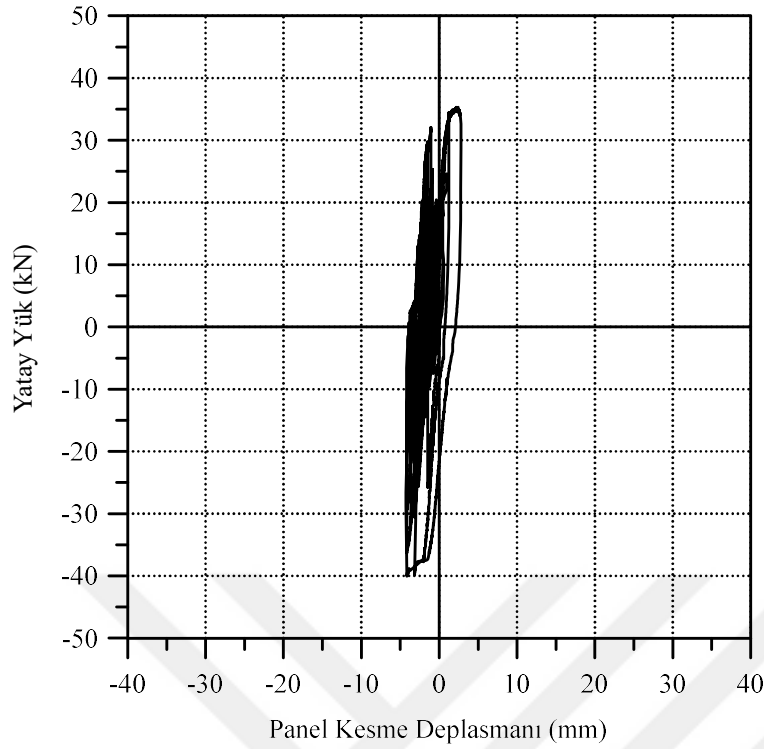
Şekil 4.7. C50-2L yatay yük-panel kesme deplasmanı grafiği
