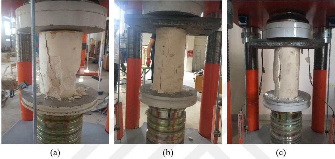
Resim 3.7. Alçı harcı karışımlarının aksel basınç deneyleri
