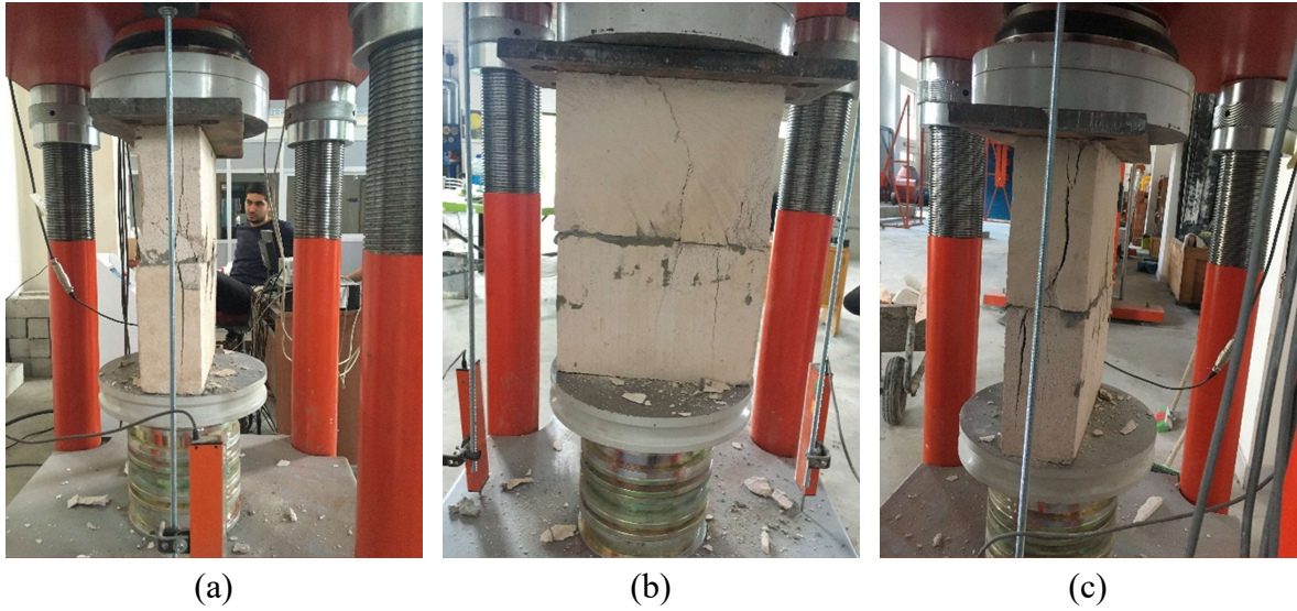
Resim 3.14. Gaz beton kâgir birimin eksenel basınç deneyleri
