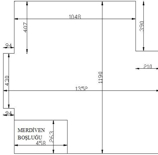
Şekil 4.12.Yapıya ait genel oturma krokisi
