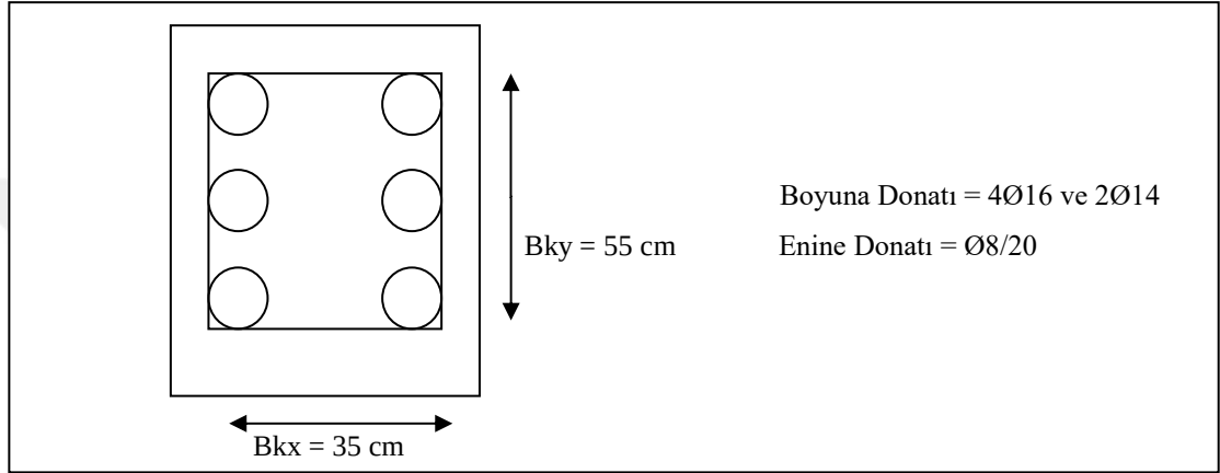
Şekil 4.11. Enine ve boyuna donatının birbirine en uzak eksenleri gösterir şema
