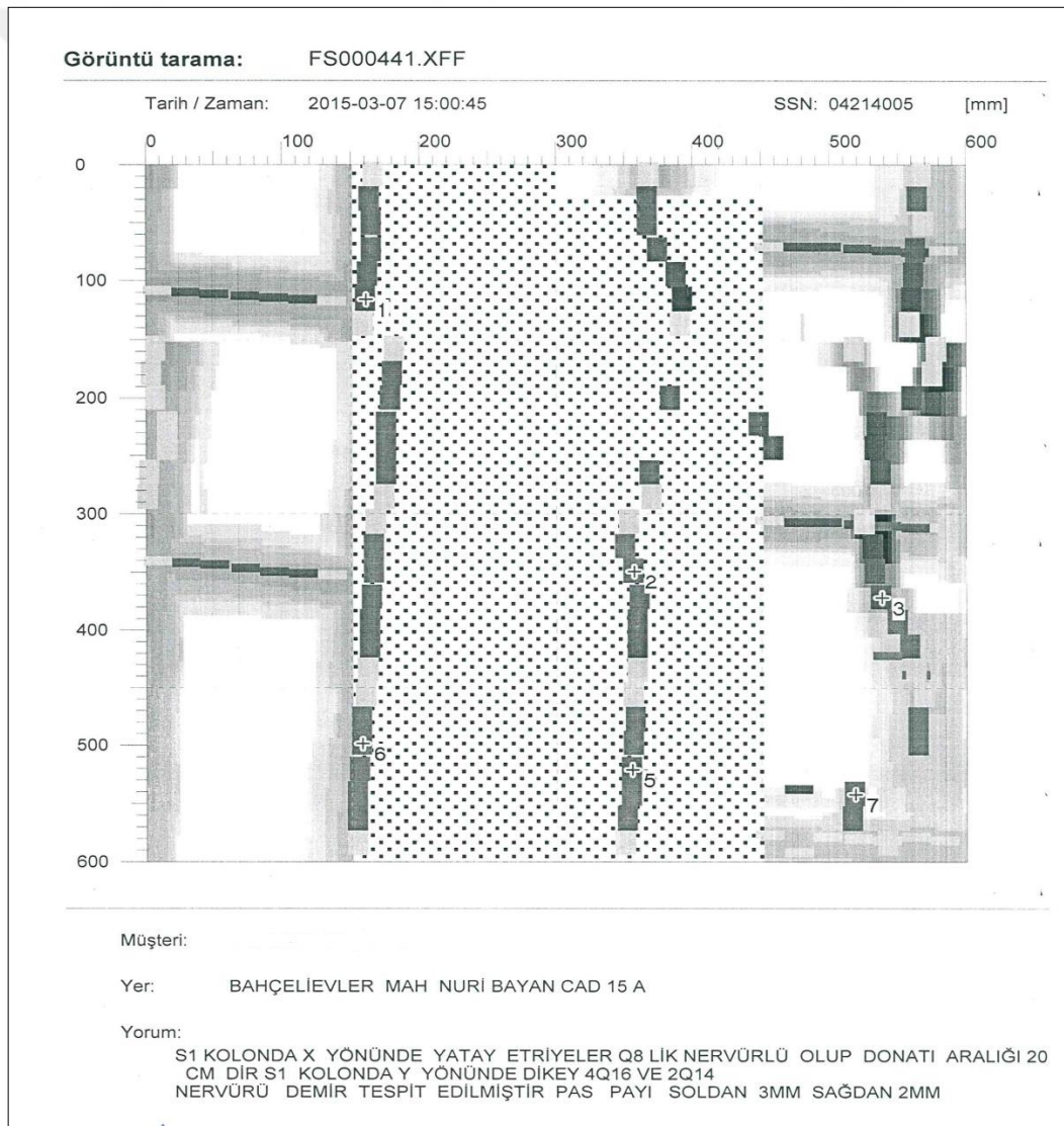
Şekil 3.17. C binası ile ilgili özel yapı analiz laboratuvarınca röntgen cihazı ile çalışma yapılarak donatı çapı, adeti ve sayısı ile ilgili tespit çalışmasını gösteren resmi evrak
