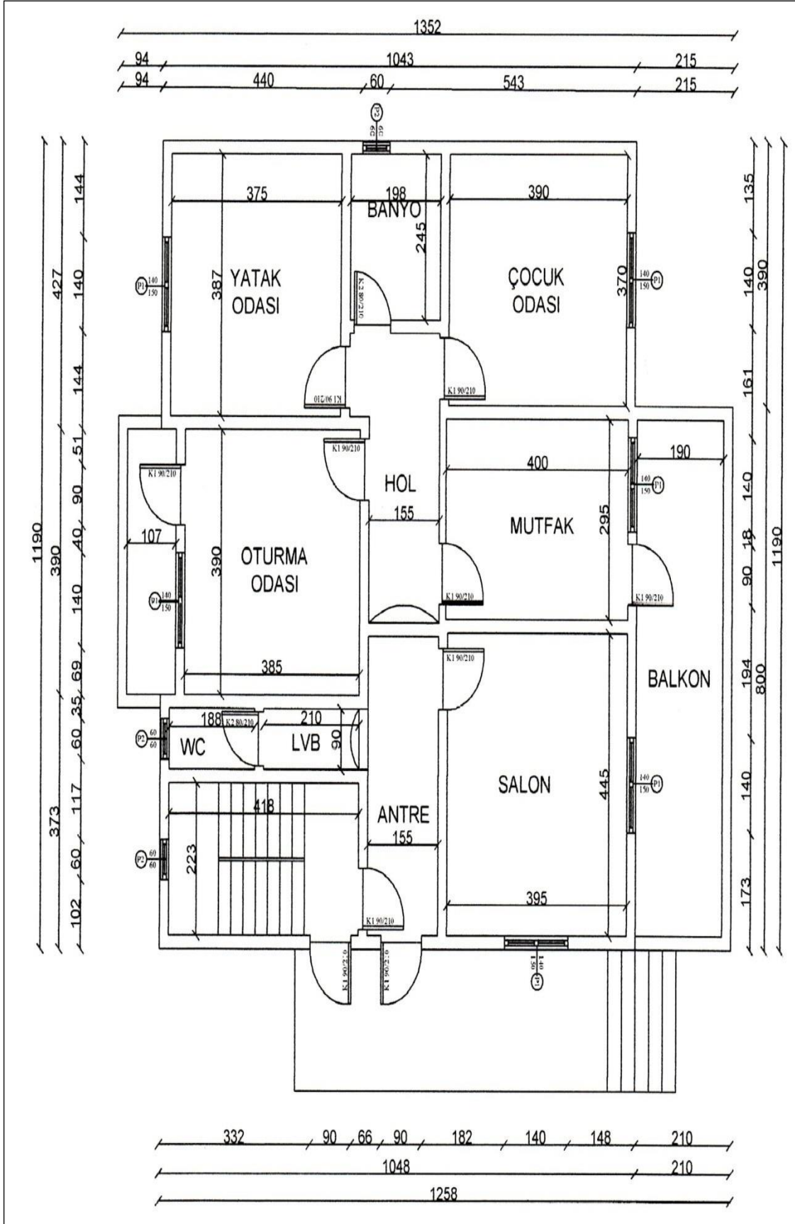
Şekil 3.19. D Yapısının kritik katının alınmış rölevesi
