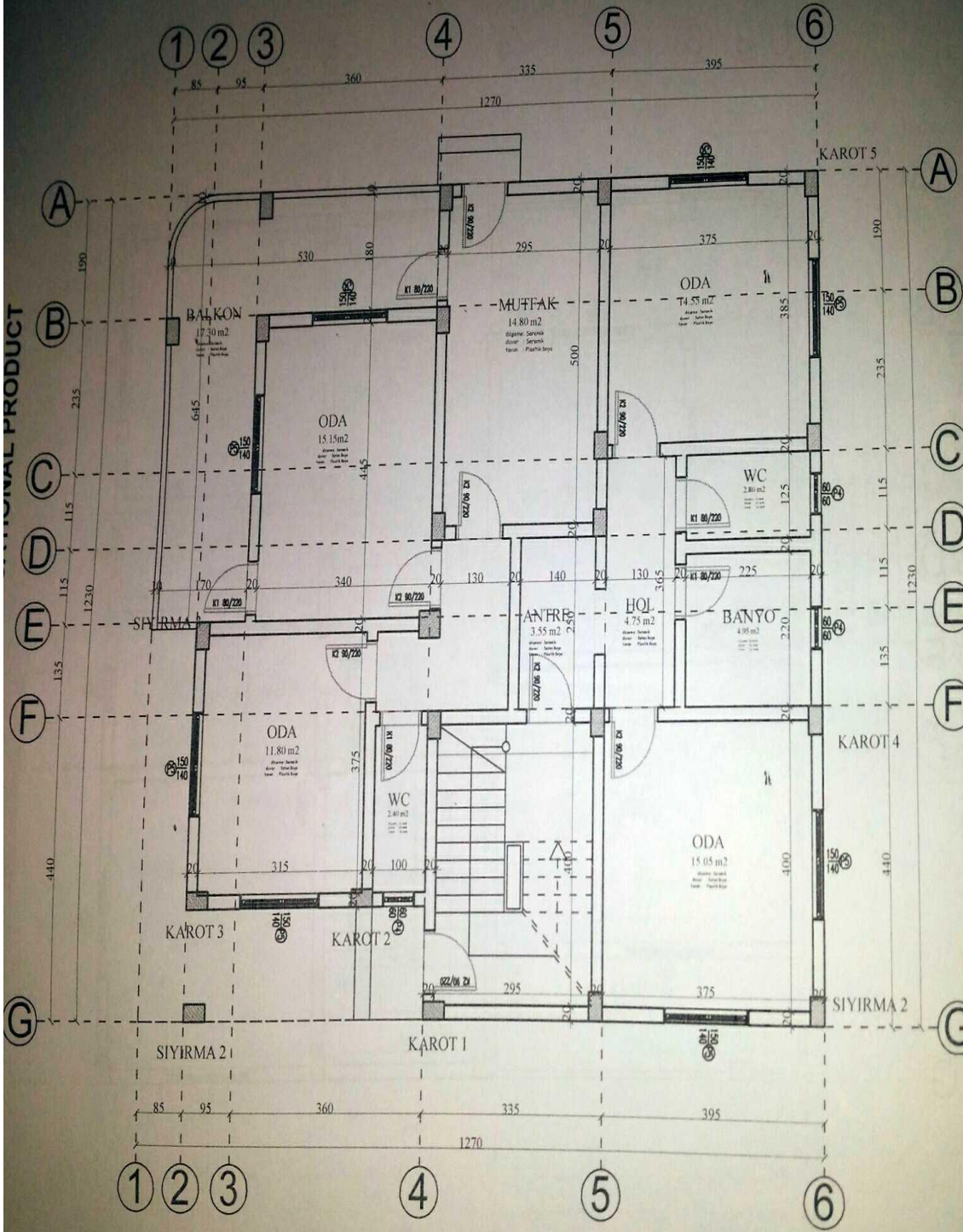
Şekil 3.28. E Yapısının kritik katının (zemin) alınmış rölevesi
