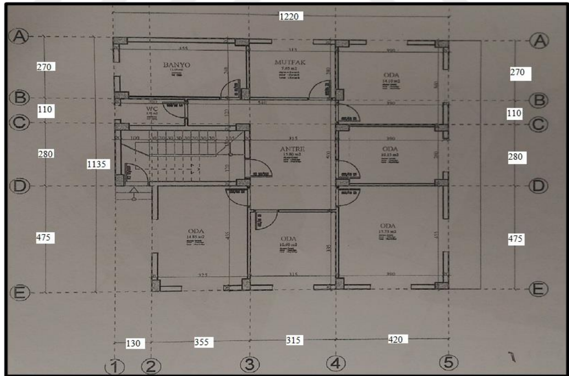
Şekil 3.3. A Yapısının alınmış rölevesi
