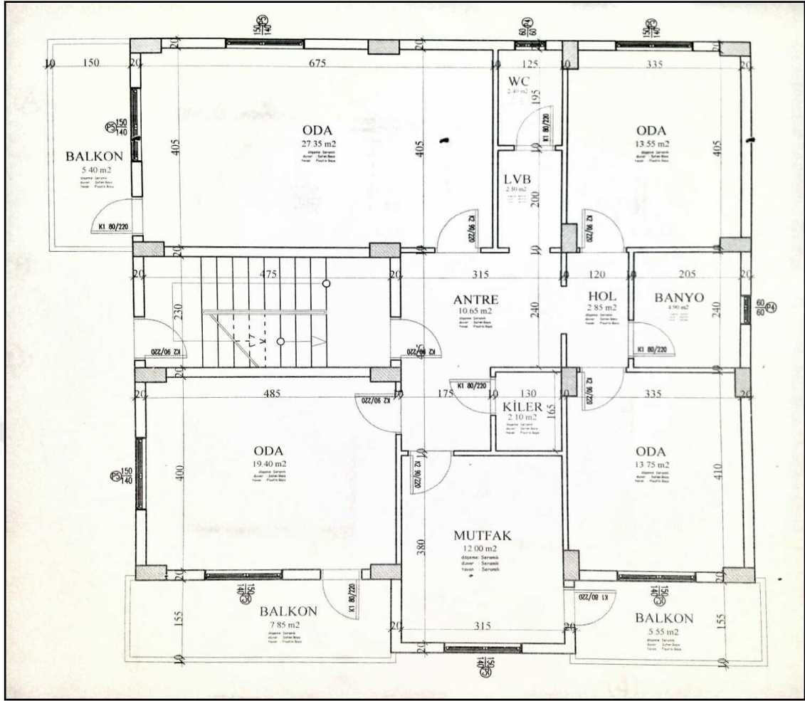
Şekil 3.9. B Yapısının alınmış rölevesi
