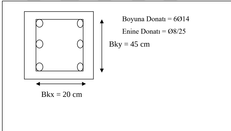
Şekil 4.13. Enine ve boyuna donatının birbirine en uzak eksenleri gösterir şema
