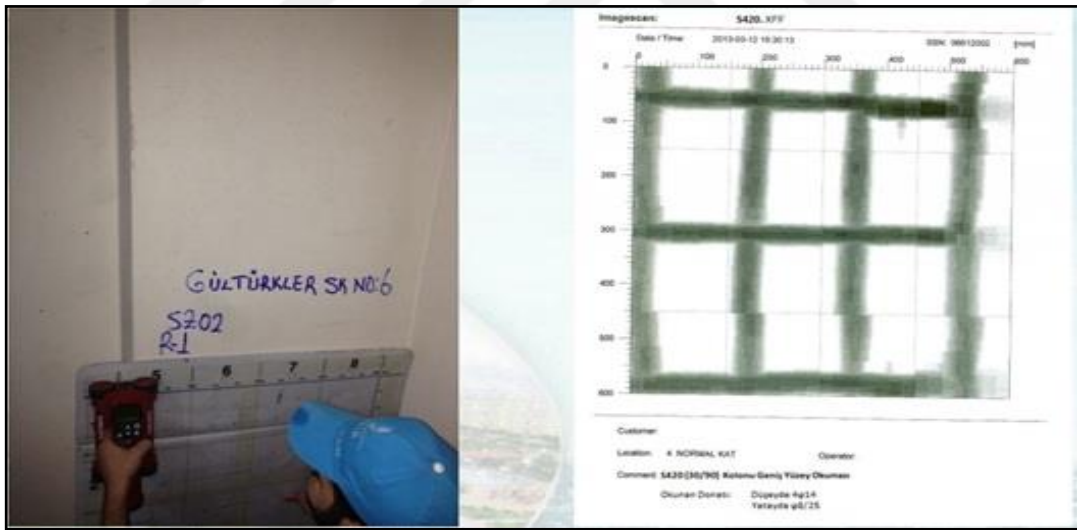
Şekil 2.13. Röntgen cihazı ile donatı taraması işlemi ve tarama sonucu örneği
