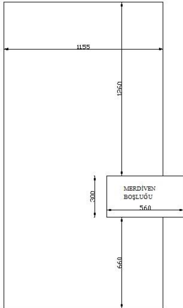
Şekil 4.10. Yapıya ait genel oturma krokisi
