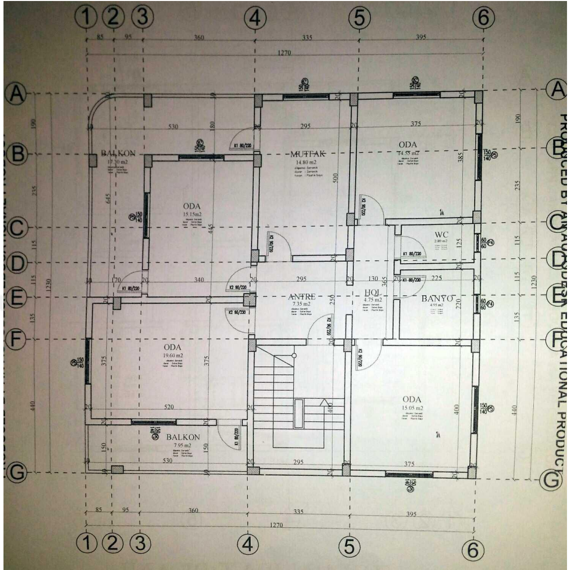
Şekil 3.29. E Yapısının normal katlarının alınmış rölevesi
