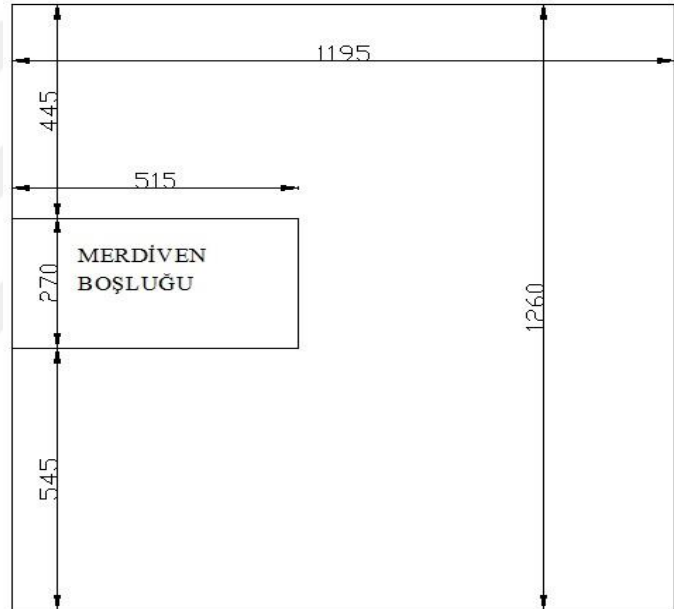
Şekil 4.8. Yapıya ait genel oturma krokisi
