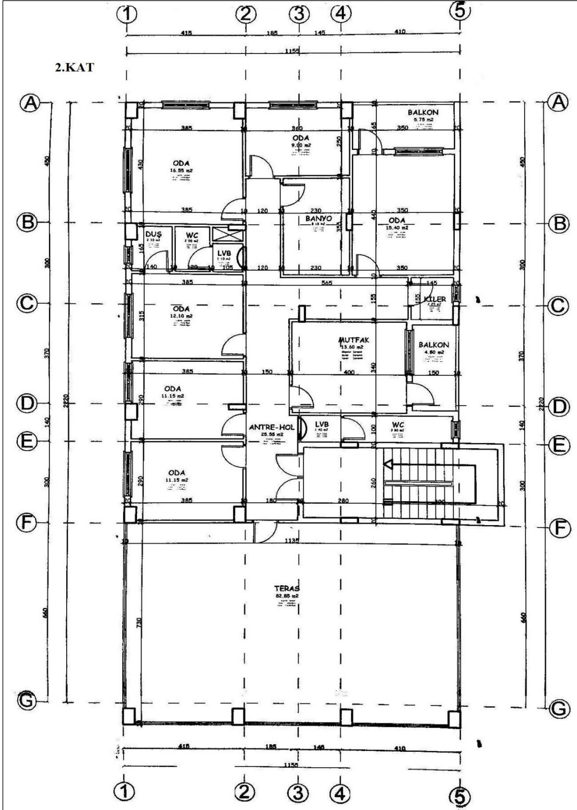
Şekil 3.14. a,b,c. Yapının sırasıyla Zemin, 1. ve 2. kat rölevelleri
