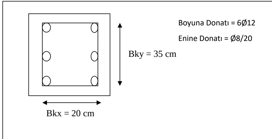
Şekil 4.15. Enine ve boyuna donatının birbirine en uzak eksenleri gösterir şema
