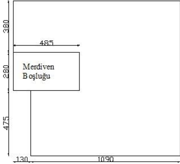
Şekil 4.6. Yapıya ait genel oturma krokisi
