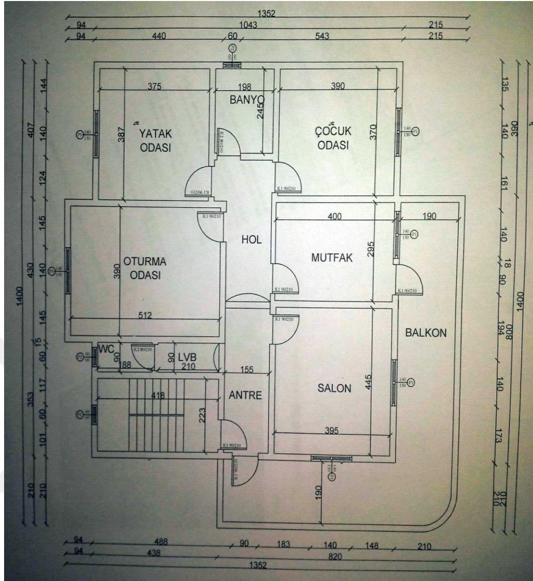
Şekil 3.20. D Yapısının 1. katının alınmış rölevesi
