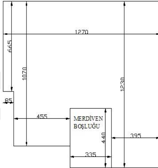
Şekil 4.14. Yapıya ait genel oturma krokisi
