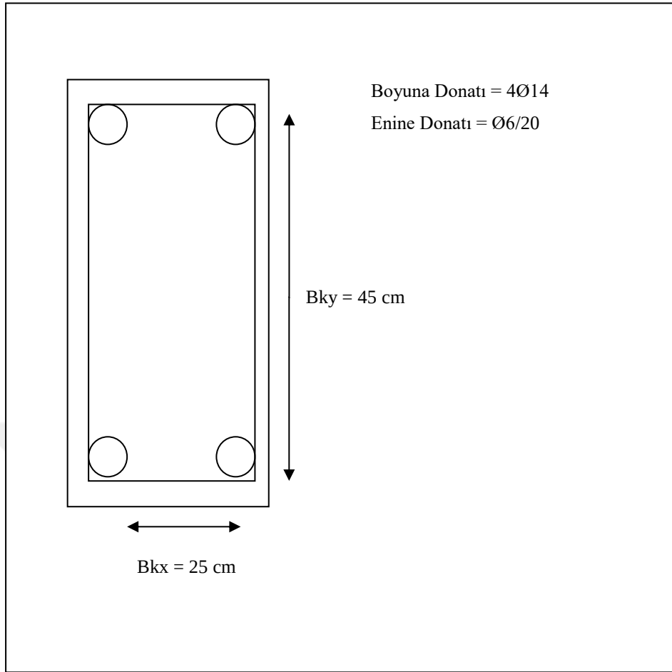
Şekil 4.7. Enine ve boyuna donatının birbirine en uzak eksenleri gösterir şema
