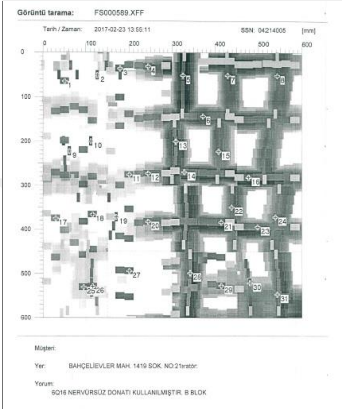
Şekil 3.12. B binası ile ilgili özel yapı analiz laboratuvarınca röntgen cihazı ile çalışma yapılarak donatı çapı, adetleri ve sayıları ile ilgili tespit çalışmasını gösteren resmi evrak
