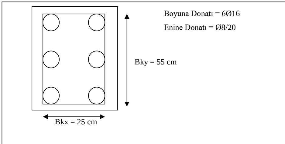
Şekil 4.9. Enine ve boyuna donatının birbirine en uzak eksenleri gösterir şema
