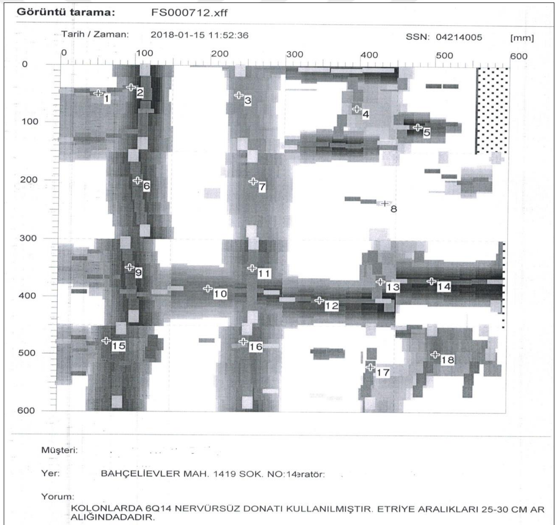
Şekil 3.26. D binası ile ilgili özel yapı analiz laboratuvarınca röntgen cihazı ile çalışma yapılarak donatı çapı, adet ve aralıkları ile ilgili tespit çalışmasını gösteren resmi evrak
