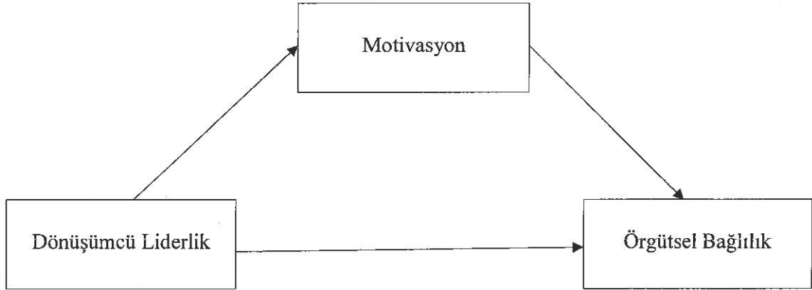
Şekil 4. Araştırmanın Modeli
