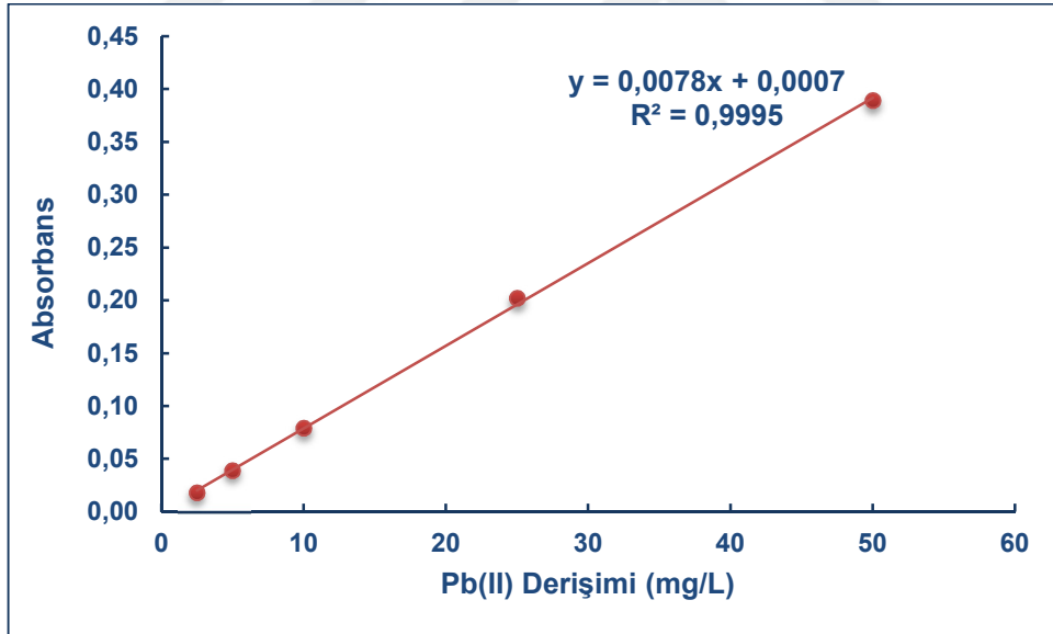
Şekil 2. Pb(II) iyonlarının tayininde kullanılan AAS'ye ait kalibrasyon grafiğı
