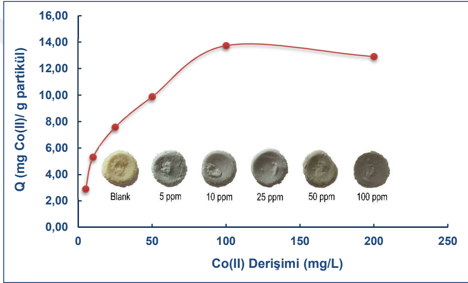
Şekil 4.26. Si-L partiküllerin adsorpsiyon kapasitesine Co(II) derişiminin etkisi (Deney koşulları; Si-L miktarı: 0.020 g, pH:6, çözeltili hacmi: 20 mL, karıştırma hızı: 400 devir/dk, karıştırma süresi: 120 dk)
