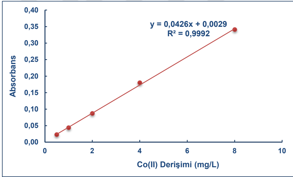
Şekil 4. Co(II) iyonlarının tayininde kullanılan AAS'ye ait kalibrasyon grafiğı
