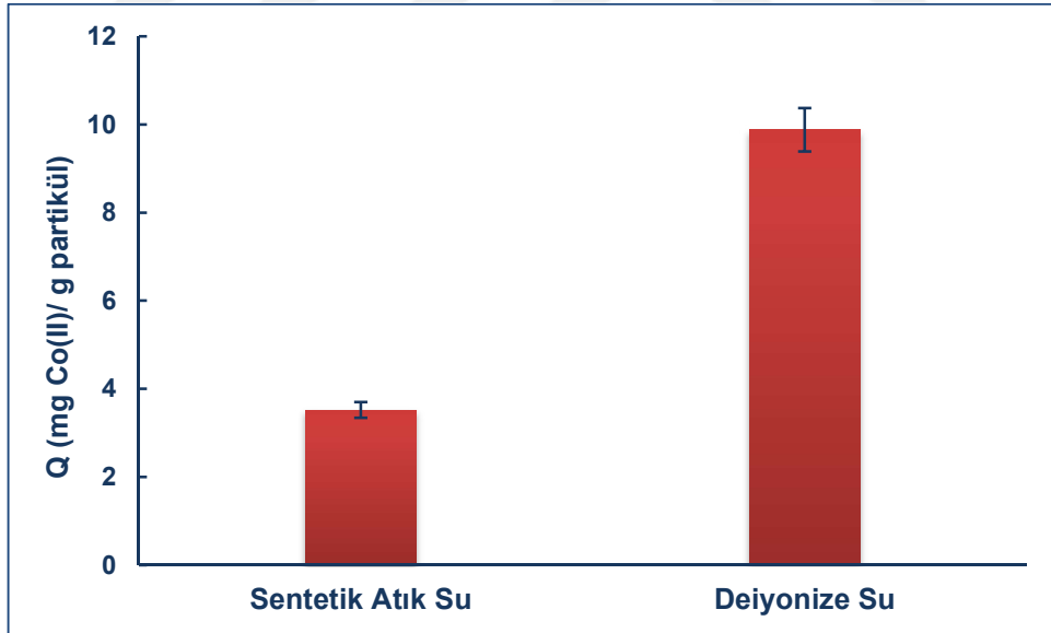
Şekil 4.28. Sentetik atık sudan Co(II) iyonu adsorpsiyonu (Deney koşulları; Si-L miktarı: 0.020 g, Co(II) derişimi: 50 mg/L, pH:6, çözelti hacmi: 20 mL, karıştırma hızı: 400 devir/dk, karıştırma süresi: 120 dk, N=3)
