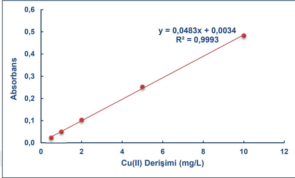
Şekil 1. Cu(II) iyonlarının tayininde kullanılan AAS'ye ait kalibrasyon grafiğı
