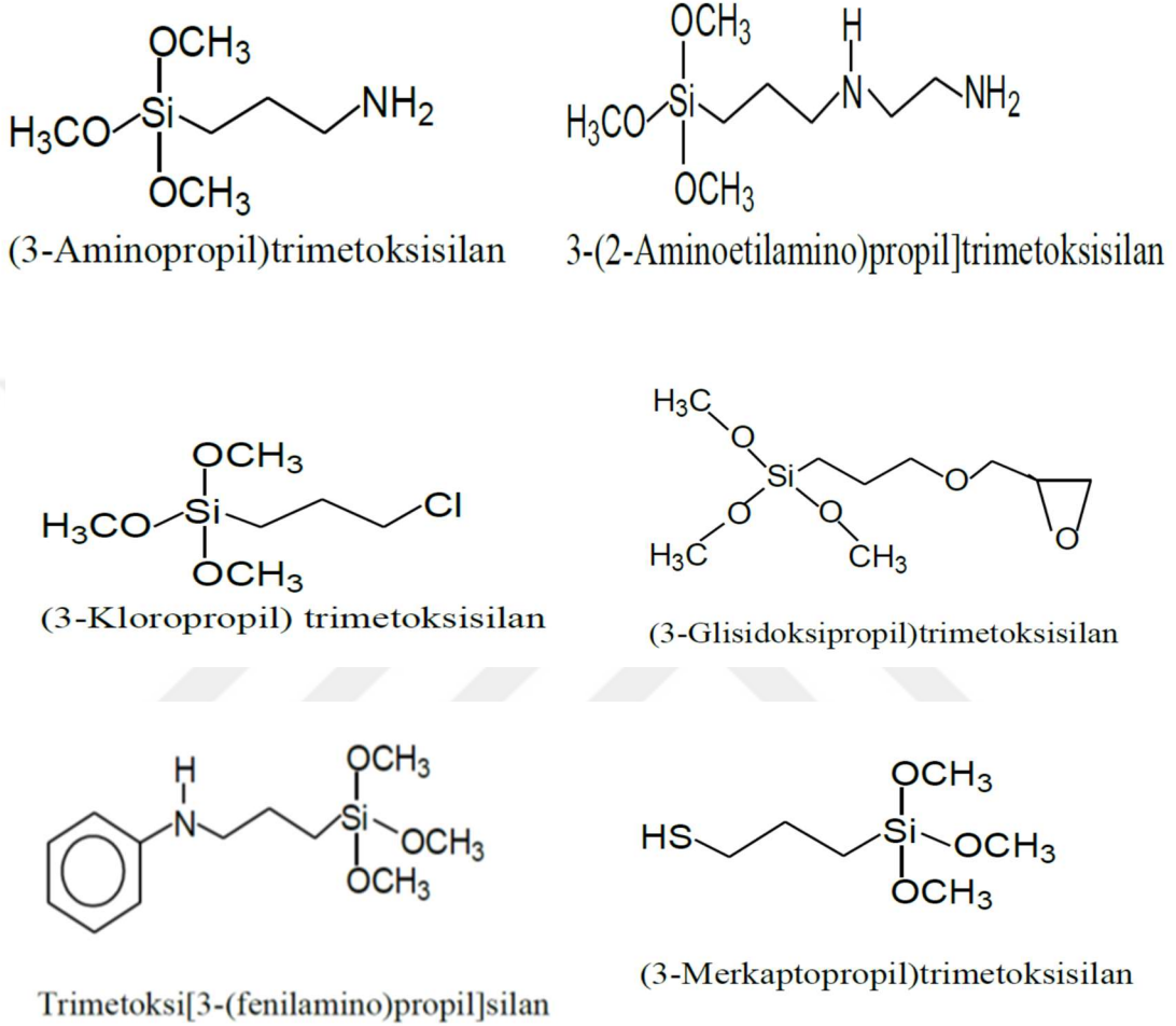
Şekil 2.7. Silanlama reaktifleri [39]
