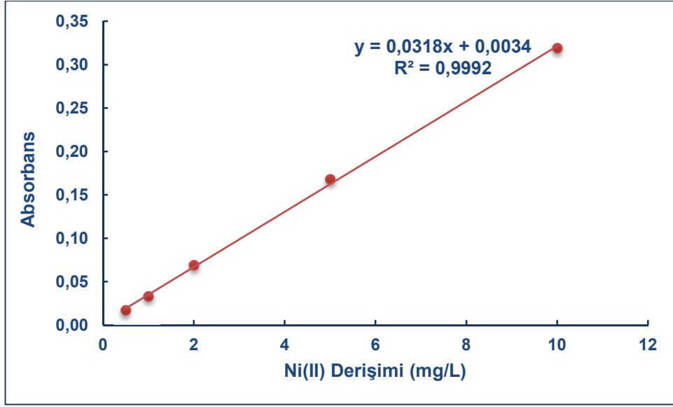
Şekil 5. Ni(II) iyonlarının tayininde kullanılan AAS'ye ait kalibrasyon grafiğı
