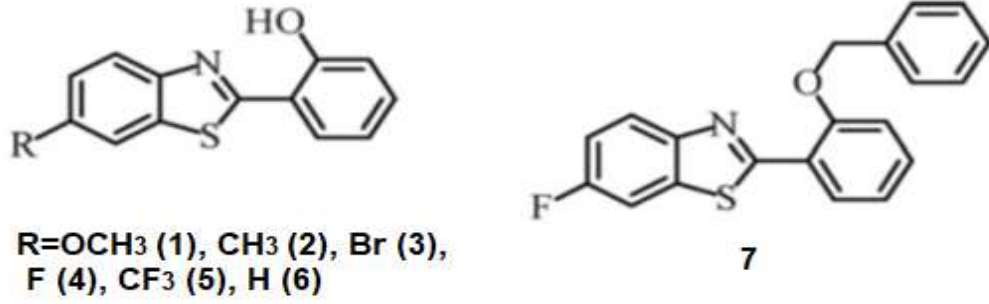
Şekil 2.23. 2-(2'-hidroksifenil)benzotiyazol türevleri
