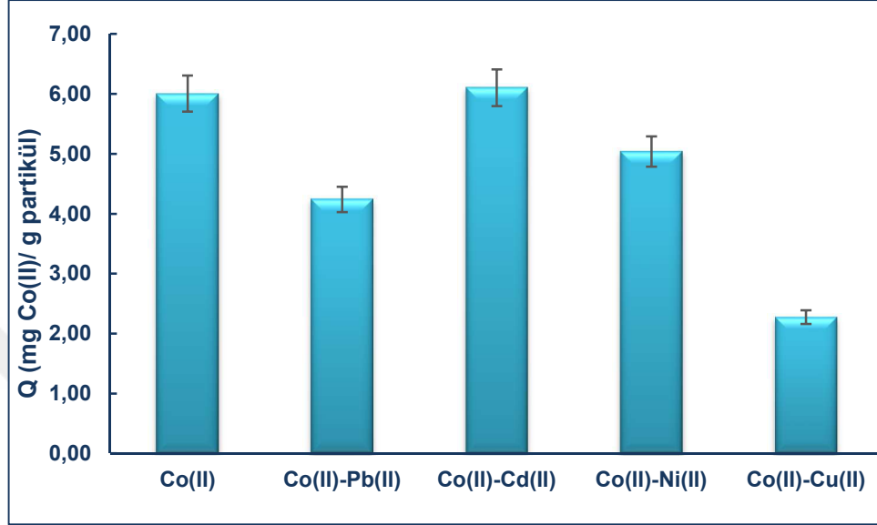
Şekil 4.37. Co(II) iyonlarının, Pb(II), Cd(II), Ni(II) ve Cu(II) iyonları ile ikili karışımlarının Si-L partiküllere yarışmalı adsorpsiyonu (Deney koşulları; Si-L miktarı: 0.020 g, metal iyon derişimi: 20 mg/L, pH:6, çözelti hacmi: 20 mL, karıştırma hızı: 400 devir/dk, karıştırma süresi: 120 dk, N=3)
