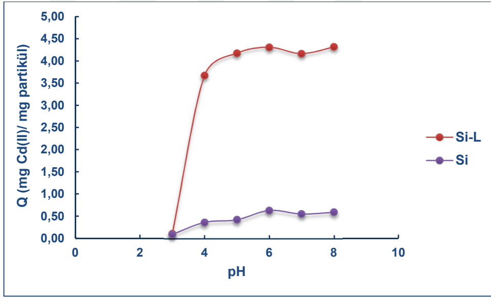
Şekil 4.19. Cd(II) adsorpsiyonuna pH'ın etkisi (Deney koşulları; Si-L miktarı: 0.020 g, Cd(II) derişimi: 5 mg/L, çözelti hacmi: 20 mL, karıştırma hızı: 400 devir/dk, karıştırma süresi: 120 dk)
