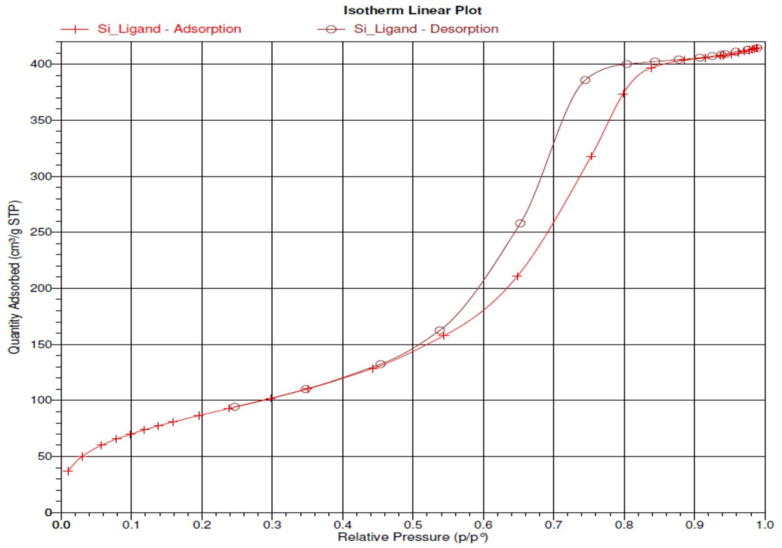
Şekil 4.8. (a) Silika partiküllere, (b) Si-L partiküllere ait N 2 adsorpsiyon-desorpsiyon izotermi
