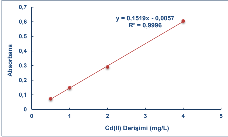
Şekil 3. Cd(II) iyonlarının tayininde kullanılan AAS'ye ait kalibrasyon grafiğı
