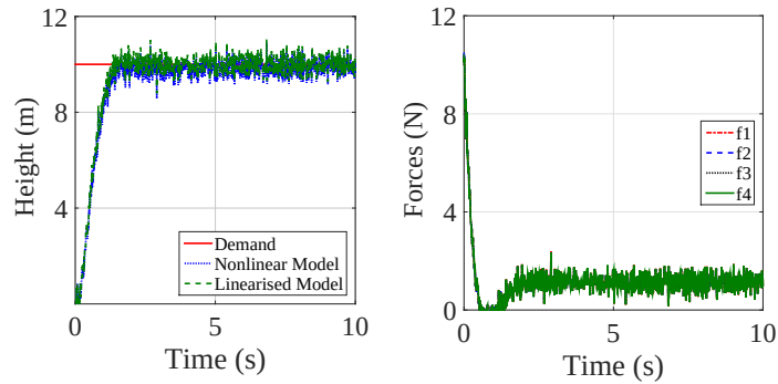
(d) Height position and corresponding motor forces.
