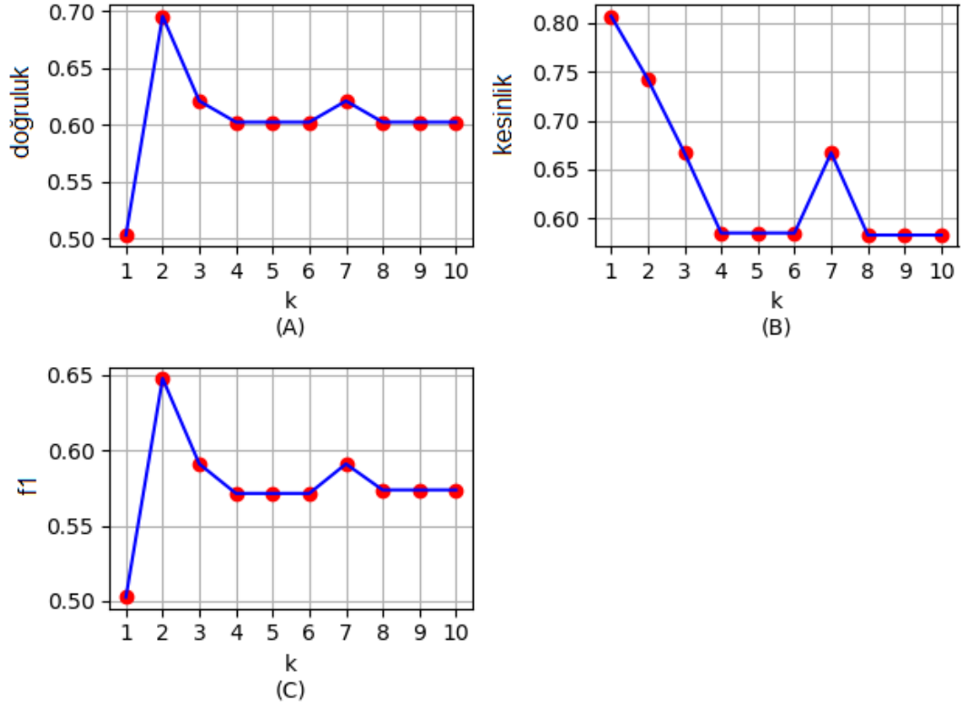
Şekil 4.8: Eğitim veri setinin C1 ve C2, özelliğın A4 olması durumunda, tahminleme başarıım ölçütlerinin ortalamasının k değeriıne göre değışimi, (A): doğruluk , (B): kesinlik , (C): f1
