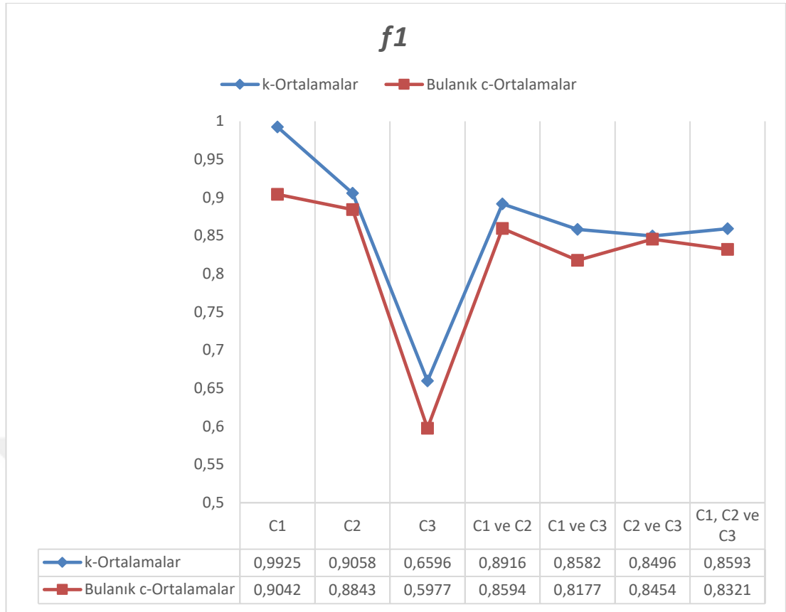
Şekil 4.21: C1, C2 ve C3 veri setlerinin farklı kombinasyonları için k -Ortalamlar ve Bulanık c -Ortalamlar yöntemleriyle elde edilen kümelemelerin karşılaştırmalı ortalama kesinlik değerleri
