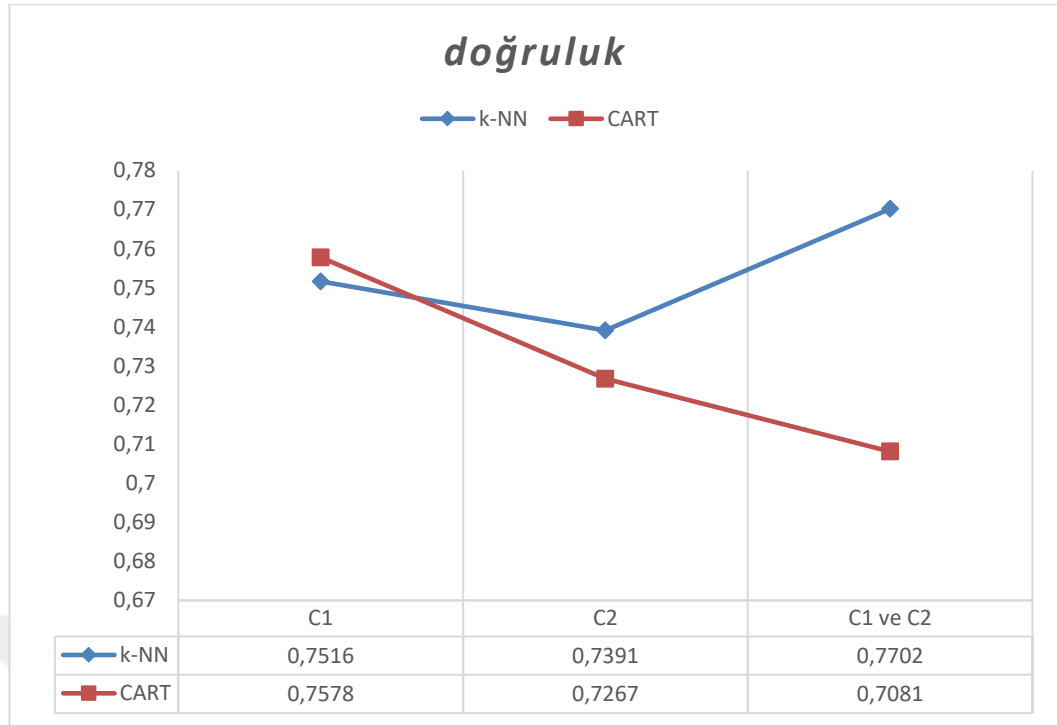
Şekil 4.16: Eğitim veri seti olarak yalnız C1, yalnız C2, C1 ve C2 seçilmesi durumunda k -NN ve karar ağacı yöntemleriyle elde edilen sınıflandırmaların karşılaştırmalı ortalama doğruluk değerleri
