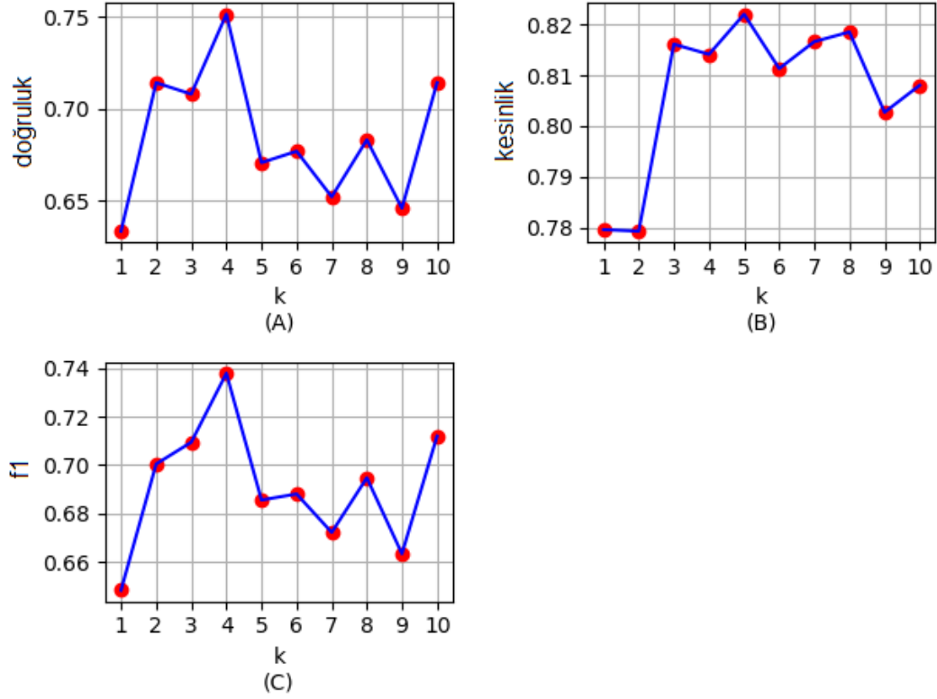
Şekil 4.1: Eğitim veri setinin C1, özelliklerin A3 ve A10 olması durumunda tahminleme başarımlarının k değerine göre değişimi, (A): dogruluk , (B): kesinlik , (C): f1
