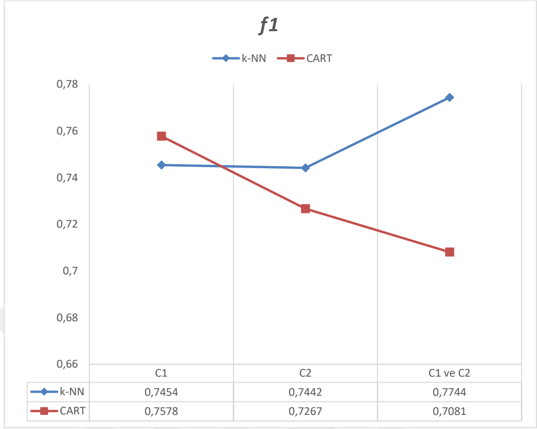
Şekil 4.18: Eğitim veri seti olarak yalnız C1, yalnız C2, C1 ve C2 seçilmesi durumunda k -NN ve karar ağacı yöntemleriyle elde edilen sınıflandırmaların karşılaştırmalı ortalama f1 değerleri
