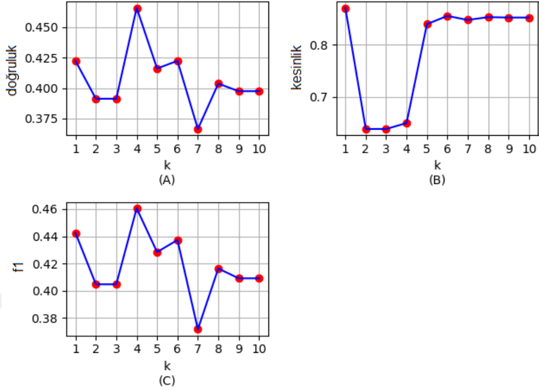
Şekil 4.2: Eğitim veri setinin C1, özelliklerin A2 ve A3 olması durumunda, tahminleme başarımlarının ortalama değerlerinin k değerine göre değişimi, (A): doğruluk , (B): kesinlik , (C): f1
