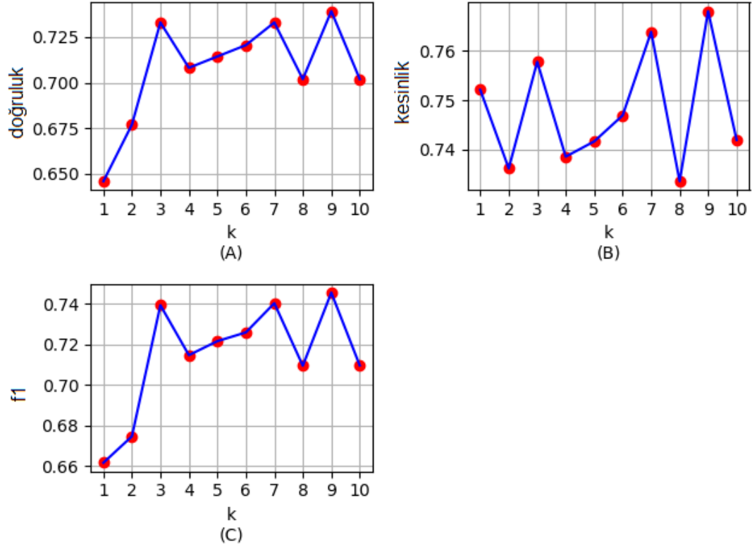
Şekil 4.3: Eğitim veri setinin C1, özelliklerin A10 ve A13 olması durumunda tahminleme başarımlarının k değerine göre değişimi, (A): doğruluk , (B): kesinlik , (C): f1
