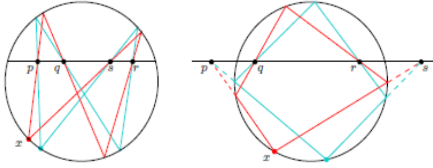
Şekil 4.2 Kirişler dörtgeni
