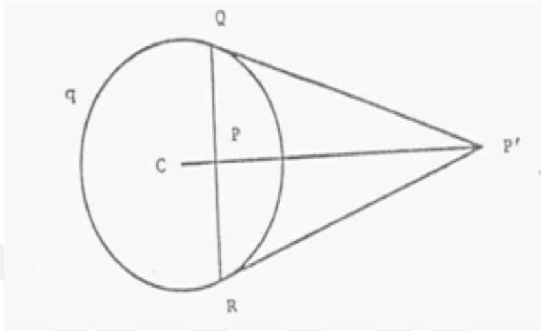
Şekil 2.1 İncersiyon
