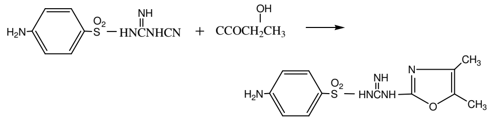
Sülfaguanol
