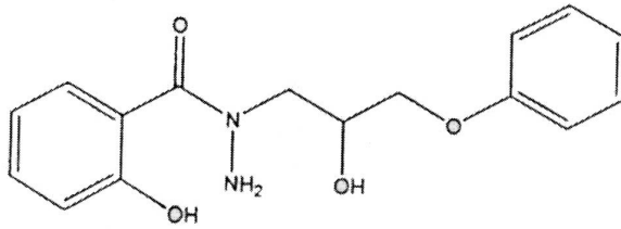
N-(2-hidroksibenzoil)-N'-(2-hidroksi-3- fenoksipropil)hidrazin
