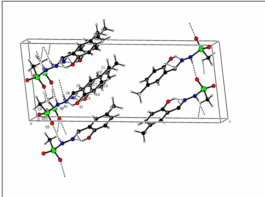
Şekil 5.2. Hidrojen bağları.
