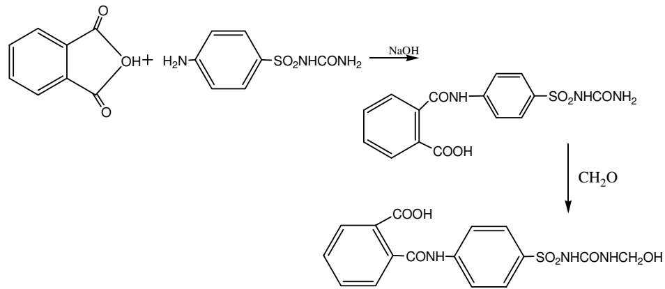
Sülfaloksik asit
