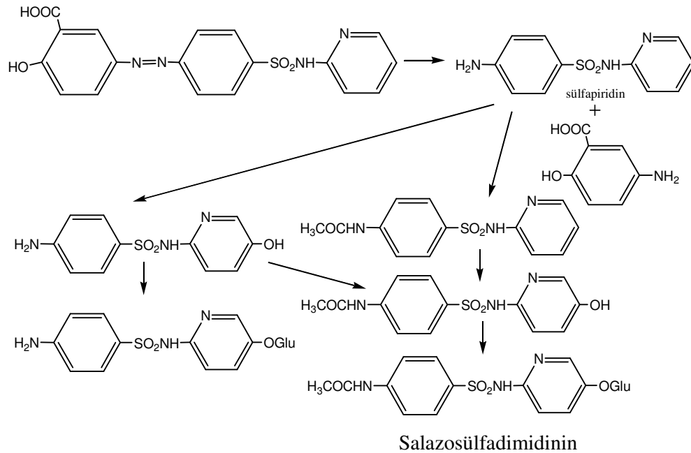
Şekil 2.4. Salazosülfadimidinin sentezi.
