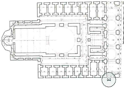
Plan 4.11 Hüdavendigar Cami Üst kat plan (Ayverdi, 1989)
