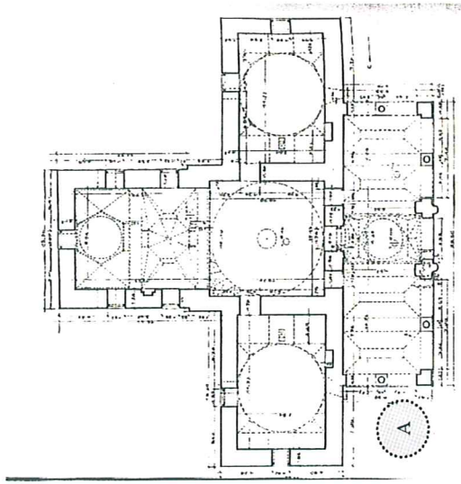
Plan 4.19 Nilüfer Hatun İmaretİ Plan (Ayverdi, 1972)
