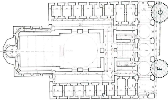
Plan 4.11 Hüdevendigar Cami Üst kat plan (Ayverdi, 1989)
