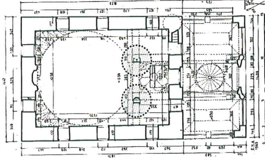
Plan 4.21 Yeşil Cami Planı (Ayverdi, 1972)
