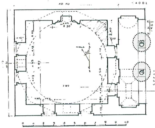
Plan 4.23 Hacı Özbek Camii Özgün Planı (Ayverdi, 1972)
