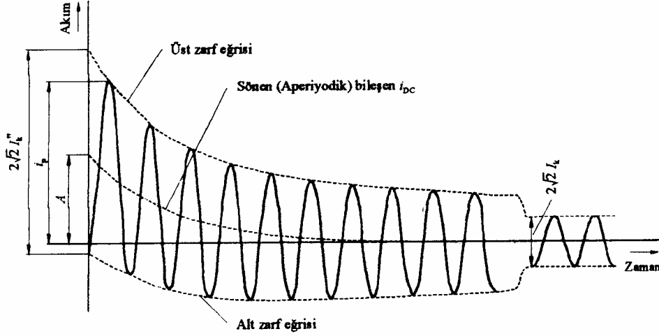
Şekil 2. 2 Generatörden yakı kısıadevrede kısıadevre akımı(Şematik çizim)
