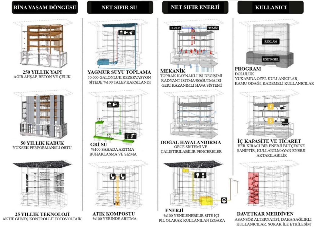
Şekil 3.20. The Bullitt Center taşıyıcı, su ve enerji sistemi (ArchDaily, 2013)
