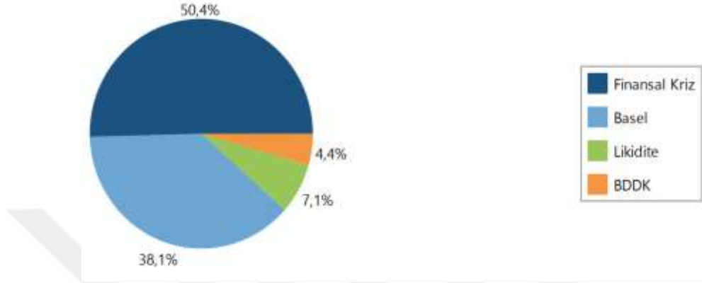
Grafik 3. Başlıklardaki Kelimelerin Dağılım Grafiği
